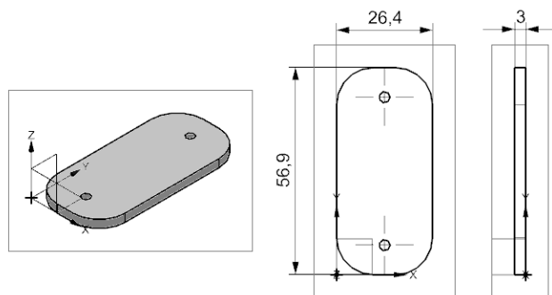
Figura 37. Tapa de la carcasa.
