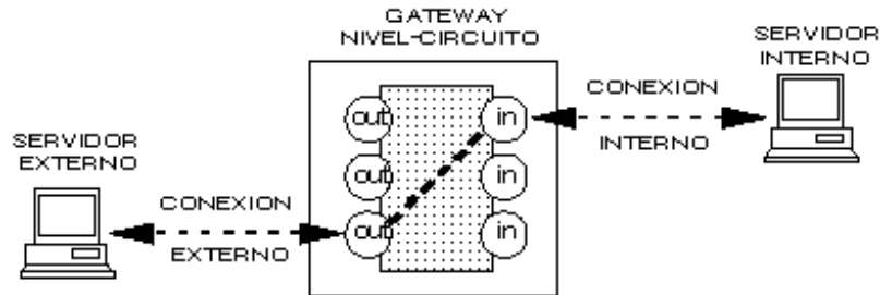
Fig. 4.9 Funcionamiento del gateway a nivel circuito
