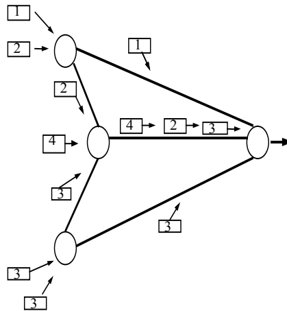
Fig. 1.17 Envío de paquete utilizando circuitos virtuales
