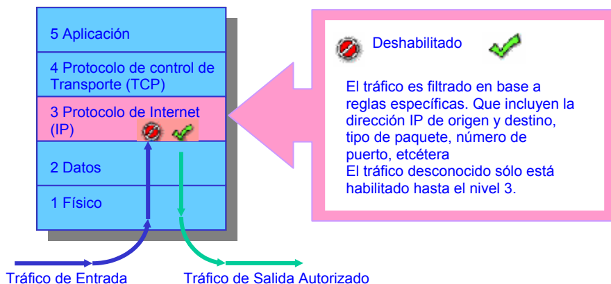
Fig. 4.4 Funcionamiento del “Firewall” Filtra-paquetes
