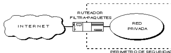
Fig. 4.5 Esquema de seguridad mediante un "Firewall" Filtra-paquetes
