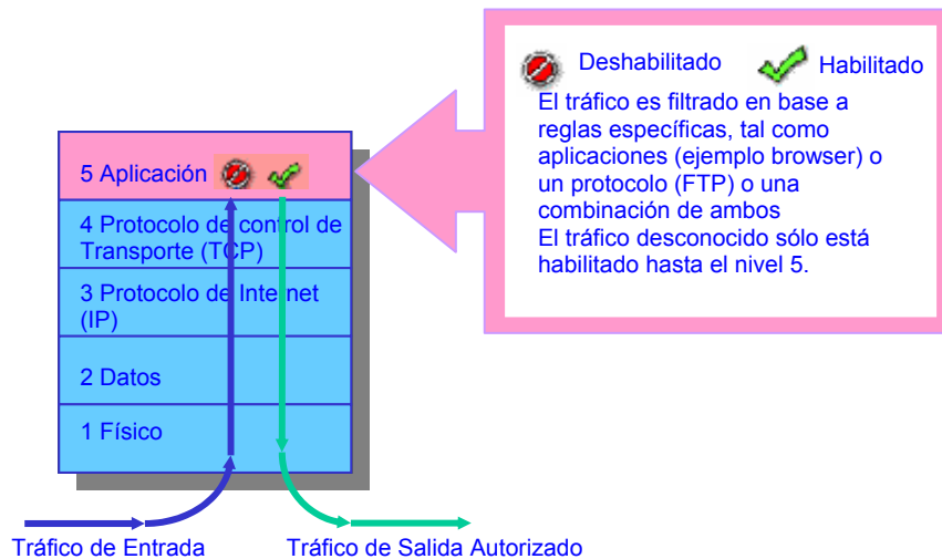
Fig. 4.6 Funcionamiento del Gateway a nivel aplicación
