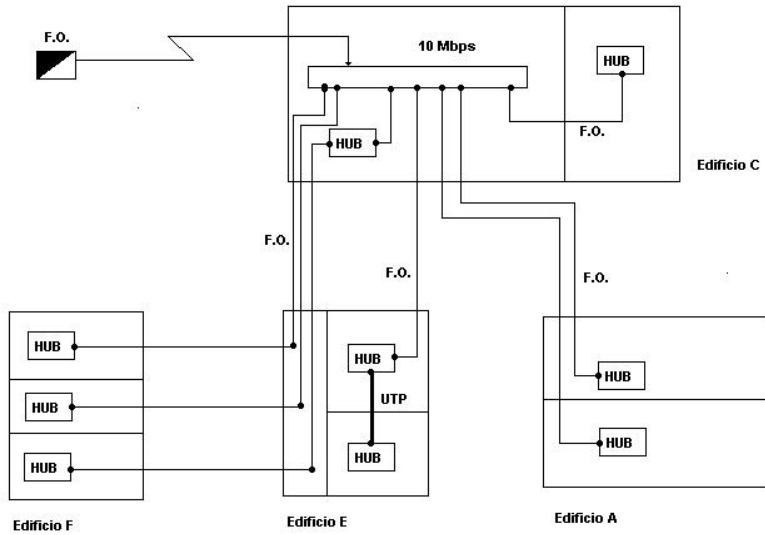
Figura V.3 Red existente y proyecto propuesto.
