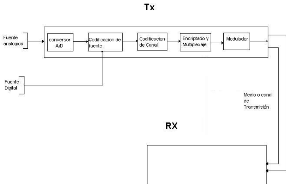
Figura 1.1 Sistema de comunicación digital.
