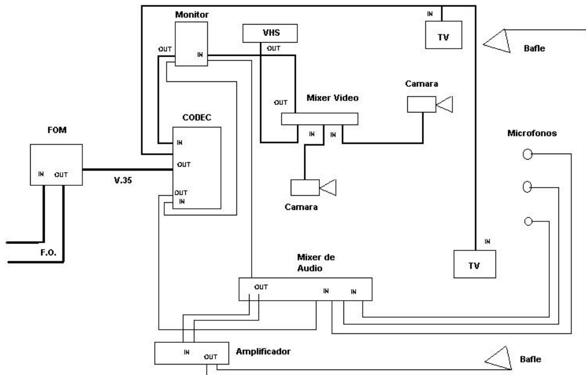
Figura VI.9 Diagrama de instalación del equipo de videoconferencia
