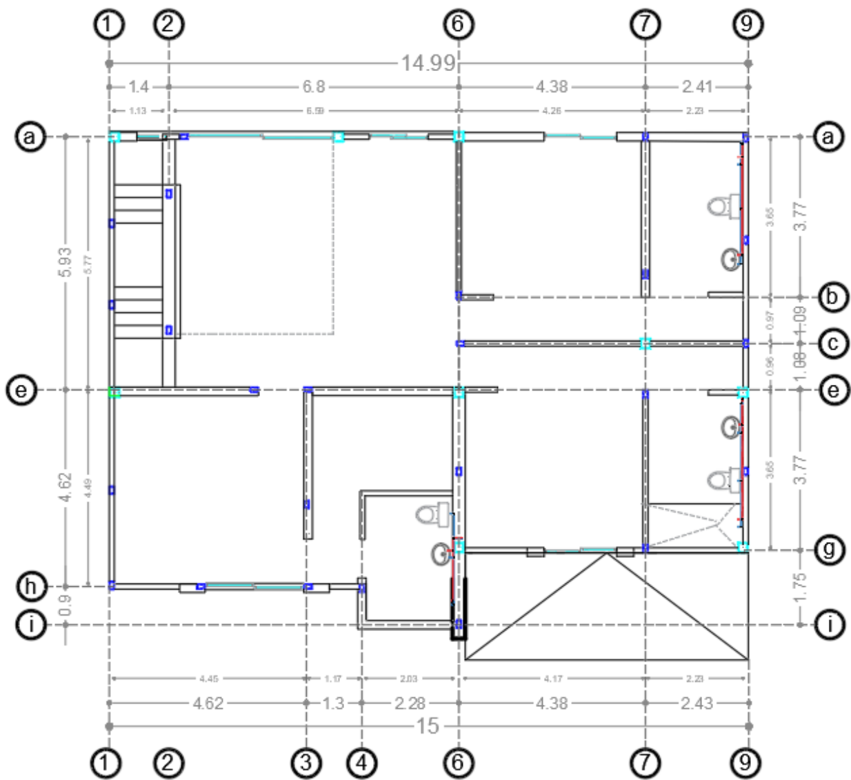
Ilustración 51 Plano hidráulico planta alta (Muciño, 2022)
