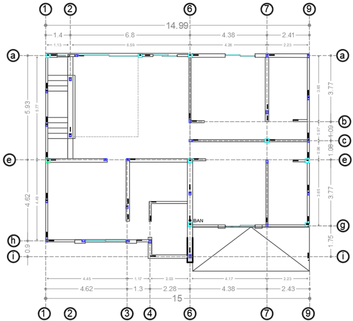
Ilustración 43 Planos Planta alta columnas, castillos (Muciño, 2022)
