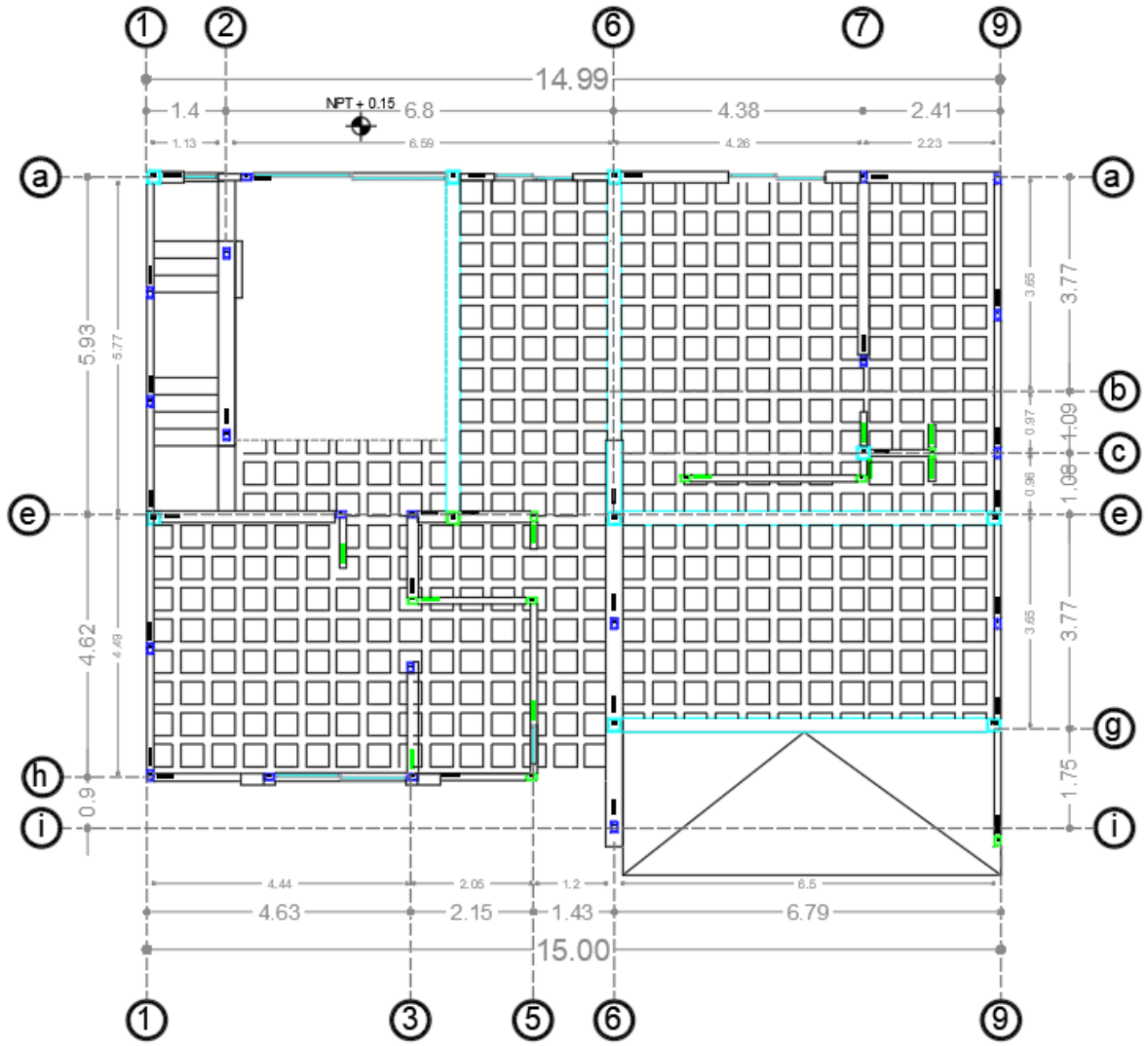
Ilustración 44 Losa reticular de entrepiso (Muciño, 2022)
