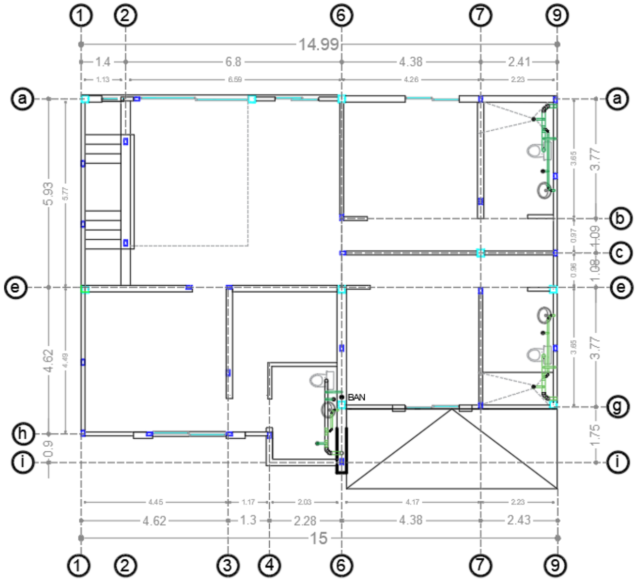
Ilustración 49 Plano sanitario planta alta (Muciño, 2022)
