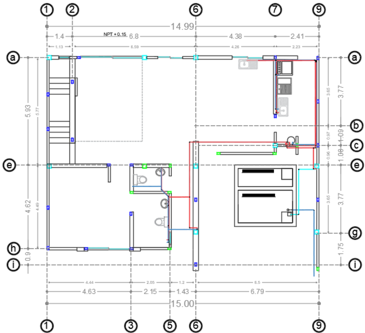
Ilustración 50 Plano hidráulico planta baja (Muciño, 2022)
