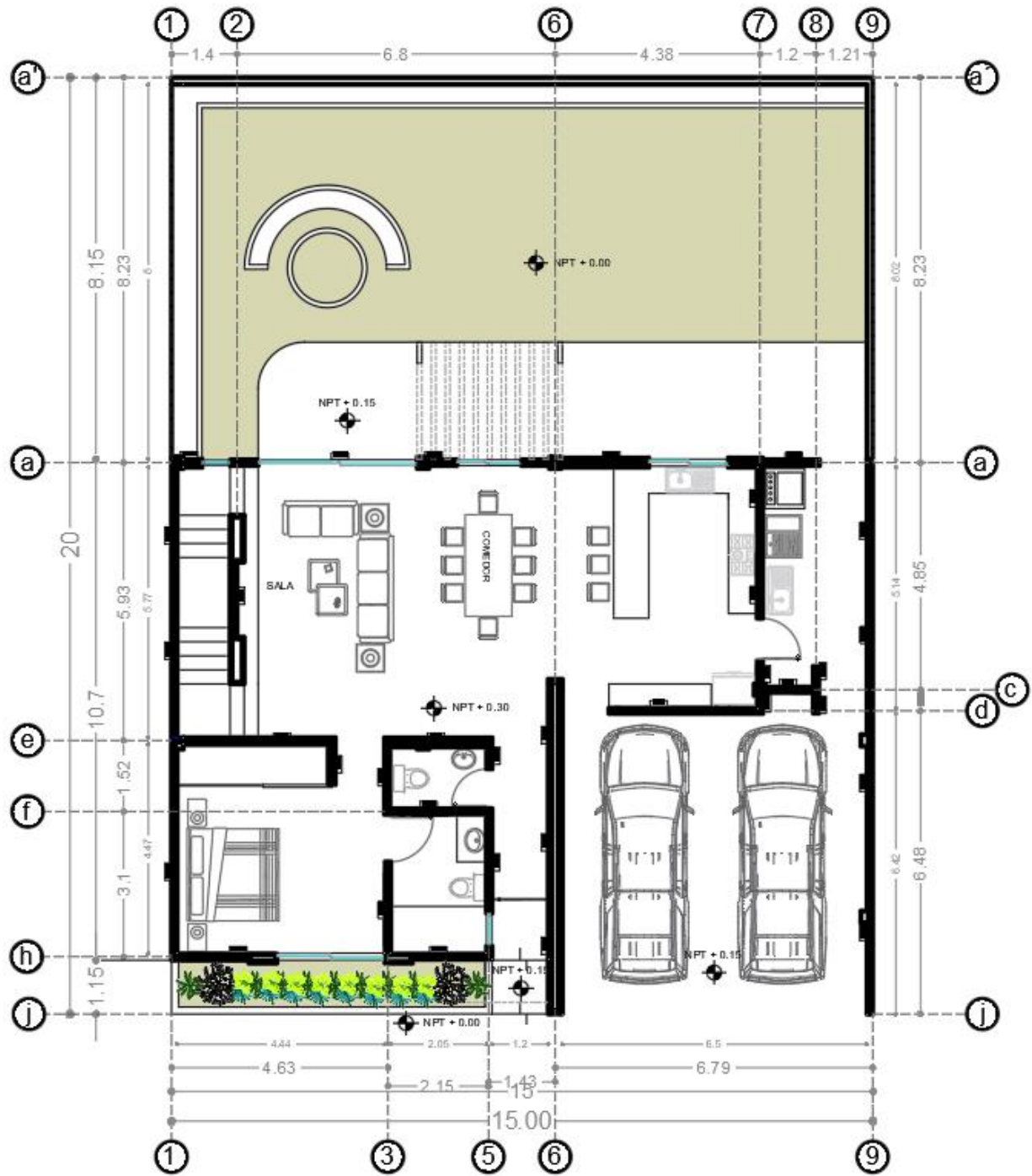
Ilustración 19 Planta baja "mi casa ecológica" (Muciño, 2022)
