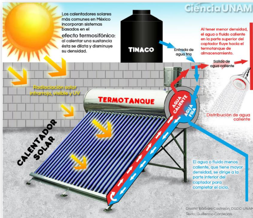
Ilustración 13 Calentador solar (UNAM, 2018)
