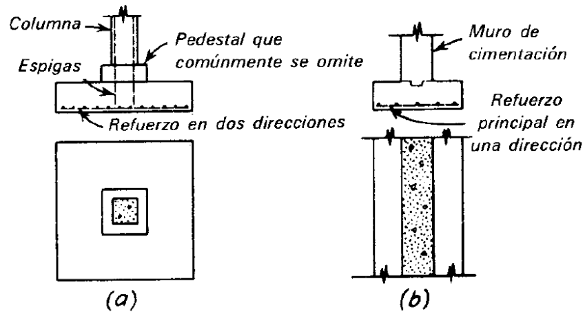
Ilustración 32 a) zapata aislada b) zapata corrida (PECK)
