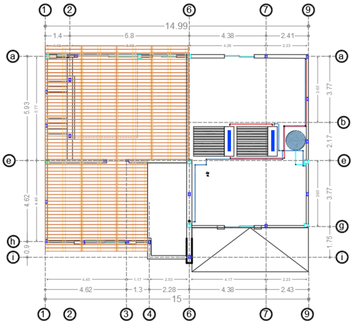
Ilustración 52 Plano hidráulico azotea (Muciño, 2022)
