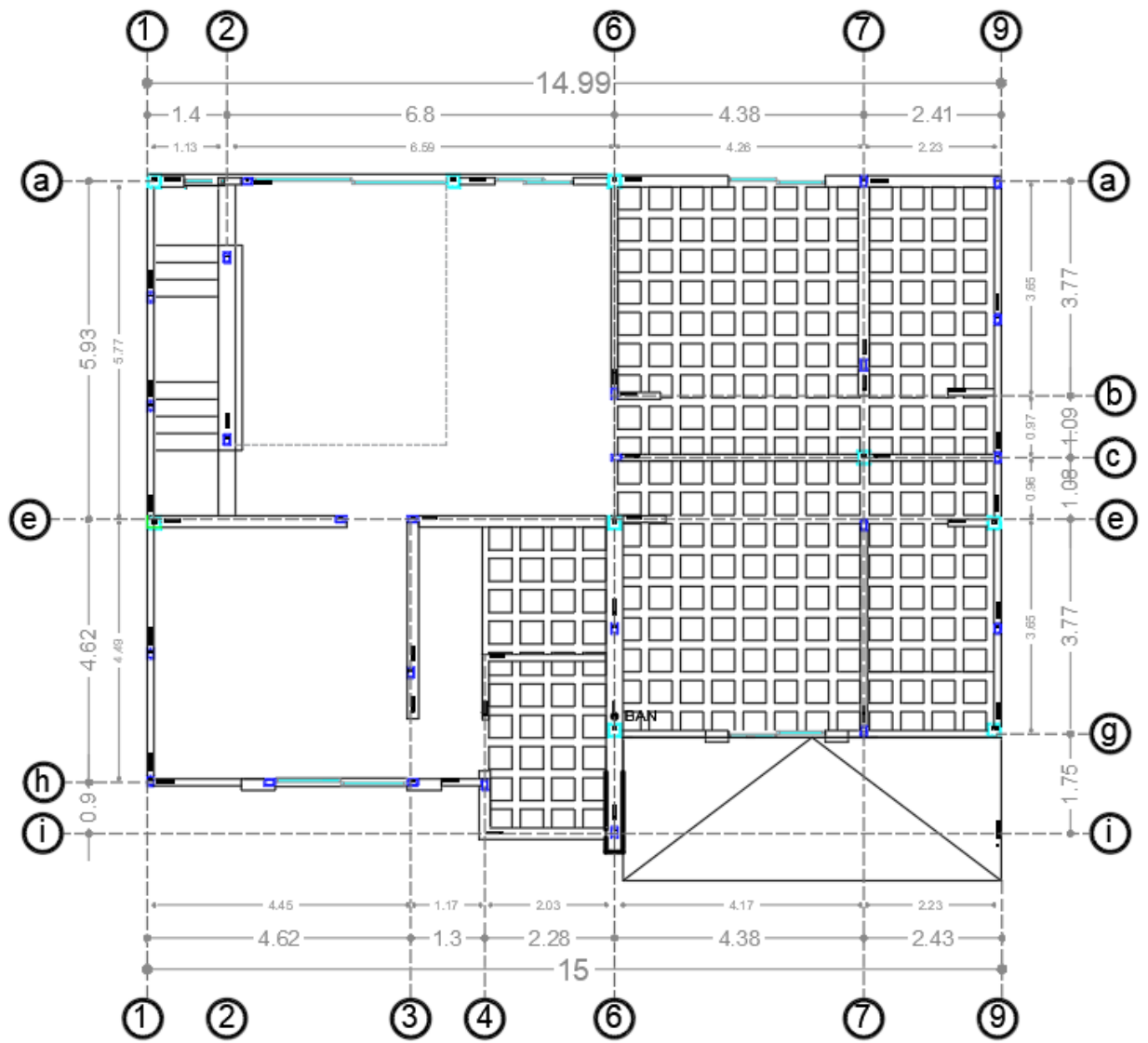
Ilustración 45 Losa aligerada de azotea, (Muciño, 2022)
