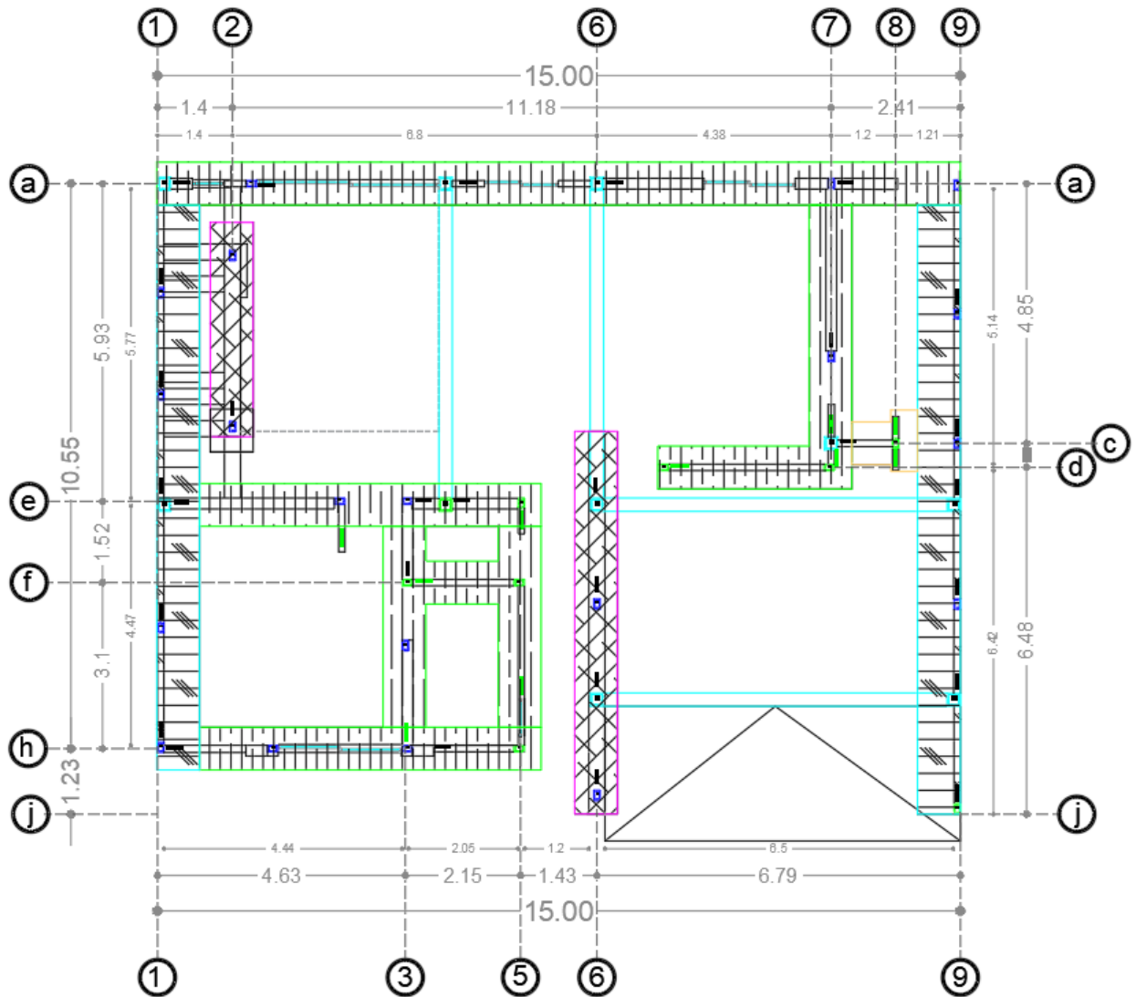
Ilustración 41 Plano de Cimentación (Muciño, 2022) (Zapatas corridas de mampostería de piedra).
