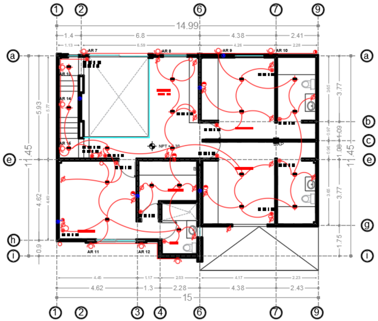
Ilustración 54 Plano eléctrico planta alta (Muciño, 2022)
