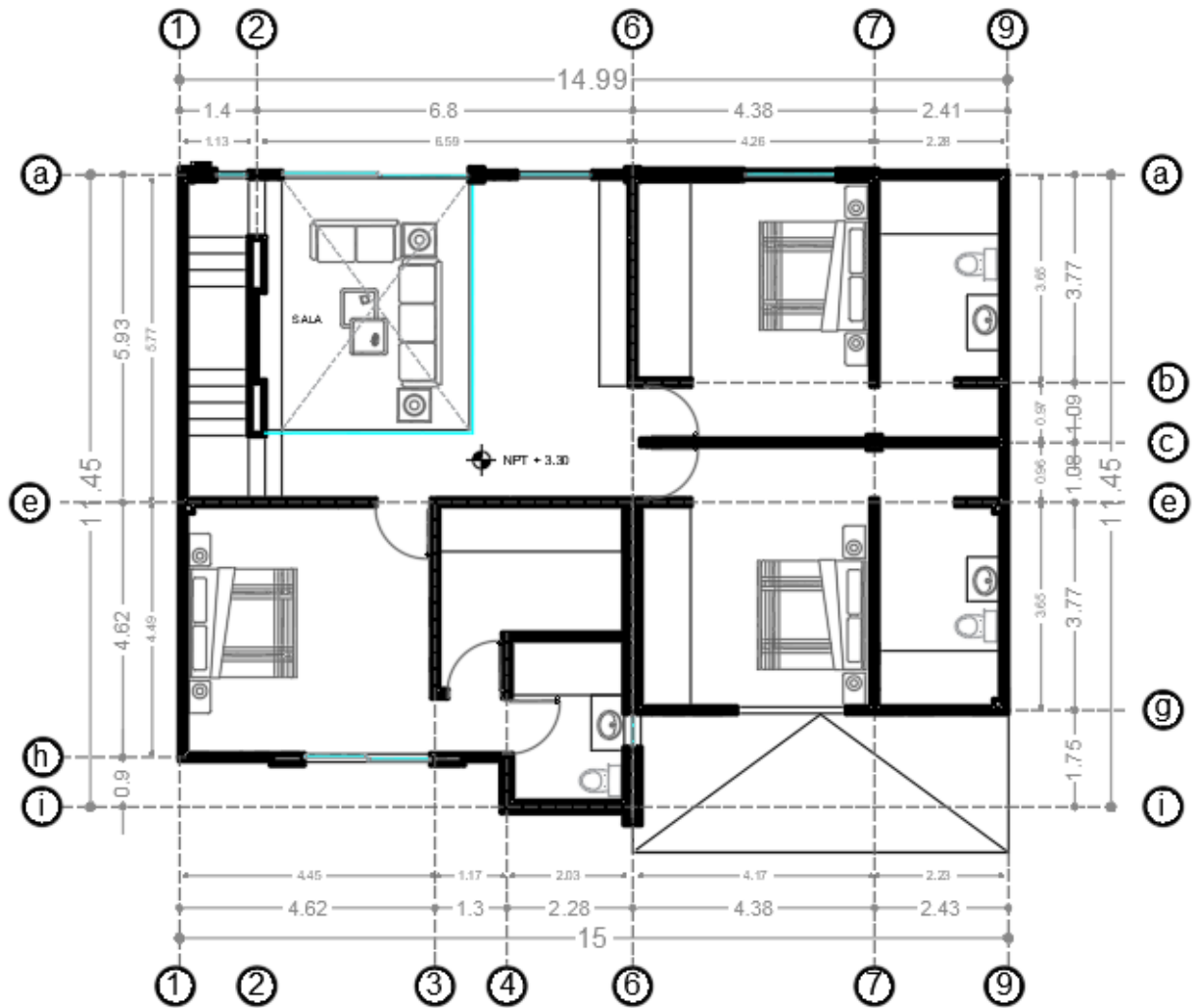
Ilustración 20 Planta alta "mi casa ecológica" (Muciño, 2022)
