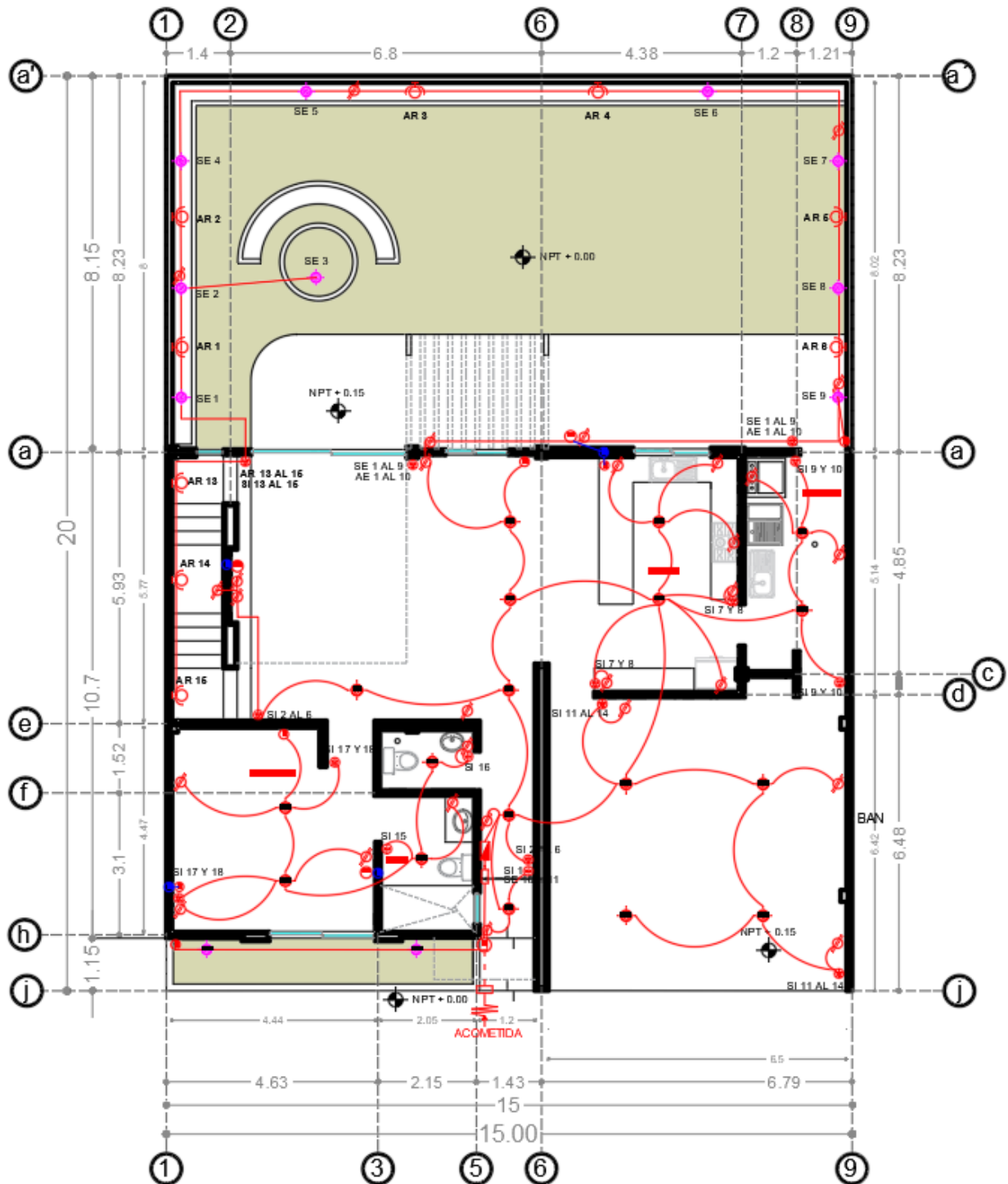
Ilustración 53 Plano eléctrico planta baja (Muciño, 2022)
