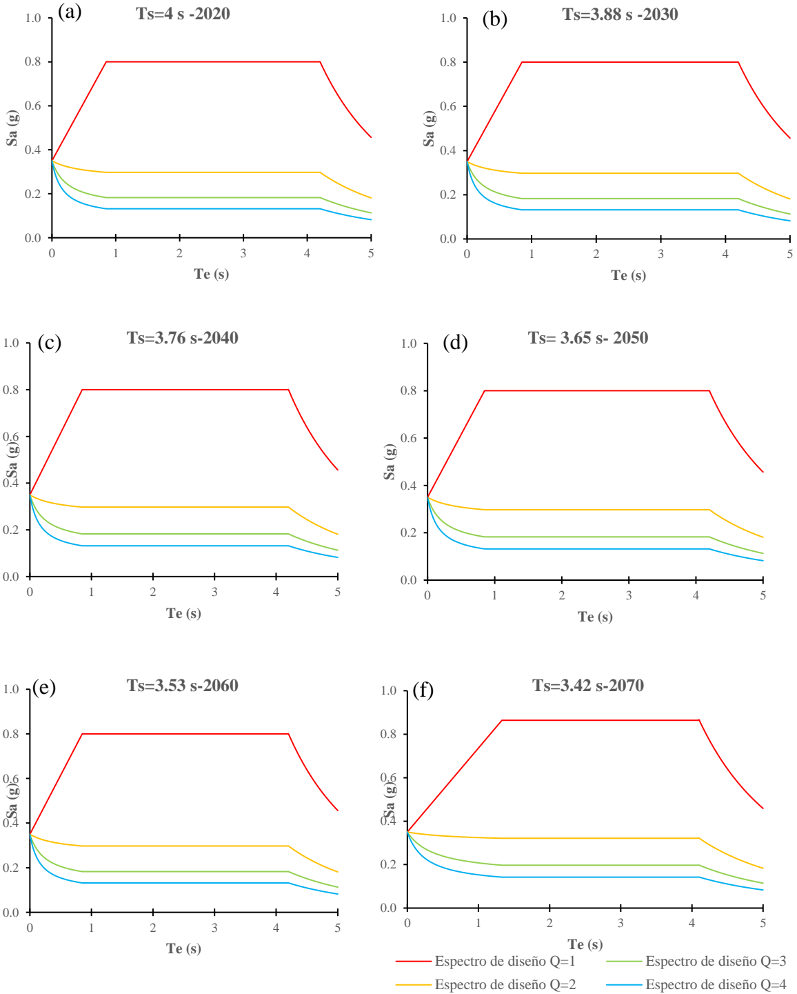
Figura 23. Cálculo de los espectros de diseño con Q=1, Q=2, Q=3 y Q=4 considerando la evolución del T_s en un periodo de 50 años (a) Espectros en el año 2020 con T_s=4 s, (b) Espectros en el año 2030 con T_s=3.88 s, (c) Espectros en el año 2040 con T_s=3.76 s, (d) Espectros en el año 2050 con T_s=3.65 s, (e) Espectros en el año 2060 con T_s=3.53 s y (f) Espectros en el año 2070 con T_s=3.42 s
