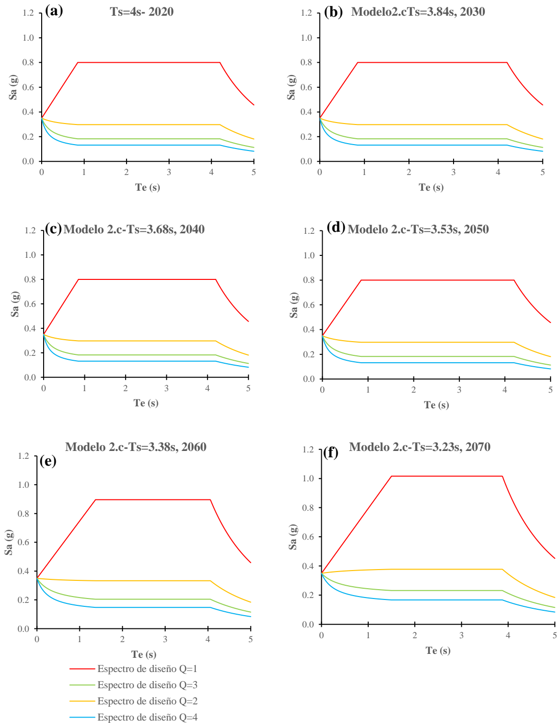
Figura 50. Cálculo de los espectros de diseño con Q=1, Q=2, Q=3 y Q=4 considerando la evolución del T_s y el cambio de V_s para el Modelo 2.c (a) Espectros en el año 2020 con T_s=4s , (b) Espectros en el año 2030 con T_s=3.84s , (c) Espectros en el año 2040 con T_s=3.68s , (d) Espectros en el año 2050 con T_s=3.53s , (e) Espectros en el año 2060 con T_s=3.38s y (f) Espectros en el año 2070 con T_s=3.23s
