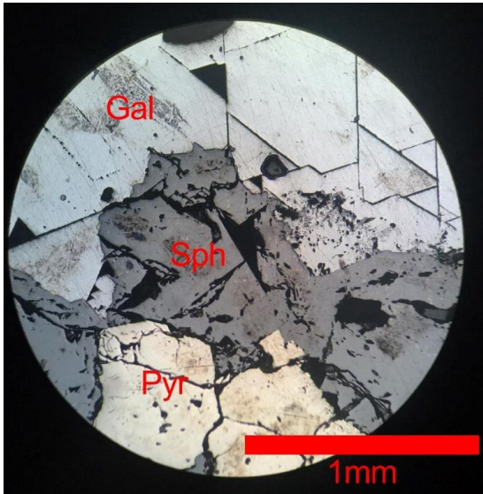
Fig. 81 (10x). Intercrecimiento entre la pirita, esfalerita y galena. Se alcanzan a distinguir pequeñas emulsiones de calcopirita en la esfalerita y la traza bien definida del crucero octaédrico en la galena.
