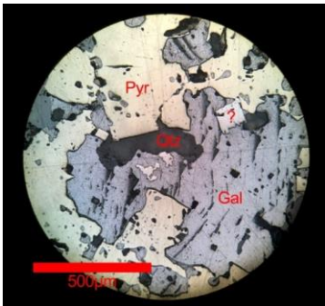
Fig. 73 (20x) Intercrecimiento de galena con un mineral más claro, siempre en las cercanías de cristalizaciones de cuarzo.
