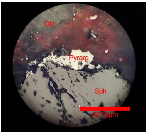
Fig. 67 (32x). Inclusiones elongadas de pirargirita en las cristalizaciones de esfalerita.
