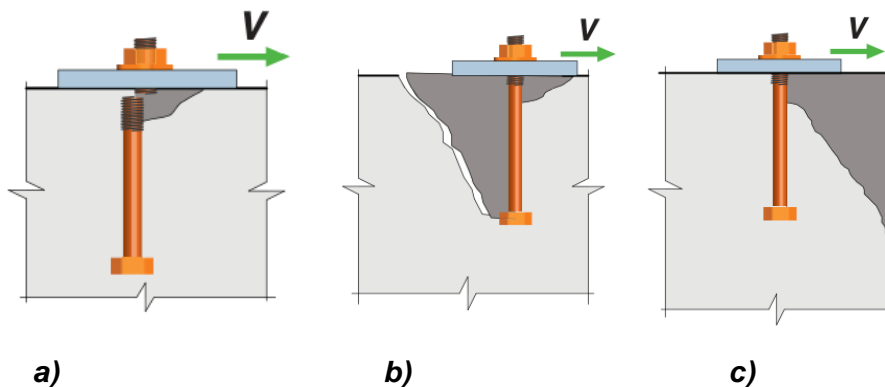
Figura 4.4.1 Mecanismos de falla de las anclas por cortante: a) resistencia a cortante del acero del ancla, b) rotura posterior del concreto y c) rotura del concreto (corte) (ACI 318)
