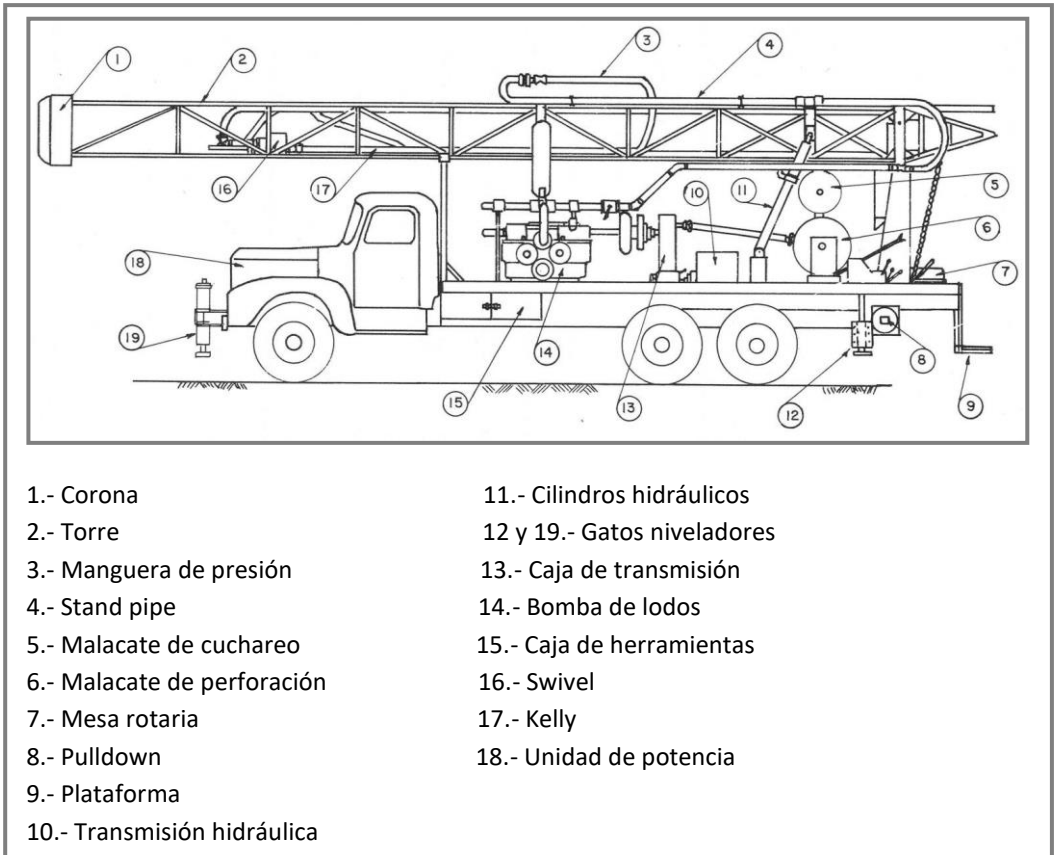
Ilustración 20 Componentes del equipo de perforación con sistema rotario. Fuente: Elaboración propia.
