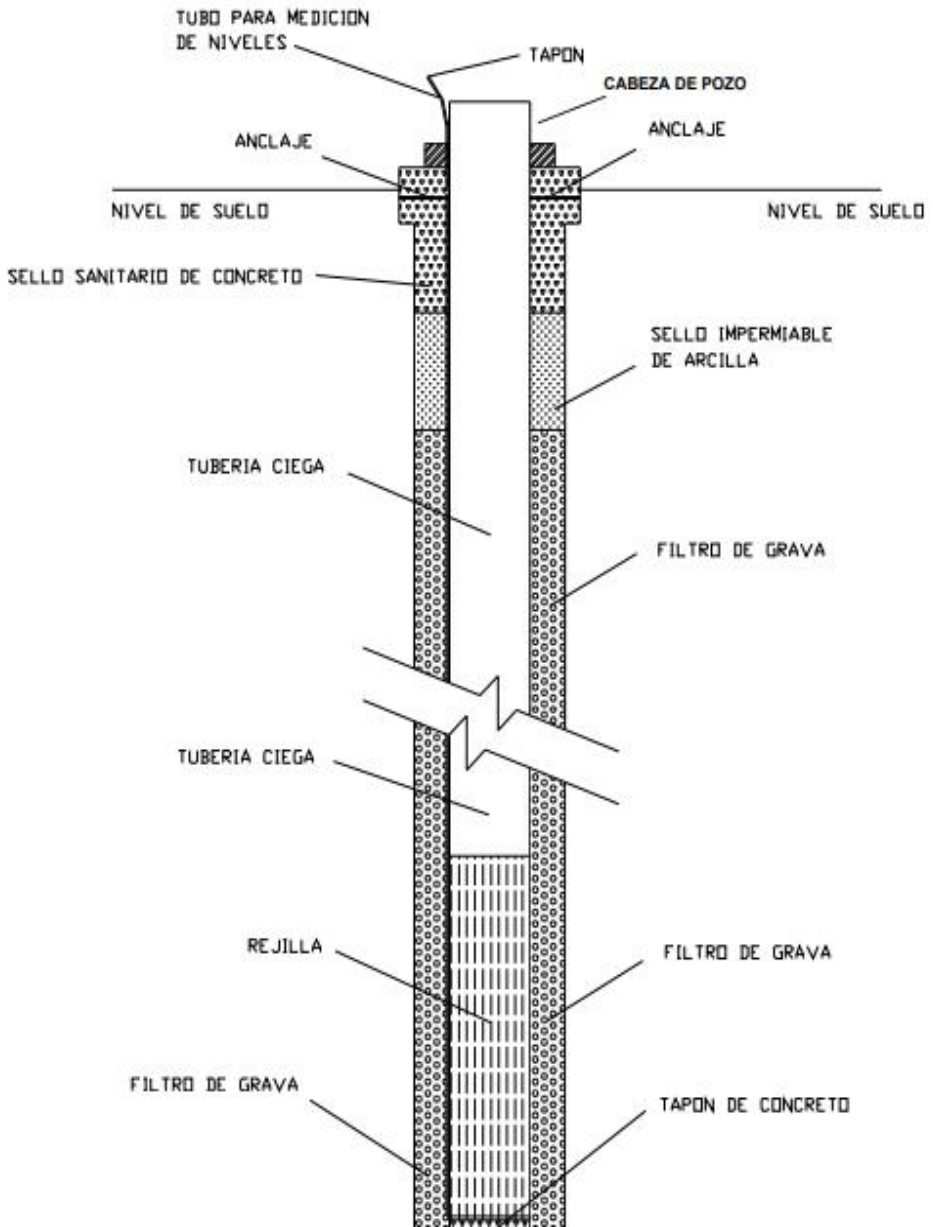
Ilustración 8 Componentes de un pozo terminado. Fuente: NORMA TECNICA PARA LA PERFORACIÓN DE POZOS PROFUNDOS EN LA ADMINISTRACIÓN NACIONAL DE ACUEDUCTOS Y ALCANTARILLADOS.
