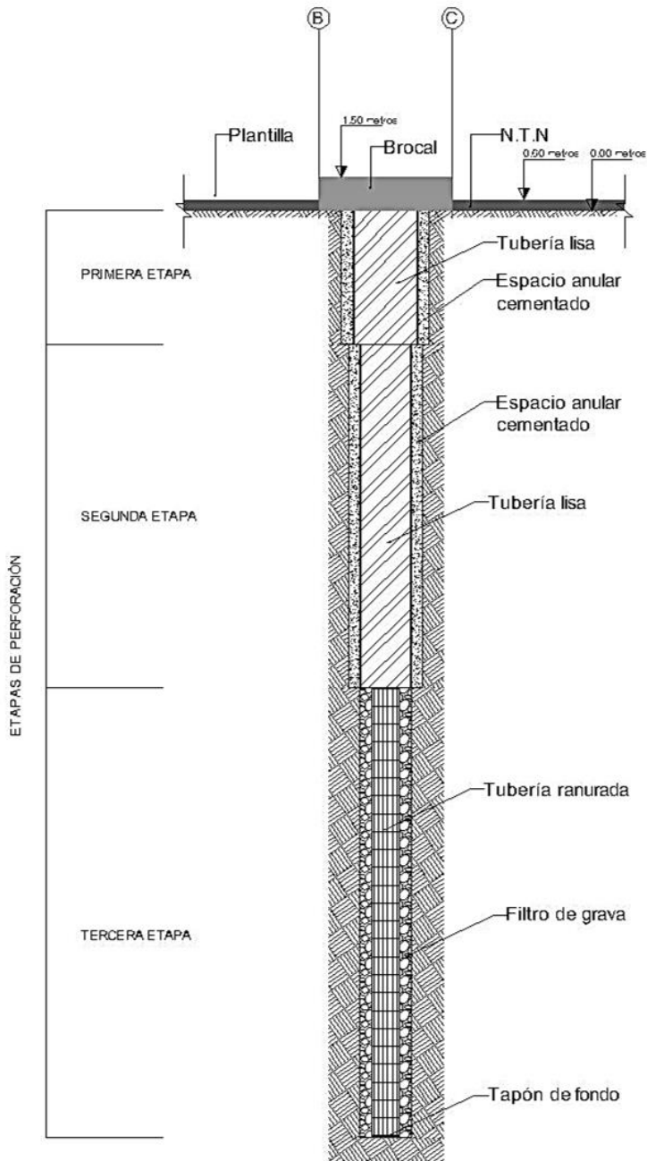
Ilustración 11 Representación de los componentes del pozo Fuente: Elaboración propia
