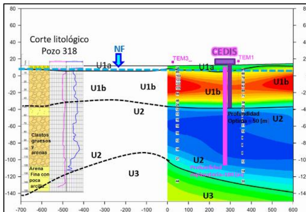
Ilustración 4 Ejemplo del comportamiento eléctrico en un corte litológico. Fuente: Registro eléctrico GEOTEM Ingeniería S.A. de C.V.
