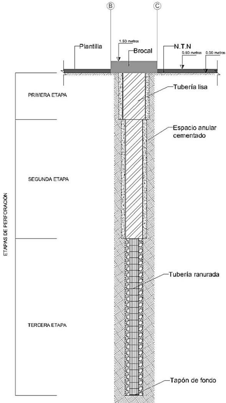
Ilustración 10 Representación de las etapas de perforación Fuente: Elaboración propia.
