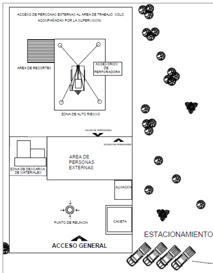
Ilustración 63 Croquis de la distribución de zonas en el sitio de los trabajos. Fuente: Elaboración propia.
