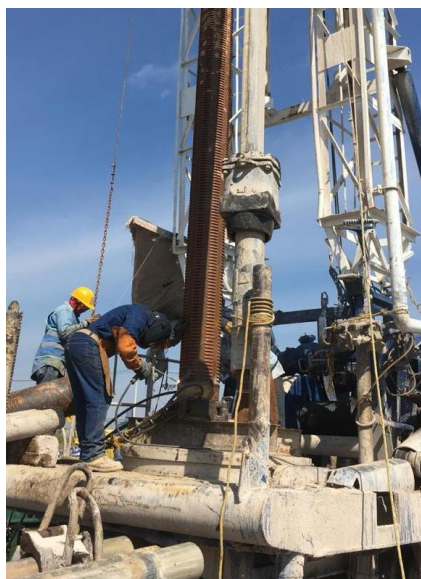
Ilustración 56 Colocación de tubería ranurada. Fuente: Elaboración propia.
