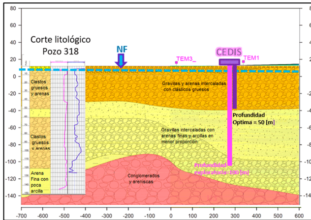
Ilustración 5 Ejemplo del comportamiento eléctrico en un corte litológico. Fuente: Registro eléctrico GEOTEM Ingeniería S.A. de C.V.
