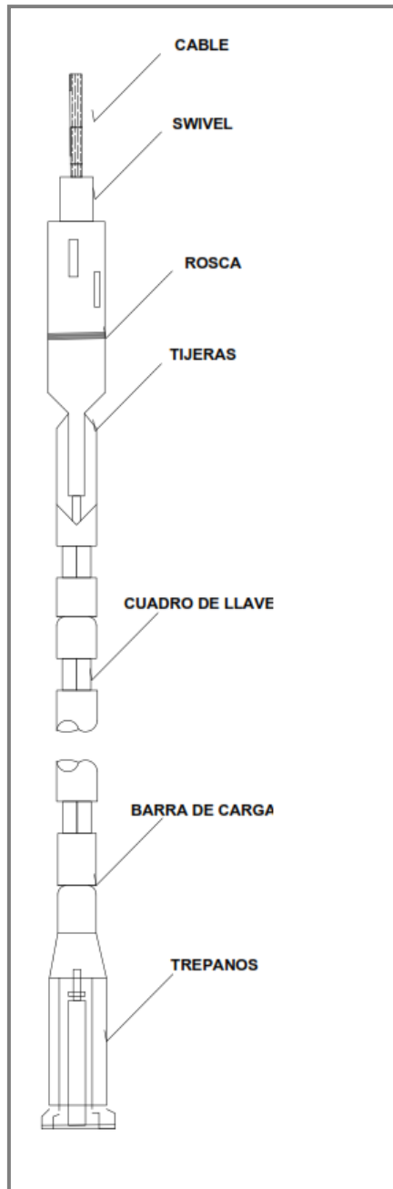
Ilustración 14 Equipo de percusión. Componentes de la sarta de perforación. Fuente: Elaboración propia.
