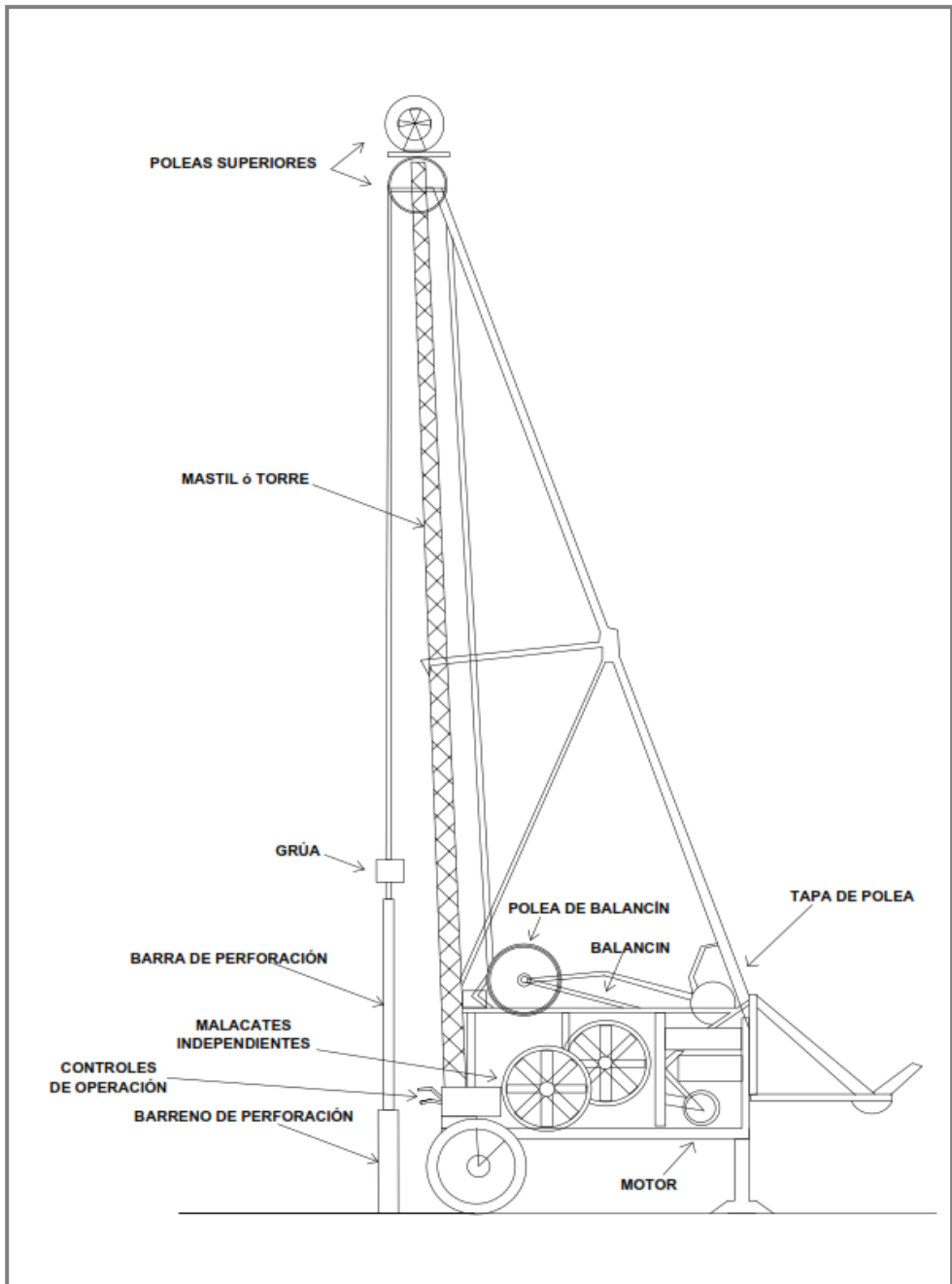
Ilustración 13 Equipo de perforación de tipo percusión. Fuente: Elaboración propia.
