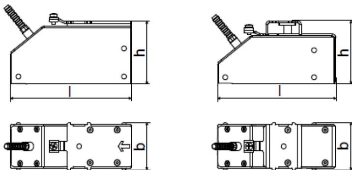
Ilustración 28. Transductores ultrasónicos usados comúnmente para la medición de Gas.
