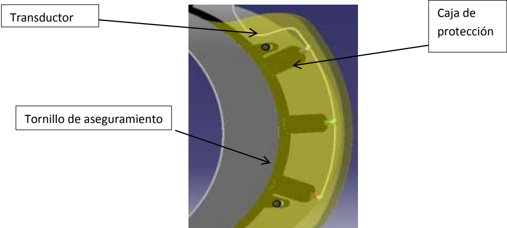
Ilustración 61. Estructura de propuesta de Medidor
