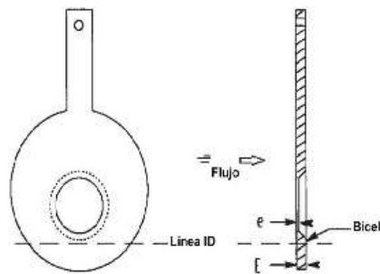
Ilustración 16. Orificio Excéntrico.
