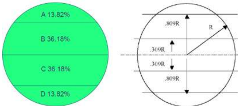
Ilustración 58. Porcentajes de flujo por área.
