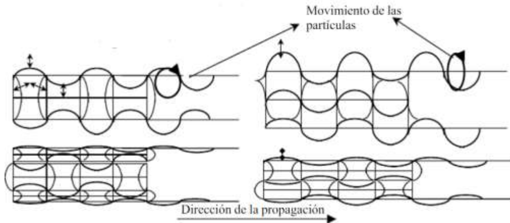
Ilustración 42. Ondas simétricas de compresión asimétricas de flexión.
