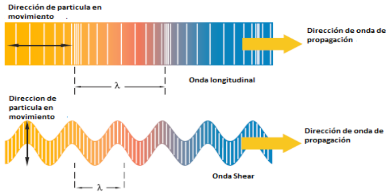
Ilustración 21. Propagación de Ondas para medición ultrasónica.
