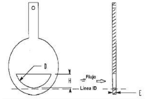
Ilustración 17. Orificio Segmentado.
