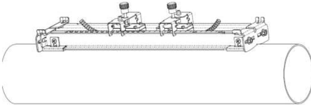
Ilustración 53. Sujetadores portátiles con imán
