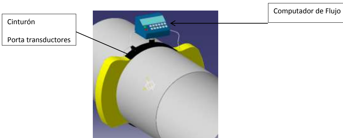
Ilustración 62. Modelo propuesta de Medidor Ultrasonico de fijación externa para la Medición de Flujo de Gas.
