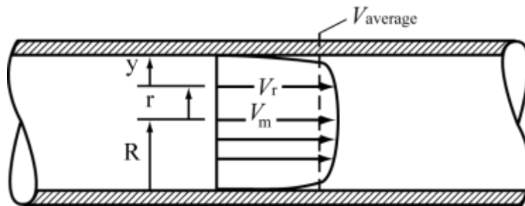
Ilustración 34. Flujo turbulento
