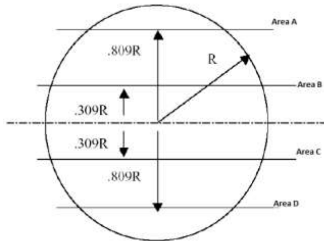
Ilustración 57. Secciones de área total de flujo.
