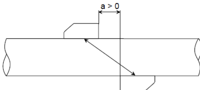
Ilustración 50. Disposición diagonal, número de trayectos del sonido: 1
