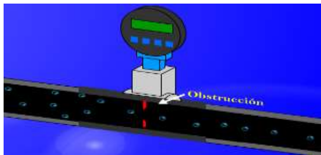
Ilustración 14. Medidor Placa de Orificio
