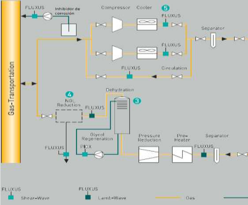
Ilustración 29. Diagrama de medición interna. Fuente Flexim.
