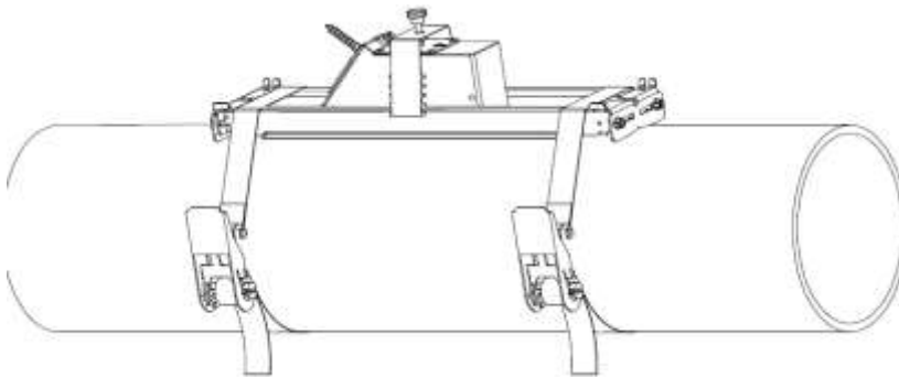
Ilustración 54. Sujetadores portátiles y correas de sujeción
