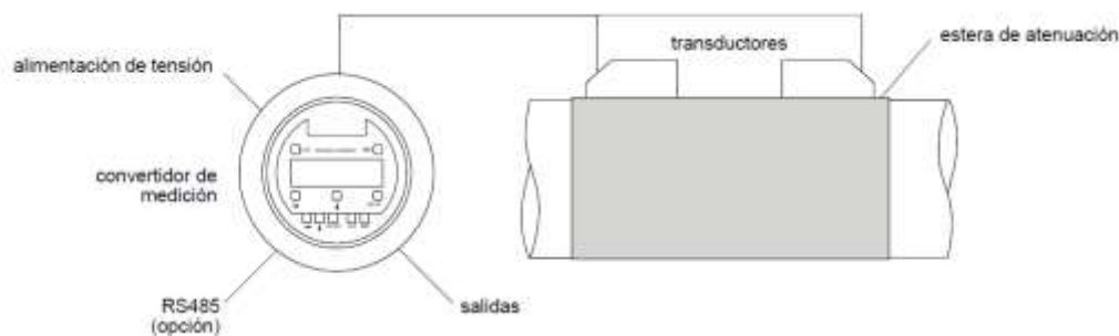
Ilustración 39. Configuración de los elementos de medidor de fijación externa.
