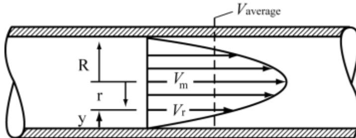
Ilustración 33. Perfil de flujo laminar
