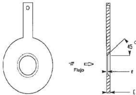
Ilustración 15. Orificio Concéntrico
