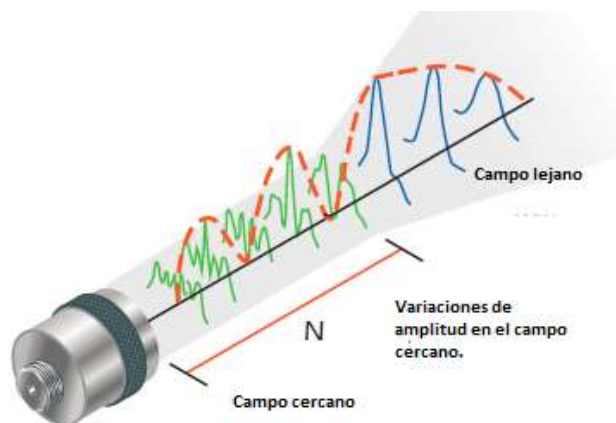
Ilustración 23. Variaciones de Amplitud.
