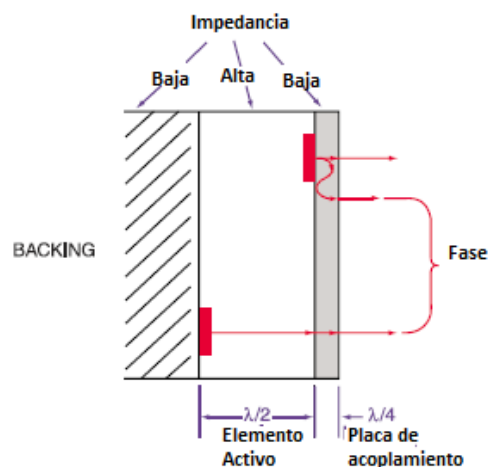
Ilustración 45. Diagrama del Backing o contramasa.
