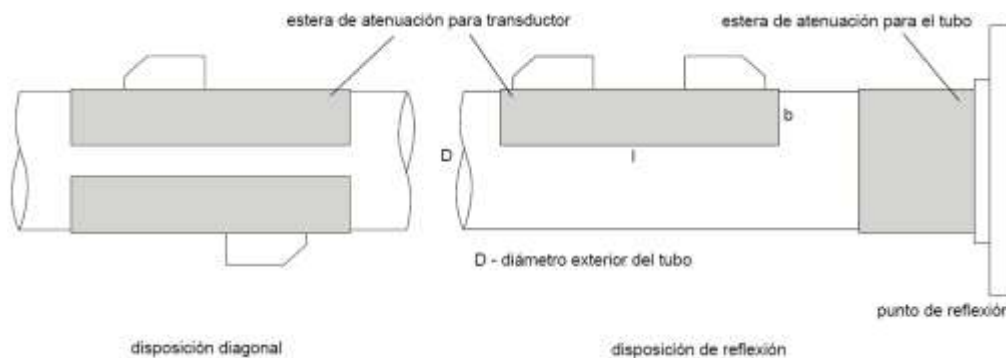
Ilustración 55. Colocación de las esferas de atenuación.
