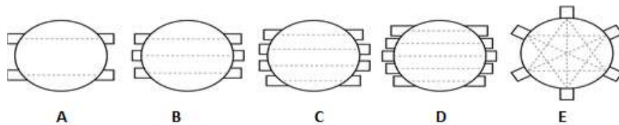
Ilustración 27. Diagramas de múltiples trayectorias de Ases.
