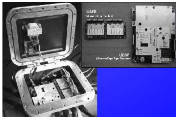
Ilustración 19. Partes eléctricas de Medidor Ultrasónico de Inserción.
