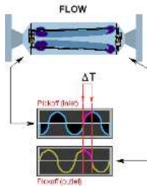
Ilustración 12. Bobina con flujo (Vista frontal).
