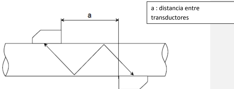
Ilustración 49. Disposición diagonal, número de trayectos del sonido: 3
