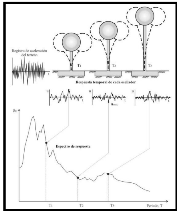
Figura 4.2 Determinación del espectro de respuesta.
