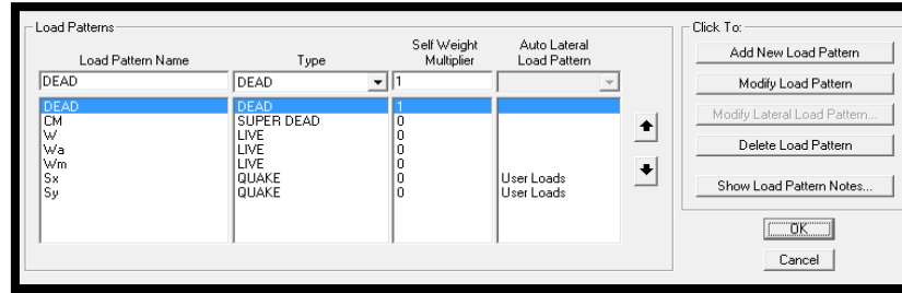
Figura 5.12 Patrones de carga para el análisis.
