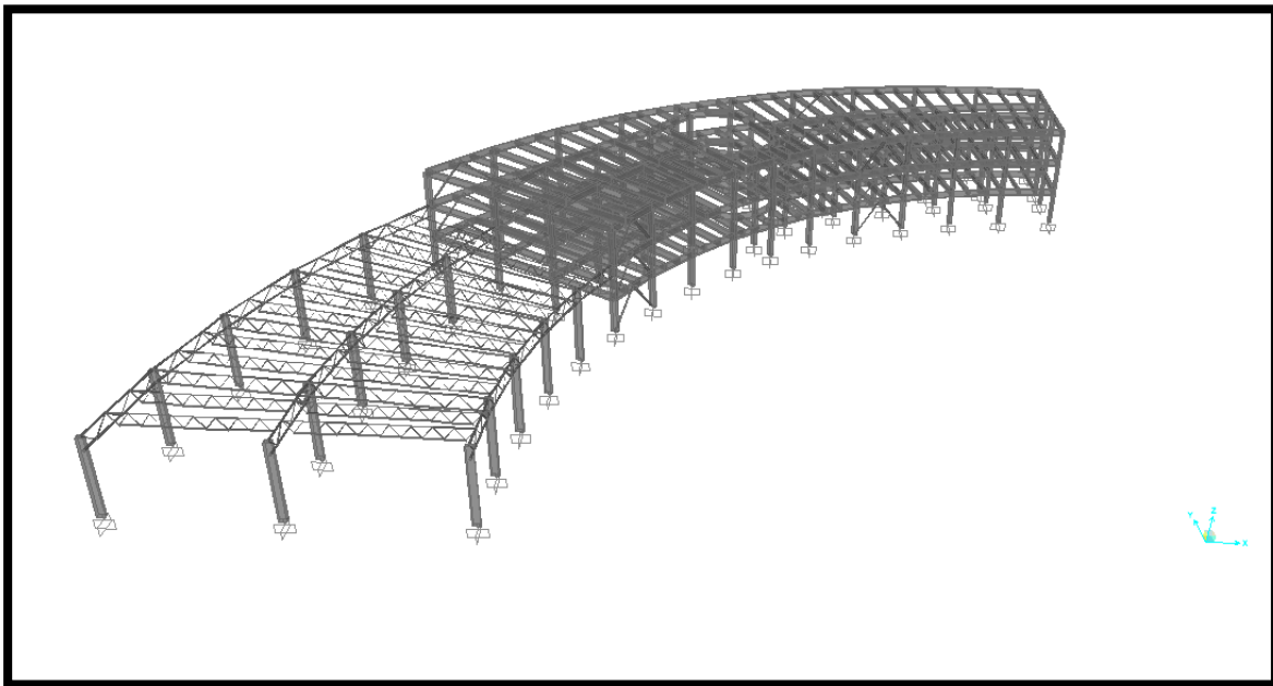
Figura 5.6 Modelo dibujado sin vista extruida en losas.
