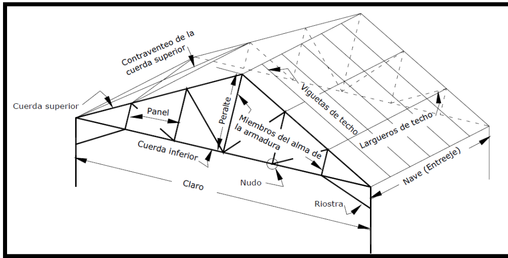
Figura 1.23. Elementos de una armadura.
