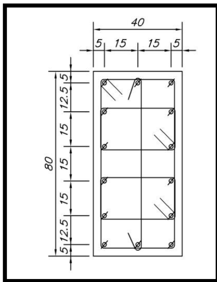
Figura 7.7a Sección transversal de la columna.
