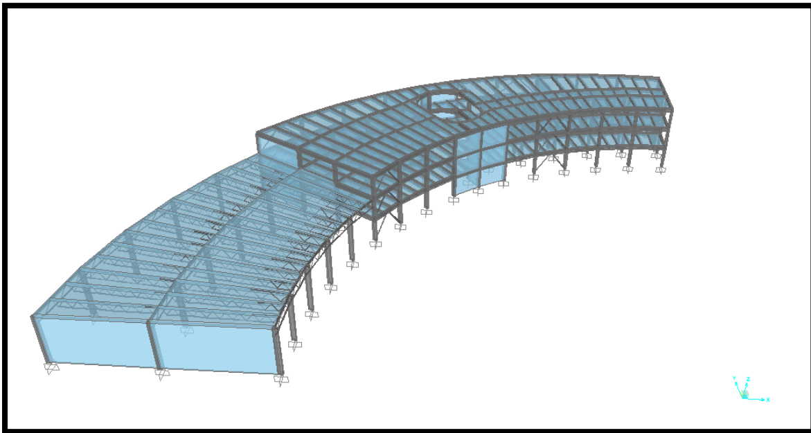
Figura 5.7 Modelo dibujado con vista extruida en losas.
