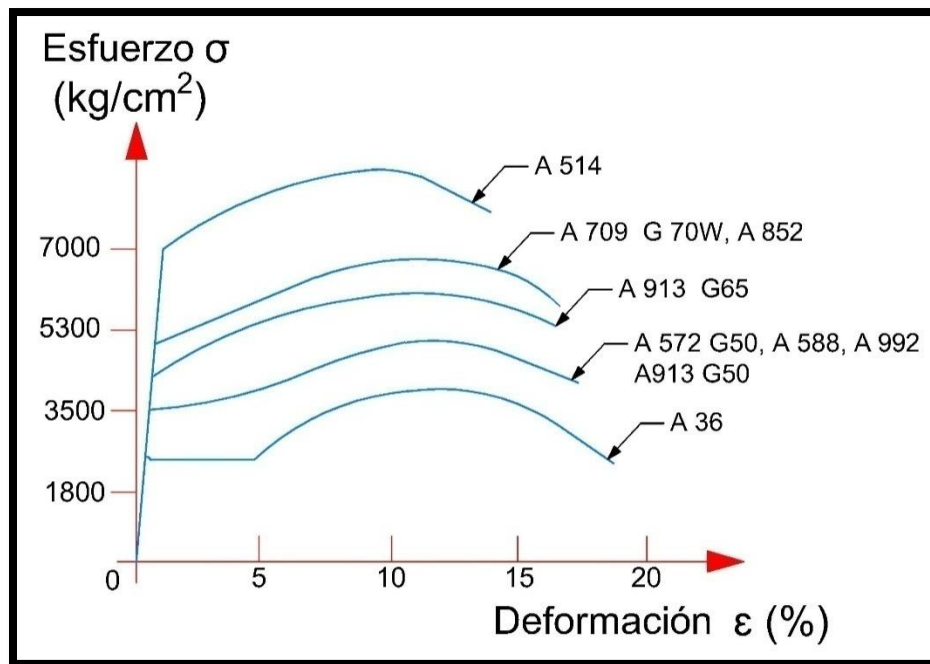
Figura 1.22. Gráfica carga-deformación de algunas calidades de acero.
