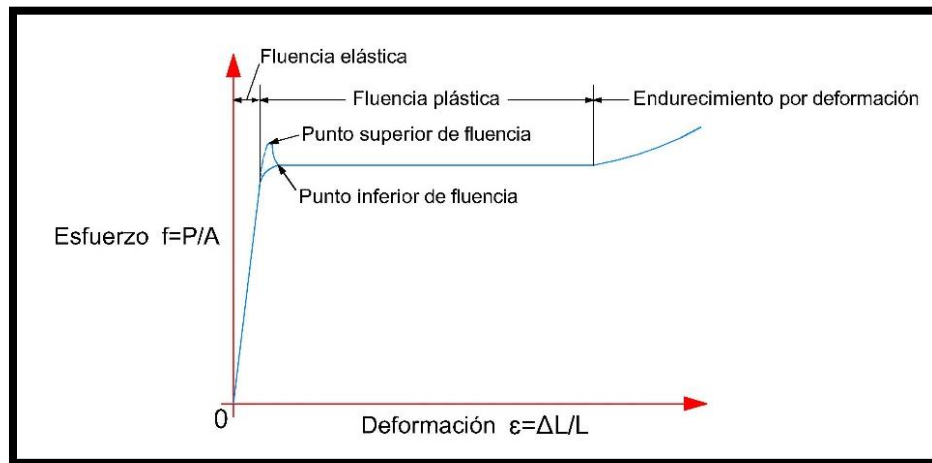
Figura 1.21. Gráfica carga-deformación del acero.
