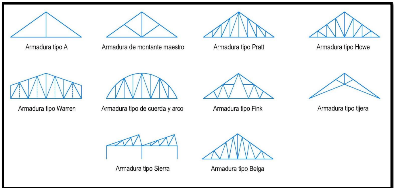
Figura 1.25. Tipos de armaduras.
