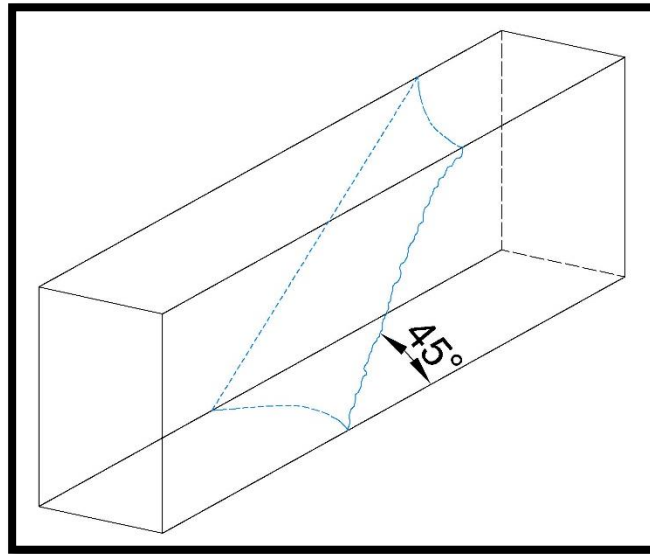
Figura 1.12. Superficie de falla de una viga de concreto simple.
