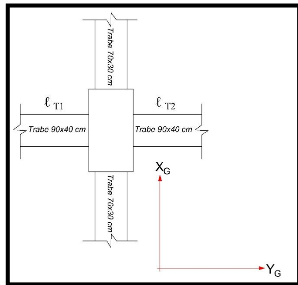
Figura 7.7b Uniones de trabes a la columna.
