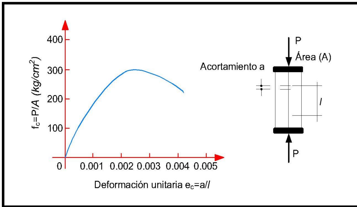
Figura 1.1. Curva esfuerzo-deformación en compresión axial.
