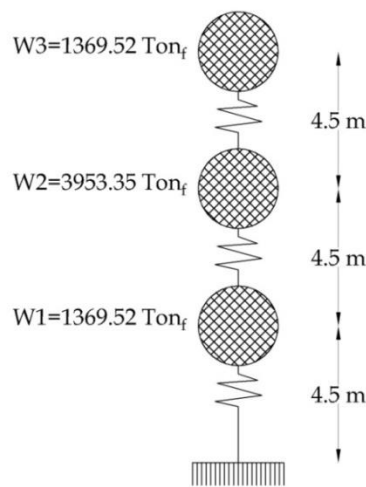
Figura 4.1 Esquema de las masas por entrepiso.
