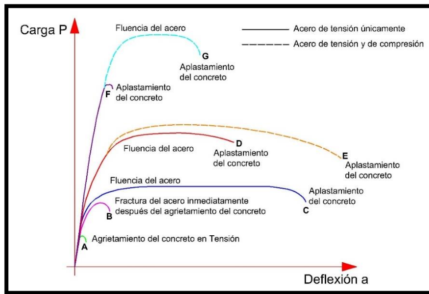
Figura 1.5. Gráficas carga-deflexión de elementos con porcentaje variable de acero sujetos a flexión simple.
