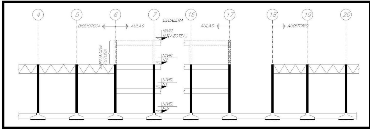
Figura 2.4. Corte esquemático de niveles.
