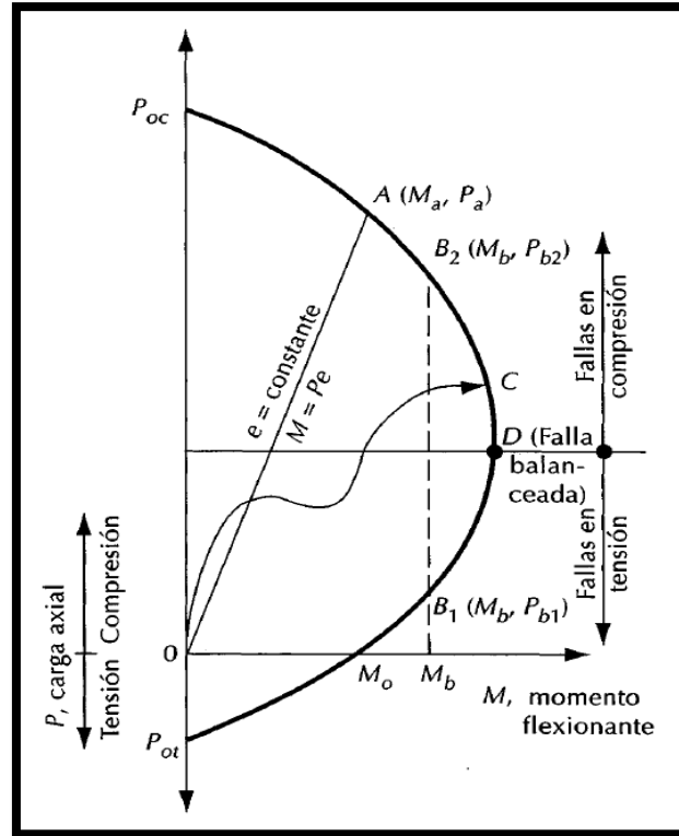
Figura 1.7. Diagrama de interacción típico de una sección rectangular.
