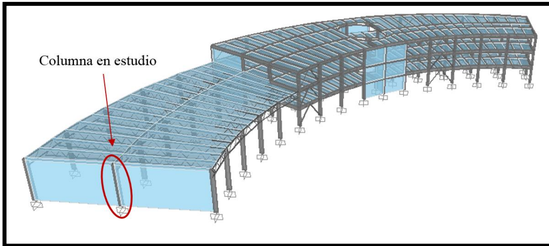
Figura 7.8 Localización de columna en estudio.
