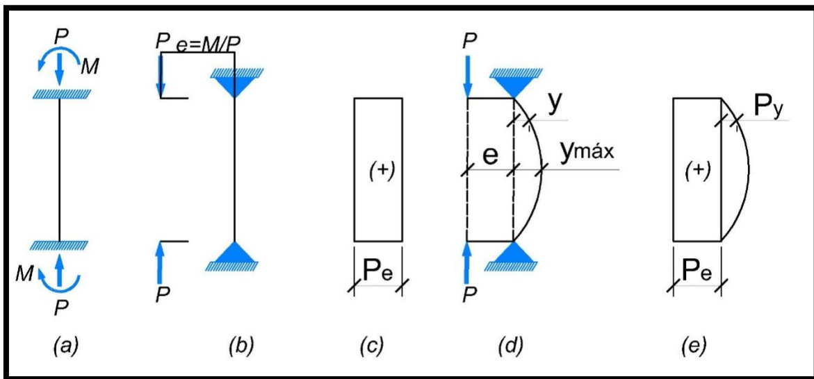
Figura 7.6 Momentos adicionales en una columna por efecto de esbeltez.
