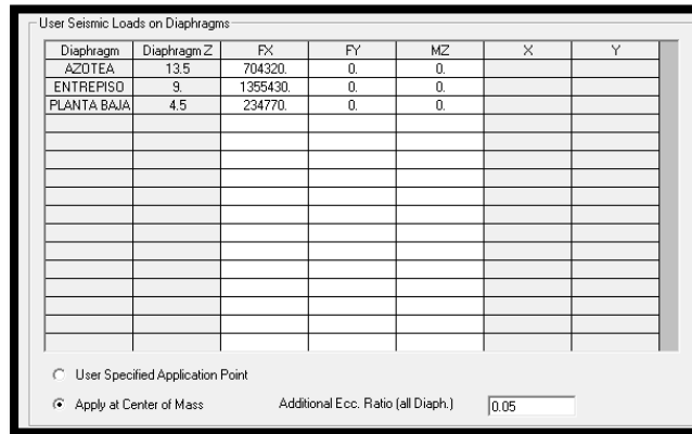
Figura 5.13 Fuerzas laterales del Análisis Estático.
