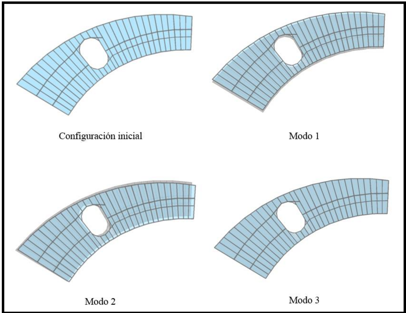
Figura 6.3 Configuración sin aplicar fuerzas y tres primeros modos de vibrar de la estructura para el tercer nivel.
