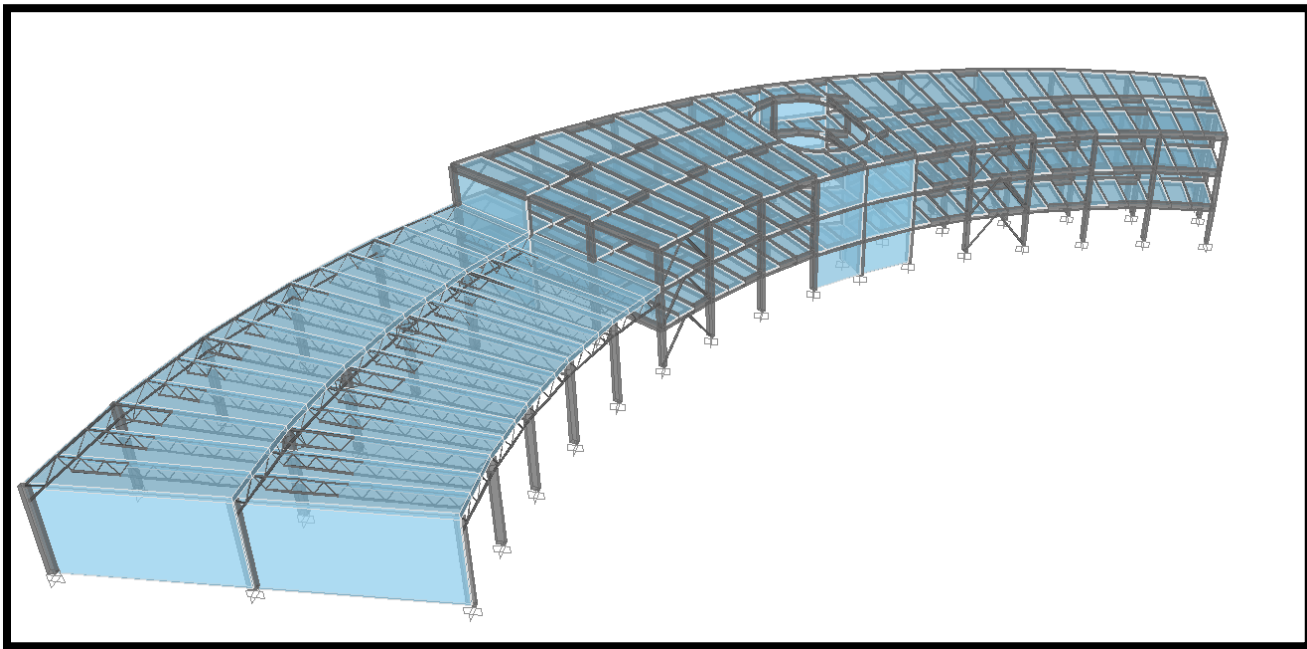
Figura 5.9 Vista del modelo en la sección de concreto que contiene el hueco de la escalera.
