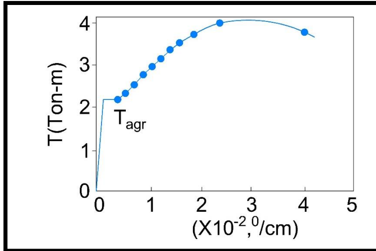
Figura 1.13. Gráfica momento torsionante-giro de un elemento con refuerzo transversal sujeto a torsión pura.
