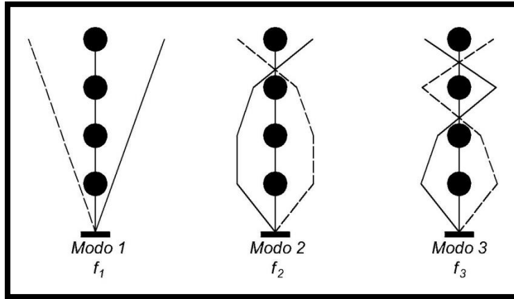
Figura 6.2 Tres primeros modos de oscilación del edificio de 4 niveles.
