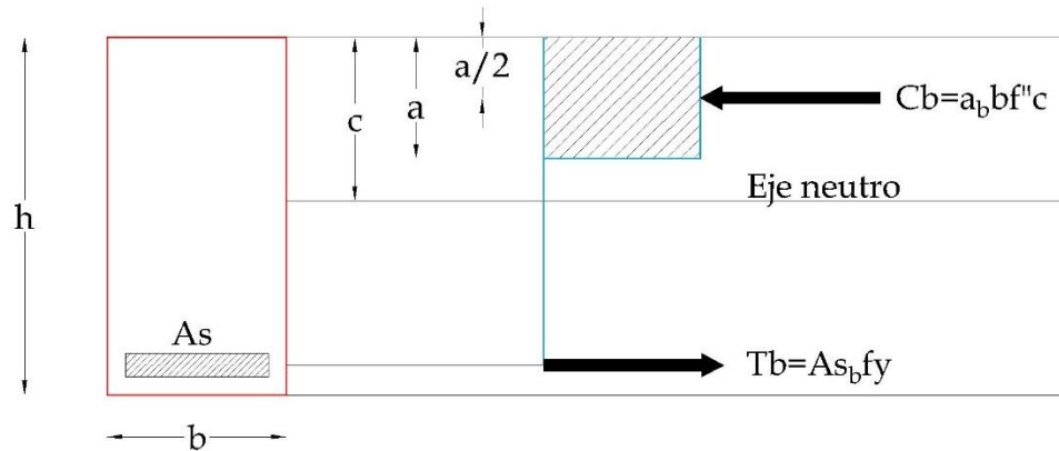
Figura 7.2 Fuerzas que intervienen en vigas simplemente armadas.
