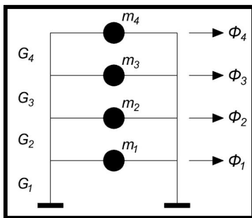
Figura 6.1 Modelo de un edificio de 4 niveles.
