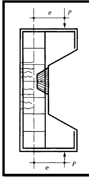
Figura 1.6. Especimen para ensayo en flexocompresión con agrietamiento típico.
