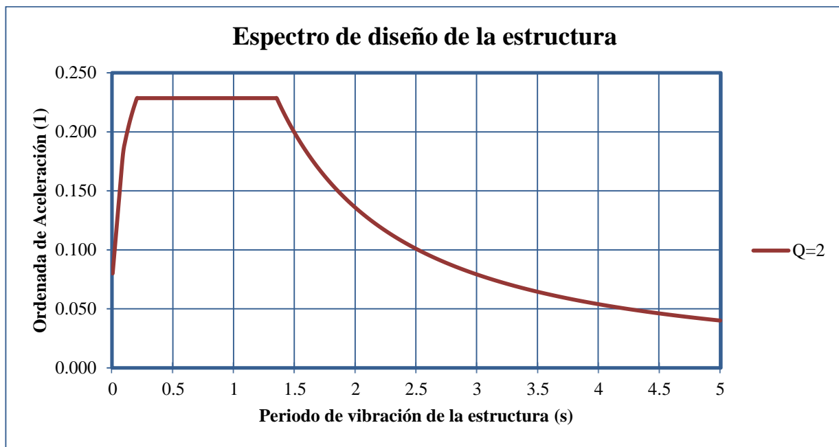
Figura 4.3 Espectro de diseño de la estructura.
