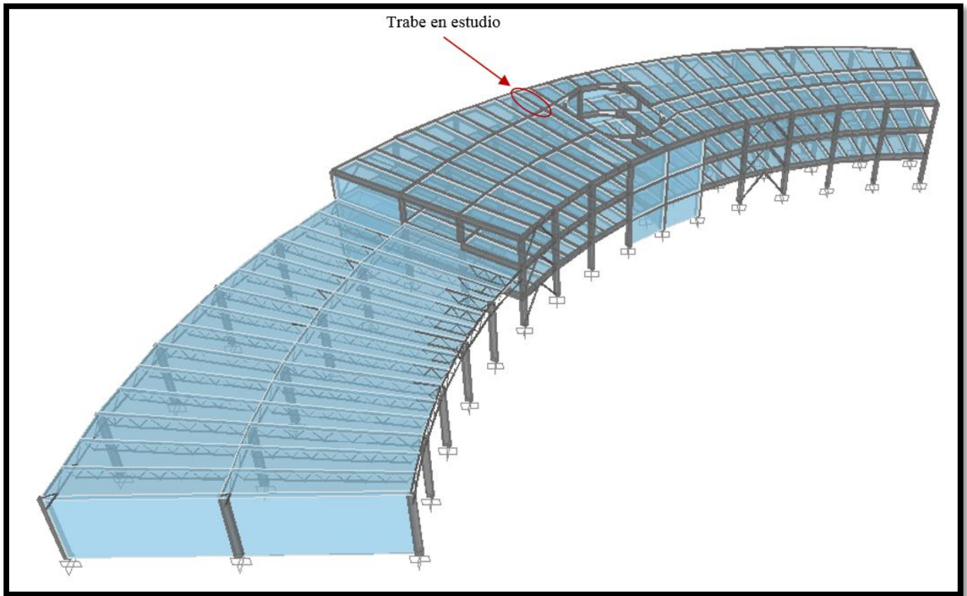
Figura 7.3b Localización de la trabe en estudio (Tercer nivel).
