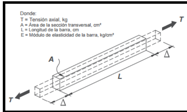
Figura 1.18. Barra sujeta a tensión axial.
