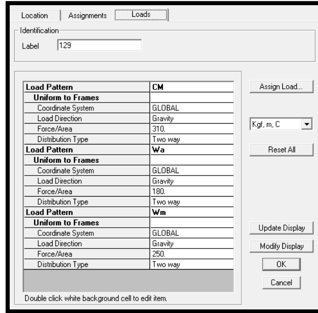
Figura 5.17 Asignación de cargas en las losas.
