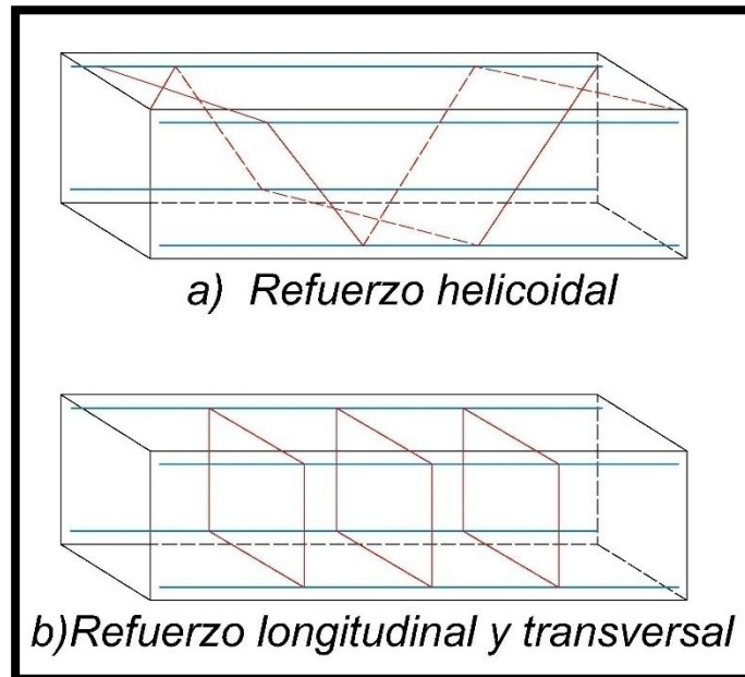
Figura 1.14. Tipos de refuerzo para torsión.
