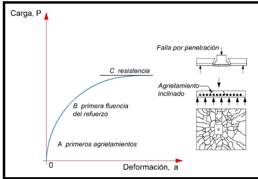
Figura 1.10. Gráfica cara-deformación de una zapata.
