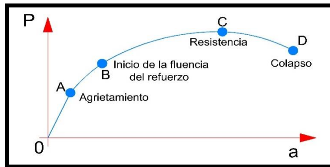
Figura 1.15. Gráfica carga-deflexión de una losa perimetral.
