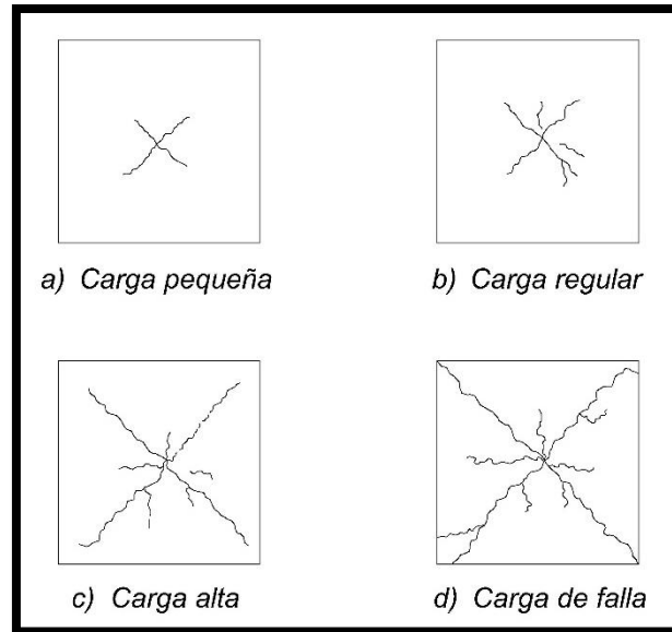
Figura 1.16. Configuraciones de agrietamiento para distintos valores de carga aplicada.
