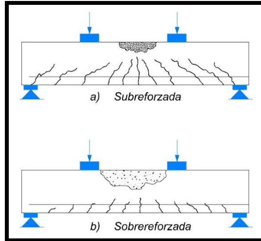
Figura 1.4. Agrietamiento en falla de vigas sujetas a flexión.
