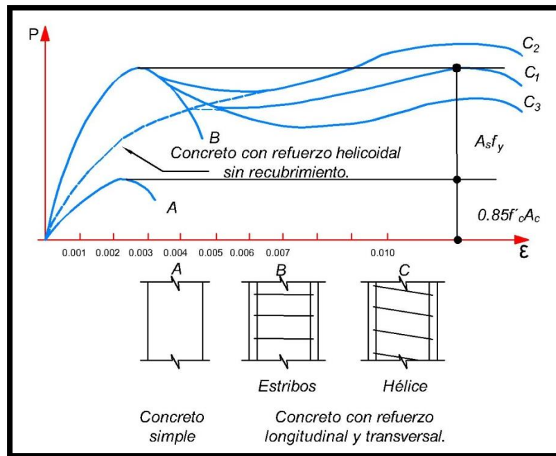
Figura 1.2. Curva esfuerzo-deformación unitaria en compresión axial para diferentes tipos de elementos de concreto.
