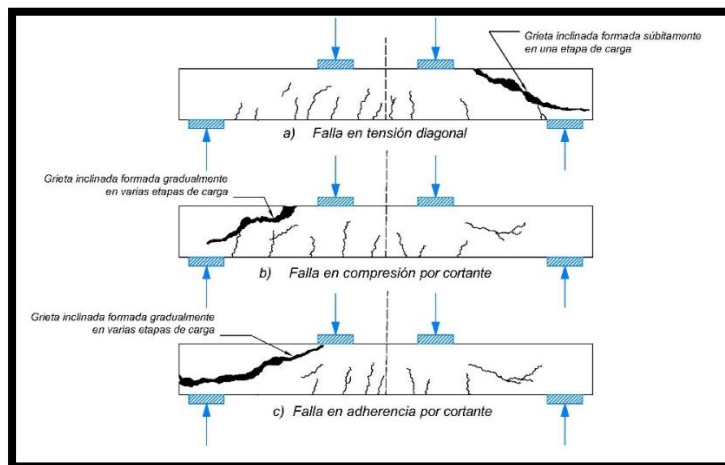
Figura 1.8. Diferentes tipos de falla en elementos donde existe fuerza cortante.
