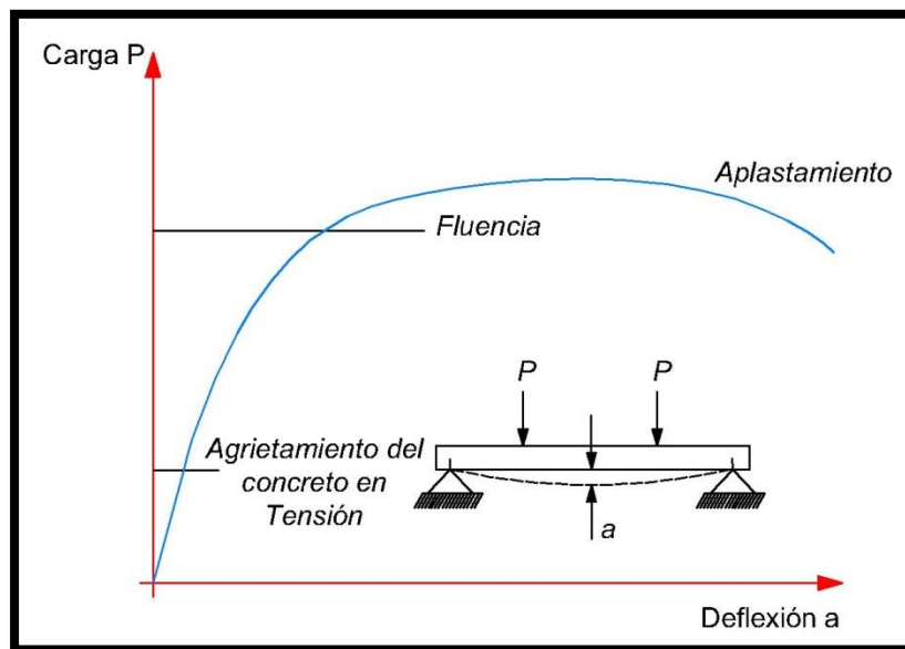
Figura 1.3. Curva carga-deflexión de un elemento con porcentaje usual de acero.
