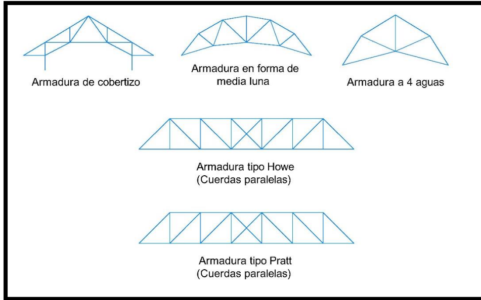
Figura 1.26. Otras armaduras.
