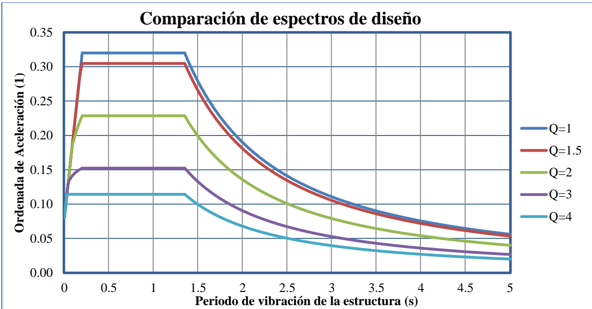
Figura 4.4 Comparación de espectros de diseño.
