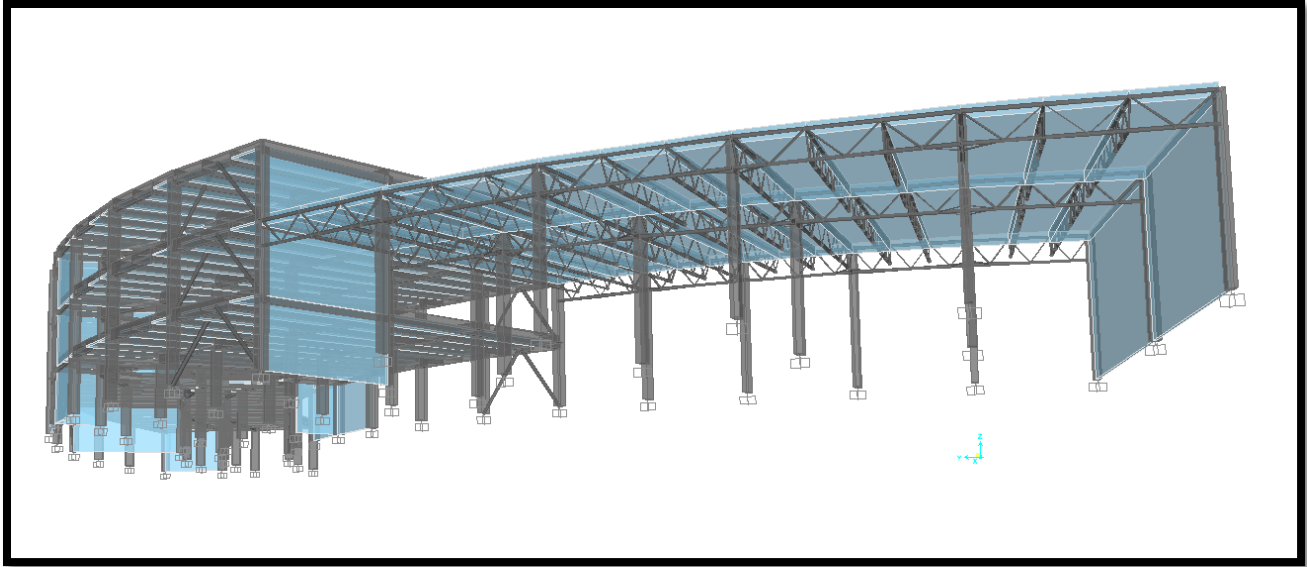
Figura 5.8 Vista del modelo en la sección con armaduras (Biblioteca).
