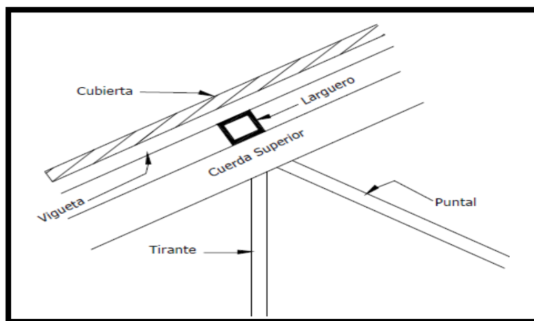
Figura 1.24. Elementos de una armadura.
