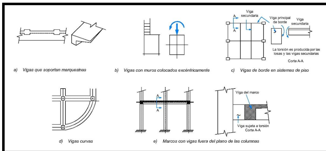
Figura 1.11. Elementos estructurales sujetos a torsión.
