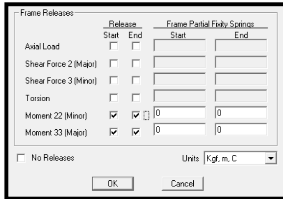
Figura 5.10 Trabe con momento igual a cero en los extremos.
