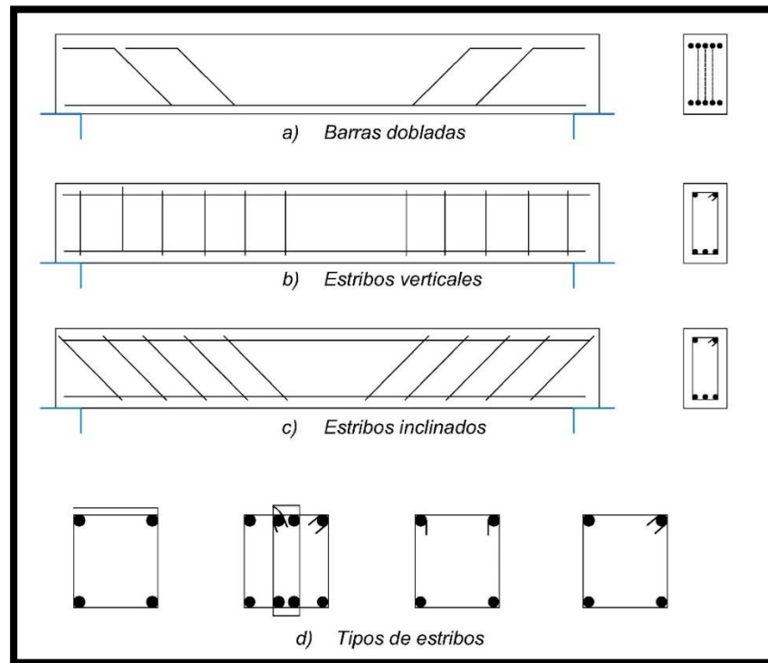
Figura 1.9. Tipos de refuerzo.
