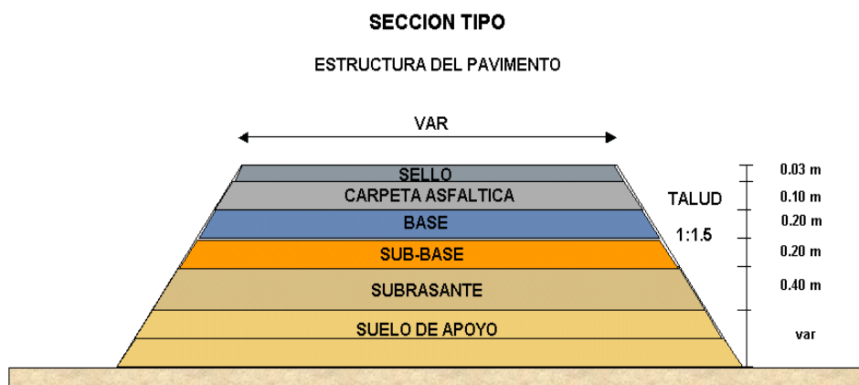
Figura 14. Sección Tipo de Pavimento Flexible
