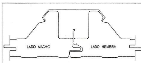
Figura 10. Junta de multytecho
