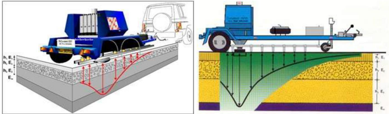
Ilustración 15 Cortes esquemáticos de las deflexiones obtenidas con el deflectómetro de impacto
