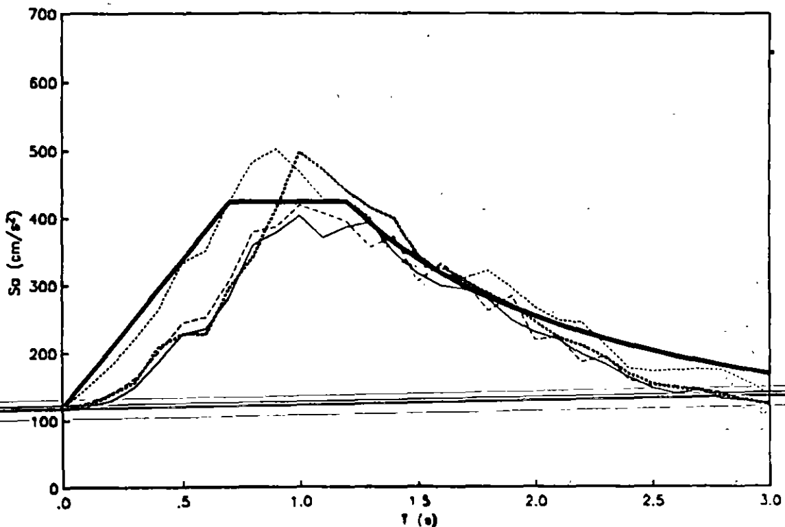
Figura 18. Espectro de diseño (línea gruesa continua) para el sitio en estudio. Con el trazo más fino se indican los espectros de respuesta inelásticos multiplicados por el factor Q'=1.5 (línea continua), 2 (línea discontinua) y 4 (línea punteada). Con línea media punteada se indica el espectro de respuesta elástico promedio
