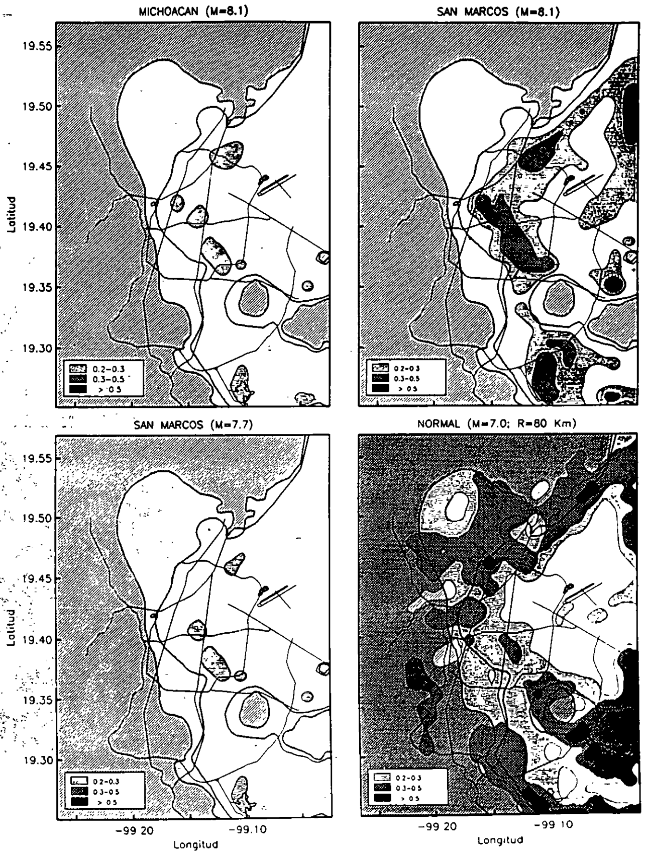
Figura 20. Distribución de aceleraciones espectrales ( S_a/g ) para periodos estructurales T_e = 0.3 \pm 0.1 s en el valle de México, correspondientes a posibles sismos intensos originados en las costa del Pacífico Mexicano y en el interior del continente
