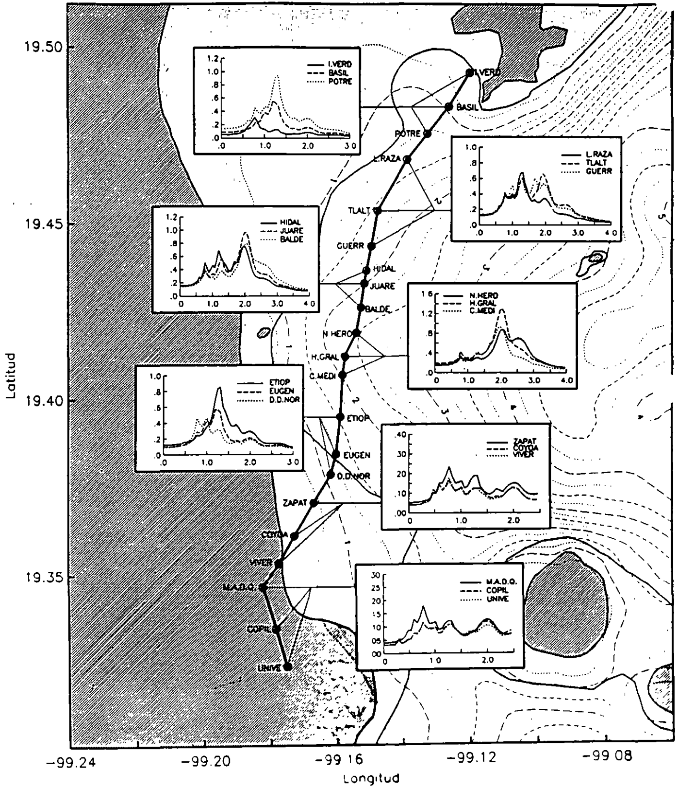
Figura 11. Igual que la figura 9. pero para la Linea 3.
