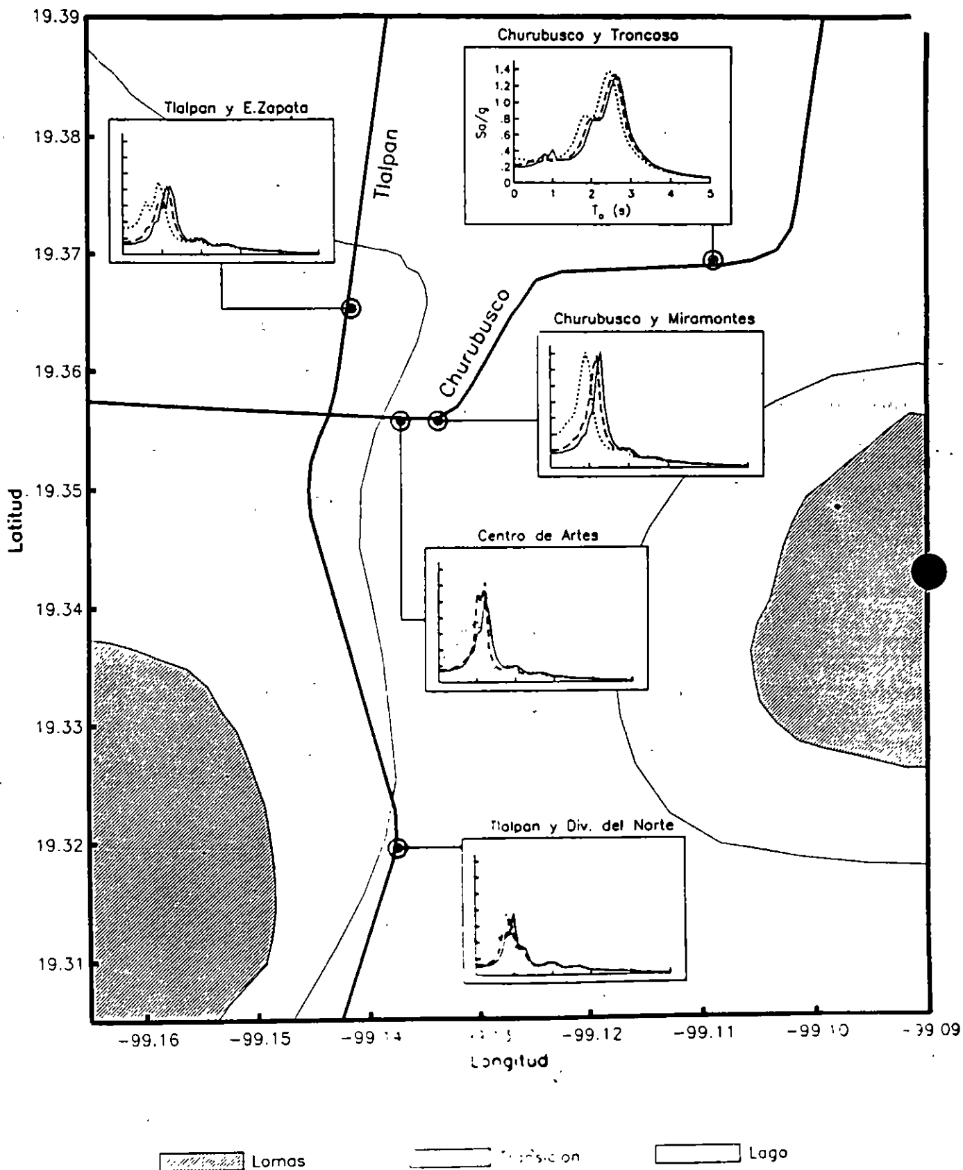
Figura 8. Espectros de respuesta para el Centro de las Artes y algunos puentes enclavados. Se indican la condición de campo libre y dos condiciones de interacción suelo-estructura.
