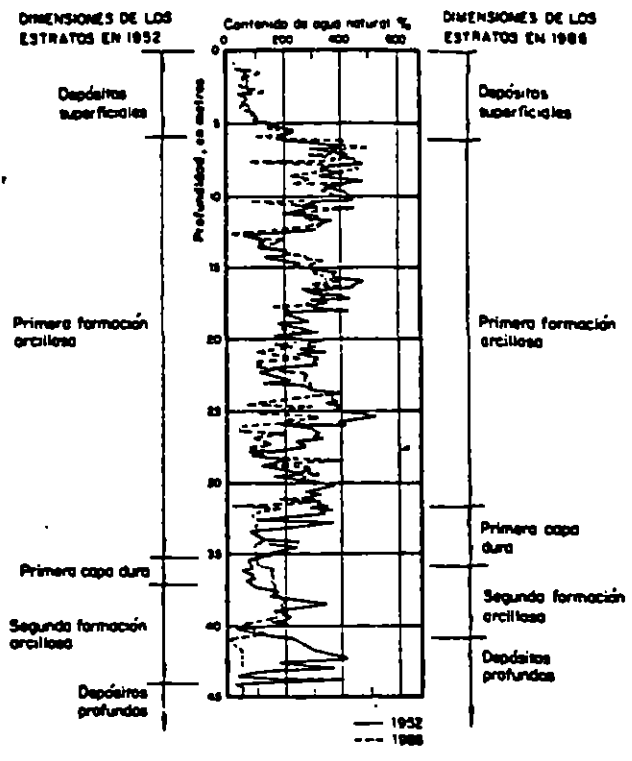
Fig 5 Estratigrafía típica de la zona lacustre
