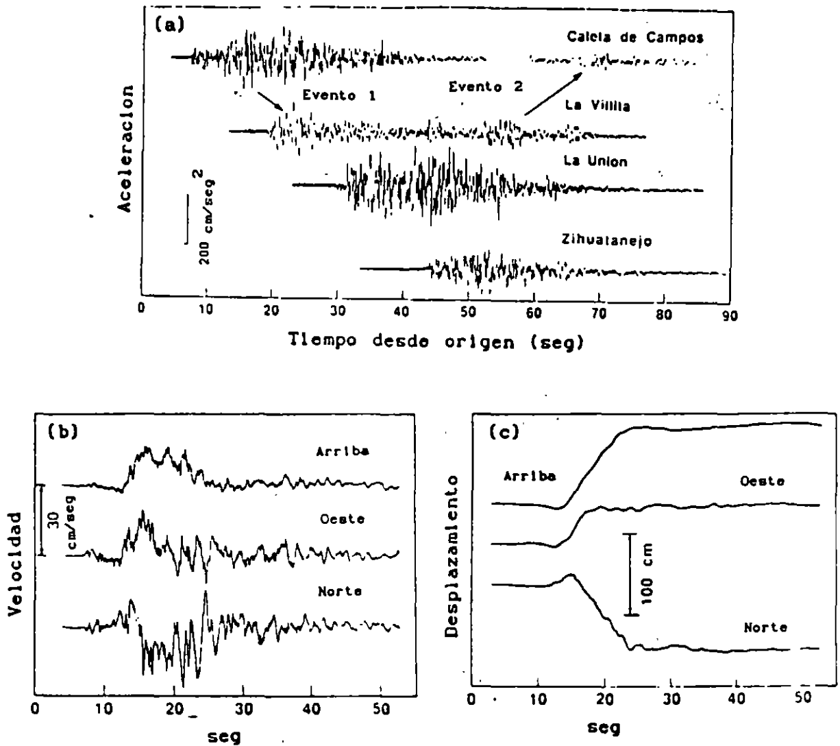
Fig 2.3. (a) Registros de las aceleraciones (componente NS) del temblor del 19 de septiembre, 1985 en la zona epicentral. Se pueden ver 2 eventos principales en las estaciones de Caleta de Campos (CALE) y La Villita. (b) Velocidad del terreno en CALE. Nótese las oscilaciones con un periodo de 0.4 seg. (c) Desplazamiento del terreno en CALE.
