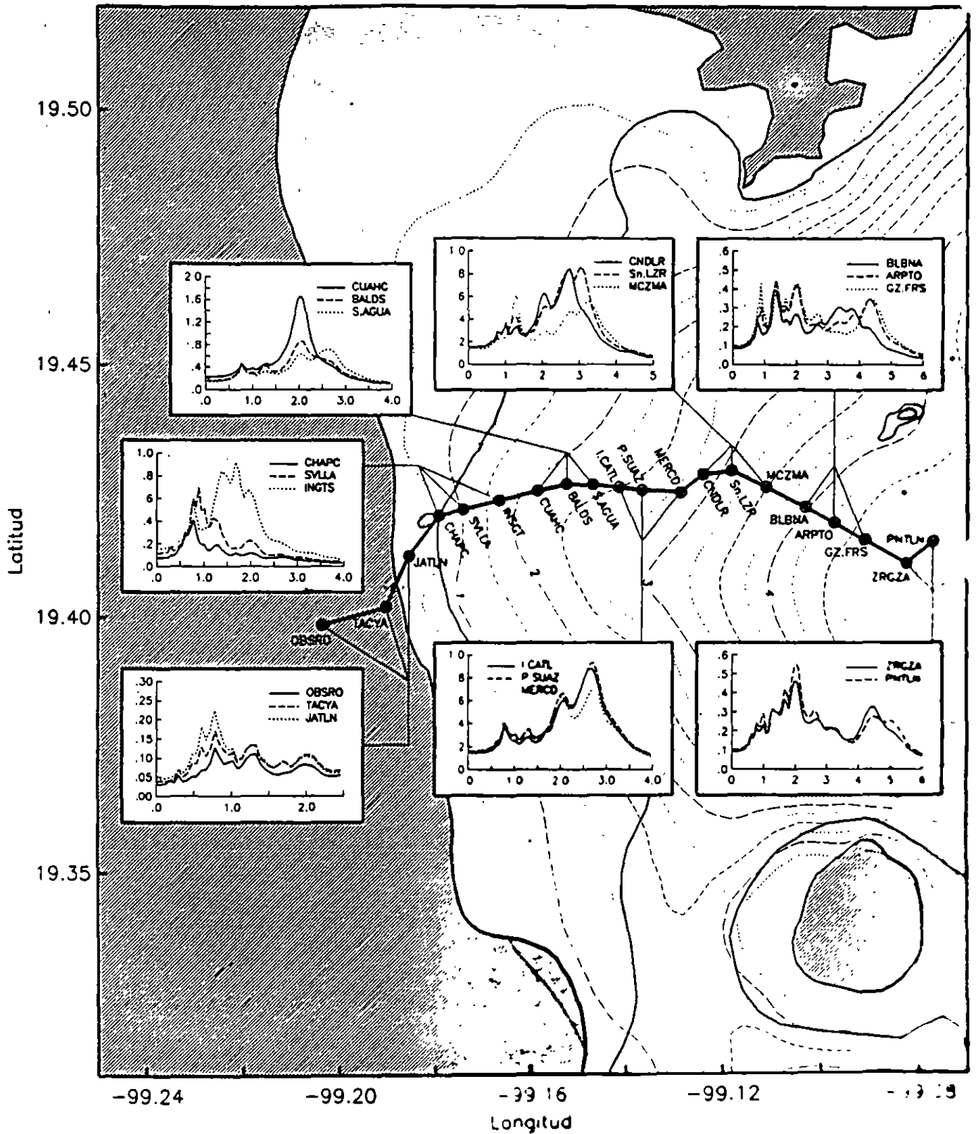
Figura 9. Espectros de respuesta para las estaciones de la Línea 1 del Sistema de Transporte Colectivo de la Ciudad de México. Se indican algunas curvas de periodos dominantes del terreno como referencia adicional.
