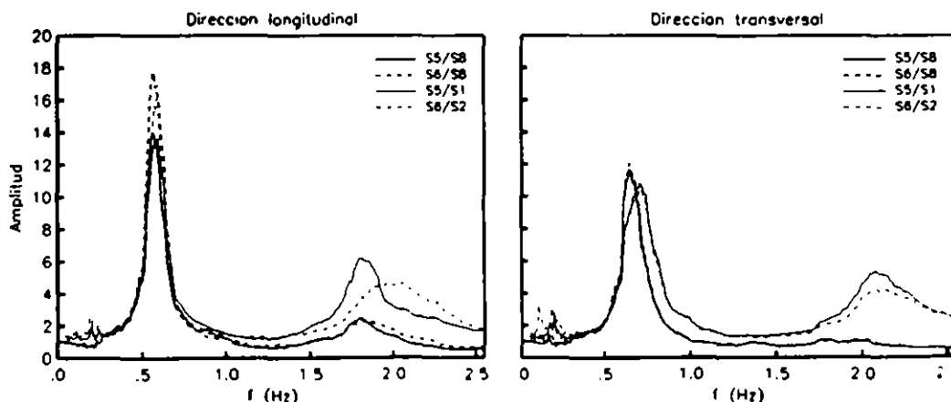
Figura 6 Funciones de trasferencia de azoteas relativas a a) campo libre (líneas gruesas) y b) sótanos (líneas delgadas).
