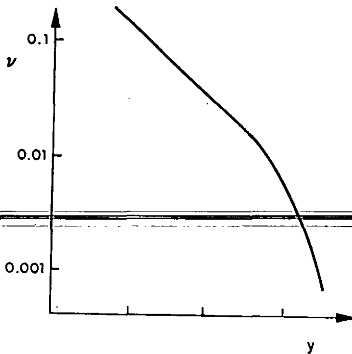
Fig 2 Tasas de excedencia de intensidades en un sitio
