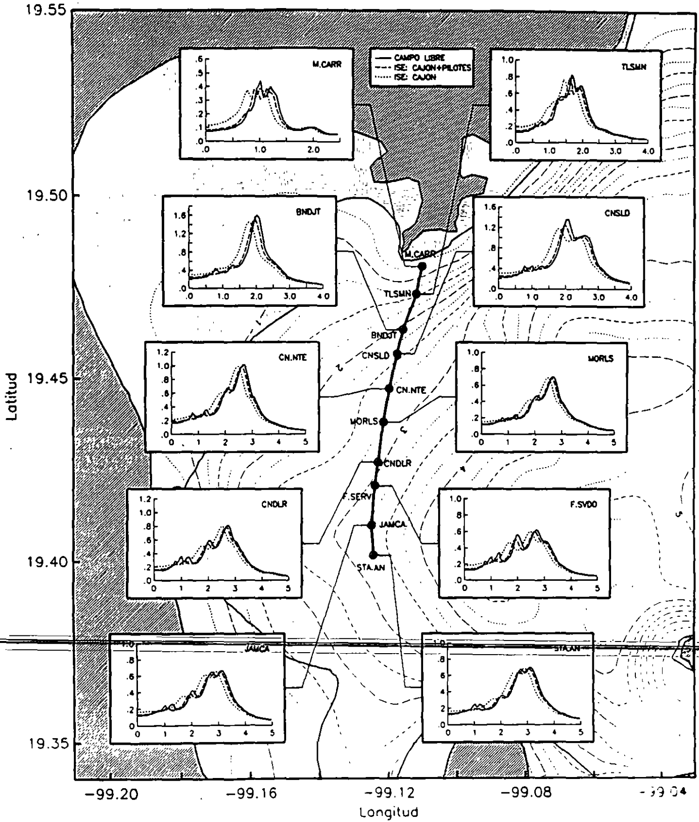
Figura 12. Igual que la figura 9, pero para la Linea 4. En adición se indican los espectros de respuesta para dos condiciones de interacción suelo-estructura
