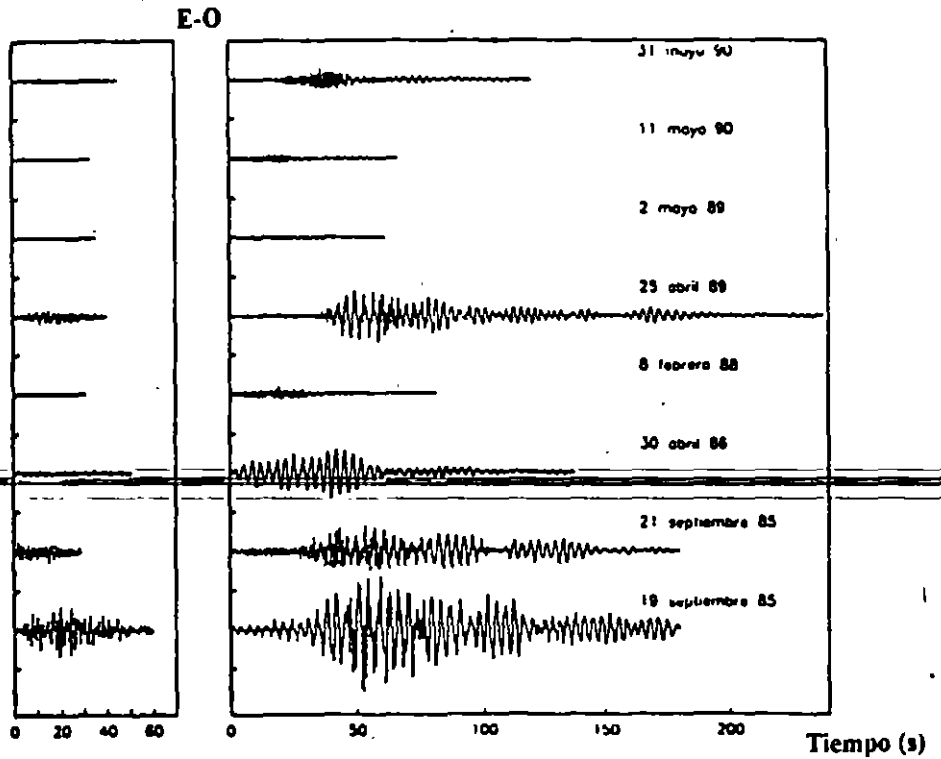
Fig 19 Registros de aceleración en Ciudad Universitaria y Central de Abastos captados durante ocho sismos recientes
