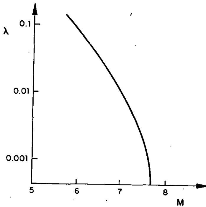
Fig 1 Tasas de excedencia de magnitudes en una fuente sísmica
