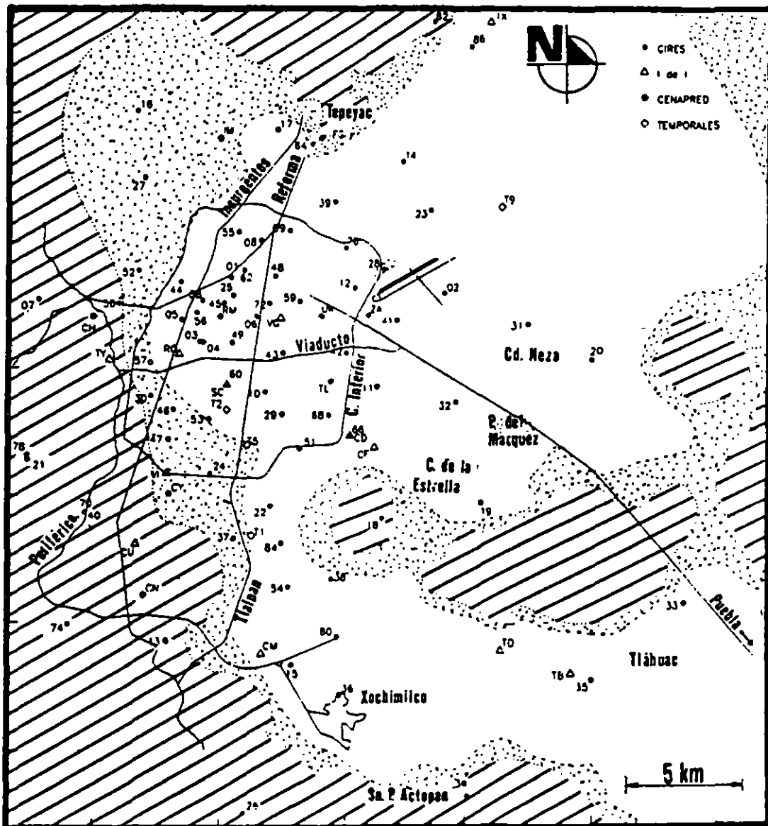
Fig 10 Red acclerométrica de la ciudad de México, zonas geotécnicas y puntos de referencia
