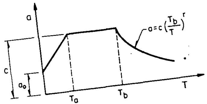
Fig 14 Forma adoptada para los espectros de diseño
