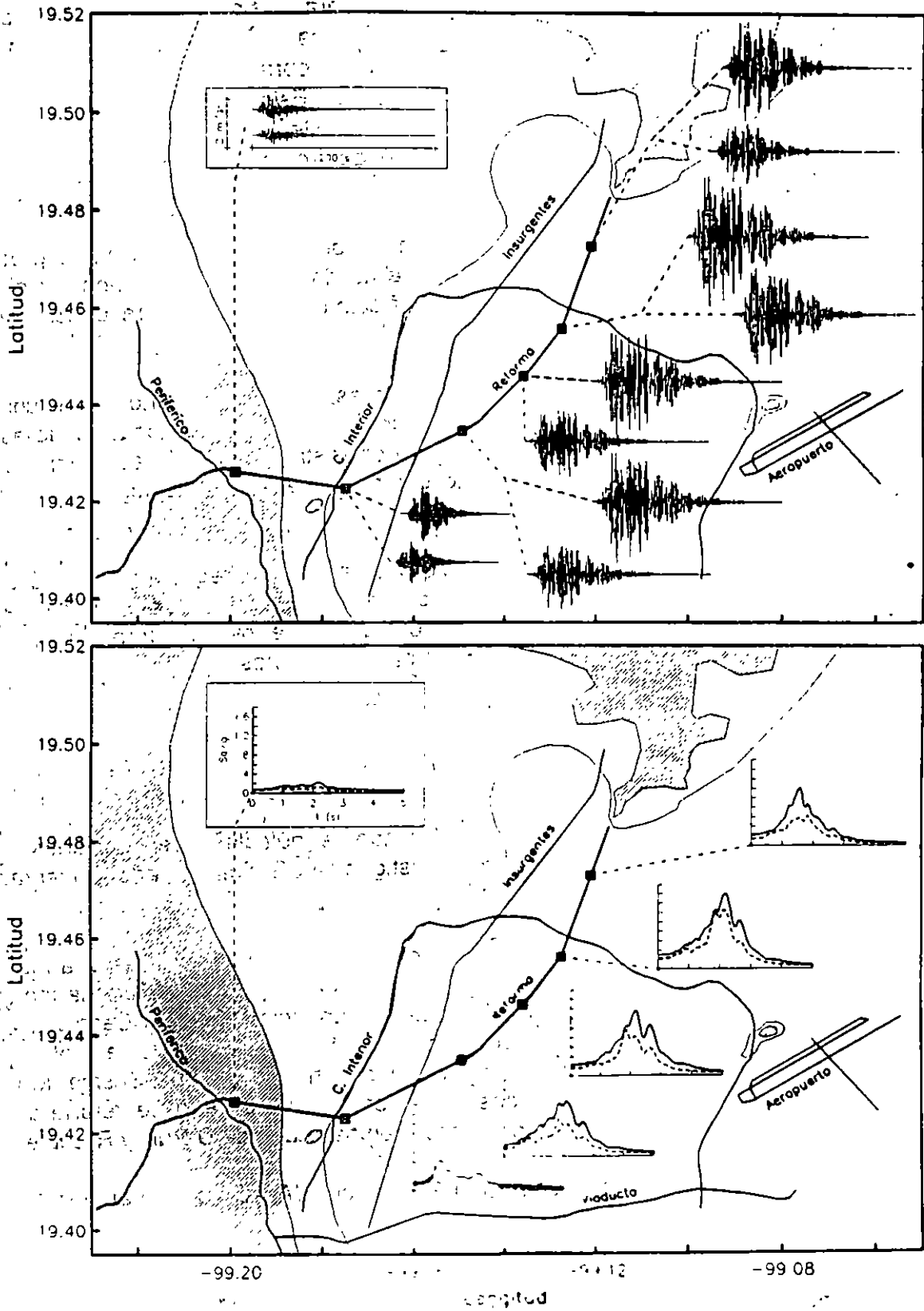
Figura 23. Parte superior: Acelerogramas sintéticos para dos sismos de subducción (M=8.1), generados en las brechas de San Marcos (arriba) y de Michoacan (abajo). Parte inferior: Espectros de respuesta. Con líneas continua y discontinua se indican los espectros para San Marcos y Michoacan respectivamente.
