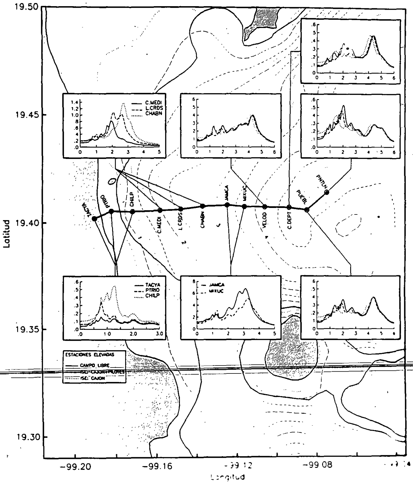
Figura 16. Igual que la figura 9, pero para la Linea 9. Para las estaciones Velódromo, Ciudad Deportiva, Puebla y Pantitlán, se consideraron dos condiciones de interacción suelo-estructura.
