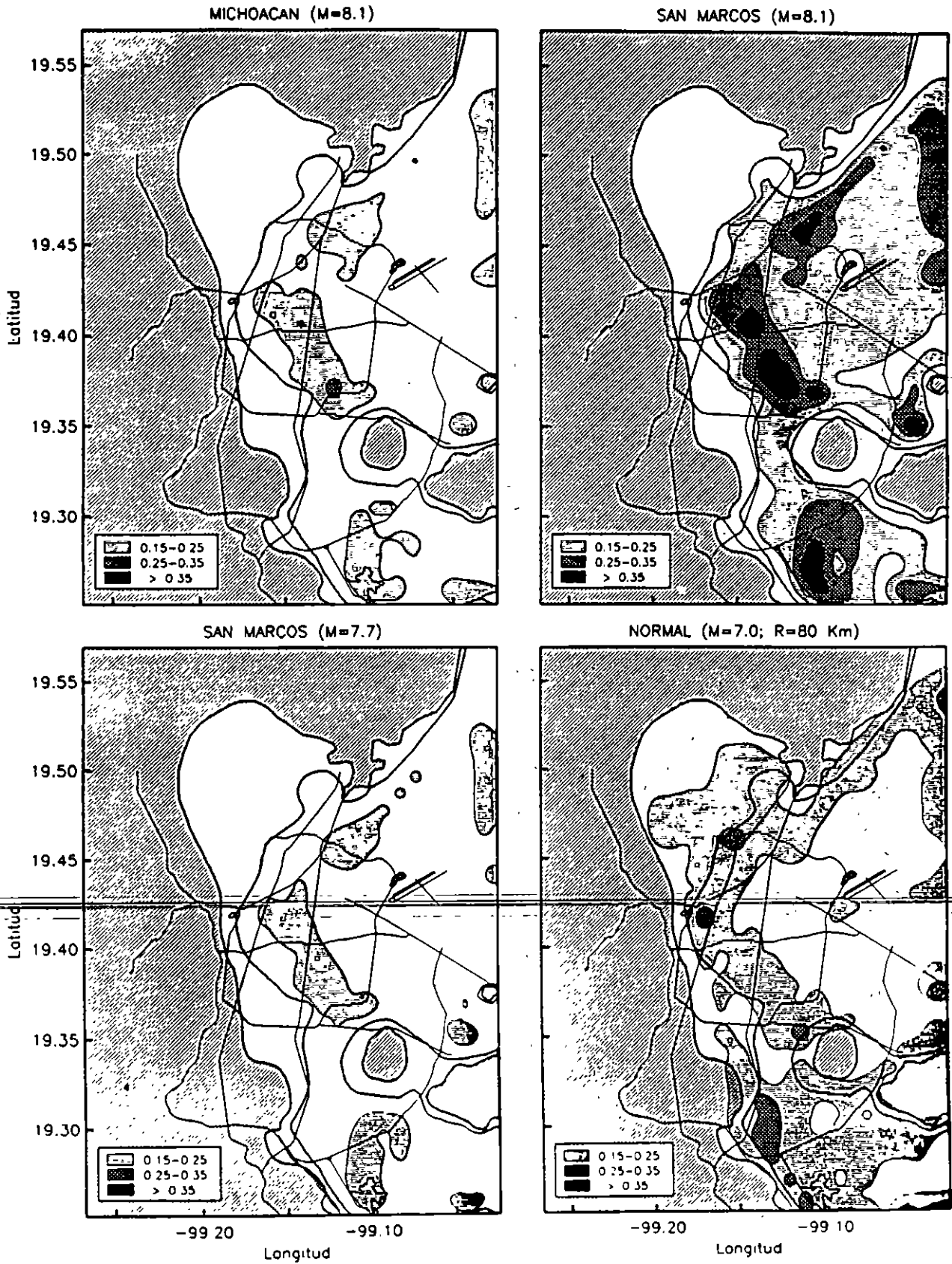
Figura 19. Distribución de aceleraciones máximas del terreno ( S_a/g ) en el valle de México correspondientes a posibles sismos intensos originados en las costa del Pacífico Mexicano y en el interior del continente
