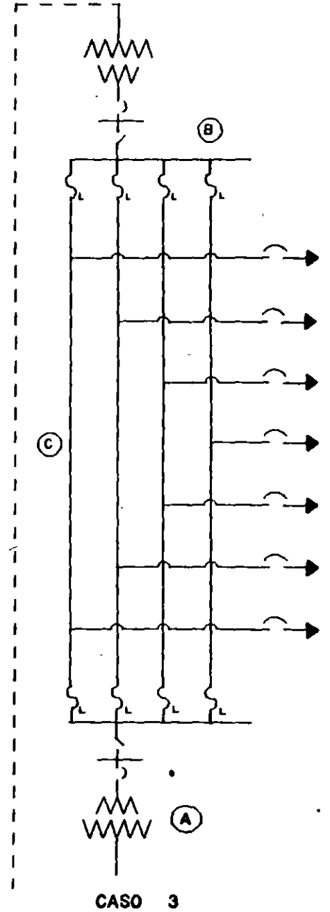
Figura 5.- Estructura de una mancha de red automática
