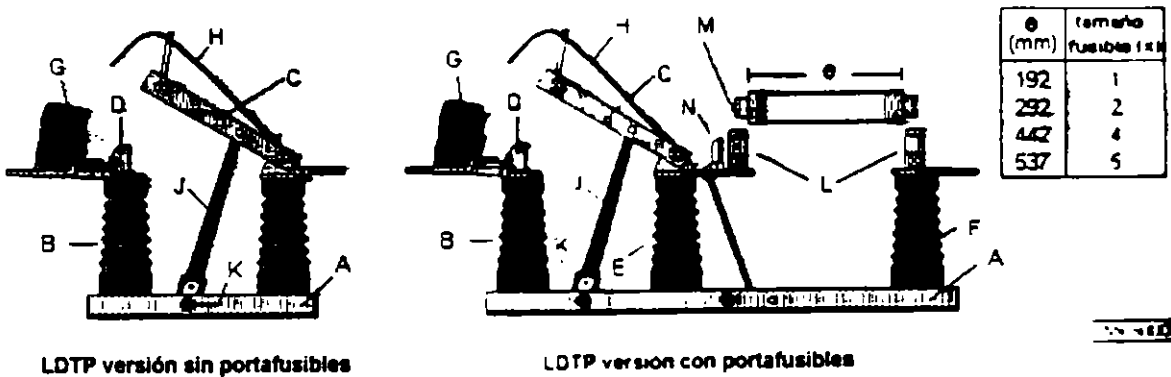
Tipos de desconectores
