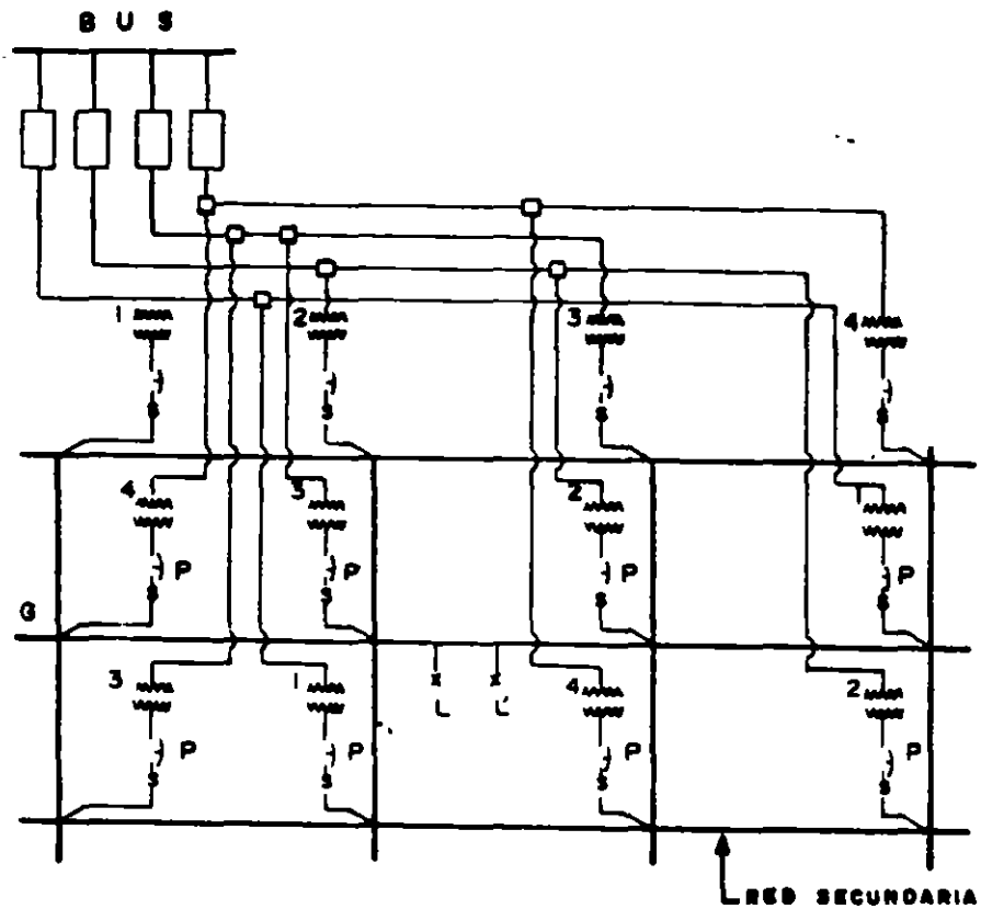
Figura 7 Red malleada de baja tensión
