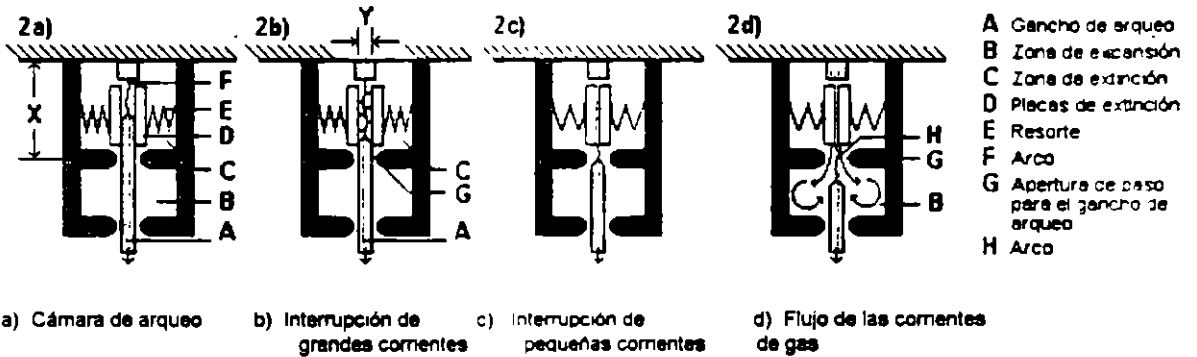
Operación de las cámaras de arco
