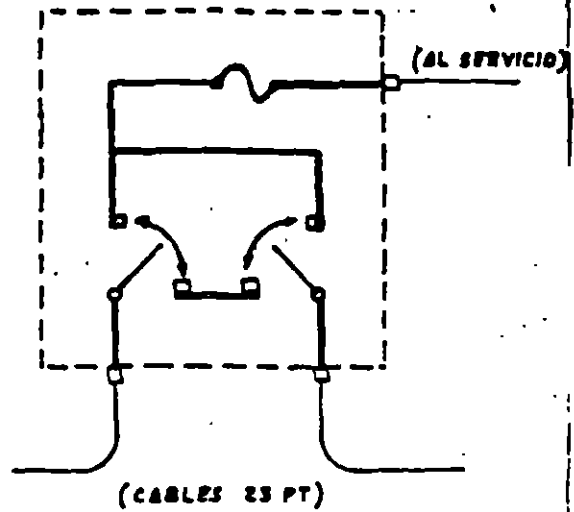
FIGURA 12. - INTERRUPTORES DE 3 Y 4 VIAS PARA CABLES SUBTERRANEOS EN 23 KV. (DIAGRAMA UNIFILAR).
