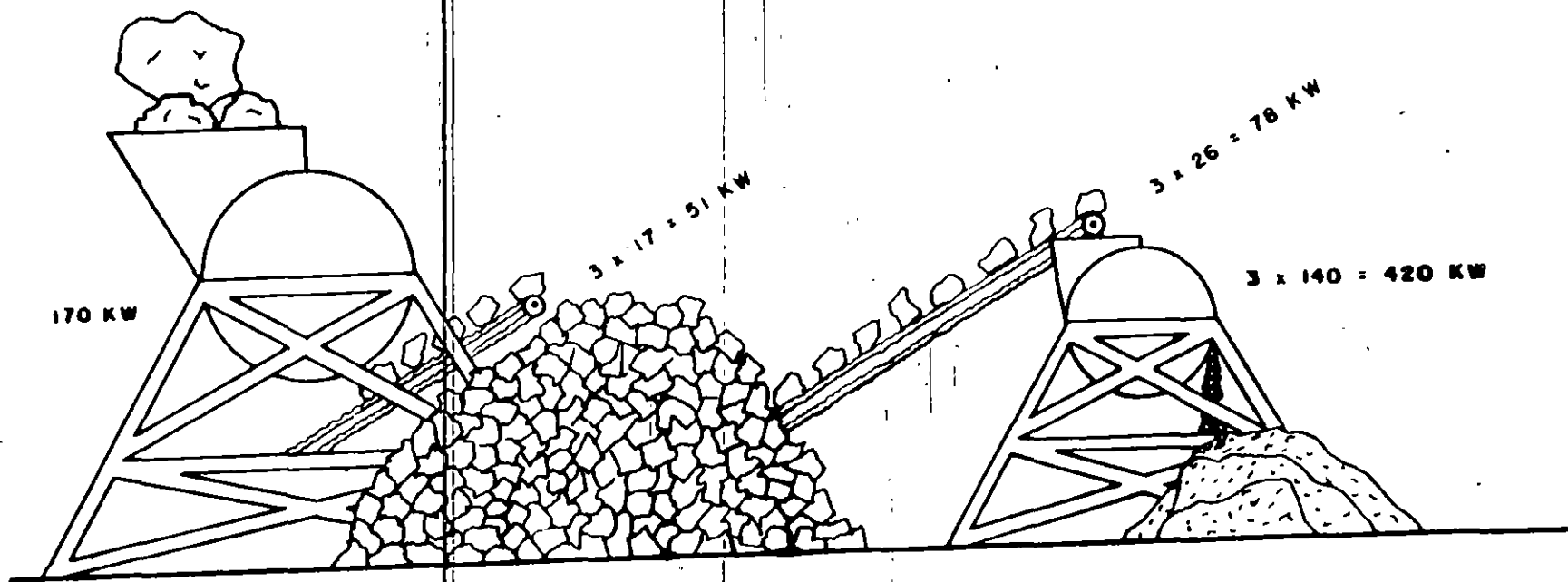
FIGURA 5.4 .- PROCESO DE UNA EMPRESA TRITURADORA DE PIEDRA
