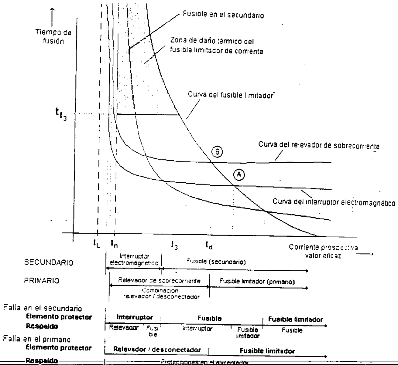
Figura 6 Protecciones por fusible y relevador de sobrecorriente en el primario y fusibles e interruptor electromagnético en el secundario
