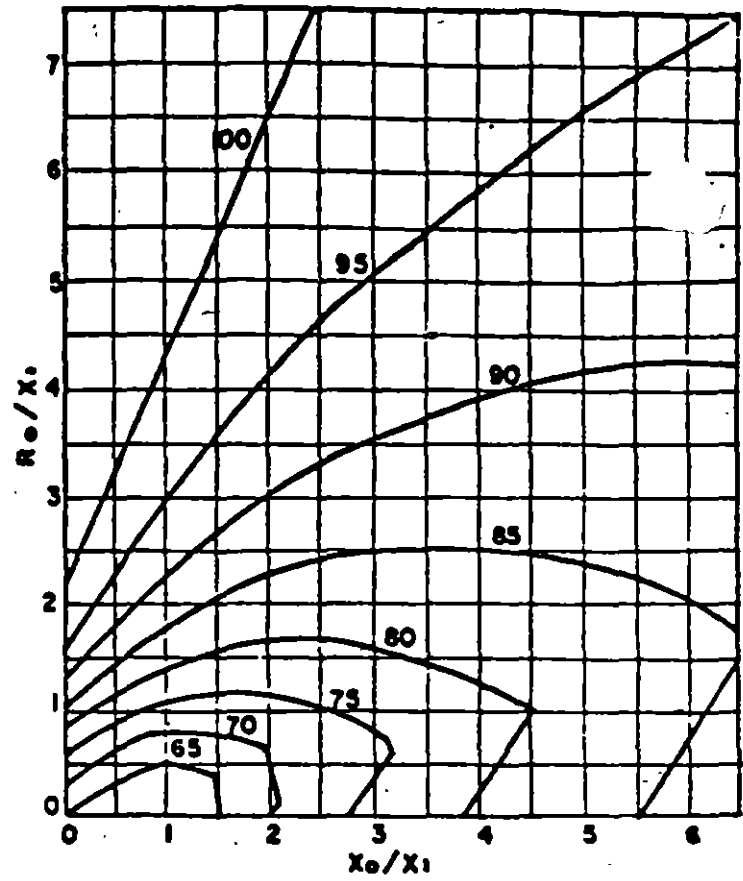
(b). CONDICIONES DE TENSION PARA R_1 = R_2 = 0.1 X_1
