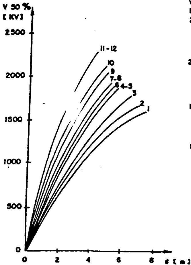
GRAFICA No. 4.4. VALOR V 50% EN FUNCION DE LA DISTANCIA d y DEL TIPO DE ELECTRODOS PROPUESTO POR L. PARIS.
