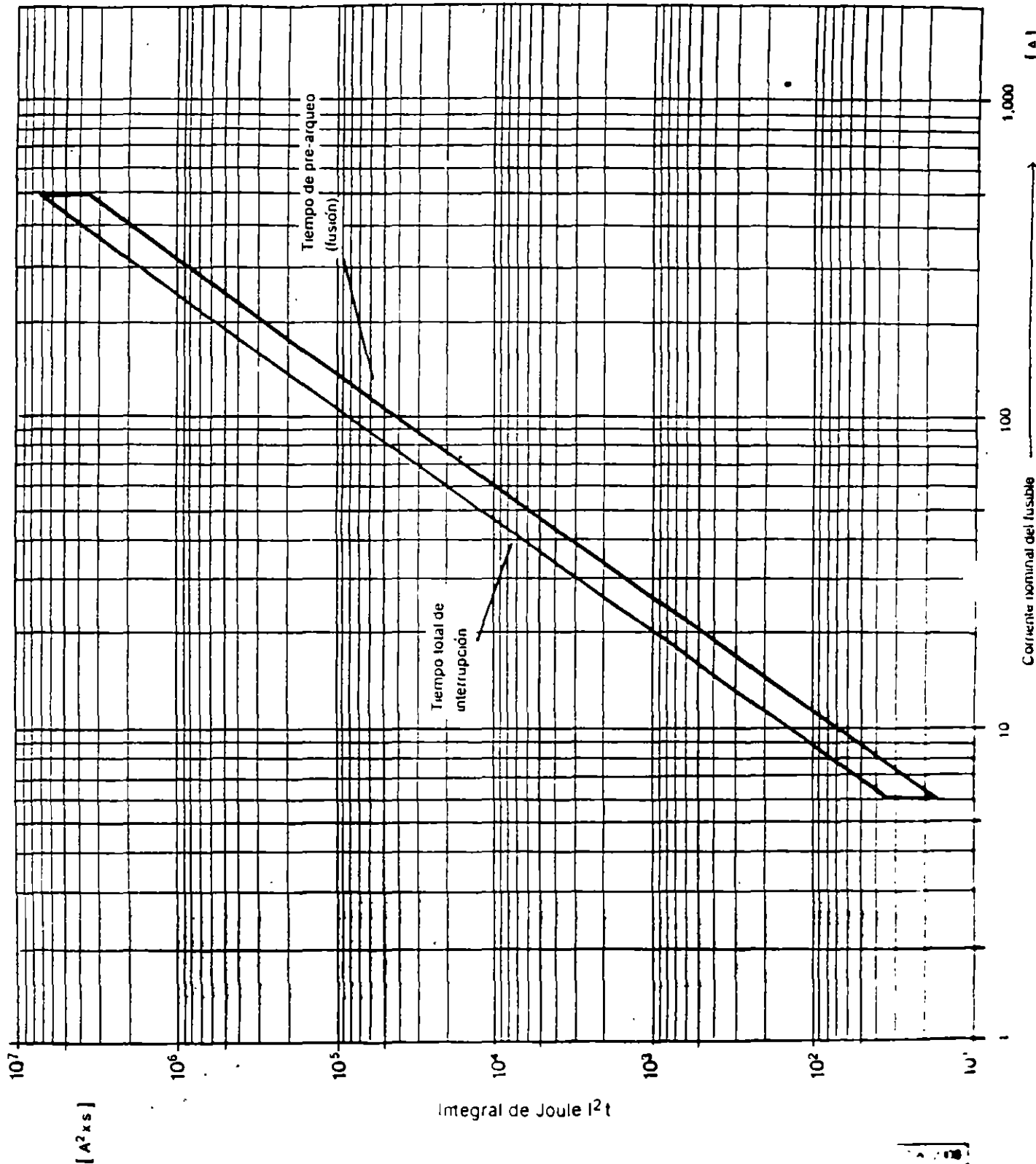
FIGURA 10 Curva característica I^2t de los fusibles DRIWISA® para tiempos de operación menores a 0.1 seg
