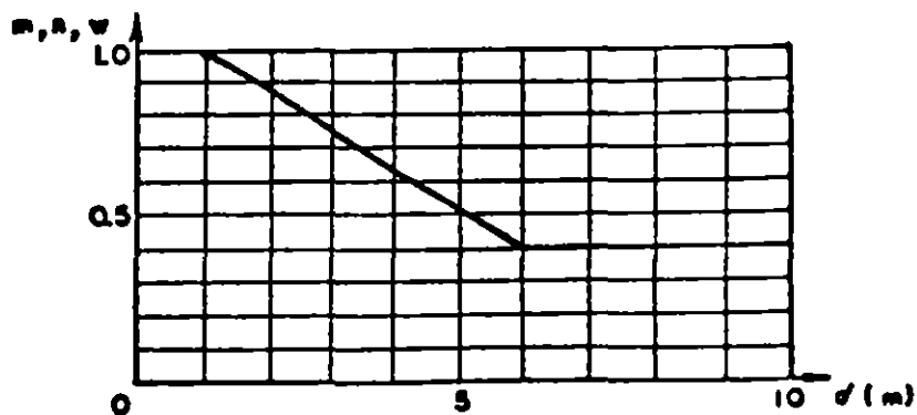
GRAFICA No. 4.1. VALORES DE LOS EXONENTES m y n PARA CORRECCION POR DENSIDAD DEL AIRE Y w PARA CORRECCION POR HUMEDAD, EN FUNCION DE LA DISTANCIA DISRUPTIVA d .
