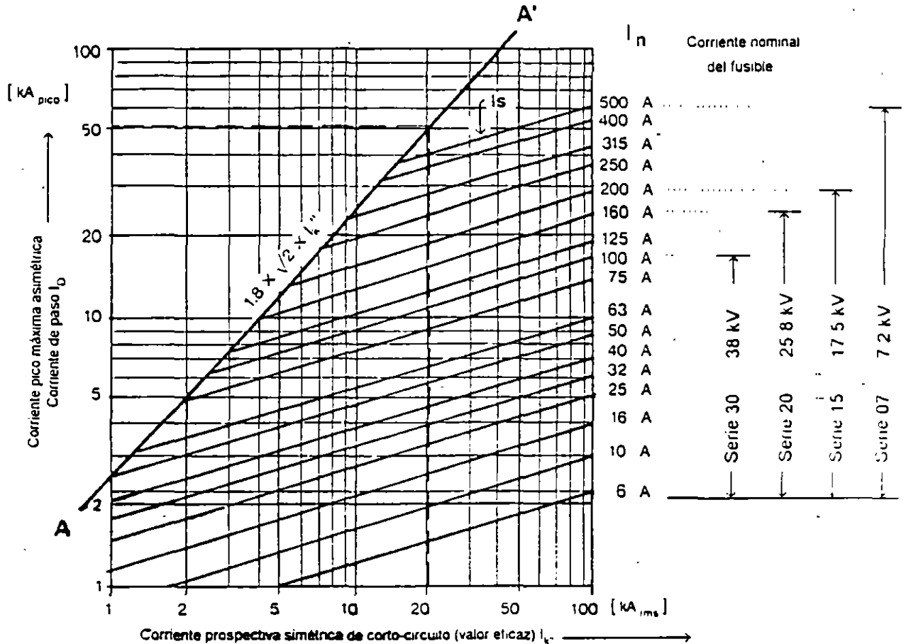
FIGURA 5 Diagrama de corriente máxima de paso I_D referida a la corriente prospectiva de corto-circuito I_k .
