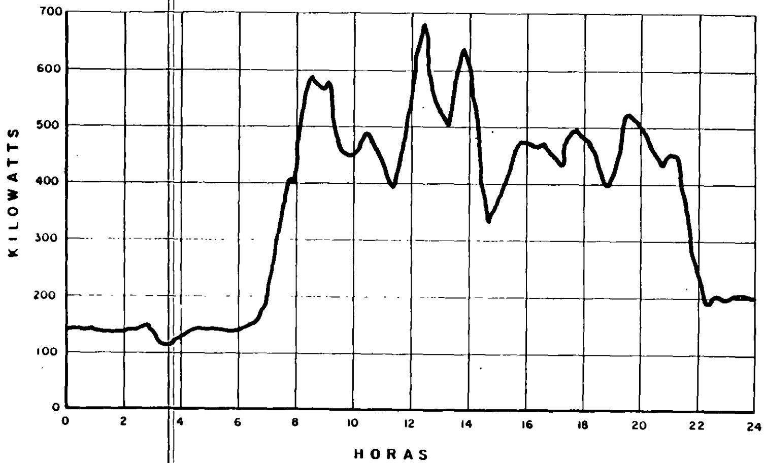
FIGURA 5 2 PERFIL DE DEMANDA (DOS TURNOS DE OPERACION)
