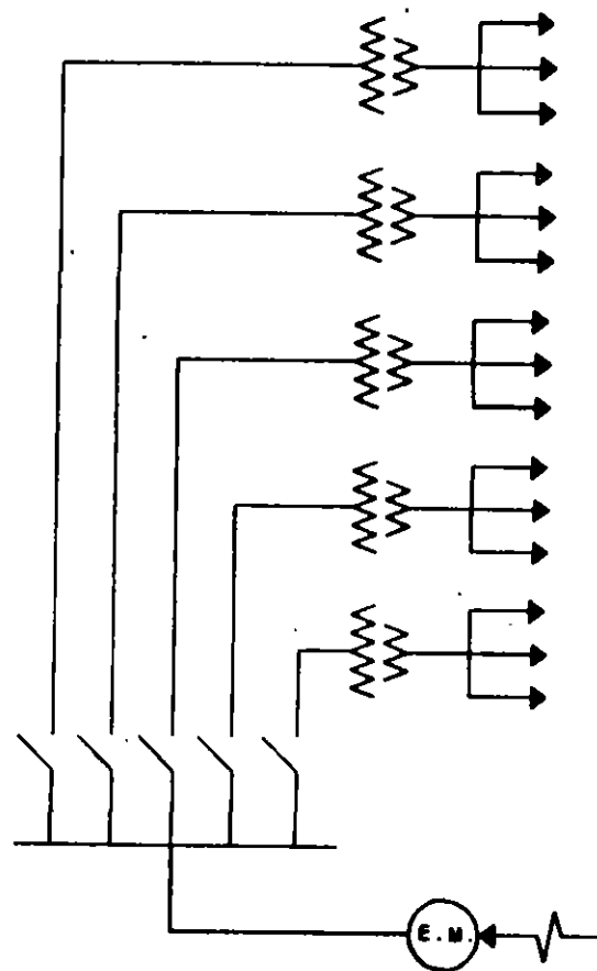
b) Un usuario en M.T. con transformadores en varios niveles, alimentador radial, varios alimentadores.
