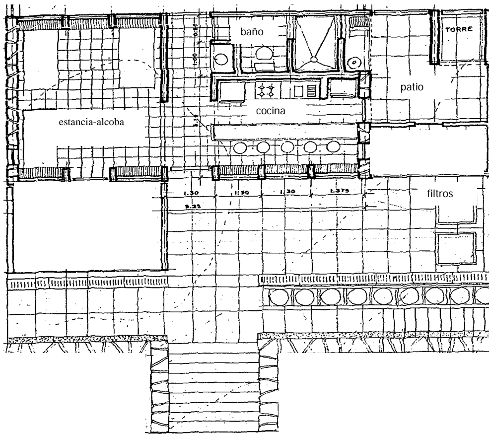
Figura 75 Planta arquitectónica de la vivienda
