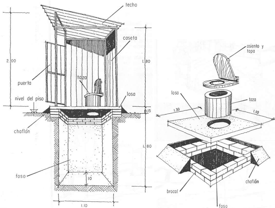
Figura 49 Elementos constitutivos de una letrina
