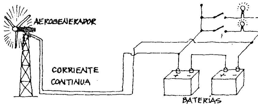
Figura 45 Sistema de almacenamiento por baterías para instalaciones de baja potencia
