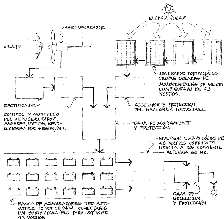
Figura 46 Sistema de generación de electricidad con sistema combinado de fotoceldas y aerogenerador
