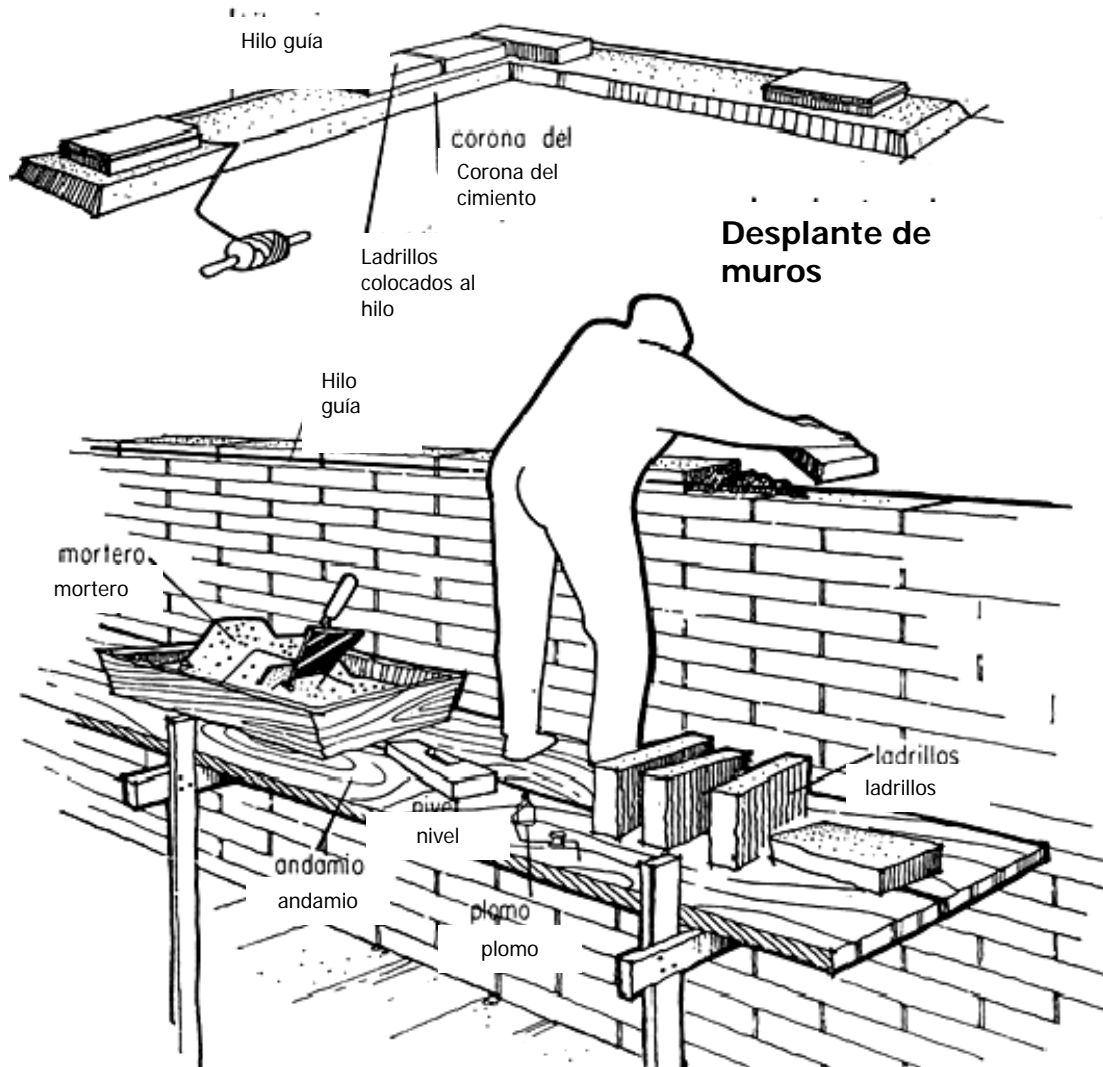
Figura 19 Construcción de un muro de ladrillos
