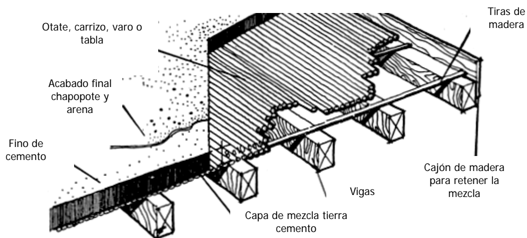
Figura 24 Techumbre de tierra-cemento
