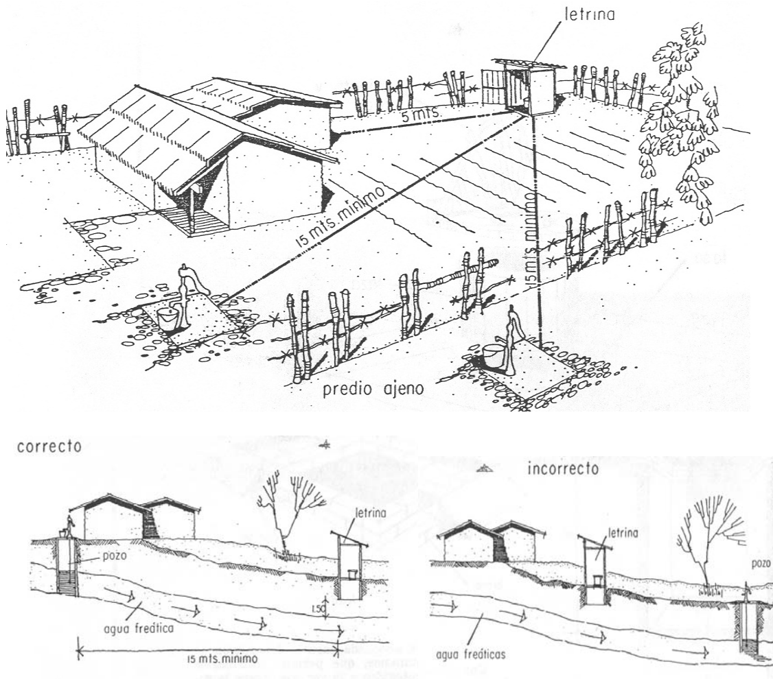
Figura 50 Localización adecuada de una letrina dentro de un predio
