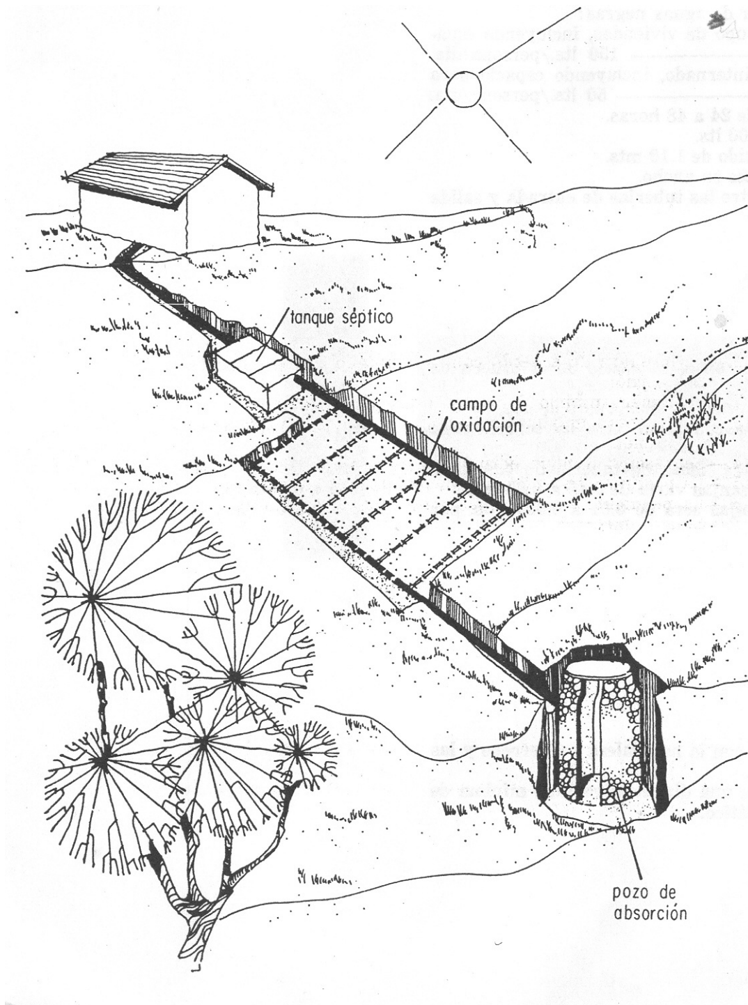
Figura 61 Esquema general de una fosa séptica
