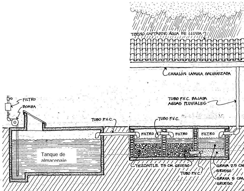
Figura 77 Sistema de captación y conducción del agua pluvial
