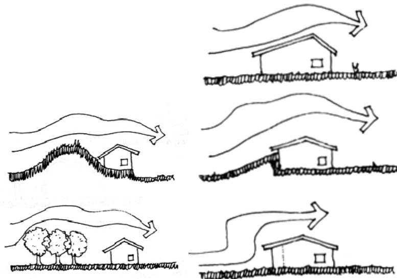
Figura 7 Protección de la casa de vientos
