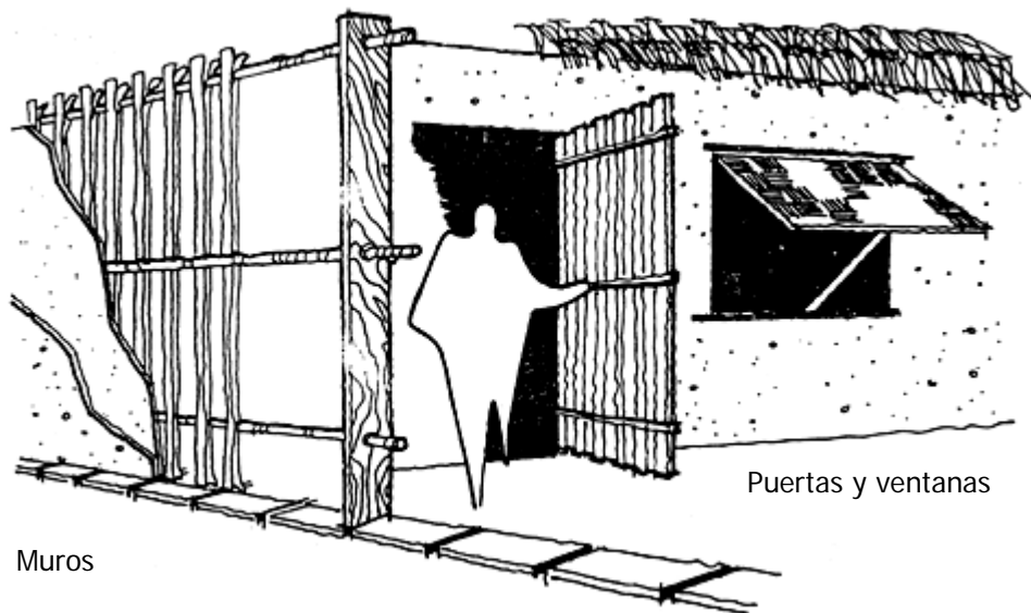
Figura 17 Ejemplo de casa construida con muros de bambú
