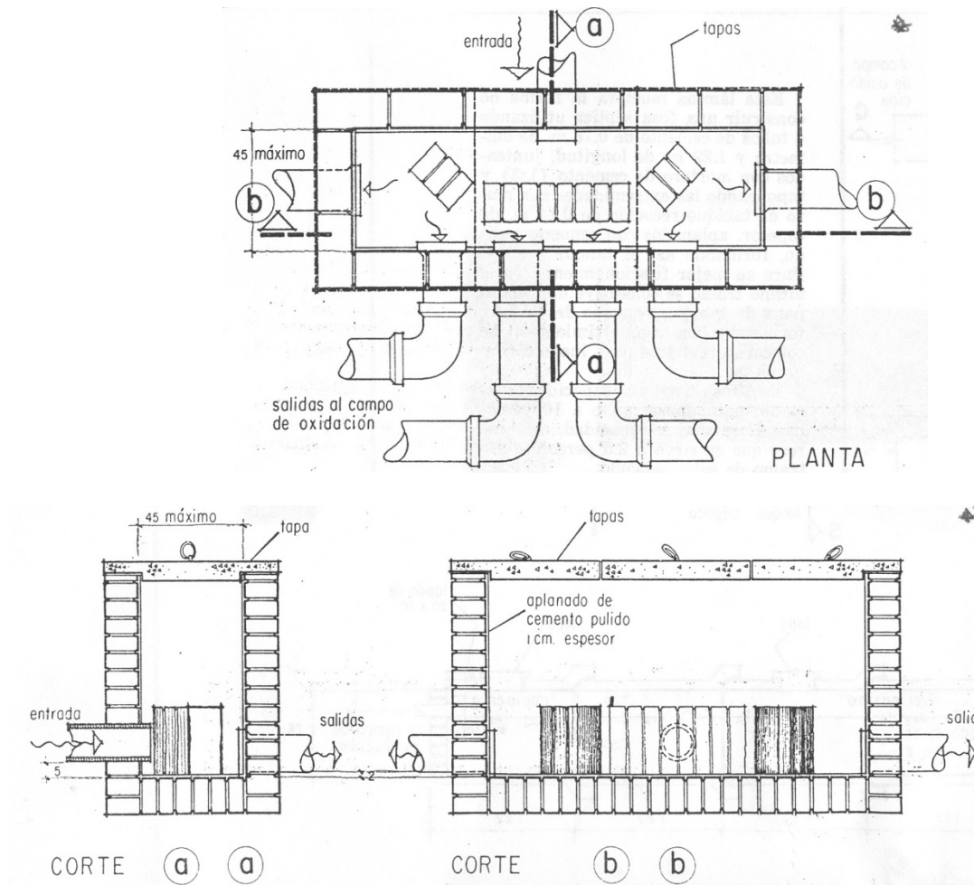
Figura 64 Caja de distribución tipo
