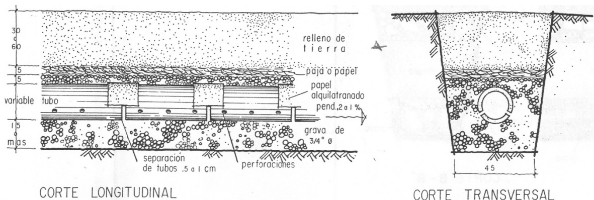
Figura 65 Instalación de tubería
