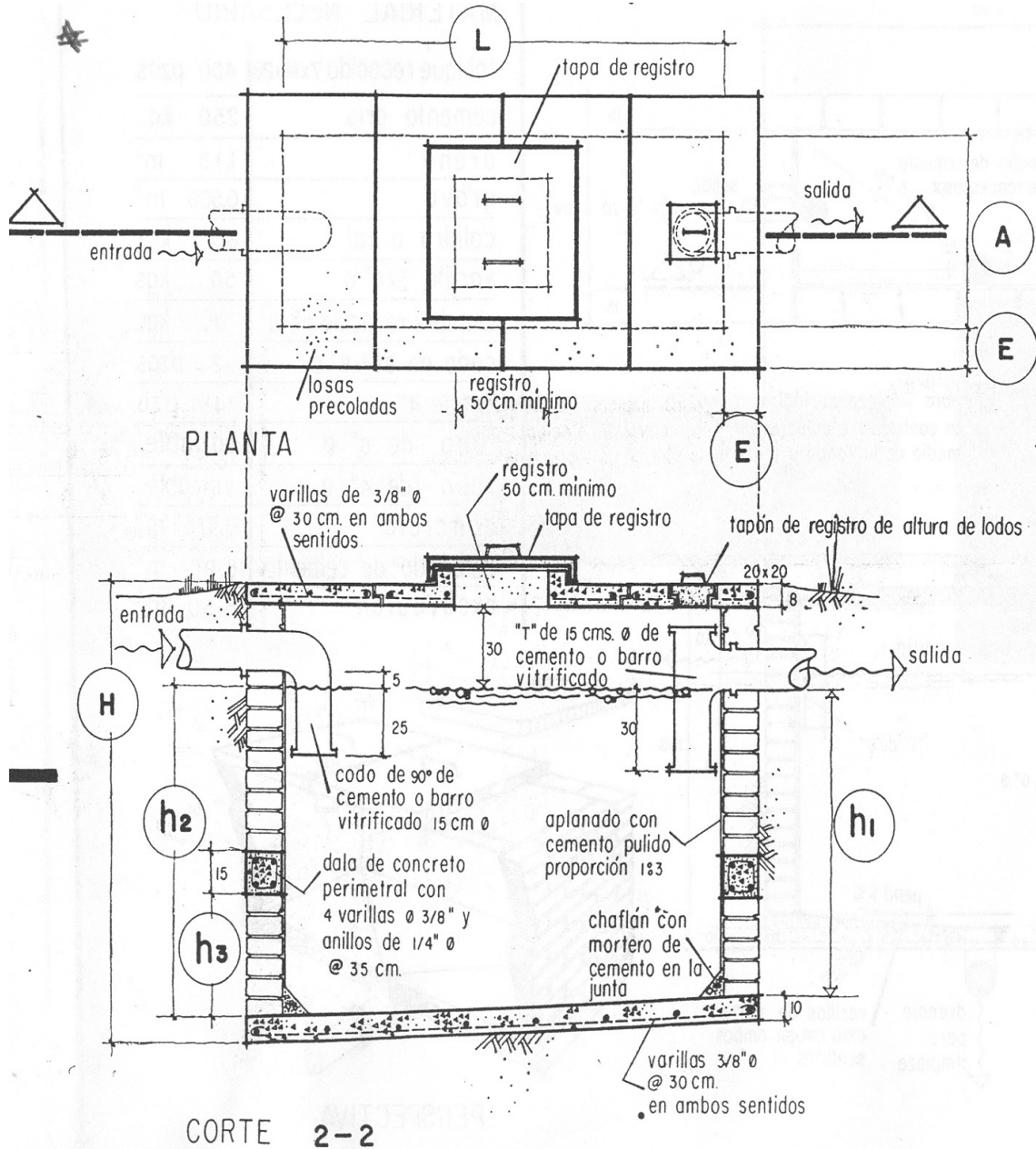
Figura 63 Tanque séptico tipo
