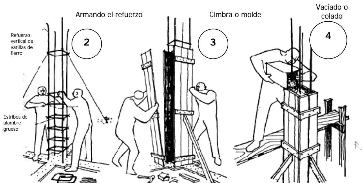
Figura 21 Construcción de castillos de concreto
