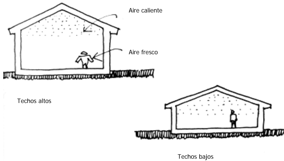
Figura 6 Distribución del calor en los cuartos de la vivienda
