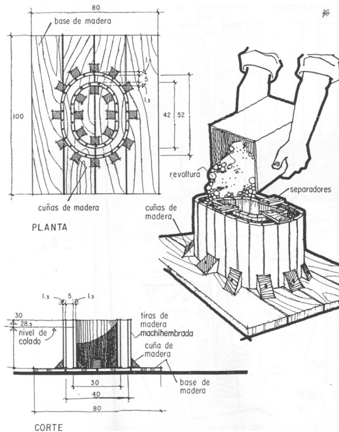
Figura 56 Moldes de madera para taza
