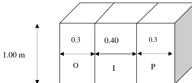
Figura 80. Separador de desechos
