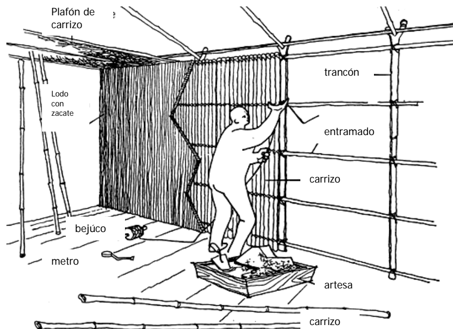
Figura 18 Construcción de un muro de carrizo
