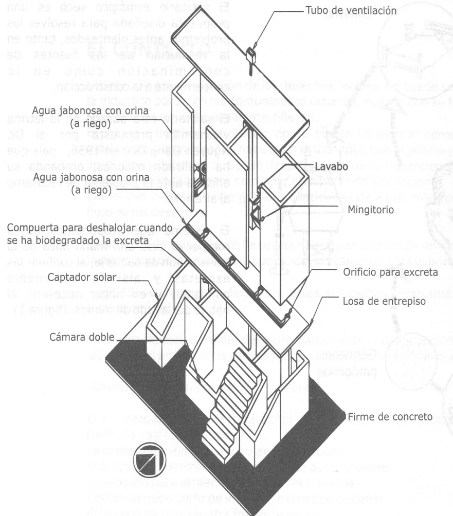
Figura 68 Componentes del sanitario ecológico seco
