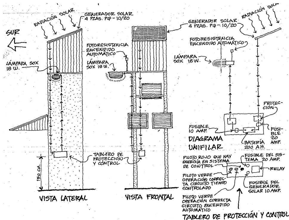
Figura 79 Torre de generación de energía para luminaria solar
