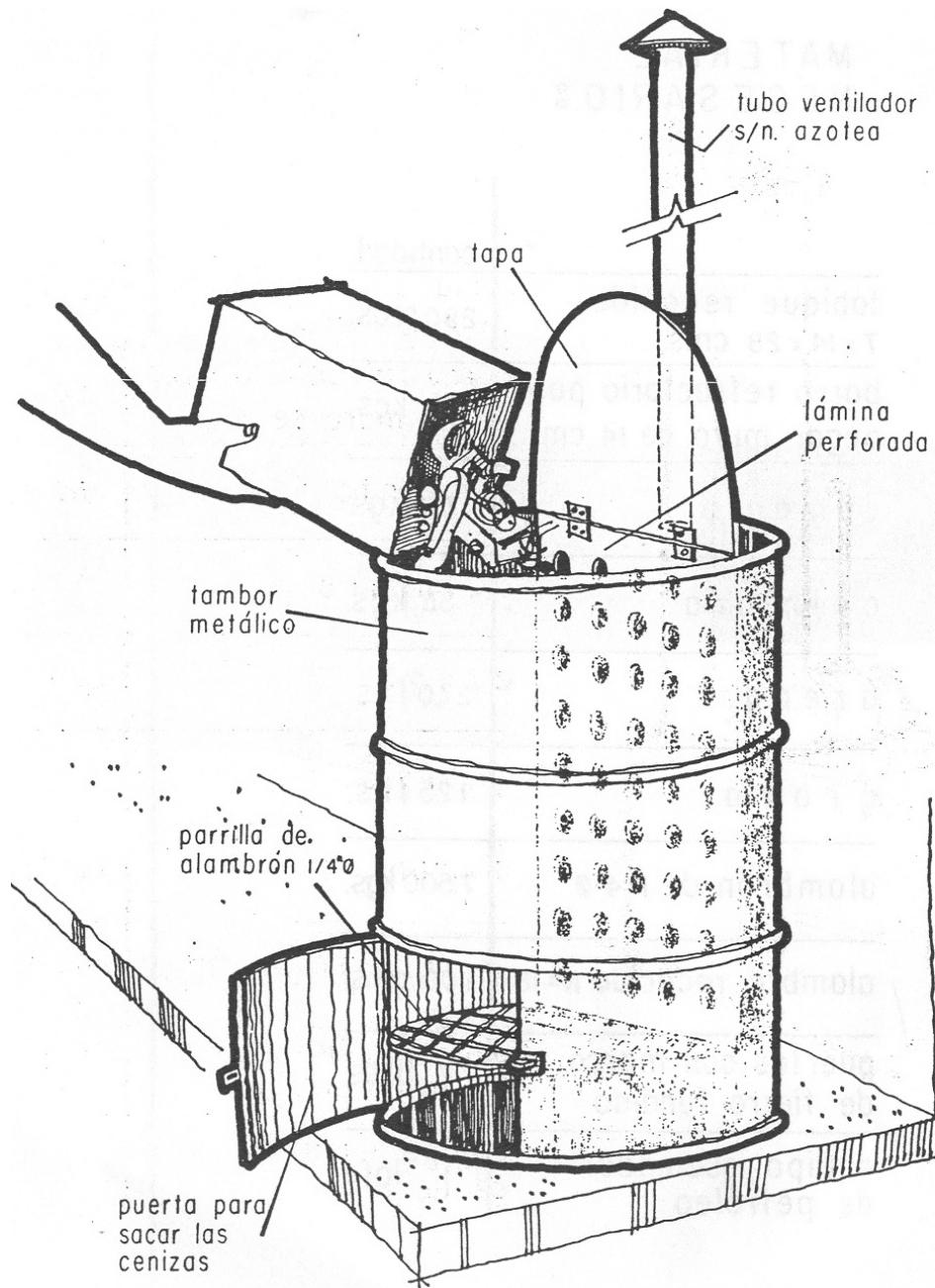
Figura 72 Quemador doméstico para basuras
