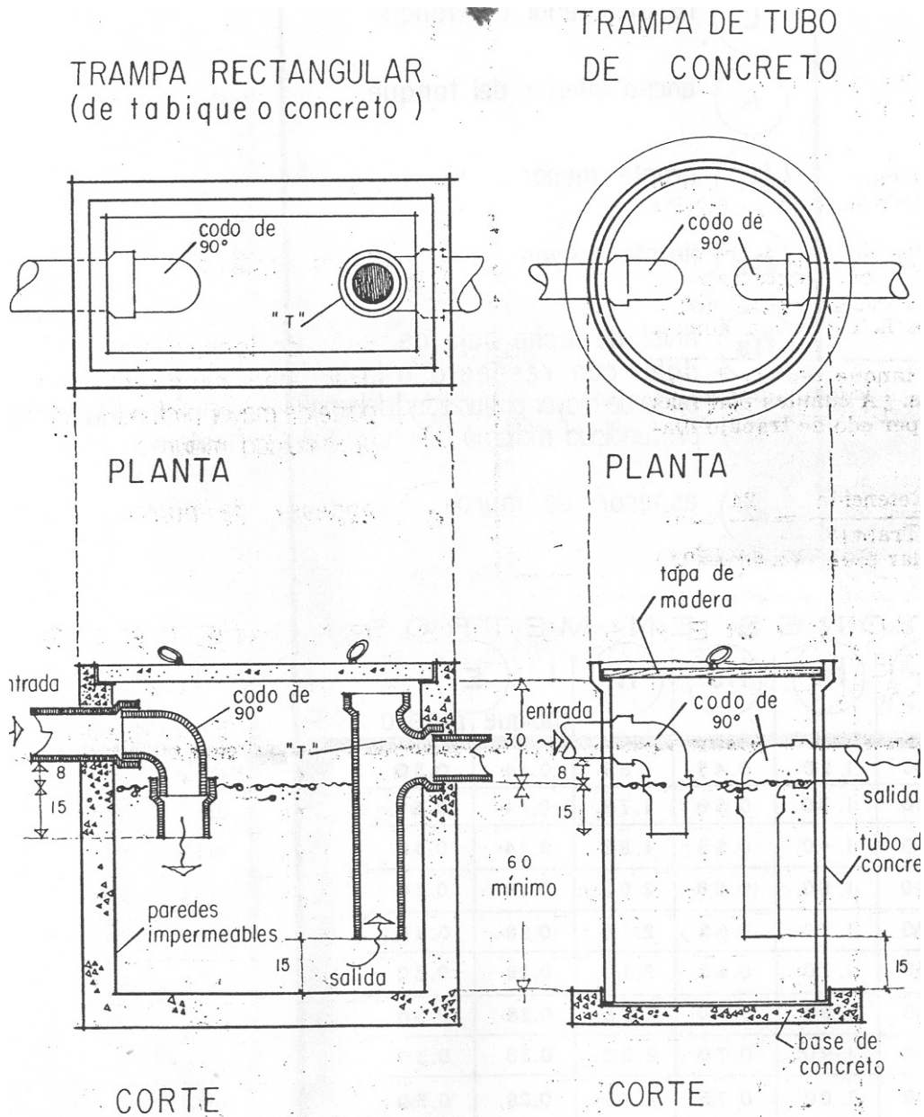
Figura 62 Trampas para grasa
