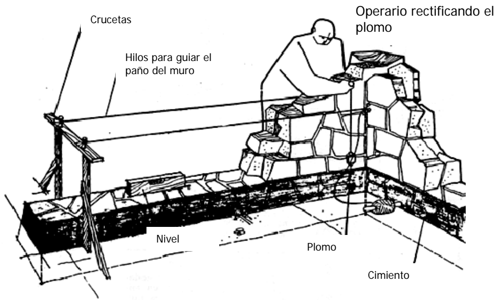
Figura 16 Inicio del proceso de construcción de un muro
