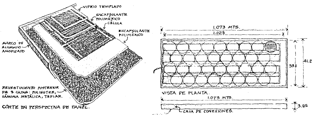
Figura 33 Panel o módulo fotovoltaico
