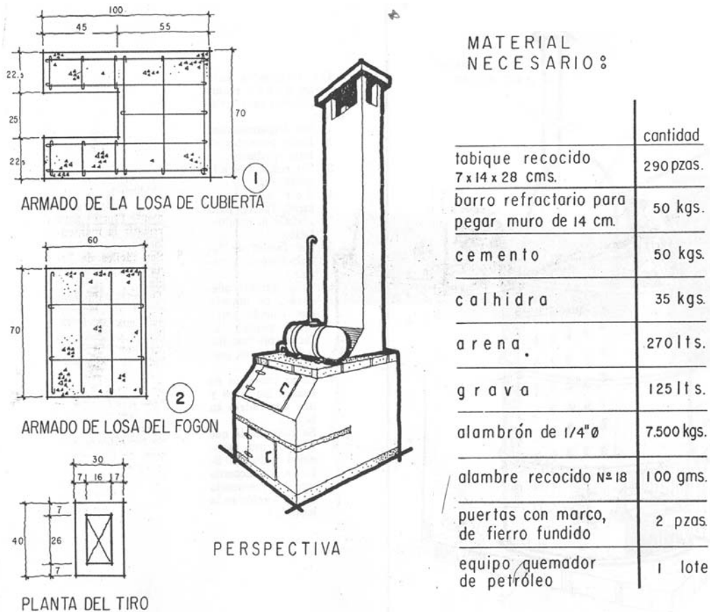
Figura 71 Incinerador
