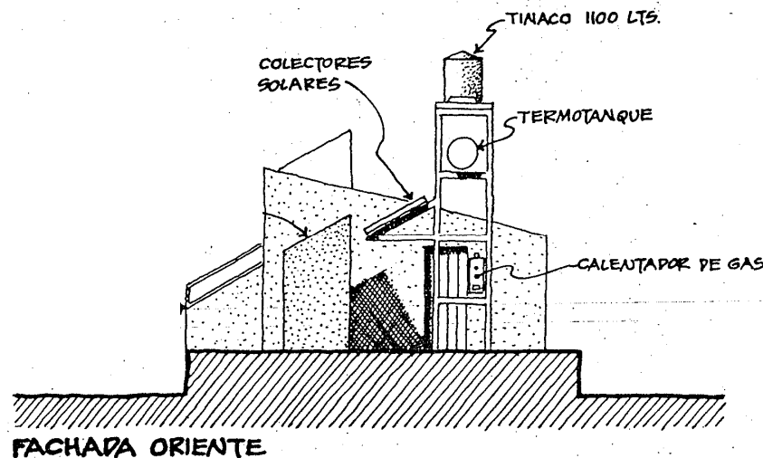
Figura 76 Fachada oriente de la vivienda
