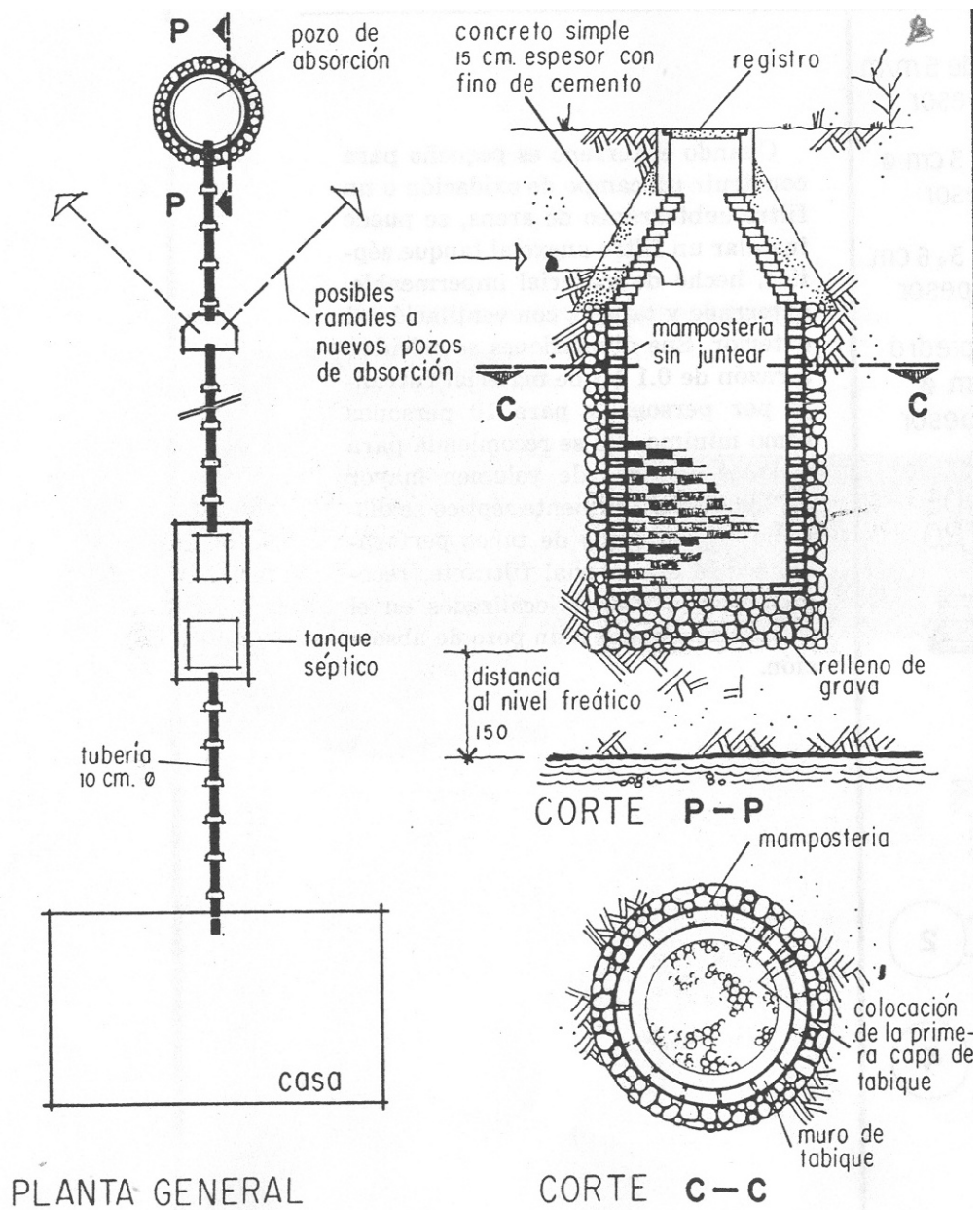
Figura 66 Pozos de absorción
