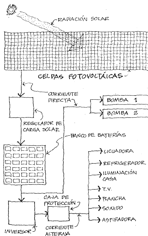
Figura 31 Diagrama de generación de energía solar fotovoltaica
