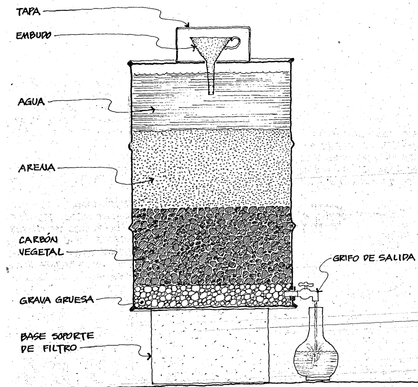
Figura 78 Filtro de agua para la potabilización
