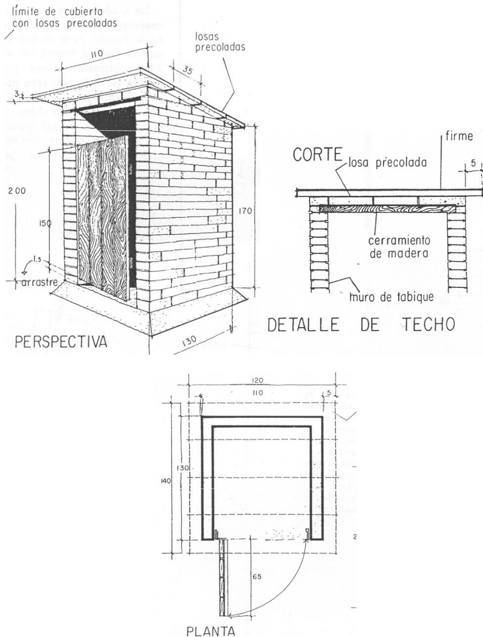
Figura 58 Caseta de tabique
