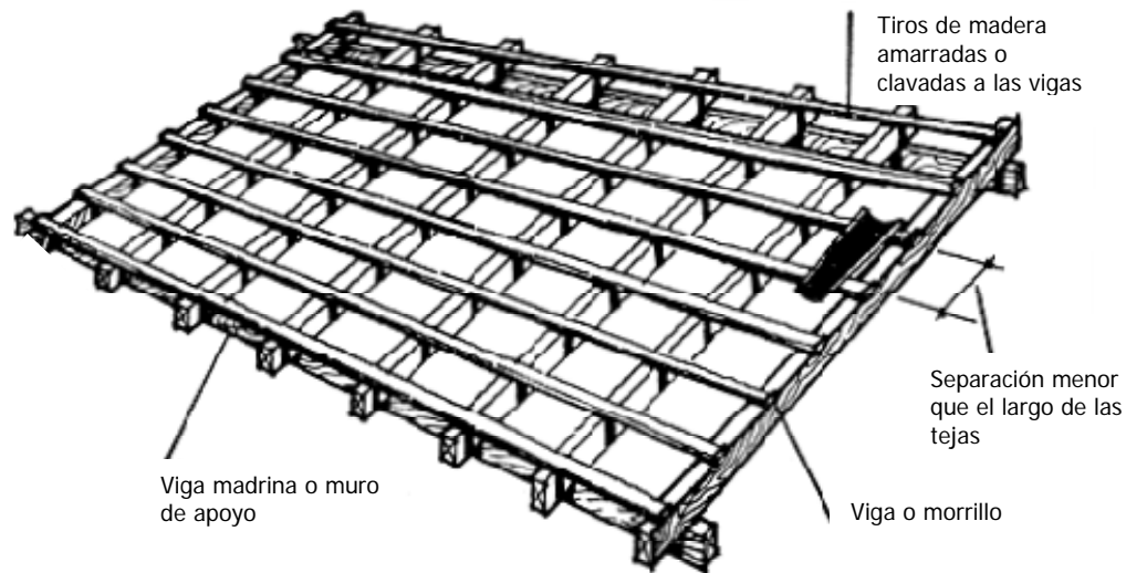
Figura 23 Techumbre realizada de tierra
