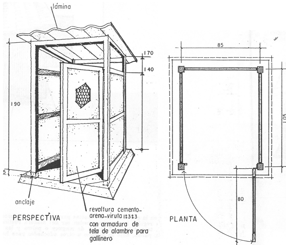
Figura 59 Caseta prefabricada
