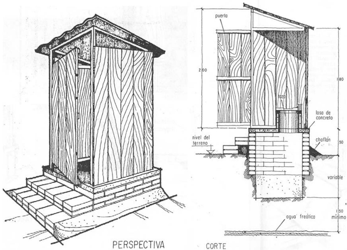
Figura 60 Letrina elevada
