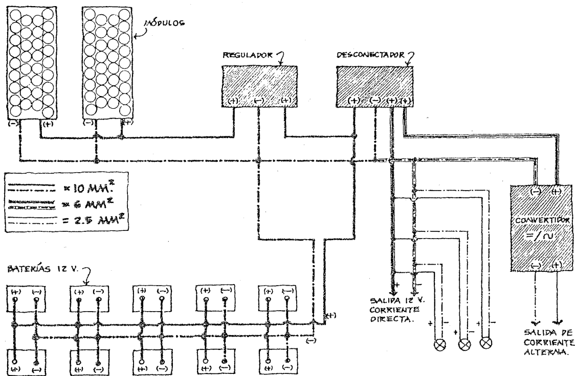
Figura 35 Esquema de montaje de un sistema solar fotovoltaico Kontakt
