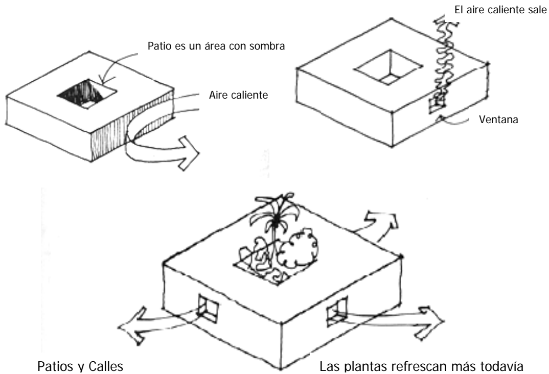
Figura 1 Formas de distribuir una vivienda para obtener una ventilación confortable
