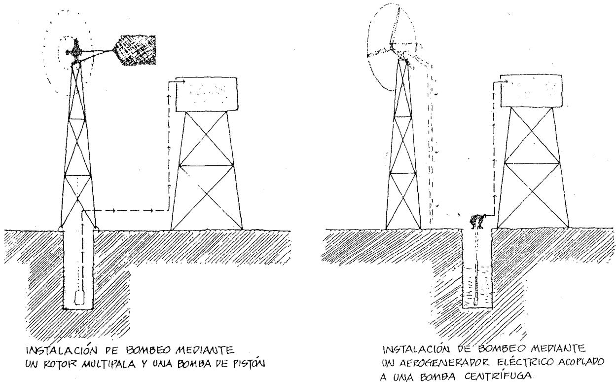
Figura 41 Instalación de bombeo
