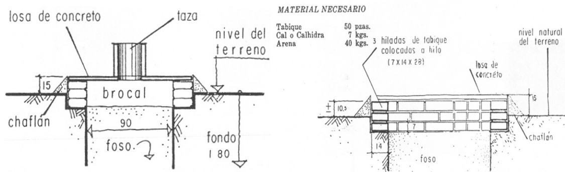
Figura 52 Tipos de brocales
