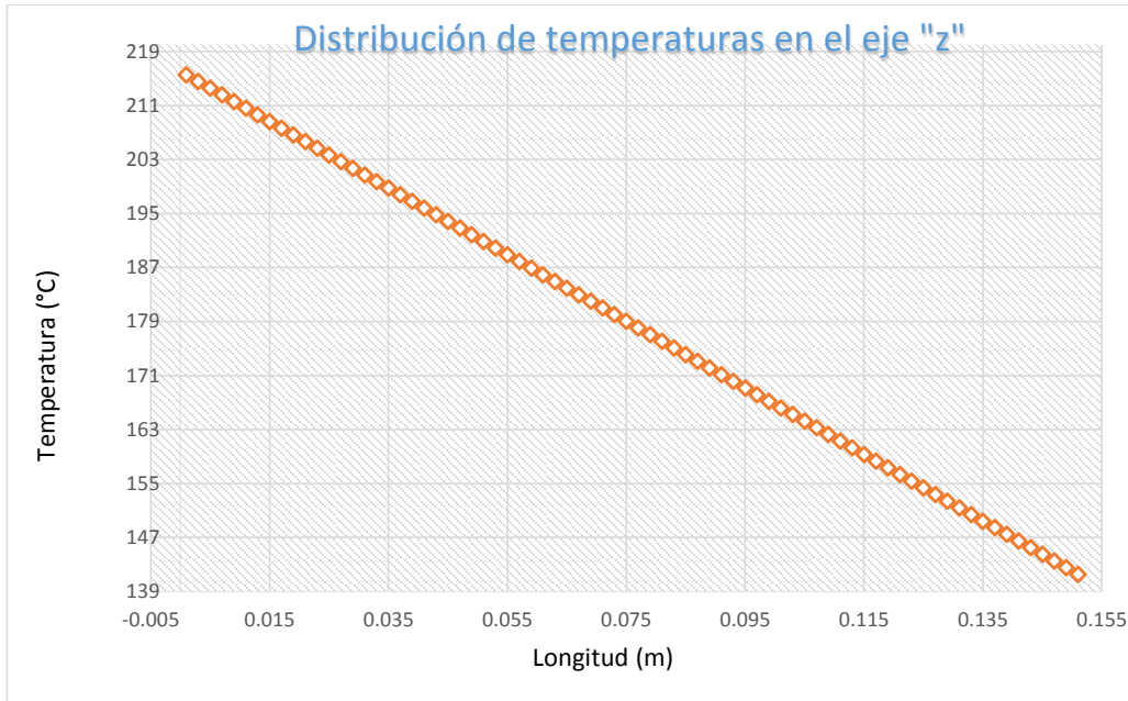
Gráfica III. 2 Distribución de temperaturas en "z"
