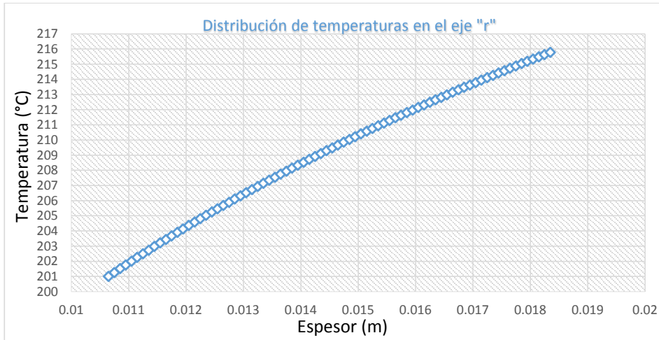
Gráfica III. 1 Distribución de temperaturas en "r"
