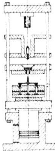
Figura I.5 Máquina de Inyección Hidráulica vertical
