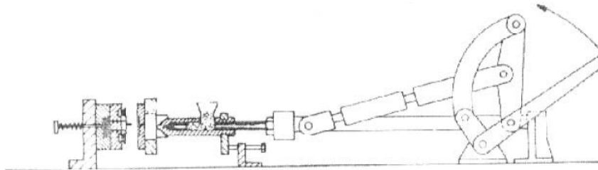
Figura I.4 Inyectora Manual Horizontal Con Sistema Hidráulico
