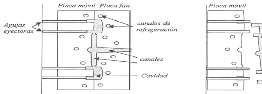
Figura 1.2 Partes del molde de inyección
