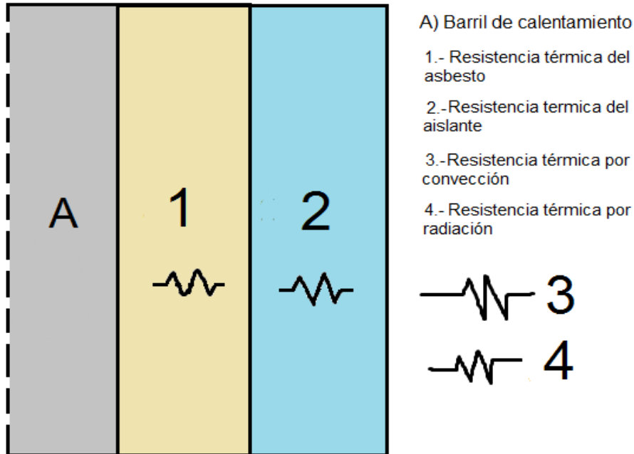
Figura III.1 Representación del orden de las resistencias térmicas en un corte vertical del cilindro de calentamiento, presentando la parte derecha debido a la simetría existente.
