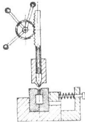
Figura 1.3 Máquina Manual accionada con cremallera y piñón
