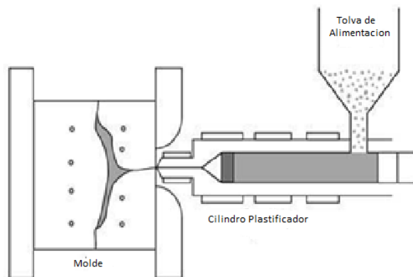
Cilindro Plastificador y Molde
