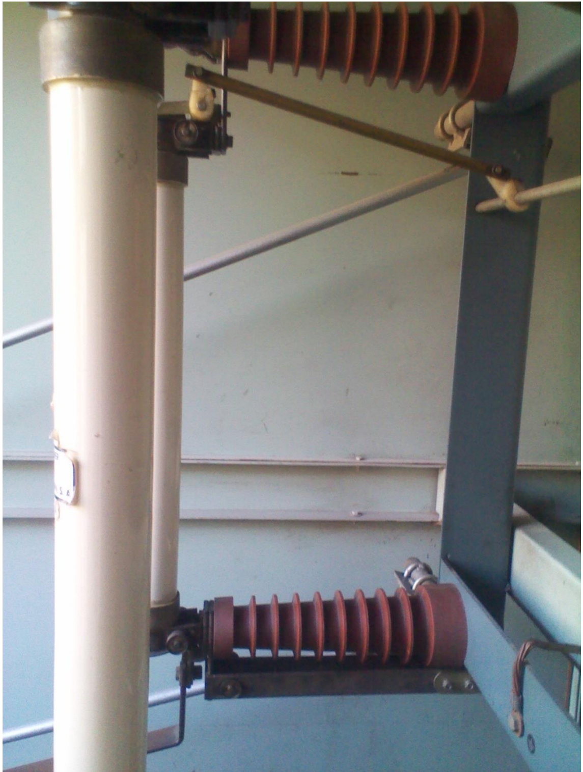
Figura 4-10 Fusibles para el transformador Tx.
