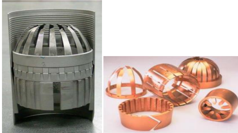
Figura 1.5. Catcher de núcleo.
