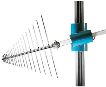
Figura A-8: Antena R&S HL223
