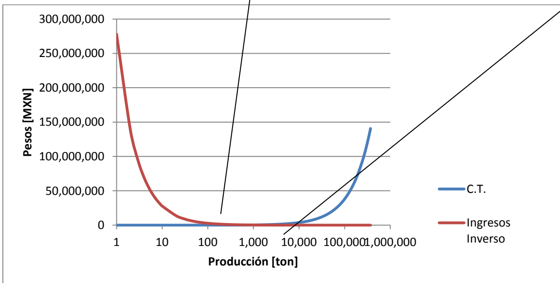
Figura 5.7 Gráfica C.T. vs ingresos.
