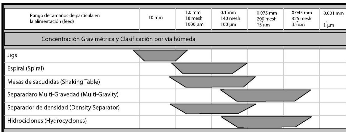
Figura 6.4 Clasificación de los separadores por gravedad más comúnmente usados, basados en el tamaño de las partículas de la alimentación.
