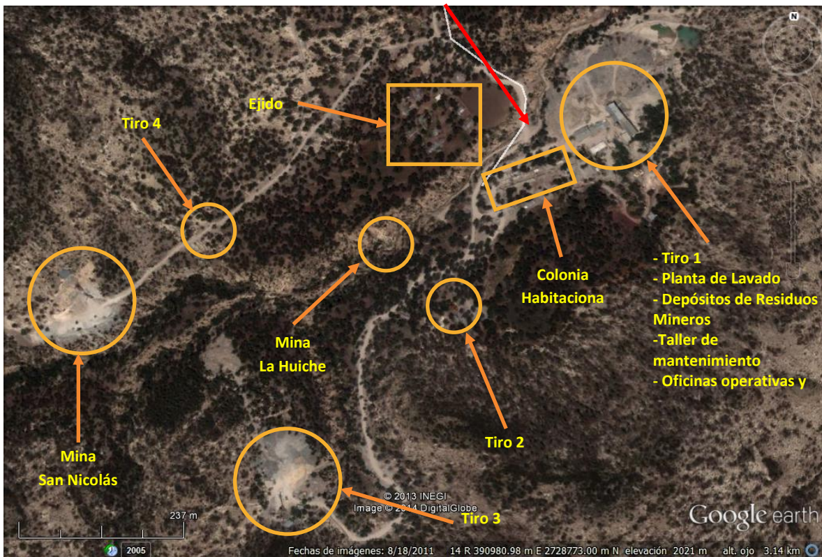
Figura 7.1 Instalaciones del fundo minero. [20]
