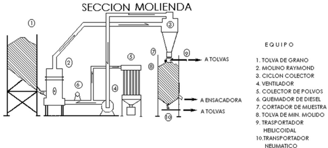
Figura 6.11 Circuito de molienda. [26]
