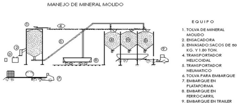
Figura 6.12 Manejo y transporte interno del mineral. [26]
