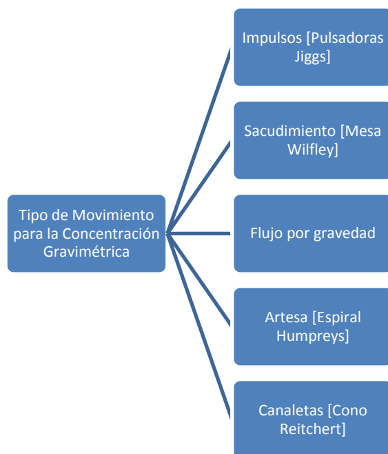
Figura 6.2 Clasificación de movimientos en la concentración gravimétrica.
