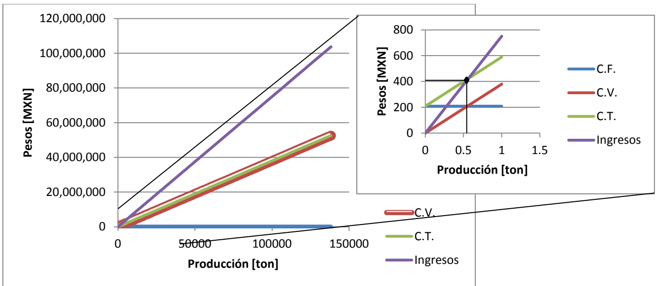
Figura 5.2 Gráfica de tonelaje vs. Ingresos mina.
