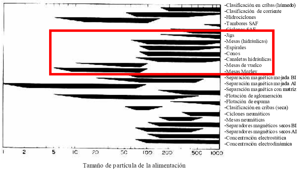
Figura 6.3 Capacidad de concentrar de los diversos equipos gravimétricos. [18]
