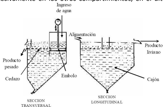
Figura 6.5 Esquemización de los jigs tipo Hazard.
