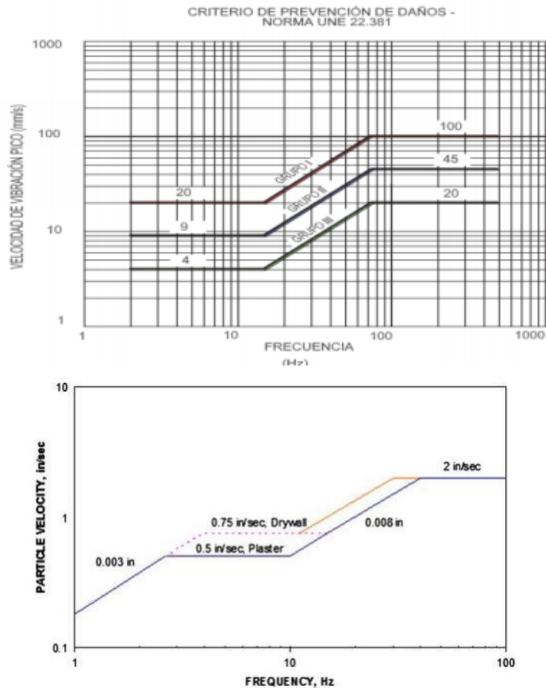
Figura 5.10 Criterios de prevención de daños por vibración.
