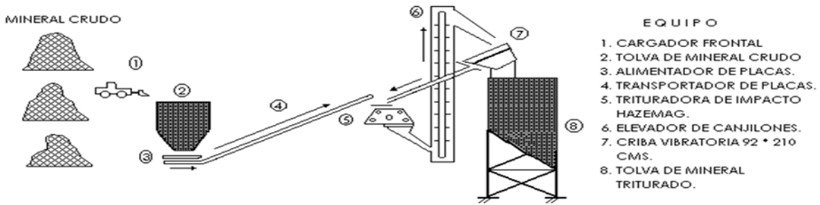
Figura 6.10 Circuito de trituración. [26]
