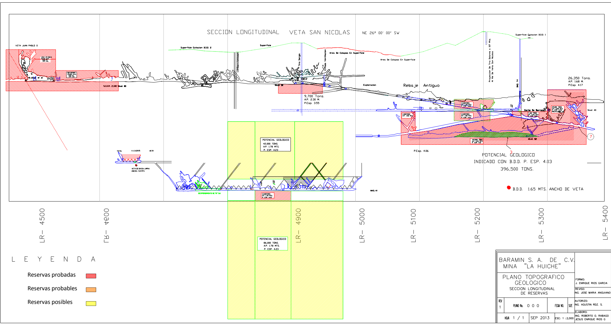
Figura 4.6 Sección longitudinal con bloques de reservas identificados en San Nicolás. [11]
