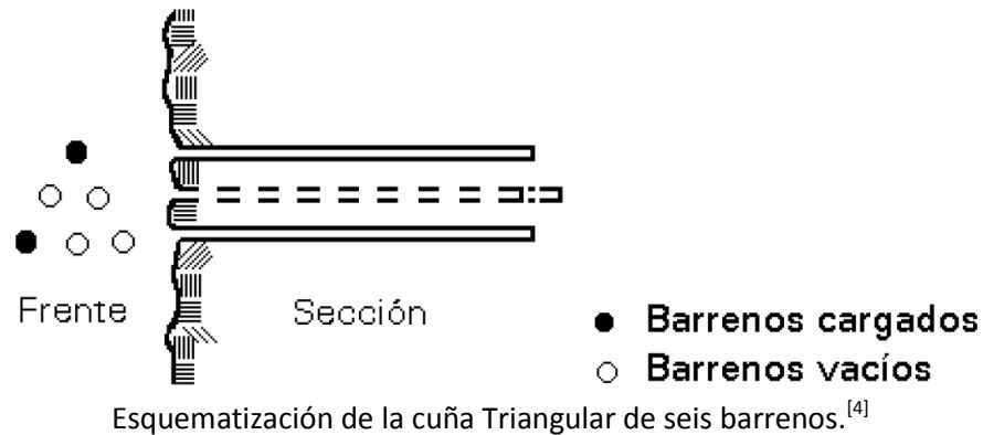
Figura 5.9 Esquema de la cuña de seis barrenos triangular. [12]
