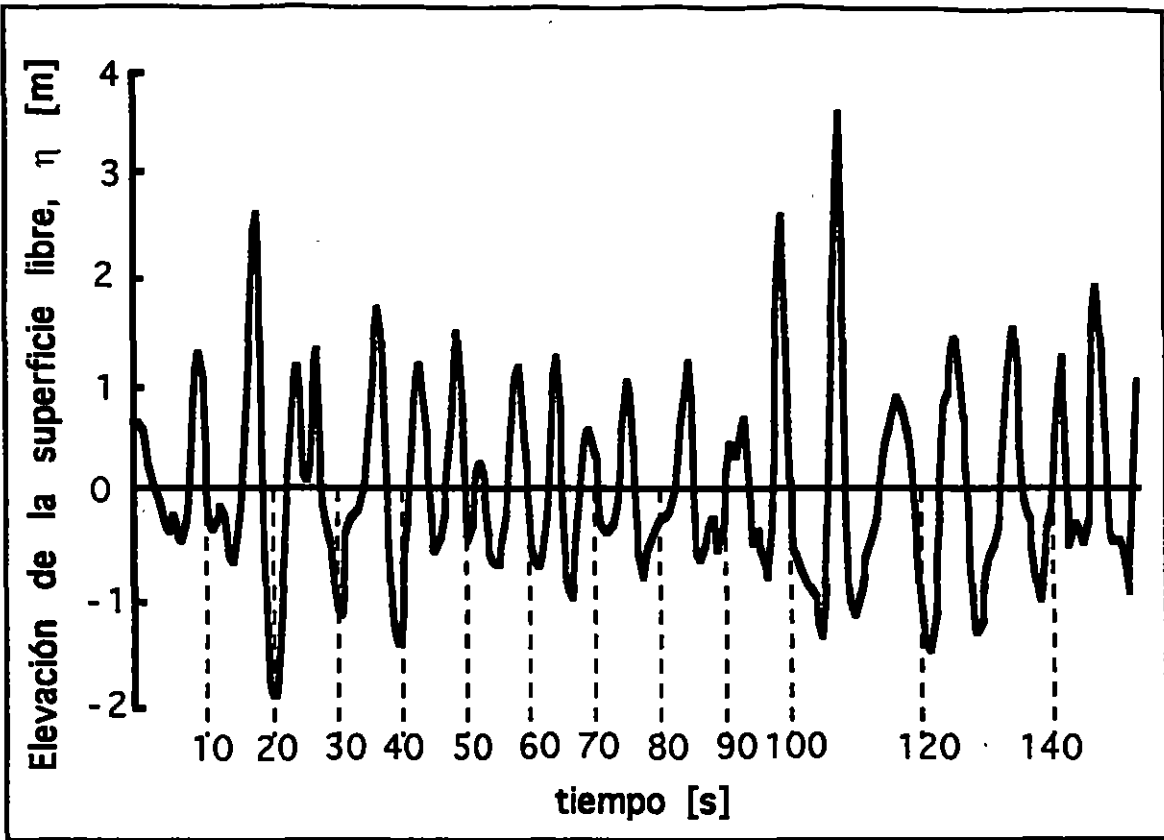
Ejemplo de un registro de oleaje (fuente: Goda, 1985).
