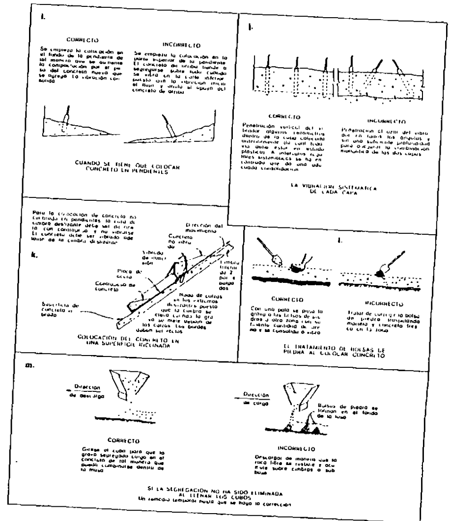
Fig. 6.1. (l-m) Métodos correctos e incorrectos de consolidación.
