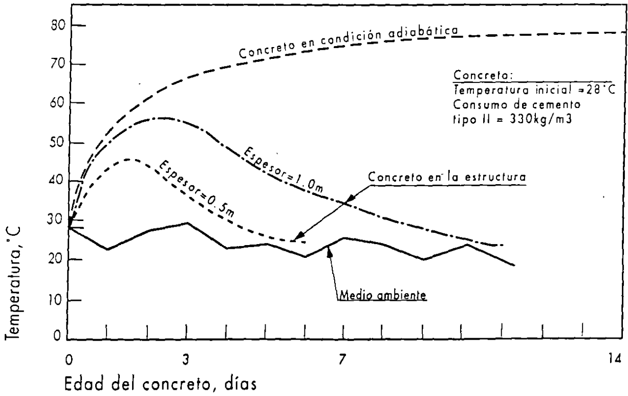
Fig. 12--Evolución del calor interno en varias condiciones
