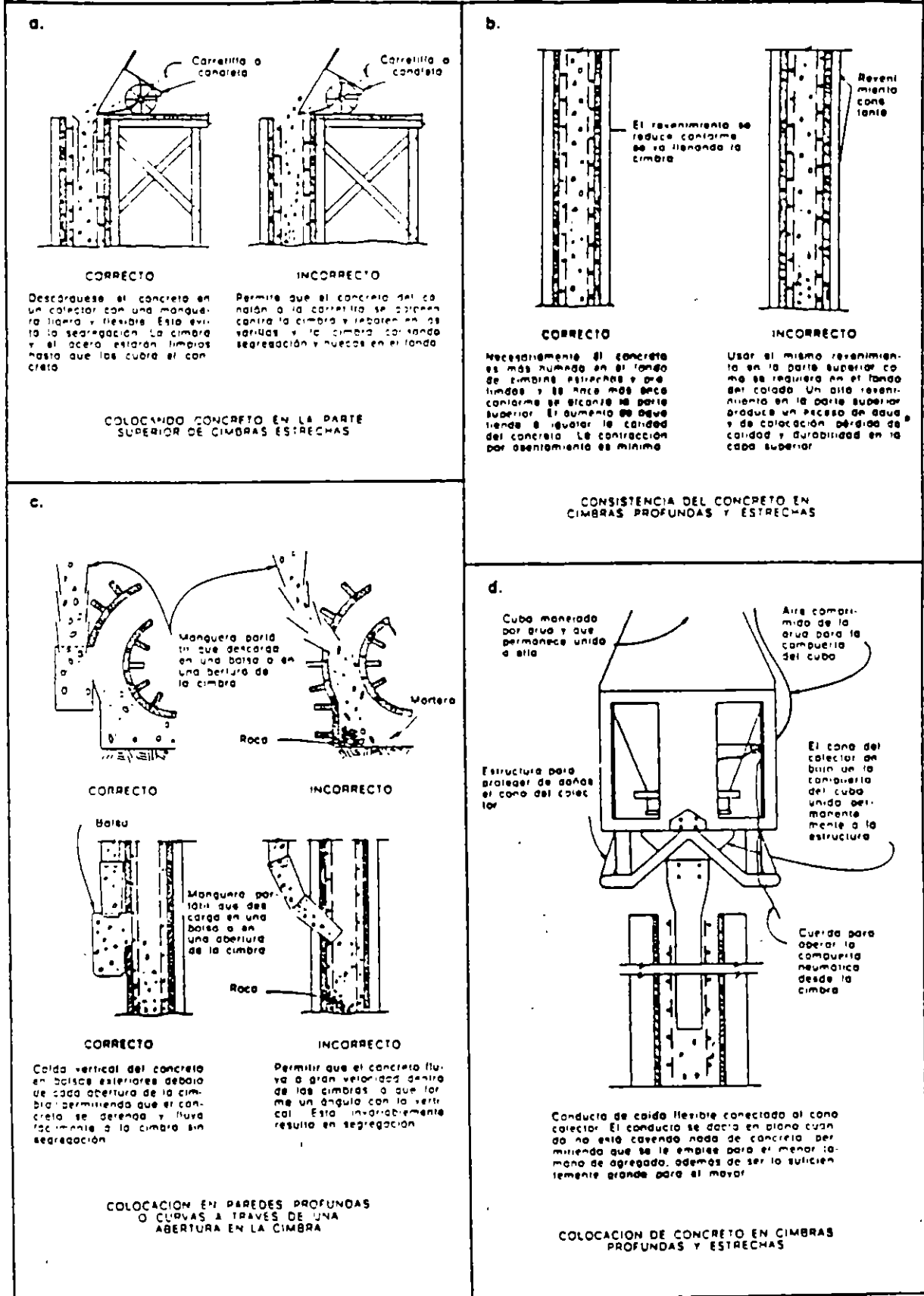
Fig. 6.1 (a-d) Métodos correctos e incorrectos de colocar concreto.
