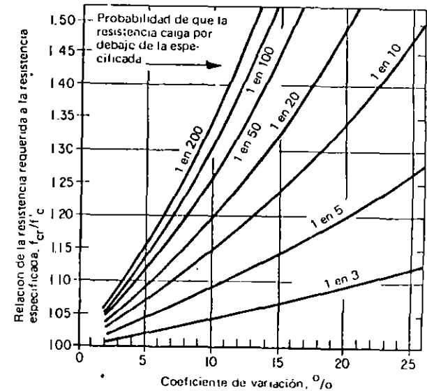
Fig. 4.1 (a).— Relación de la resistencia promedio requerida f_{cr} a la resistencia especificada f'_c para varios coeficientes de variación y probabilidades de que caigan por debajo de la resistencia especificada
