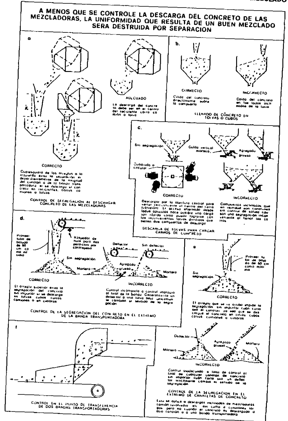
Fig. 4.8. Métodos correctos e incorrectos de manejo de con
