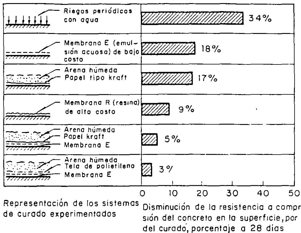
Fig. 7--Eficiencia de diversos sistemas de curado (12)
