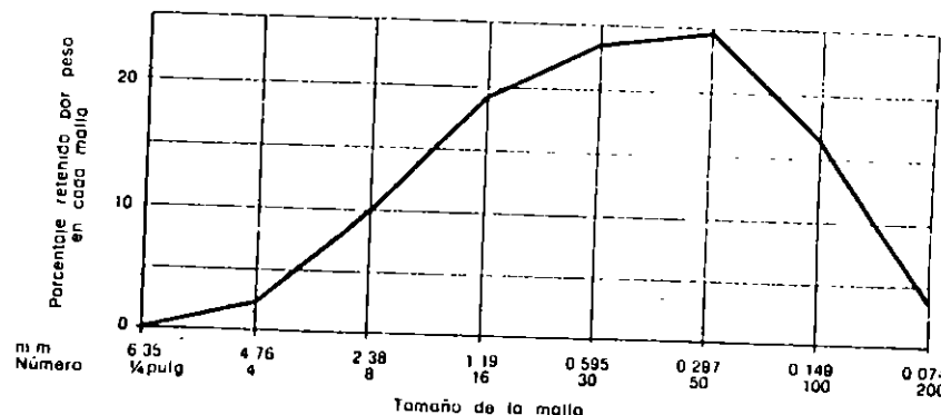
Fig. 9.4.2 b. Valores sugeridos de granulometría en cada malla para arena de peso normal para concreto bombeado.
