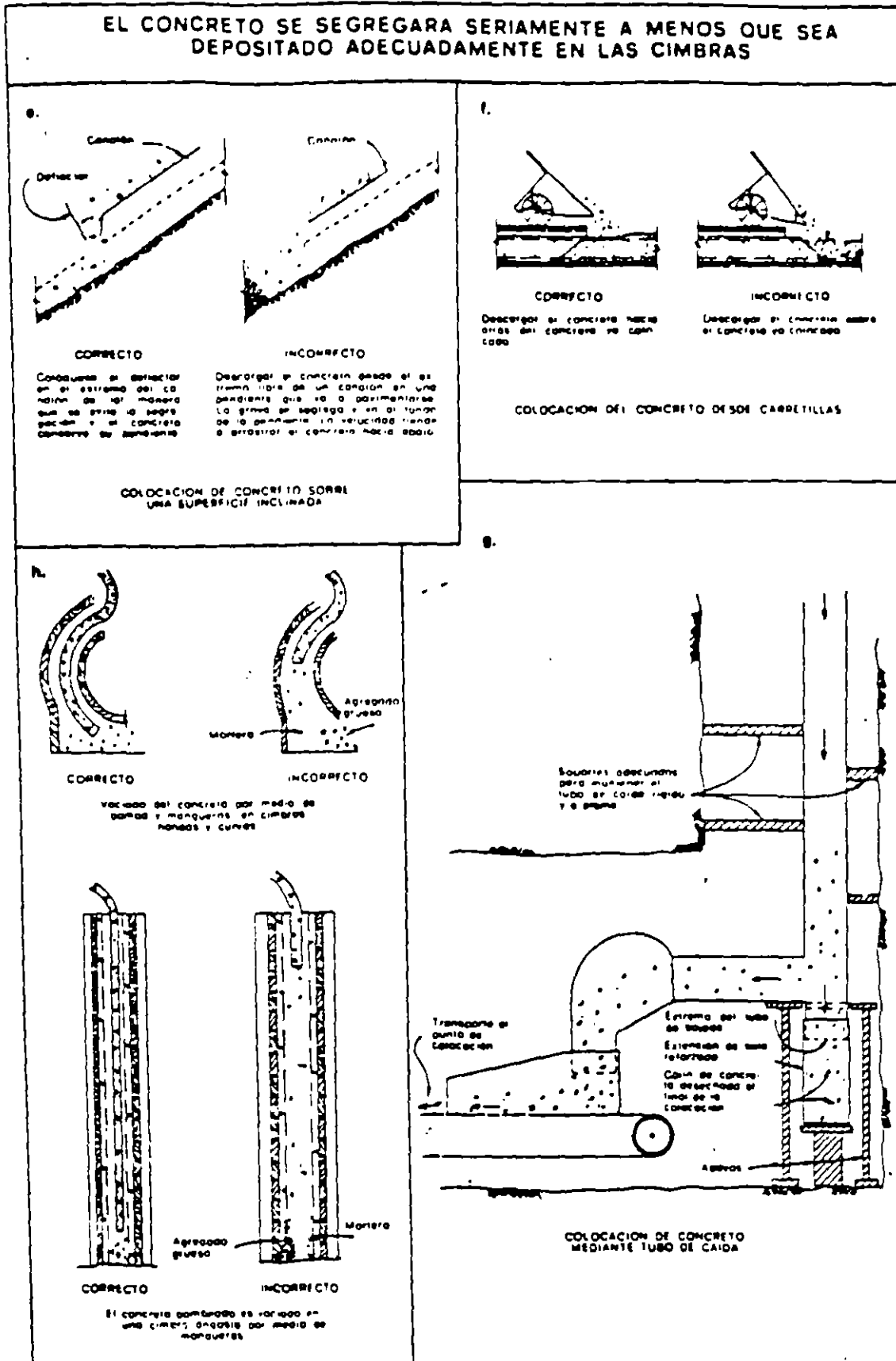
Fig. 8.1 (e-h) Métodos correctos e incorrectos de colocación de concreto.
