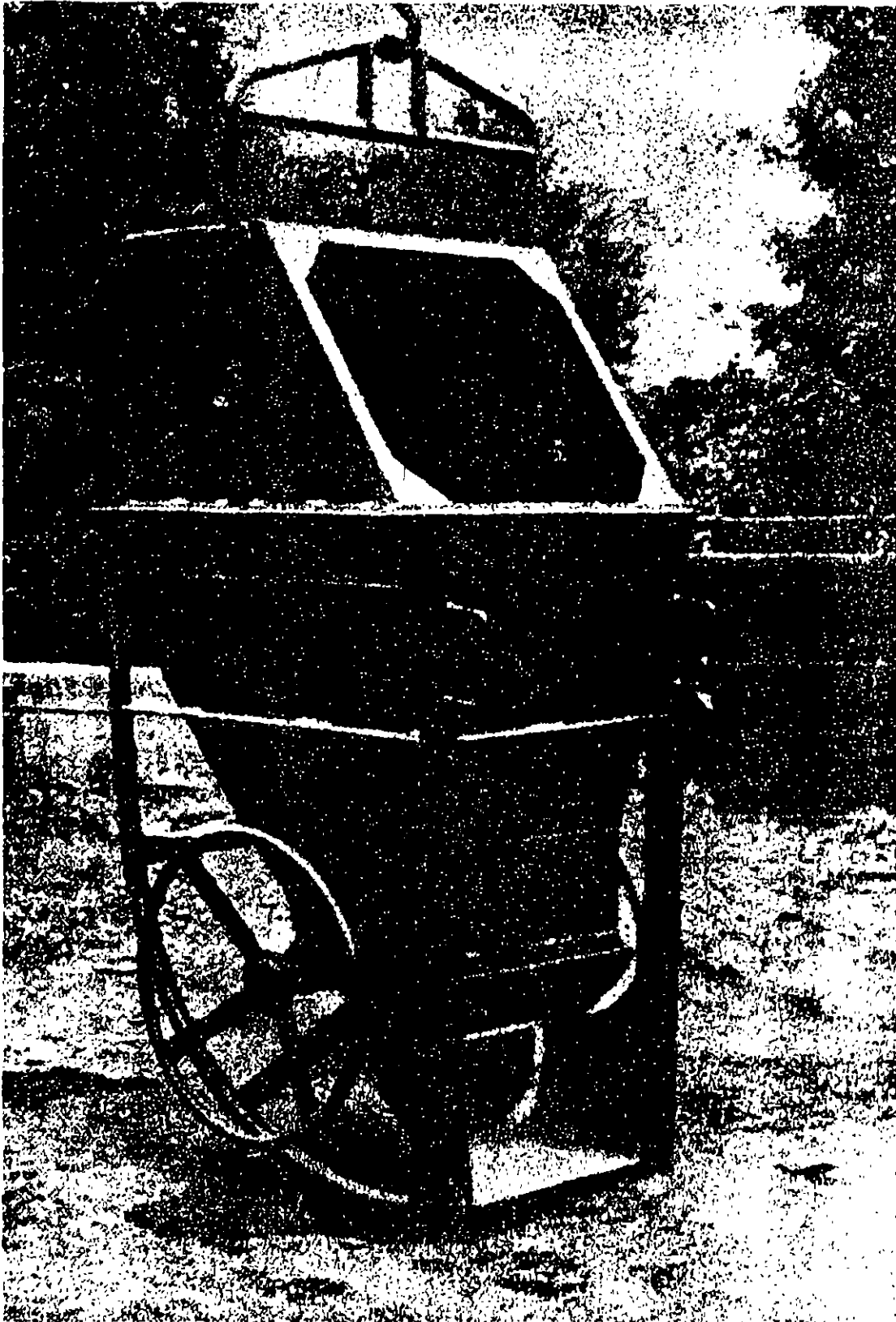
Toiva móvil de volteo (capacidad 0.75 m 3 ) con mecanismo de descarga de cierre de mordaza y abertura lateral con control de rueda
