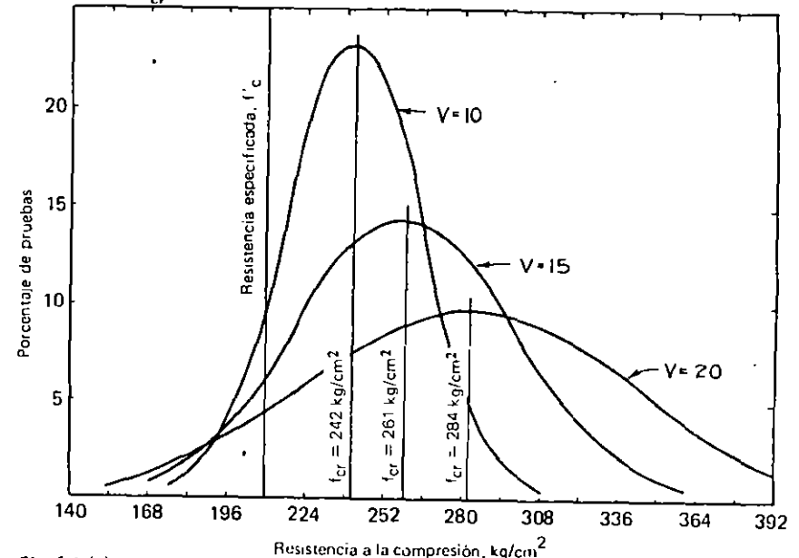
Fig. 4.1 (c).— Curvas normales de frecuencia para coeficientes de variación de 10, 15 y 20% /o
