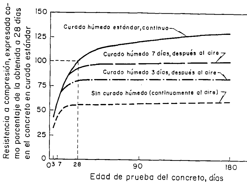
Fig. 5--Detrimento en la resistencia a compresión del concreto por falta de curado húmedo (9)
