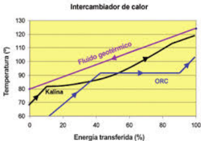
Figura 0.8 Comparación del perfil de temperatura del fluido de trabajo en un ciclo Rankine (ORC, en azul) y en un ciclo Kalina (en negro (Chamorro, 2009))
