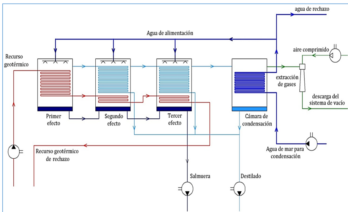
Figura 0.3 Desaladora modular geotérmica DMG
