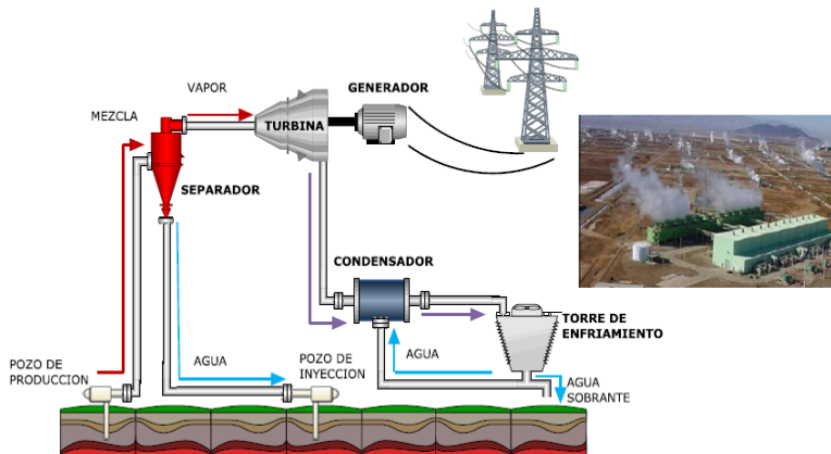
Figura 0.10 Ciclo a contrapresión
