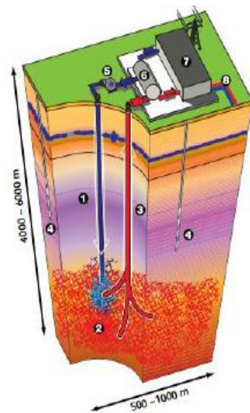
Figura 0.4 Sistemas de roca seca caliente Fuente (Llopis & Angulo, 2008)
