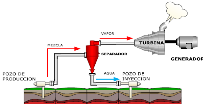
Figura 0.9 Ciclo a contrapresión
