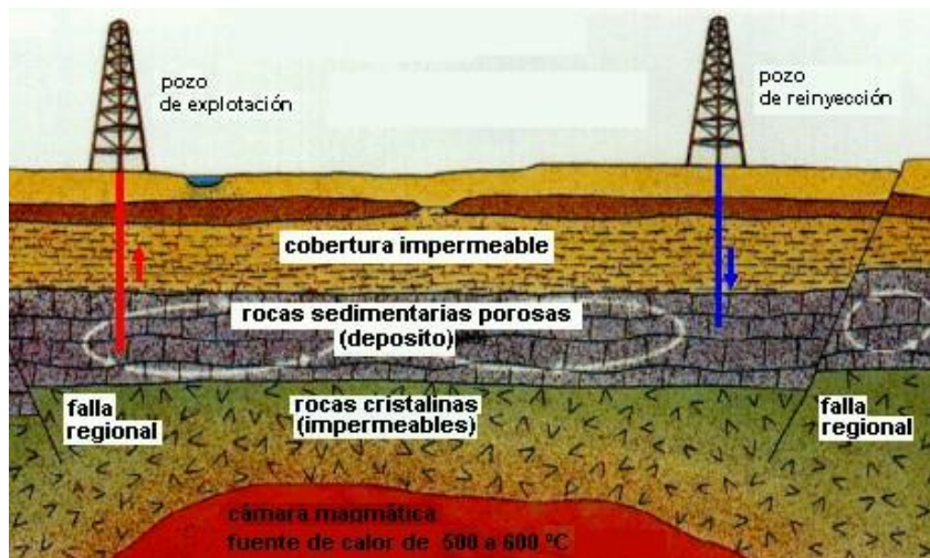
Figura 0.5 Sistemas geopresurizados
