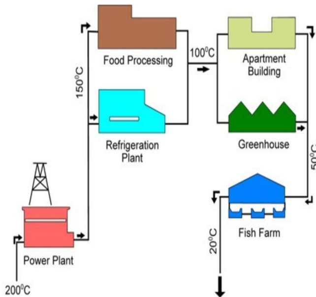
Figura 0.13 Uso en línea o cascada de la energía geotérmica
