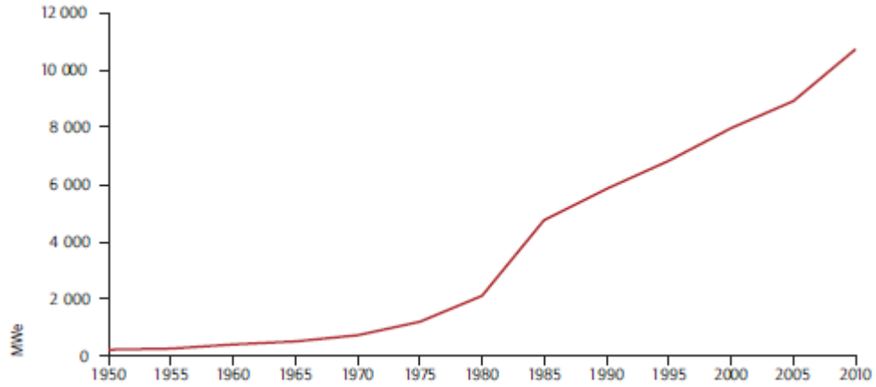
Figura 0.3 Capacidad mundial instalada de energía geotérmica
