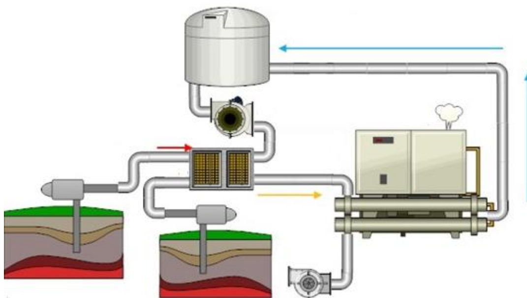
Figura 0.4 Deshidratador geotérmico de alimentos
