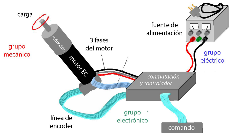
Fig. 3.18 Componentes del sistema de actuación EC
