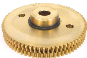
Fig. 3.7 Corona de precisión anti-juego ( http://www.hpcgears.com/ )
