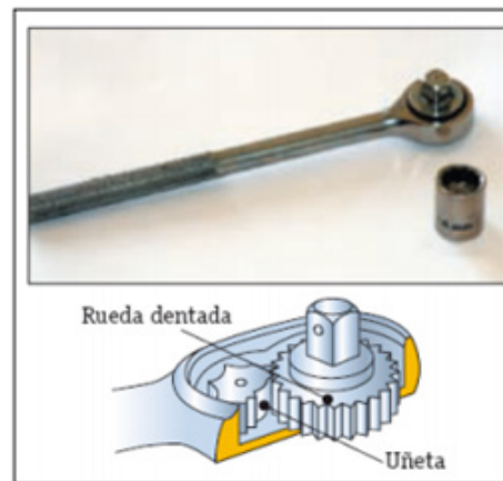
Fig. 3.8 Aplicación comercial del trinquete
