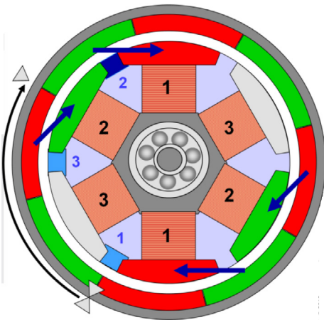
Fig.4.7 Los tres sensores incorporados de efecto Hall (azul) suministran seis combinaciones de señal distintas por secuencia de conmutación. Las tres fases son alimentadas en seis diferentes fases de conducción acordes con esta información del sensor. Las curvas de corriente y voltaje son en forma de bloque. La posición de cambio en cada conmutación electrónica se encuentra simétricamente alrededor del respectivo par máximo.
