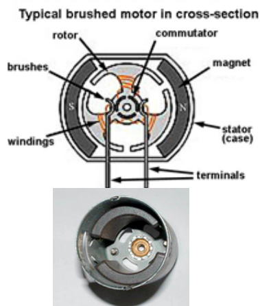
Fig. 3.15 Elementos de un motor con escobillas.
