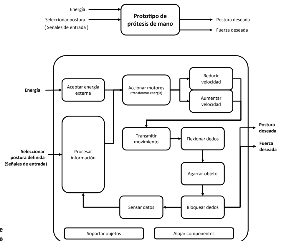
Figura 3.2 Diagrama funcional del prototipo de prótesis de mano
