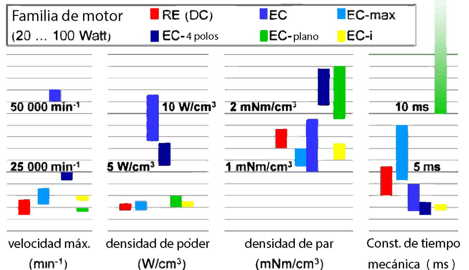
Fig. 3.20 Comparación de motor DC vs EC
