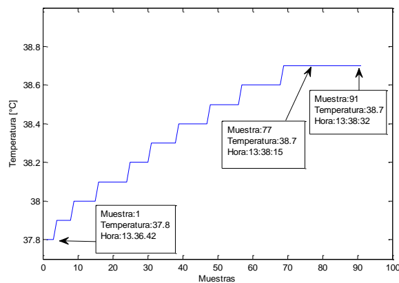
Figura 4.6: Mediciones de Temperatura [44].
