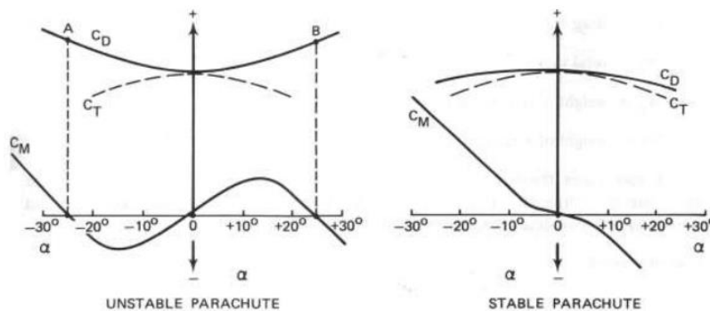
Figura 5.3: Coeficientes C_D , C_T , y C_M contra ángulo de ataque \alpha , para un paracaídas estable e inestable [45].
