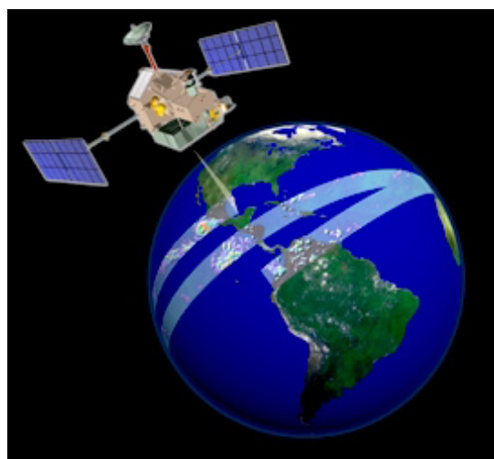
Figura 2.4. Franja de barrido de la órbita inclinada del satélite de la TRMM (NASA, 1997).
