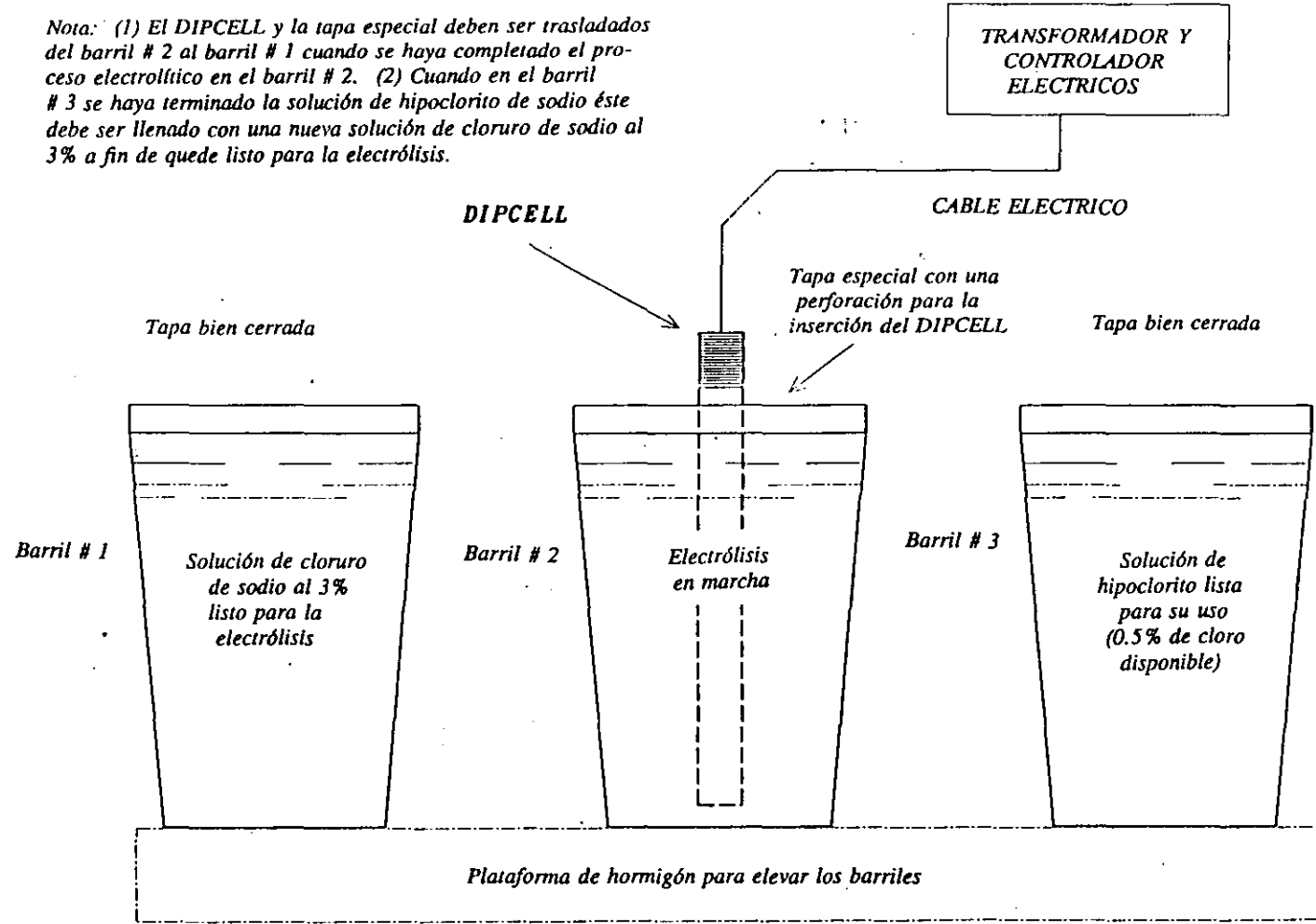
FIGURA 1 Diagrama de una instalación típica del DIPCELL que utiliza tres barriles a fin de facilitar la producción continua de hipoclorito de sodio
