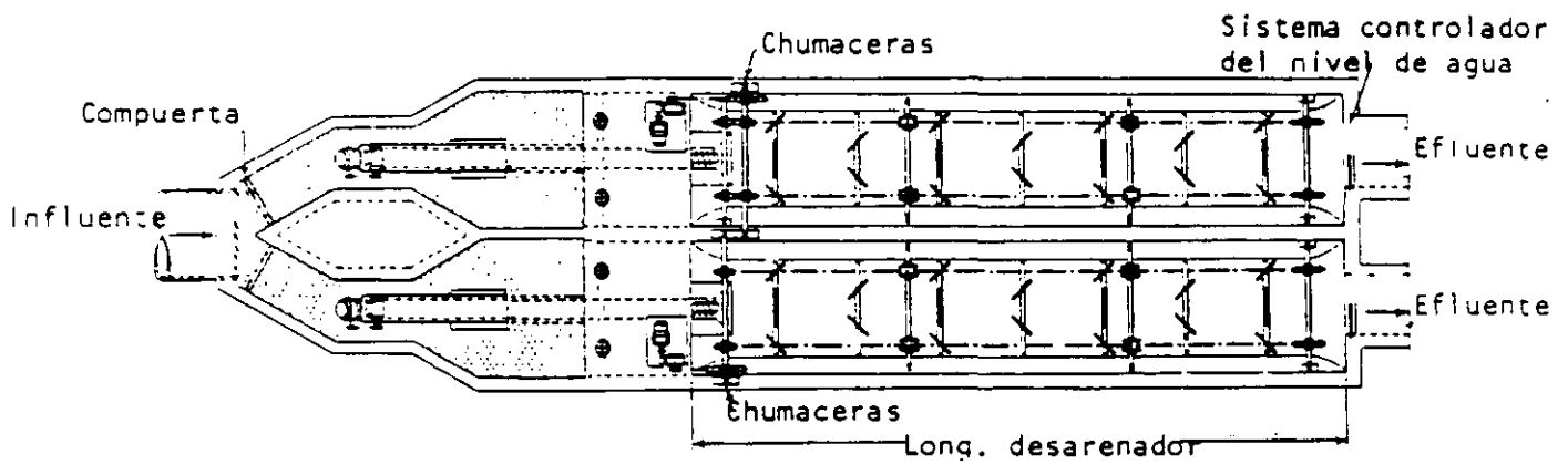
(a) Planta
