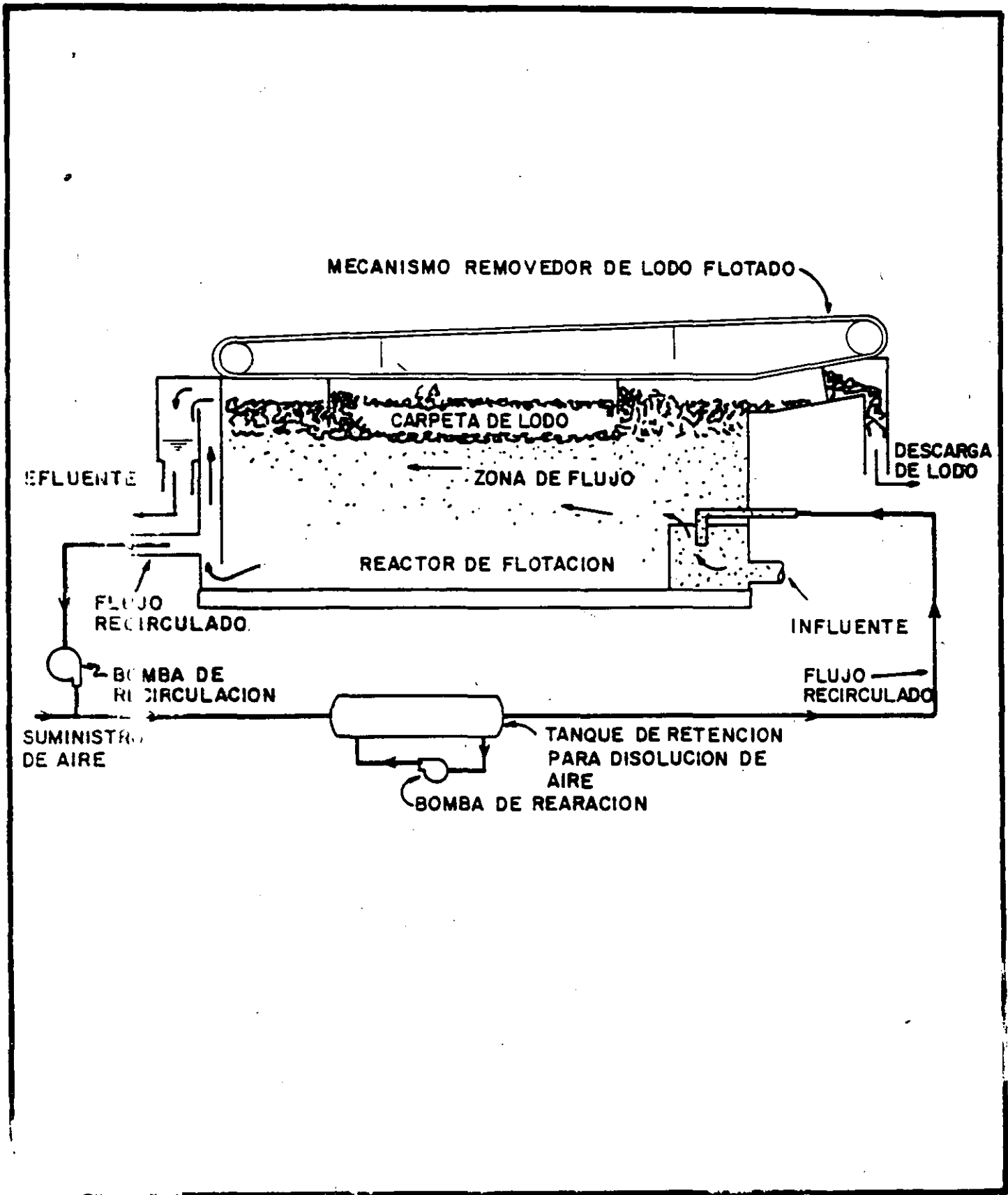
1.5 SISTEMA DE FLCTACION CON AIRE DISUELTO
