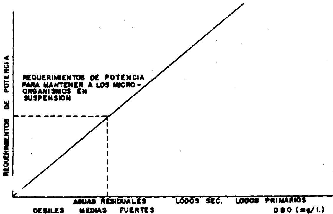
FIG:10 RELACION ENTRE POTENCIA REQUERIDA Y CONCENTRACION DE MATERIA ORGANICA DEGRADABLE EN EL DESECHO.
