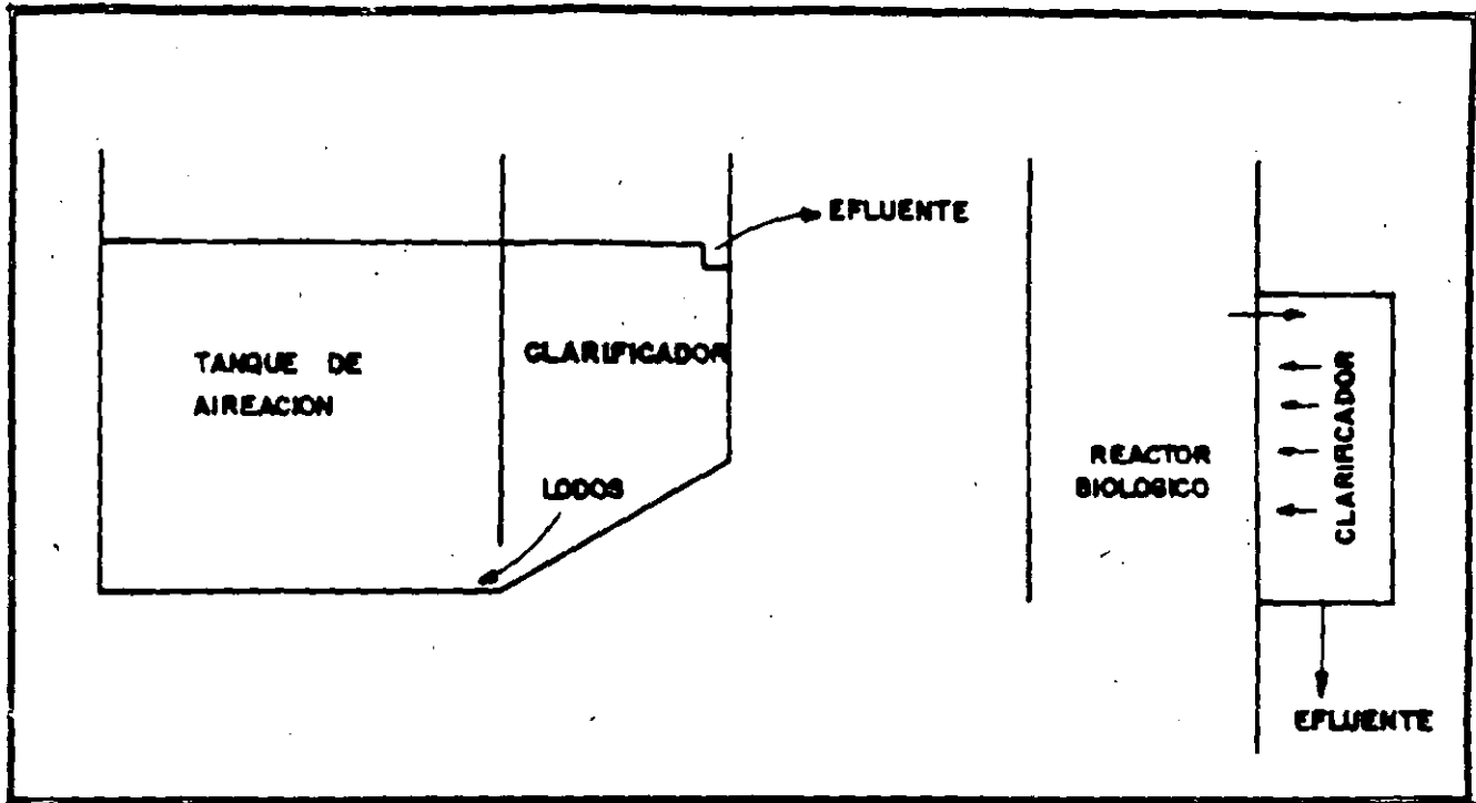
FIG. II REPRESENTACION ESQUEMATICA DE SISTEMA DE ZANJAS DE OXIDACION CON CLARIFICADOR, RETORNADO LOS LODOS DIRECTAMENTE AL REACTOR BIOLÓGICO.
