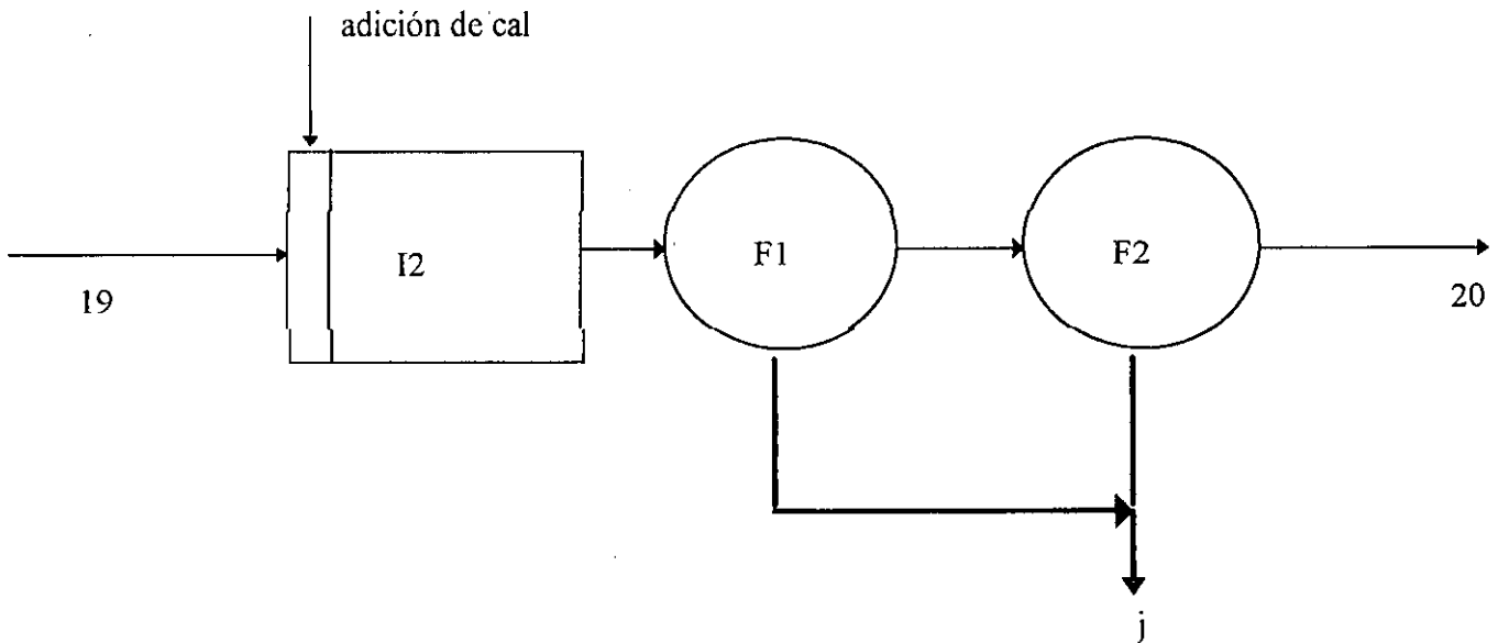
ADICIÓN DE CAL( DOS ETAPAS) DESPUÉS DE TRATAMIENTO PRIMARIO O SECUNDARIO
