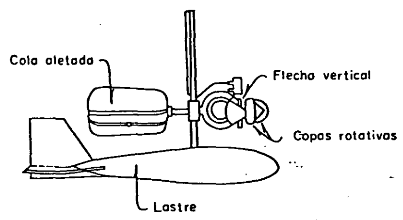
MEDIDOR DE CORRIENTE TIPO PRICE
