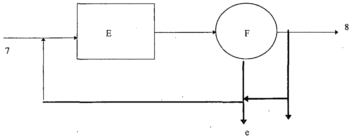
REACTOR DE CRECIMIENTO CON PELÍCULA FIJA (TRATAMIENTO SECUNDARIO)
