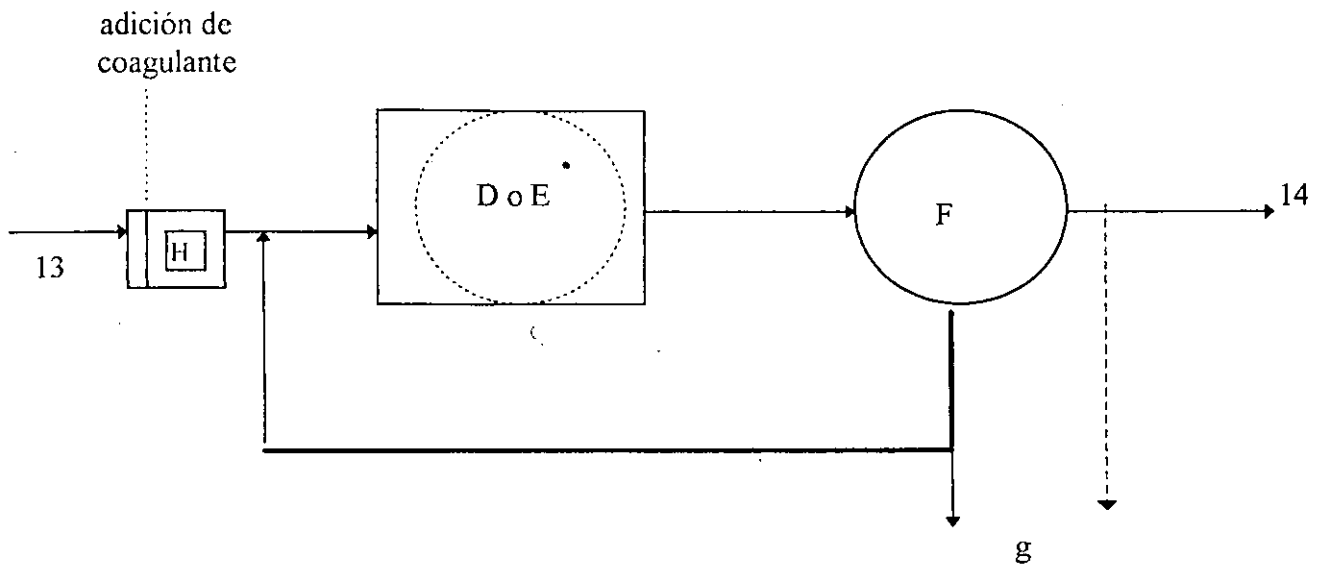
COAGULACIÓN CON TRATAMIENTO BIOLÓGICO
