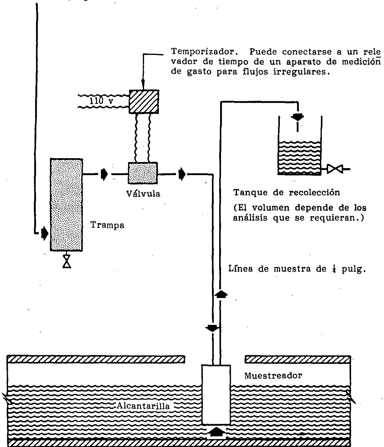
Muestreador automático de puente de aire (airlift). Puede utilizarse para subir muestras de alcantarillas
