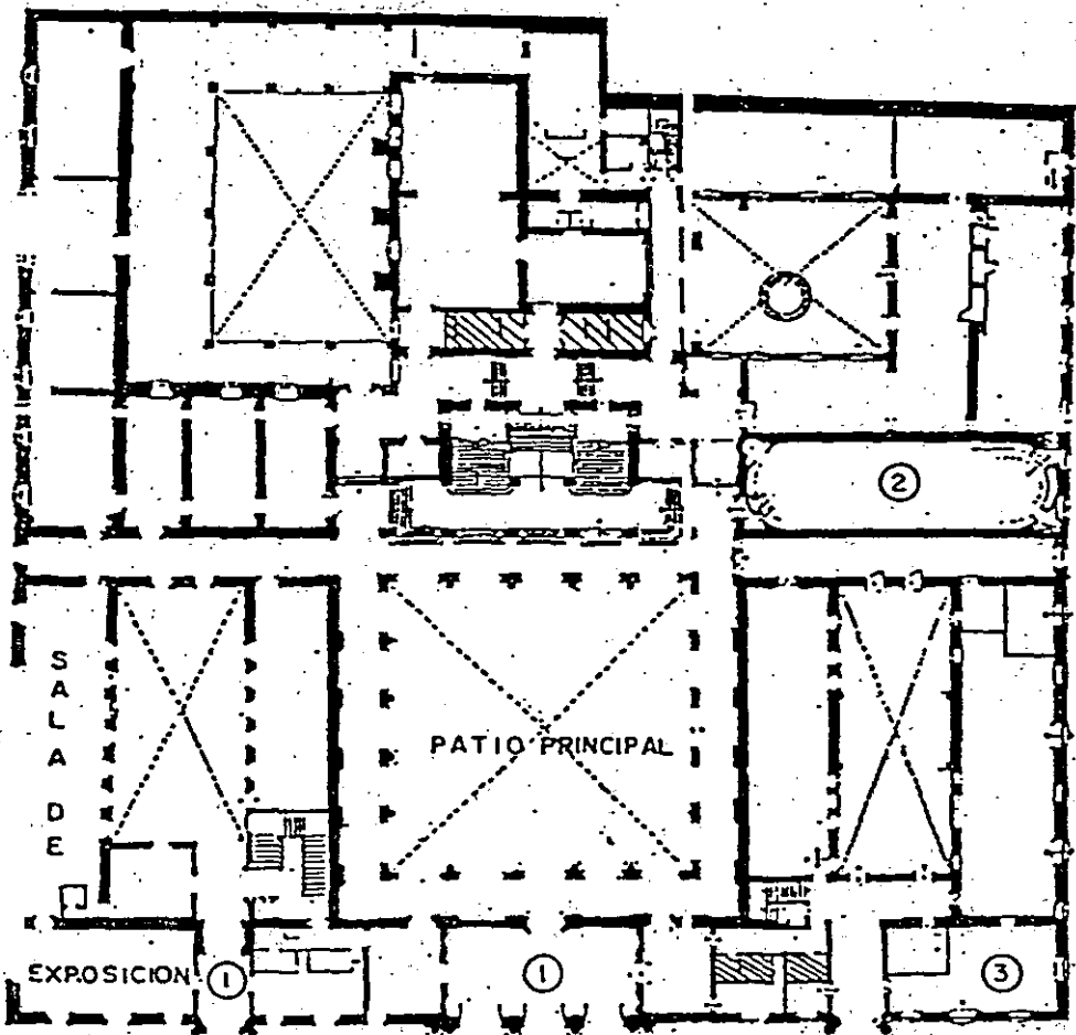
PLANTA BAJA
