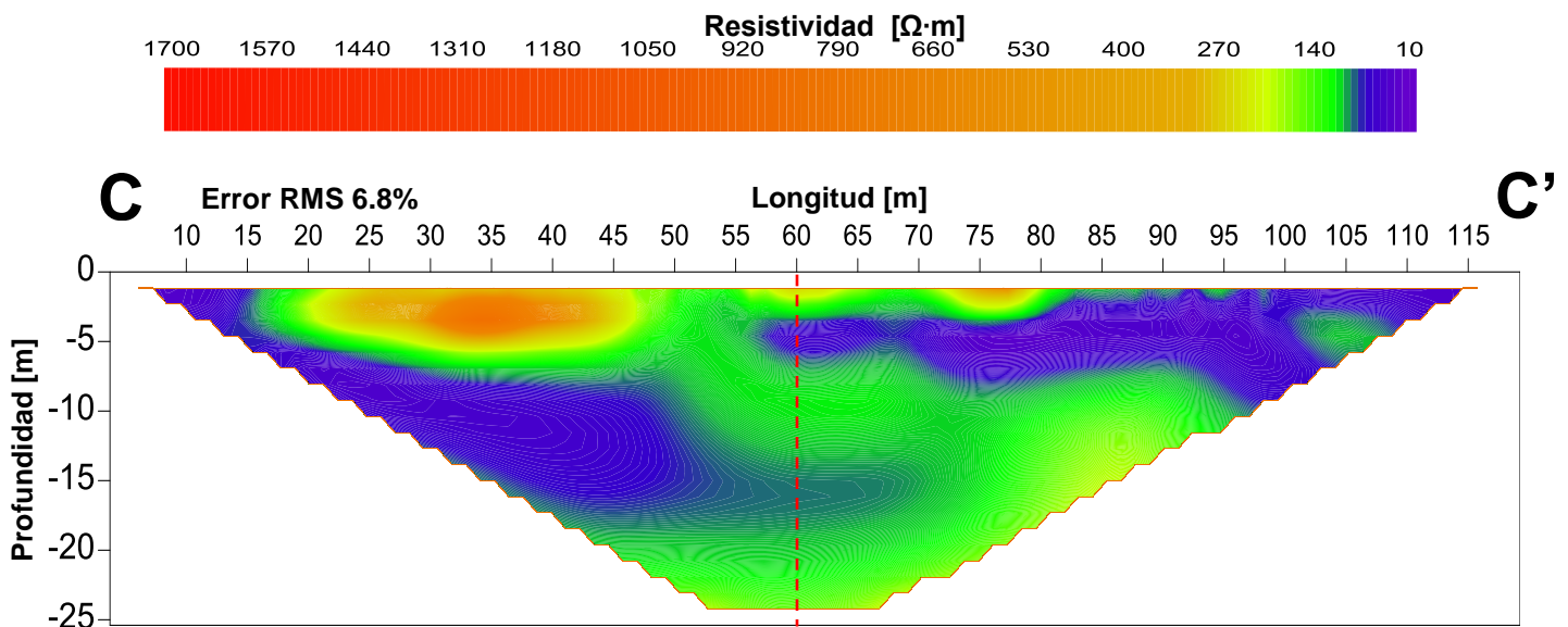
Figura 5.1.3.-Modelo de resistividades de la línea 3.
