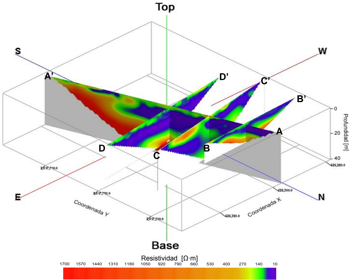
Figura 5.2.2.-Visualización del Modelo Pseudo 3D con vista en dirección NE.
