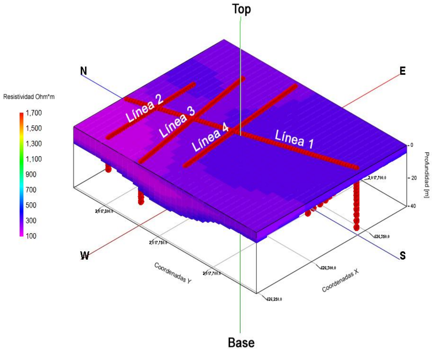
Figura 5.3.2.-Cubo de resistividades con el volumen estimado del acuífero (UG1/UH1).
