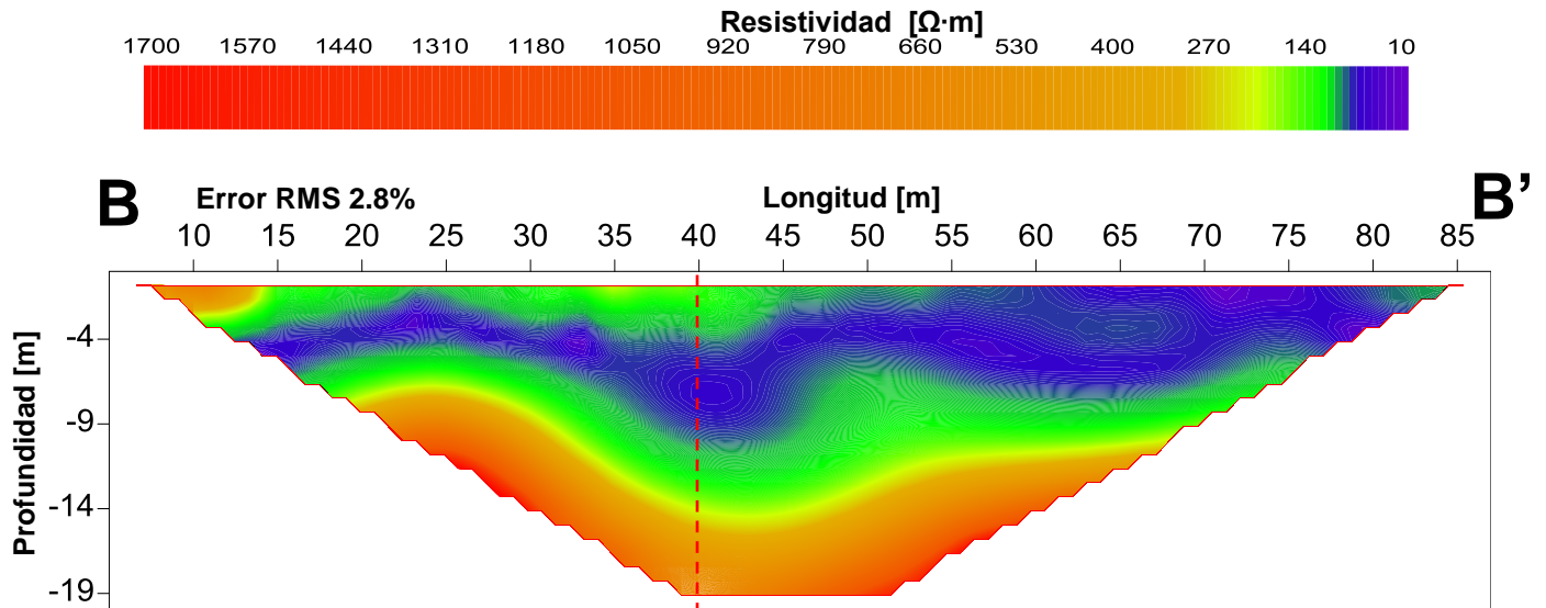
Figura 5.1.2.-Modelo de resistividades de la línea 2.
