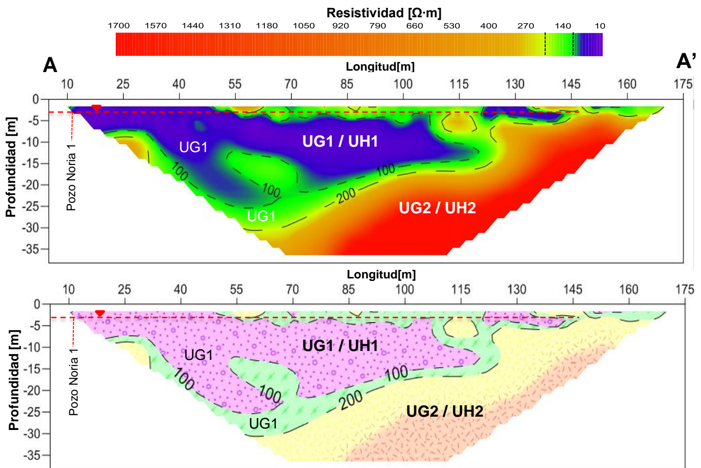
Figura 5.3.1.-Integración de resultados en la línea 1, capas geoeléctricas e hidrogeológicas.
