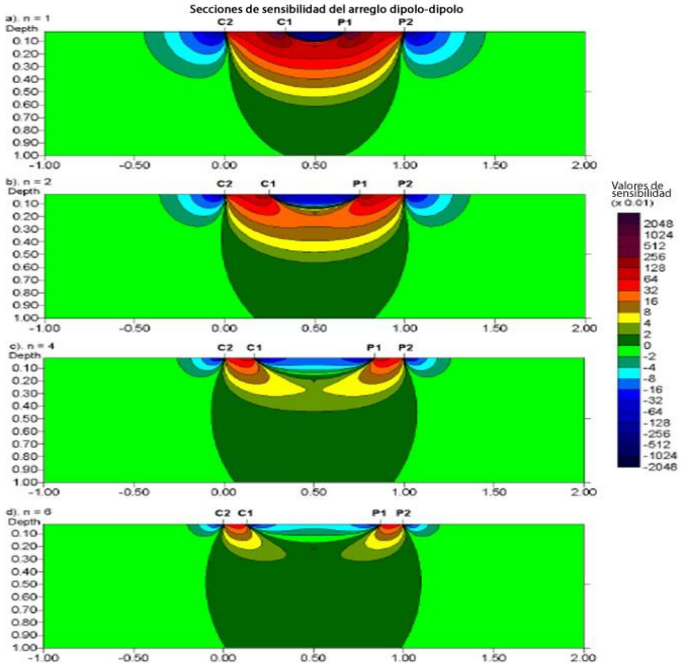
Figura 2.2.7. Secciones de sensibilidad para el arreglo dipolo-dipolo. Secciones con valores de (a) n=1 , (b) n=2 , (c) n=4 , y (d) n=6 (Loke, 2004).
