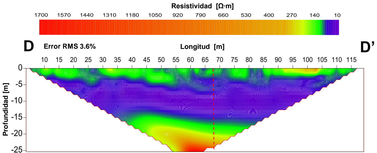
Figura 5.1.4.-Modelo de resistividades de la línea 4
