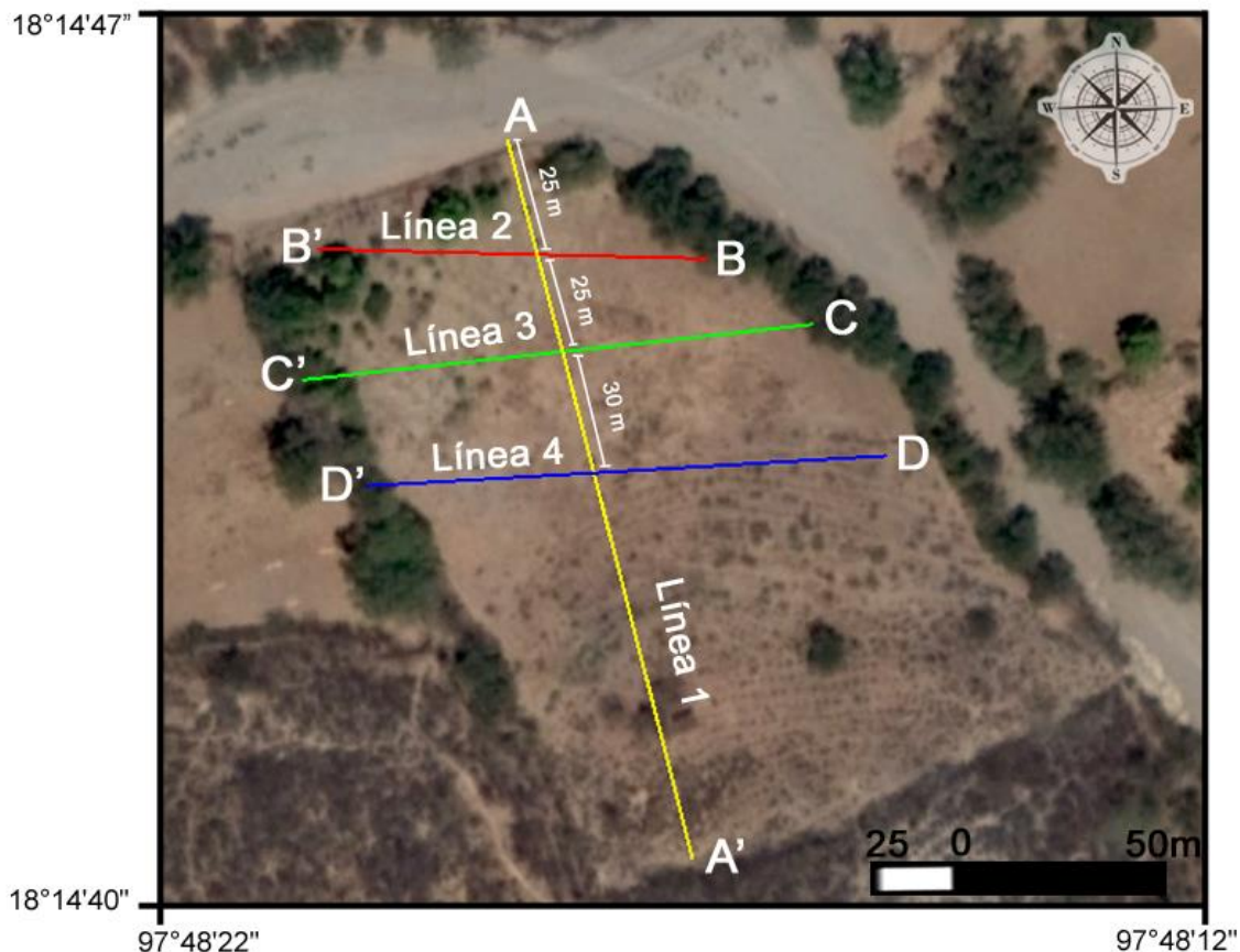
Figura 4.1.1.- Localización de las líneas en el terreno de estudio para los perfiles de TRE (Google Earth, 2015).
