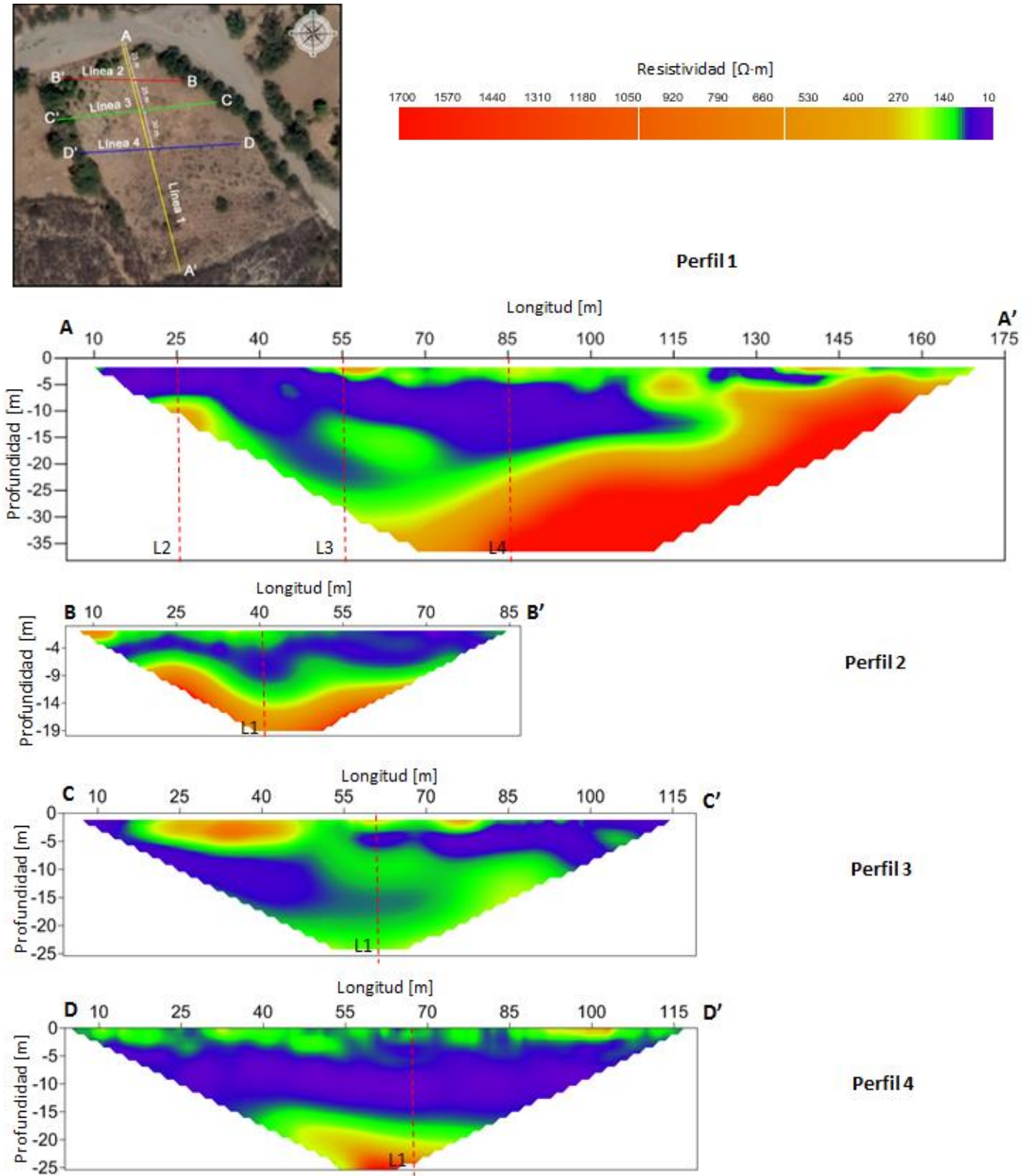
Figura 5.1.5.-Modelos de resistividades con escala y localización
