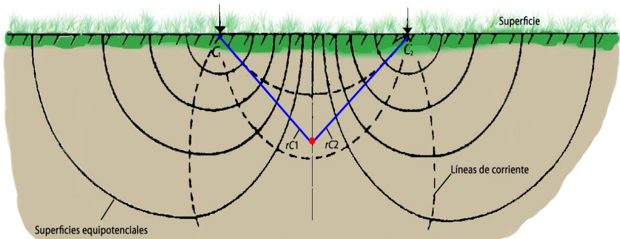
Figura 2.2.3.- Potencial medido en el subsuelo con un par de electrodos (Telford et al., 1990).
