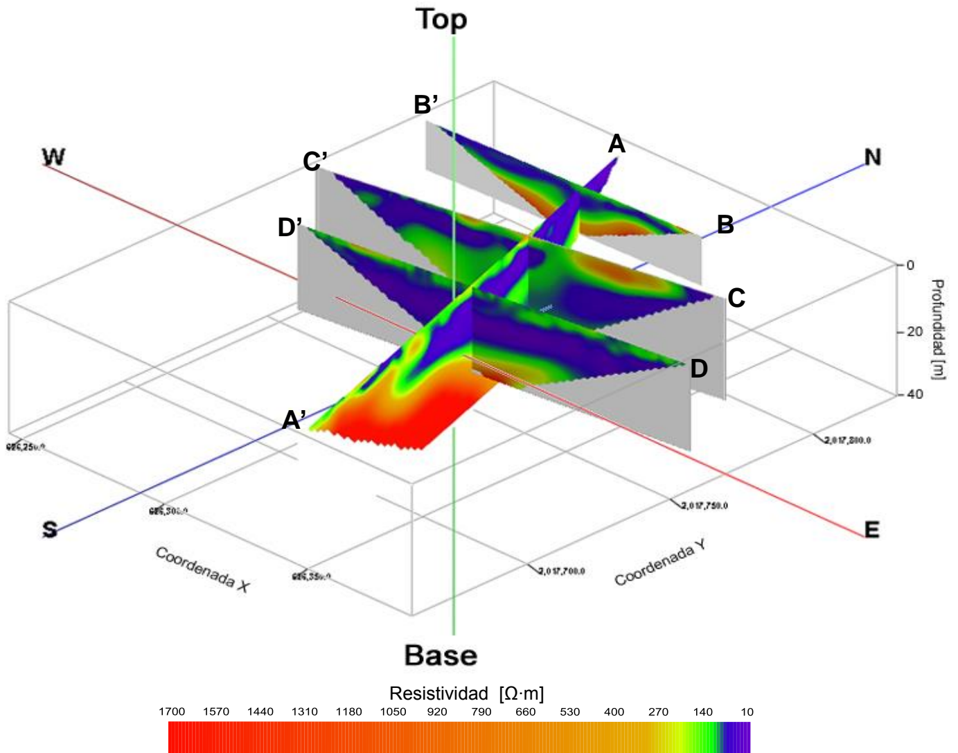
Figura 5.2.1.-Visualización del Modelo Pseudo 3D con vista en dirección SE.
