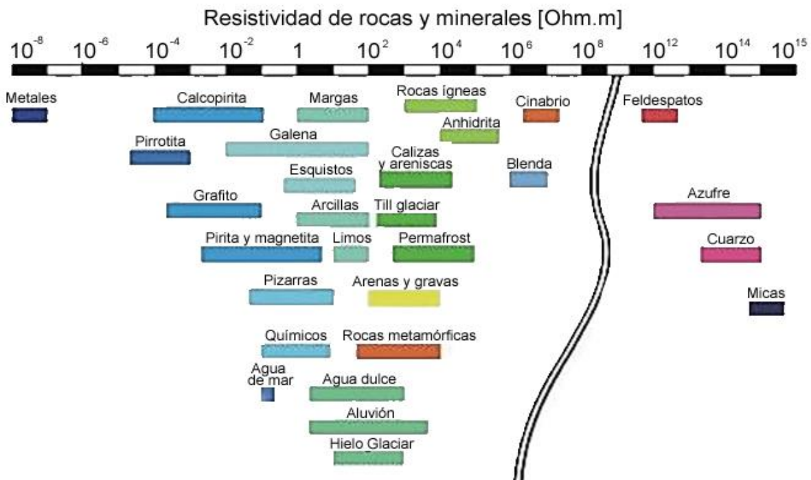
Figura 2.1.3.- Resistividades de algunos minerales y rocas (Orellana, 1982)
