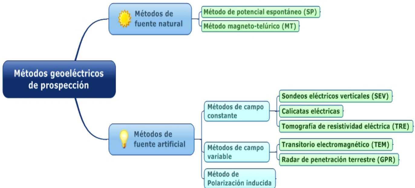
Figura 2.1.1.- Esquema de clasificación de métodos de prospección eléctrica (Orellana, 1982).
