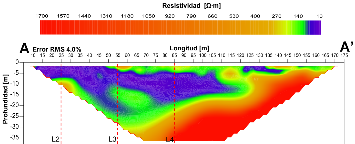
Figura 5.1.1-Modelo de resistividades de la línea 1.
