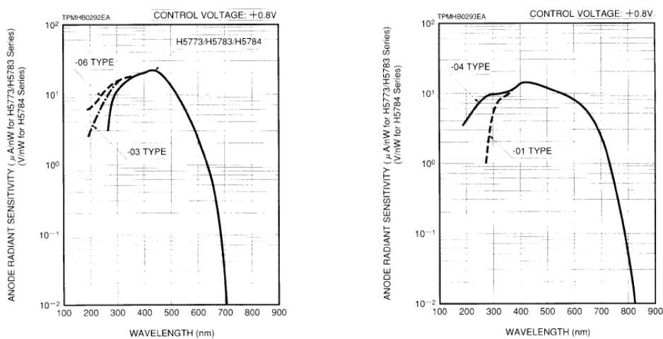
Fig 50 Gráficas de longitud de onda vs sensibilidad del fotomultiplicador
