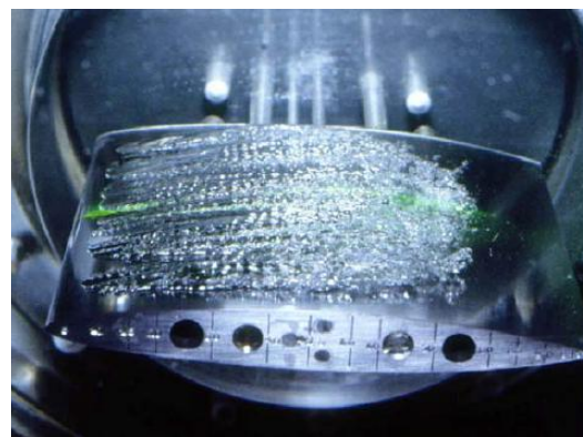
Fig. 8. Cavitación superficial [17].
