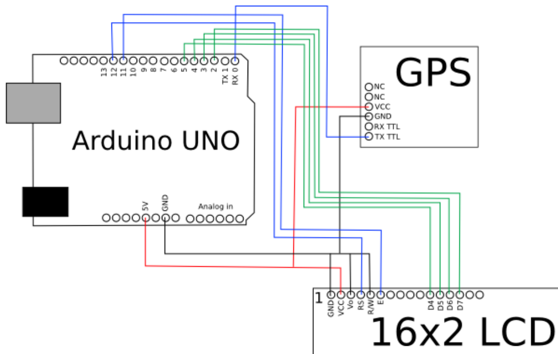
Figura 1. 12 Esquema de integración de GPS con Arduino
