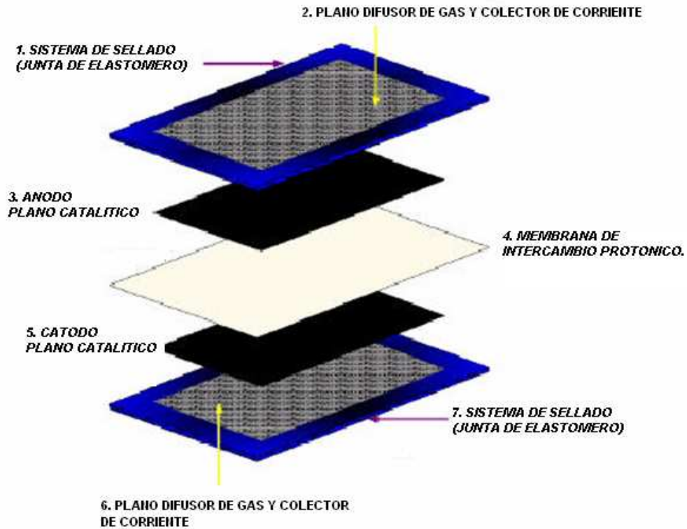
Figura I.1.1. Ensamble Membrana-Electrodo
