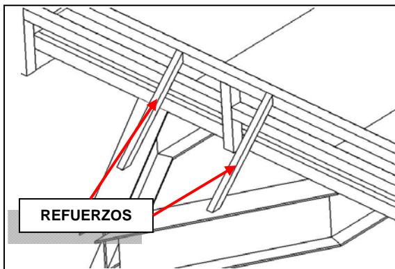
Fig. 2.16 Propuesta para reforzo de portería delantera.
