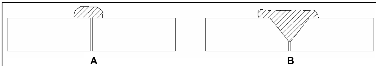
Fig. 4.19 A) Soldadura sin filete. B) Soldadura con filete.
