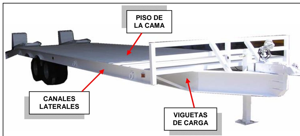
Fig. 3.5 Posición de piso, canales y viguetas en el remolque.
