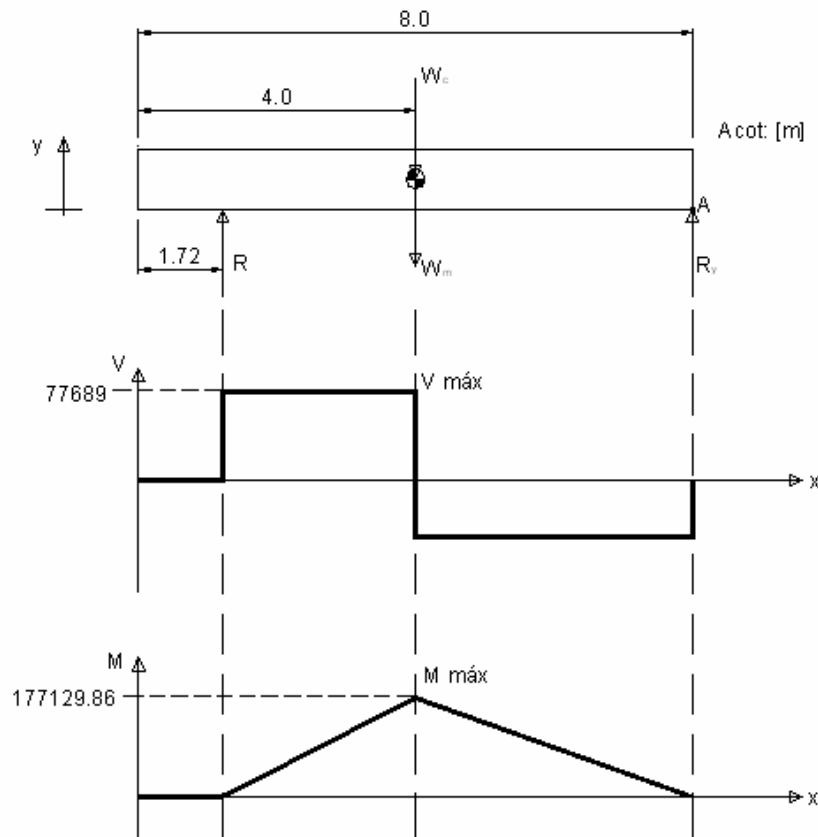
Fig. 3.38 Diagrama V-M de la viga de carga
