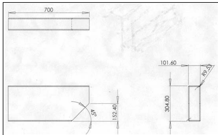
Fig. 2.12 Primer diseño >>> para el pie de rampa.
