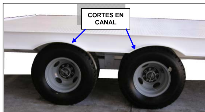
Fig. 3.4 Detalle de cortes para salpicaderas en canal lateral.
