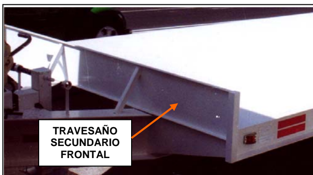
Fig. 2.7 Parte frontal del remolque de línea con travesaño secundario frontal.
