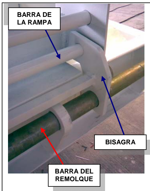
<<< Fig. 3.13 Detalle de bisagra en el remolque
