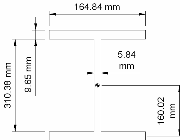
Fig. 3.39 Sección transversal de la vigueta IPR
