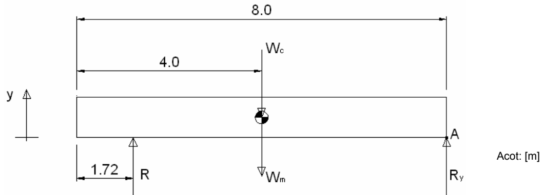
Fig. 3.37 Diagrama de Cuerpo Libre de la viga de carga.
