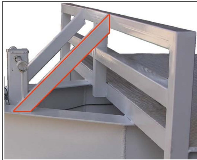
Fig. 3.19 Detalle del refuerzo de portería en el remolque.
