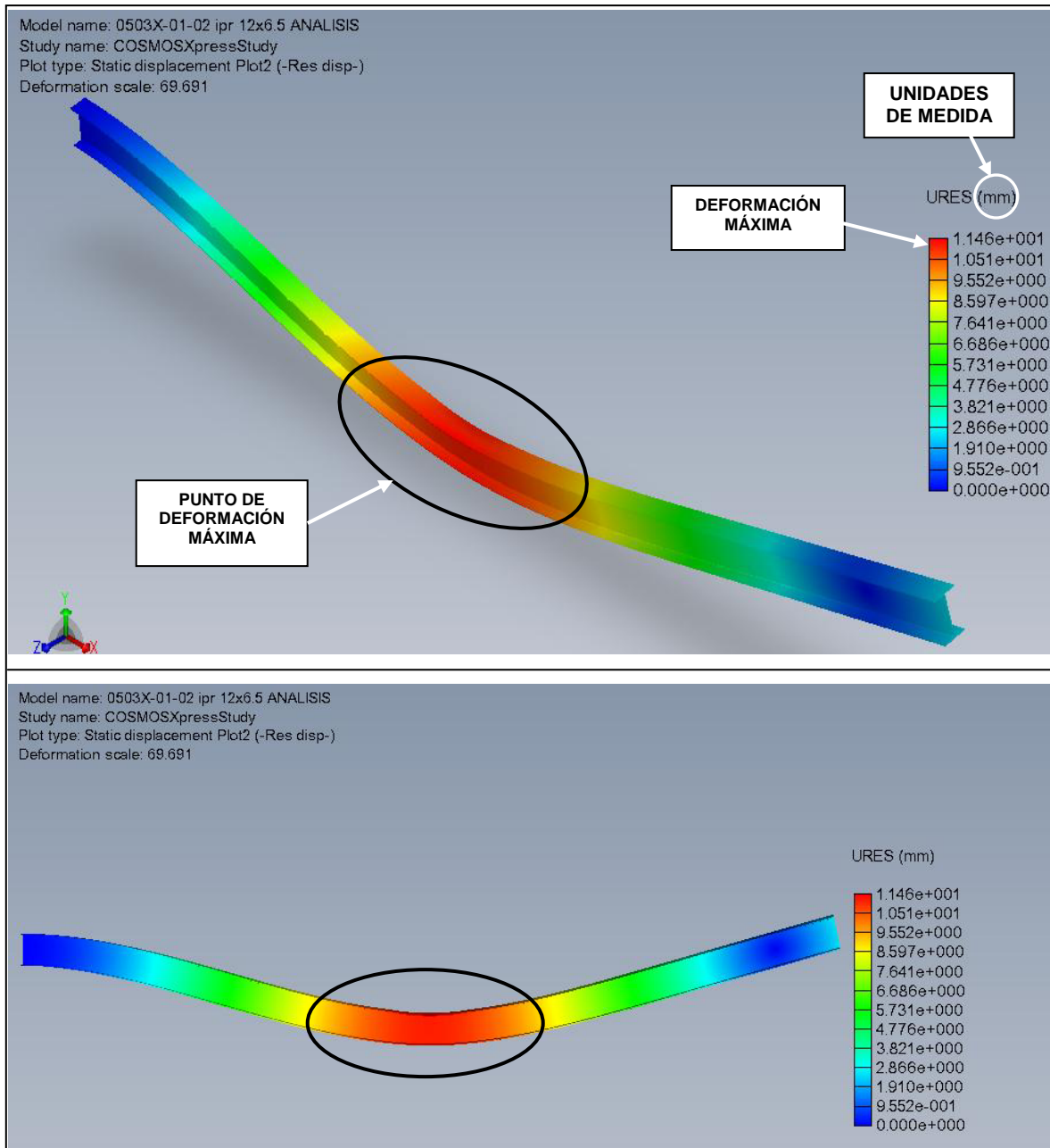
Fig. 3.42 Distribución de deformación en la viga de carga.
