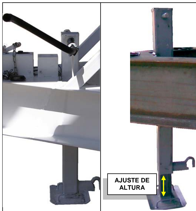
Fig. 3.36 Detalle de gato cuello de ganso.
