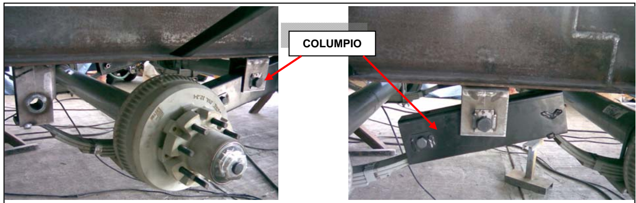
Fig. 3.32 Kit tándem instalado con columpios.
