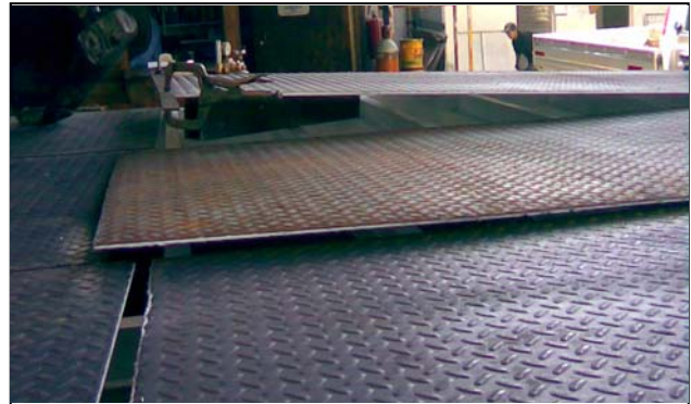
Fig. 4.2 Montaje de placas en posición >>>
