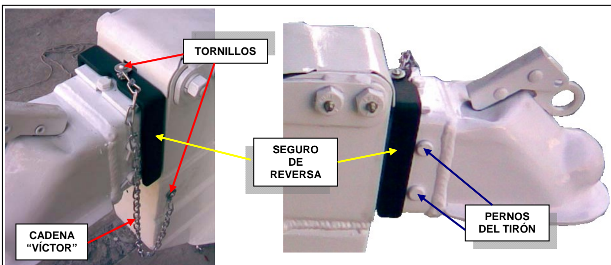
Fig. 3.18 Detalle del seguro de reversa en el remolque.
