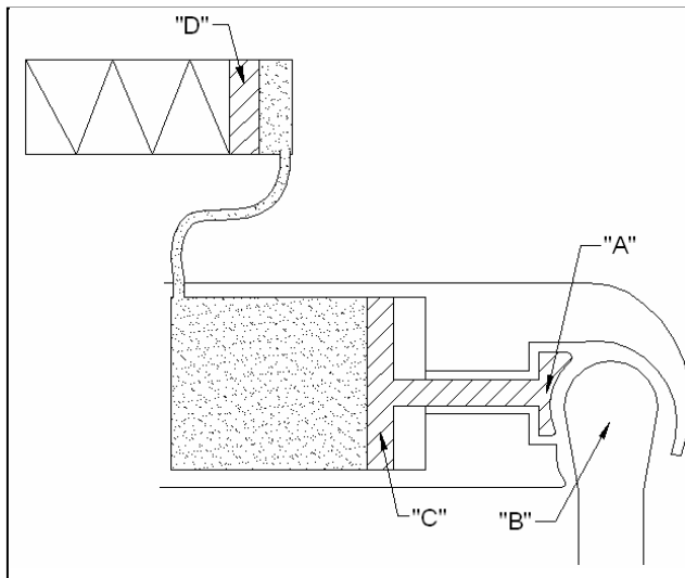
Fig. 2.13 Diagrama de funcionamiento del tirón hidráulico.
