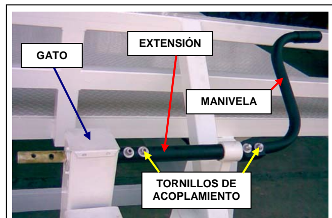
Fig. 3.24 Detalle de extensión >>> para manivela en el remolque
