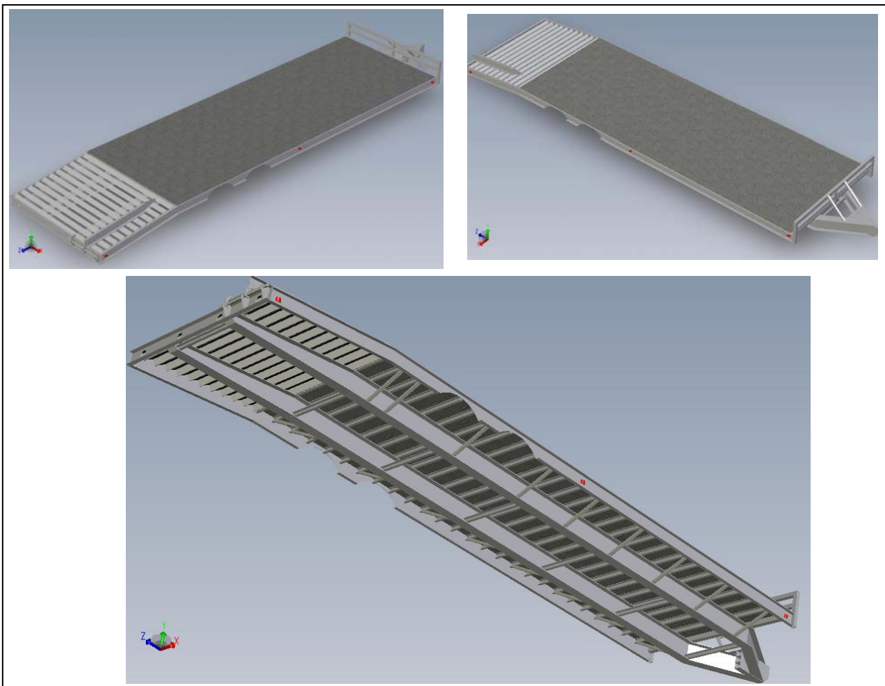
Fig. 3.43 Modelo de computadora del remolque
