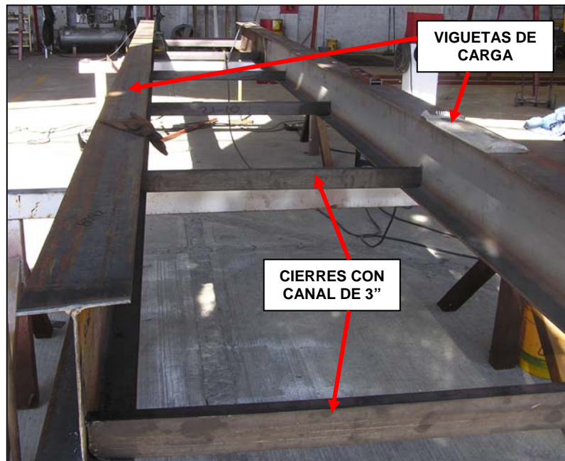
Fig. 4.22 Detalle de cierres con canal de 3" >>>
