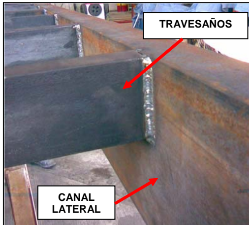
<<< Fig. 4.28 Detalle de armado de canales laterales.
