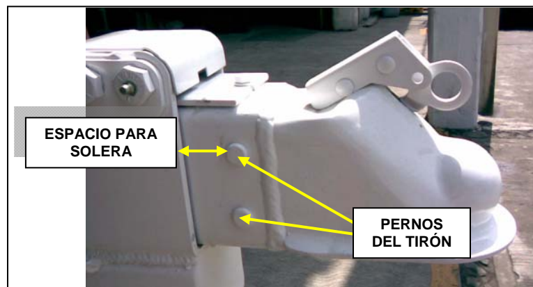
Fig. 2.14 Detalle del tirón hidráulico.
