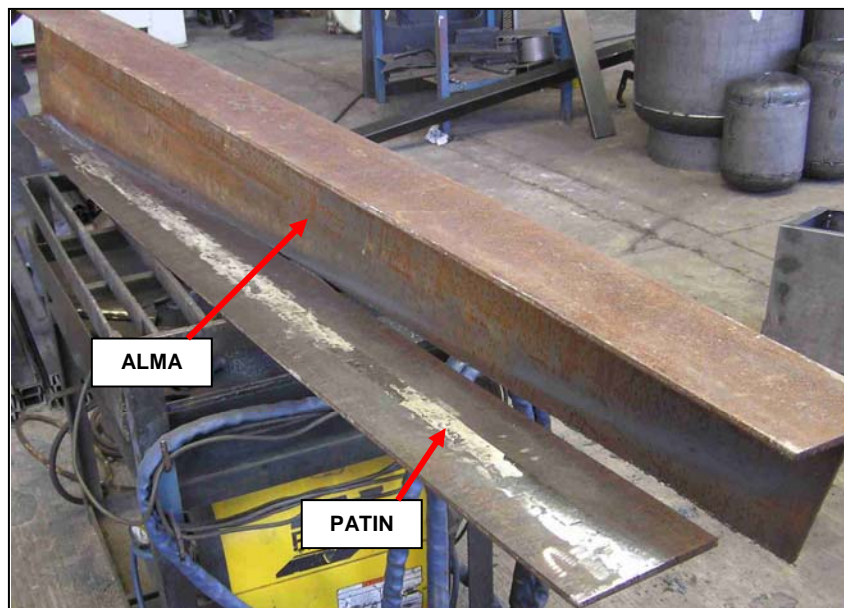
Fig. 4.23 Corte para separar alma y patín de la vigueta.
