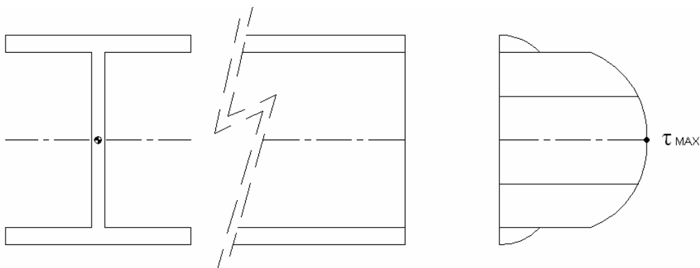
Fig. 3.40 Distribución del esfuerzo cortante en la vigueta IPR
