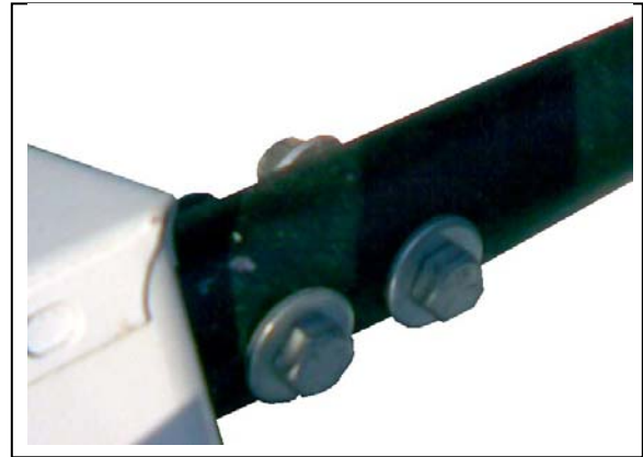
Fig. 3.22 Detalle de acoplamiento >>> entre gato y extensión
