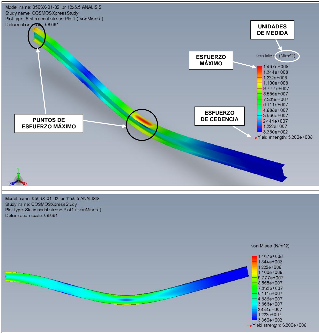
Fig. 3.41 Distribución de esfuerzos en la viga de carga.
