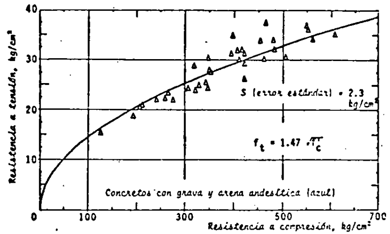
Fig 2 Resistencia a tensión por compresión diametral
