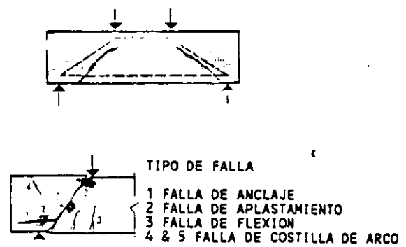
Fig. 3.4 a/d = 0 TO 1 Modelos de Falla de Vigas de Gran Peralte
