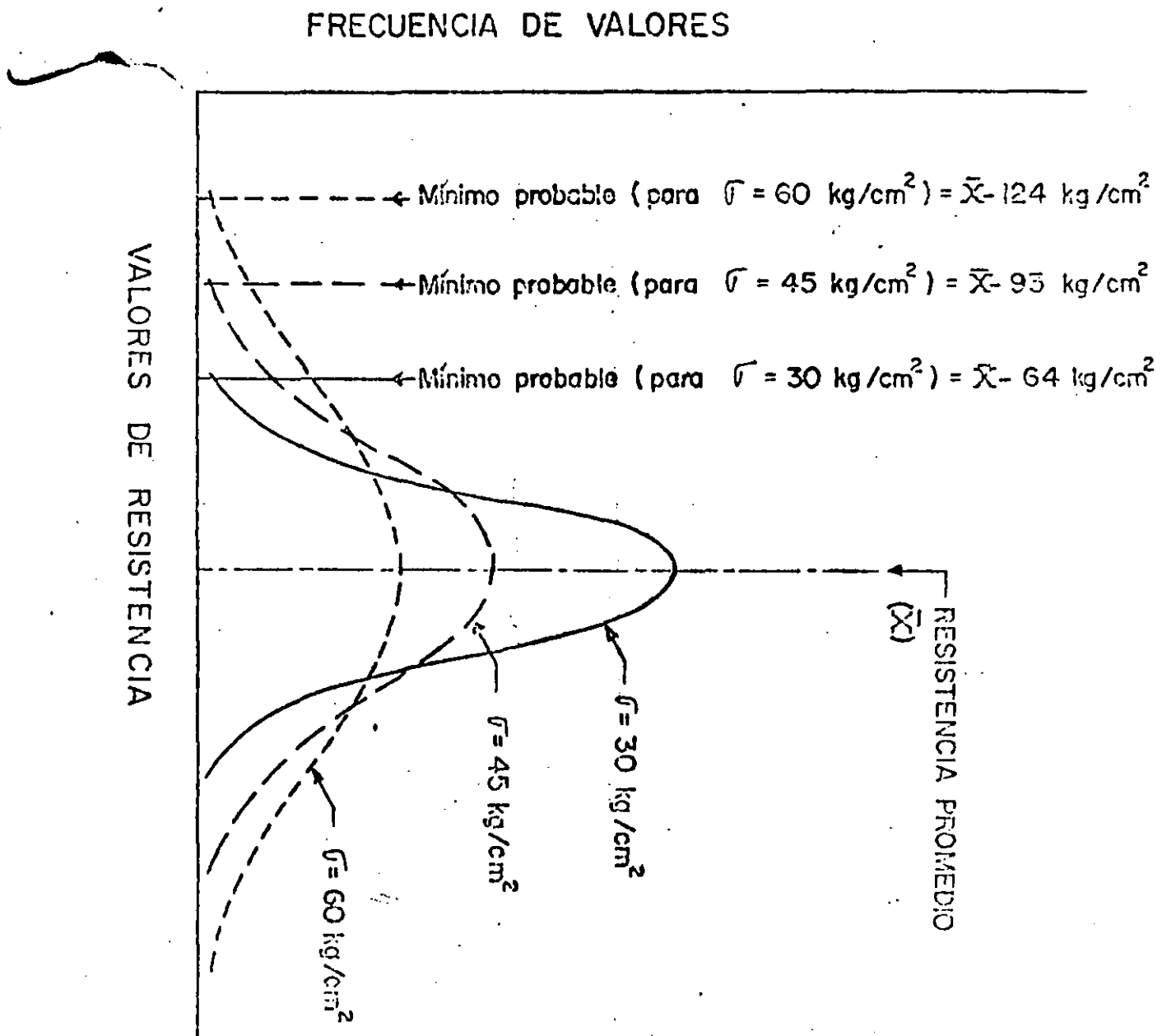
FIG.1.8 - VARIACION DEL VALOR MINIMO PROBABLE DE ACUERDO CON LA DISPERSION OBTENIDA EN LAS RESISTENCIAS
