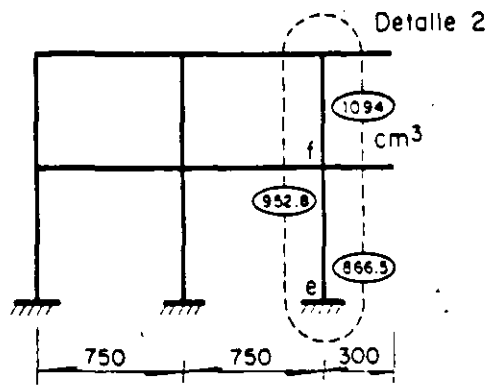
Elevación eje 2
