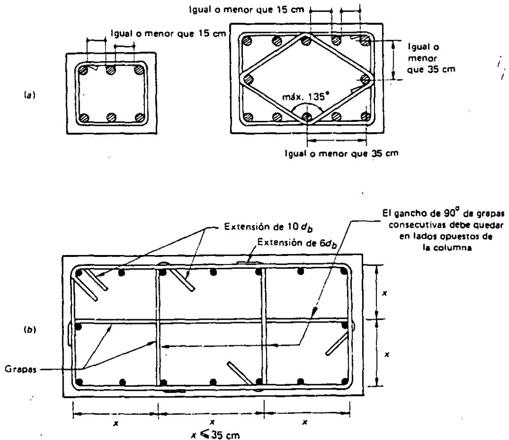
Figura 15.3 Detalles del refuerzo transversal de columnas.
