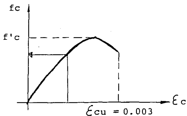
CURVA TIPICA DEL CONCRETO EN COMPRESION.
