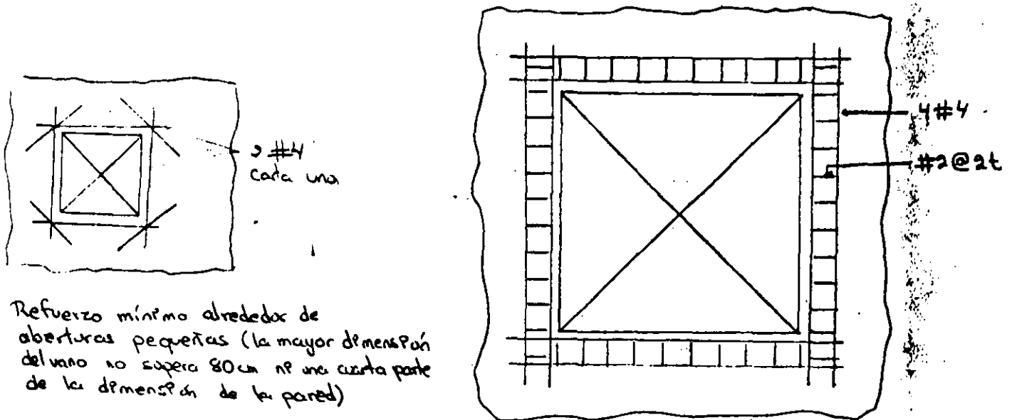
Fig. 10.20 Detalles recomendados de refuerzo alrededor de aberturas en muros de concreto.
