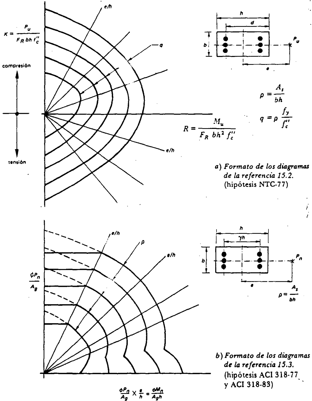
Figura 15.5 Formatos típicos de diagramas de interacción.
