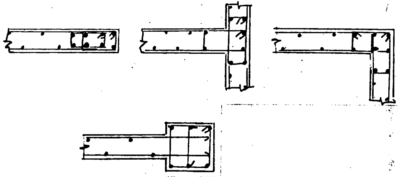
Fig. 10.14 Refuerzo en los extremos de muros
