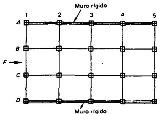
Figura 13.8 Estructura con muros rígidos.
