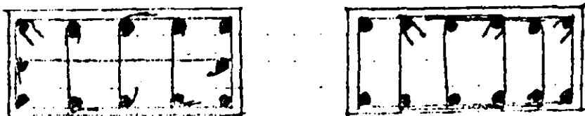
Fig. 9.10 - Arreglos admisibles de refuerzo en columnas de muros de vigas de concreto
