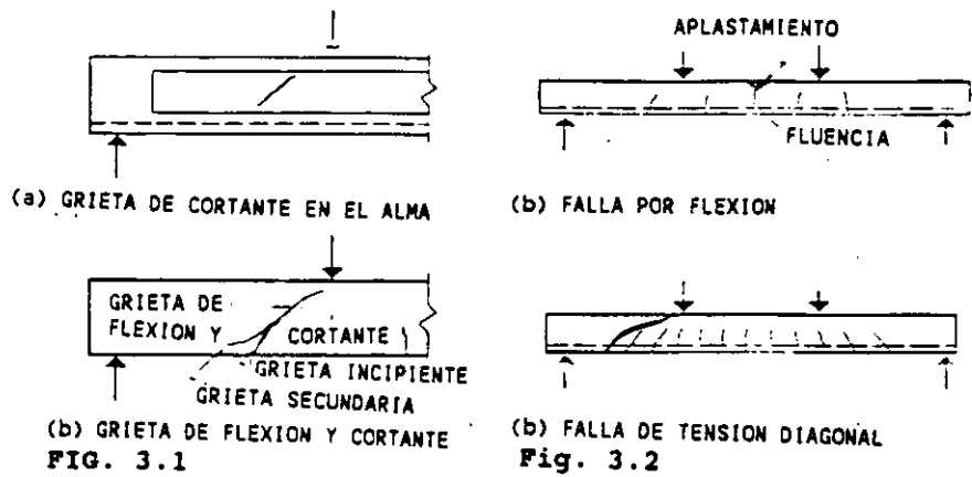
FIG. 3.1 Tipos de Grietas Inclinadas Fig. 3.2 Fallas de Vigas Esbeltas
