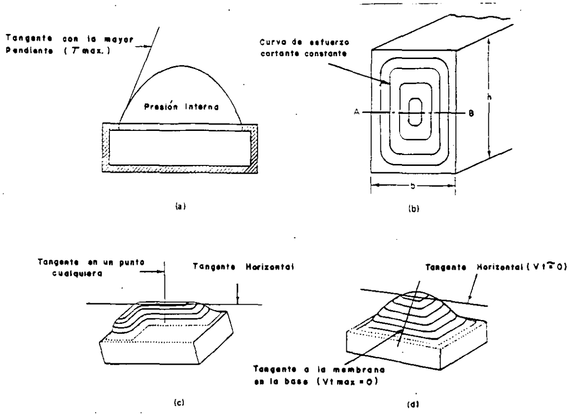
Fig. 7.3 Analogía con la membrana en la torsión pura elástica. (a) Membrana bajo presión; (b) Curvas en una viga real o en una membrana; (c) Sección L; (d) Sección rectangular.
