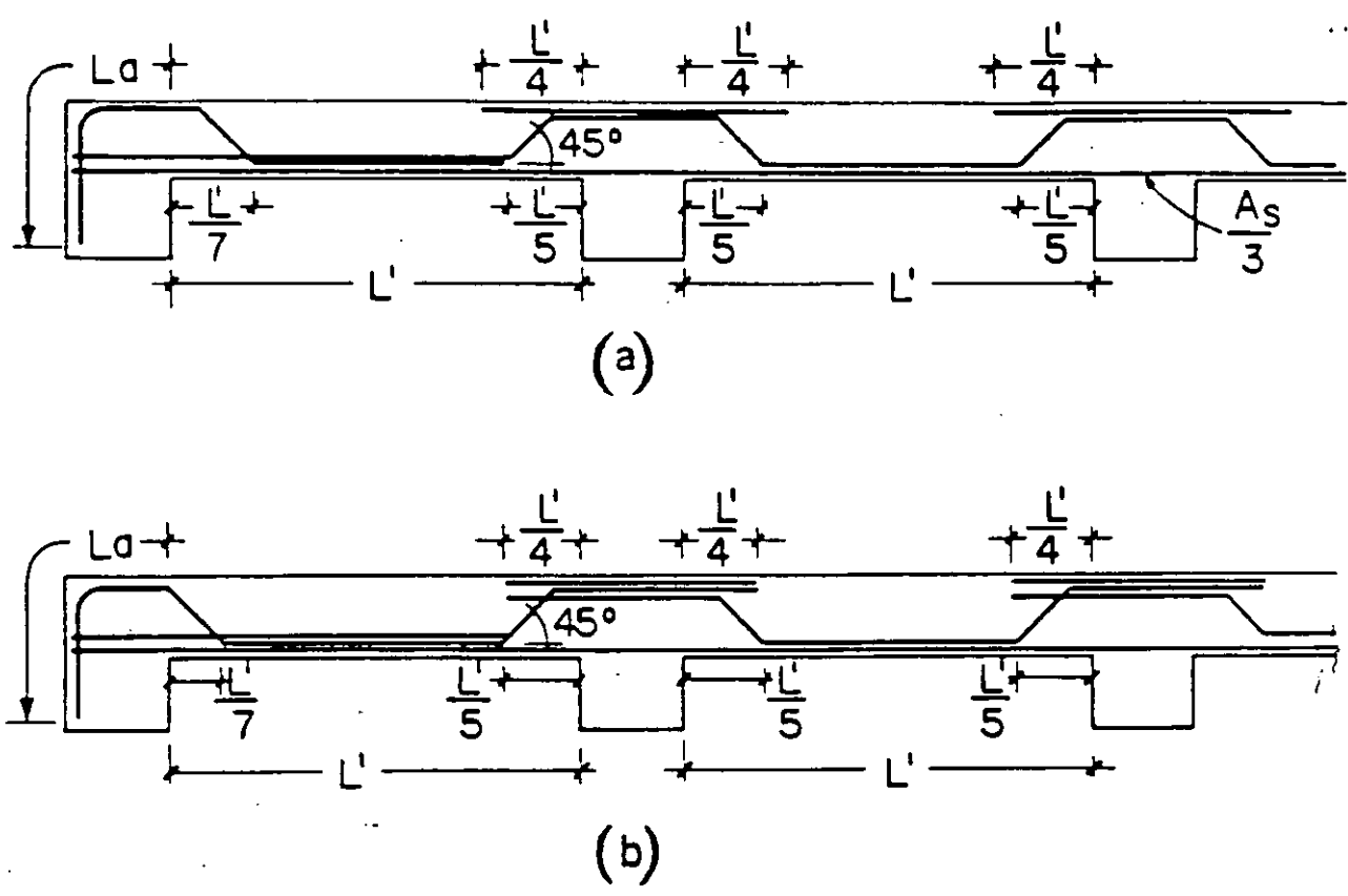
FIG. 11 Recomendaciones para la colocación de refuerzo en losas.
