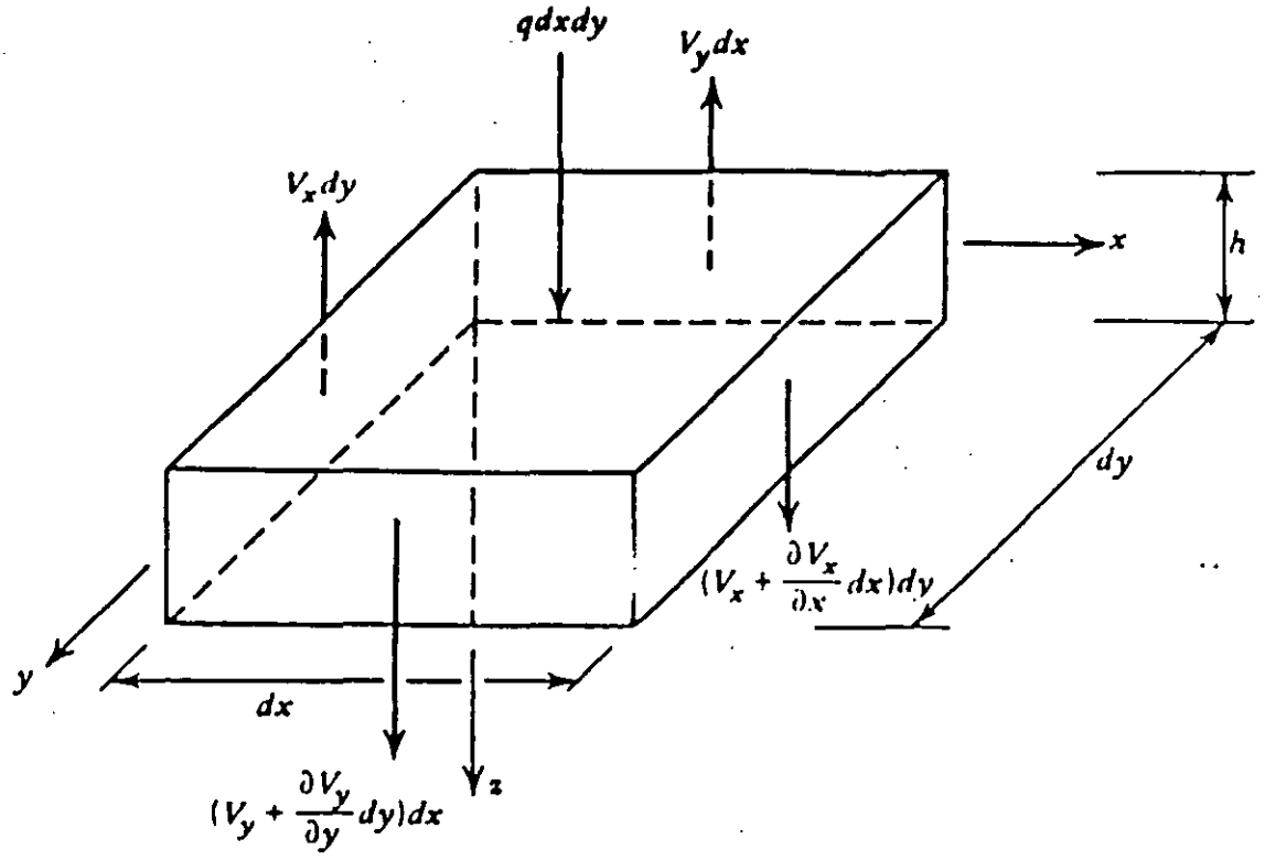
FIG. 6 FUERZAS DE SUPERFICIE Y CORTANTE
