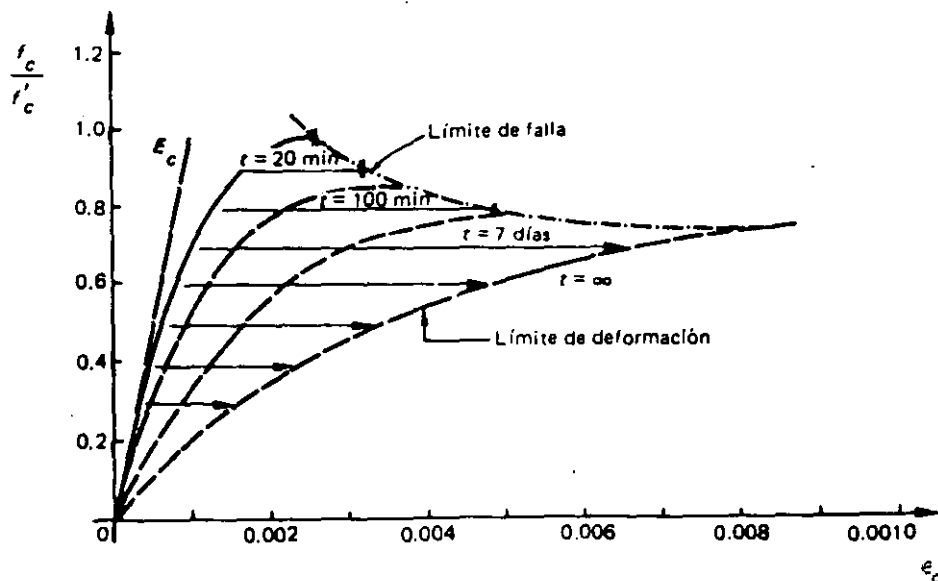
Figura 2.14 Efecto de la permanencia de la carga (Rüschi) [2.5].
