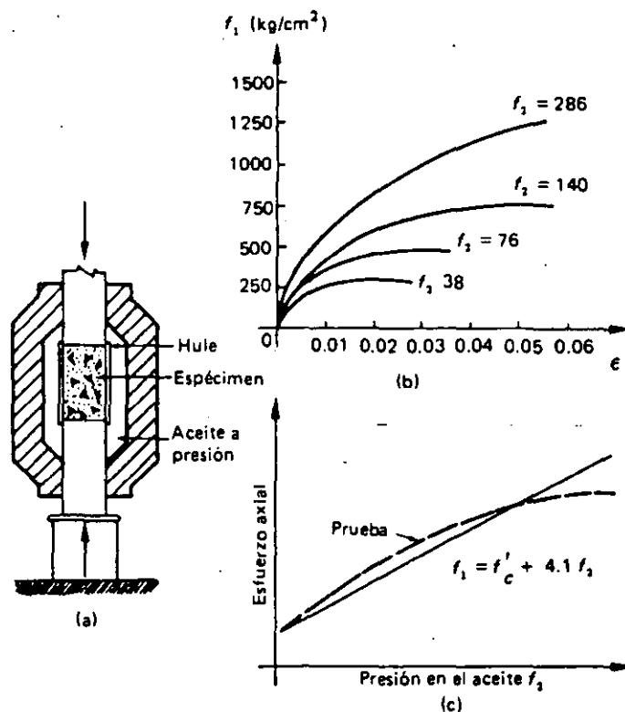
Figura 2.10 Compresión triaxial (Brandtzaeg [2.3]).
