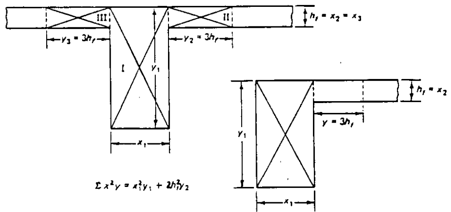
Fig. 7.6 Rectángulos compuestos para el cálculo de T_a .
