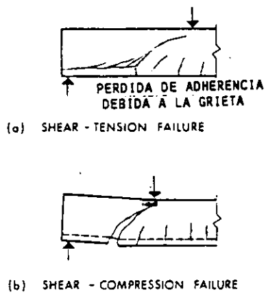
Fig. 3.3 a/d = 1 TO 2.5 Fallas Típicas de Cortantes en las Vigas Cortas
