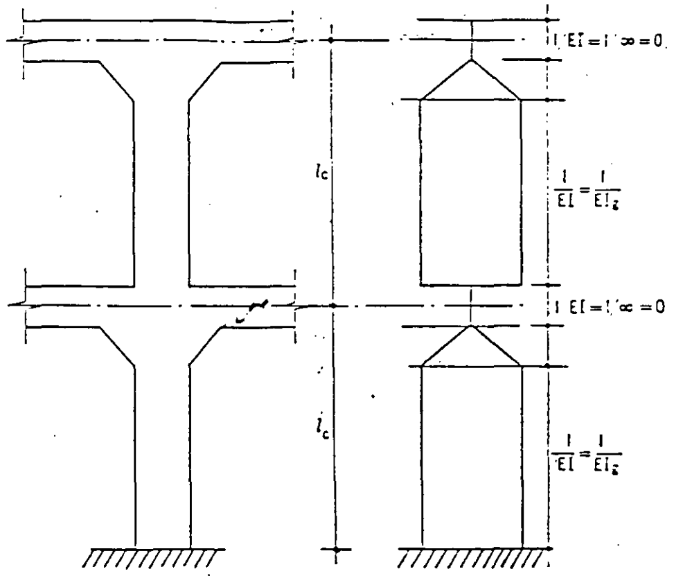
Figura 21 Cálculo de la rigidez a flexión de las columnas equivalentes en sistemas sin vigas
