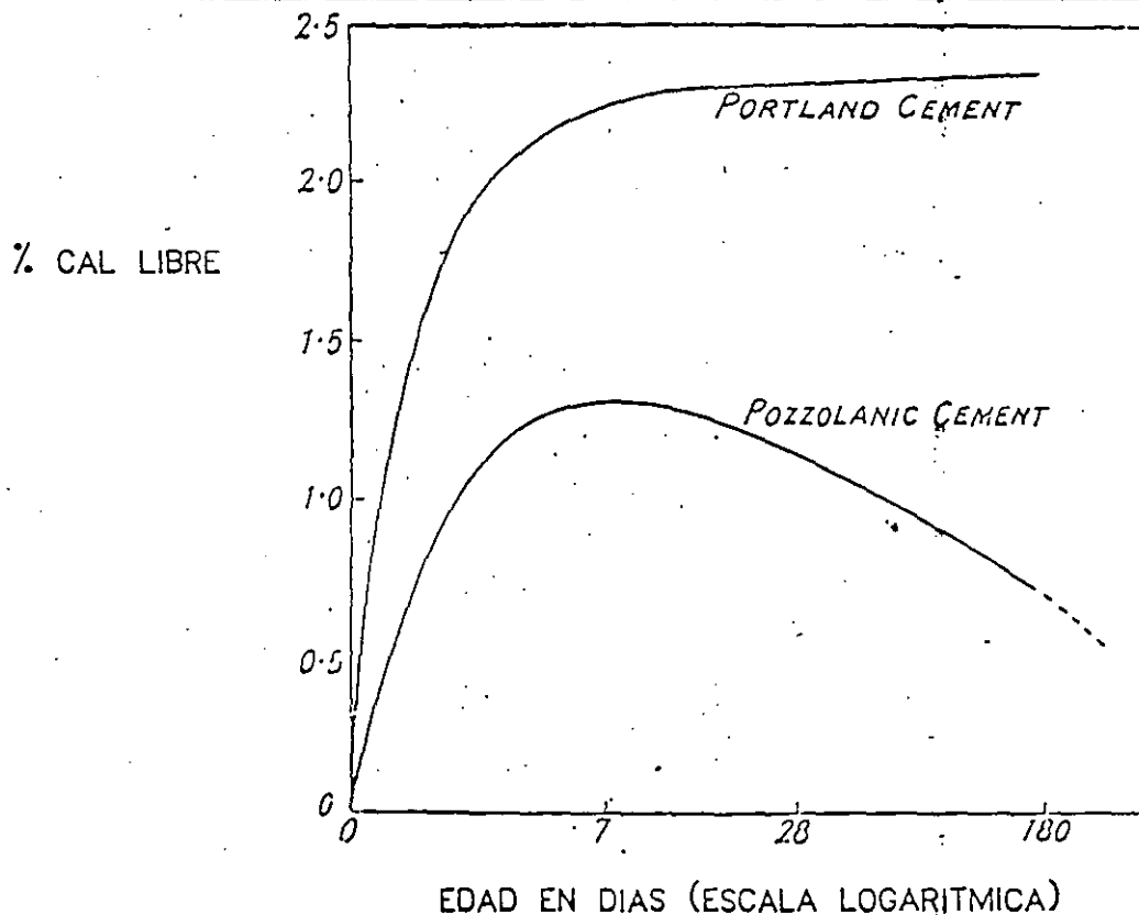
CONTENIDO DE CAL LIBRE EN MORTERO 1:3 CEMENTO-ARENA.
