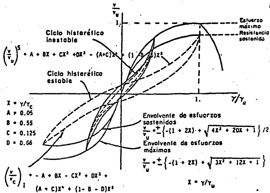
Fig 3 Comportamiento típico de muros con falla por cortante
