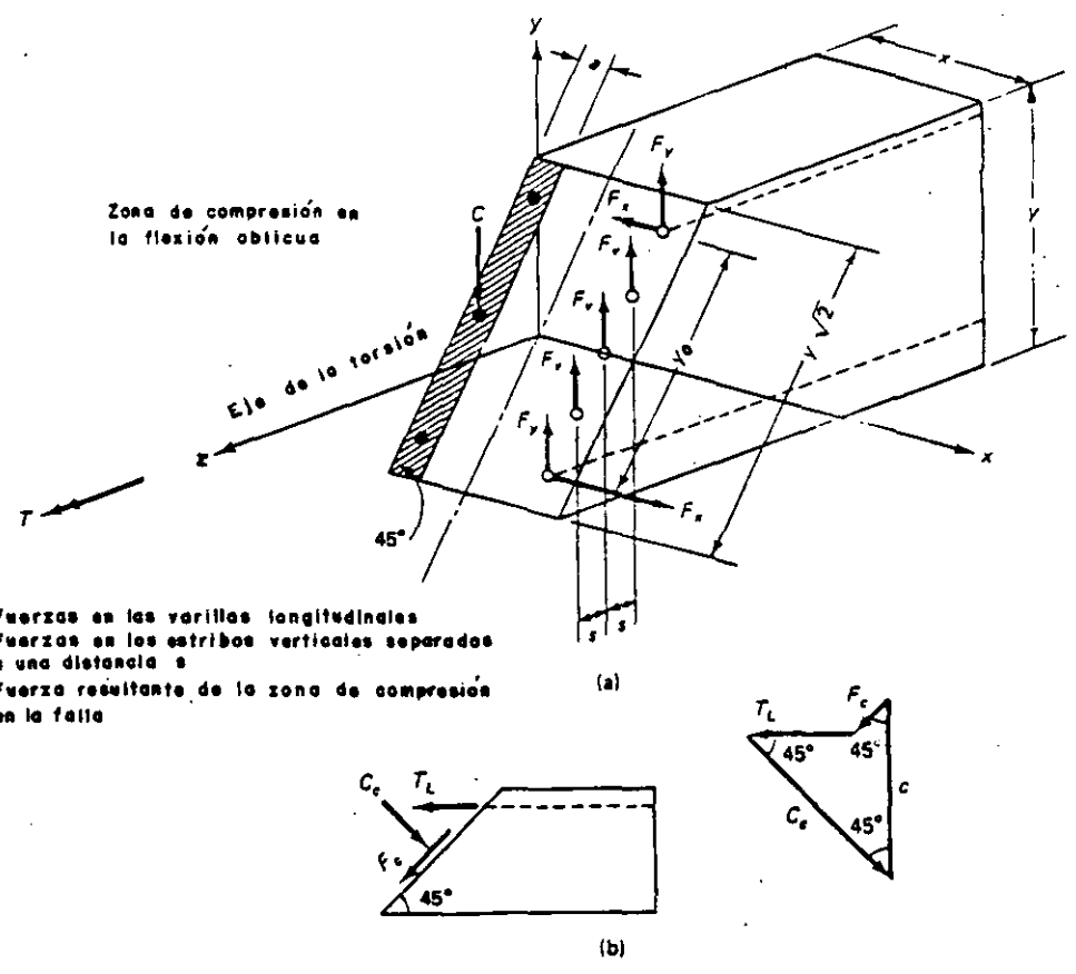
Fig. 7.8 Fuerza en los planos flexionados oblicuamente (a) Todas las fuerzas actúan en un plano oblicuo en la falla; (b) Fuerza vectoriales en la zona de compresión.
