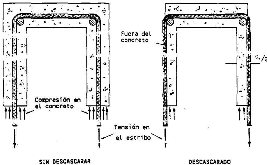
Fig. 6. Descascaramiento del recubrimiento del concreto debido al cortante.
