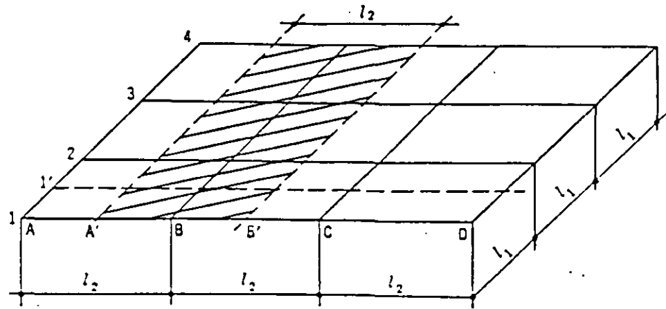
Figura 13 Franja de una losa en la cual se determinan los momentos flexionantes
