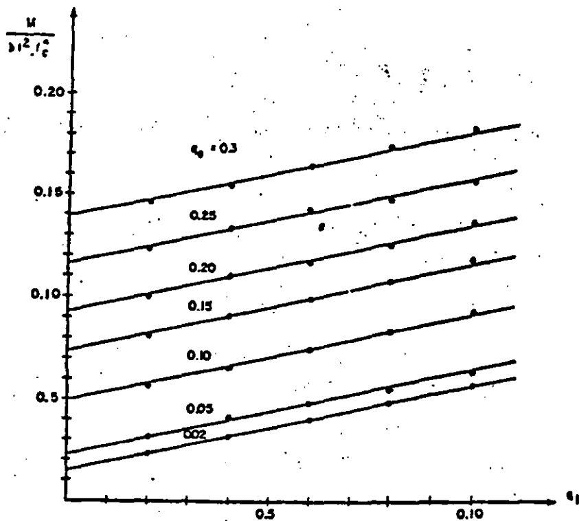
Fig 2 Variación del momento en flexión pura con la cuantía de refuerzo
