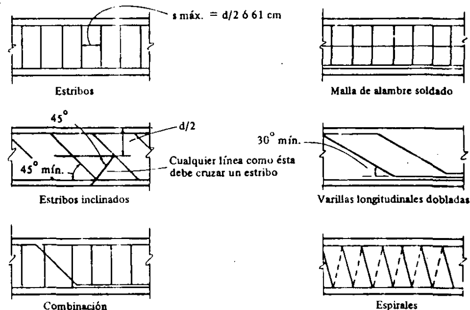
Fig. 13.7 Tipos y distribución del refuerzo por cortante.
