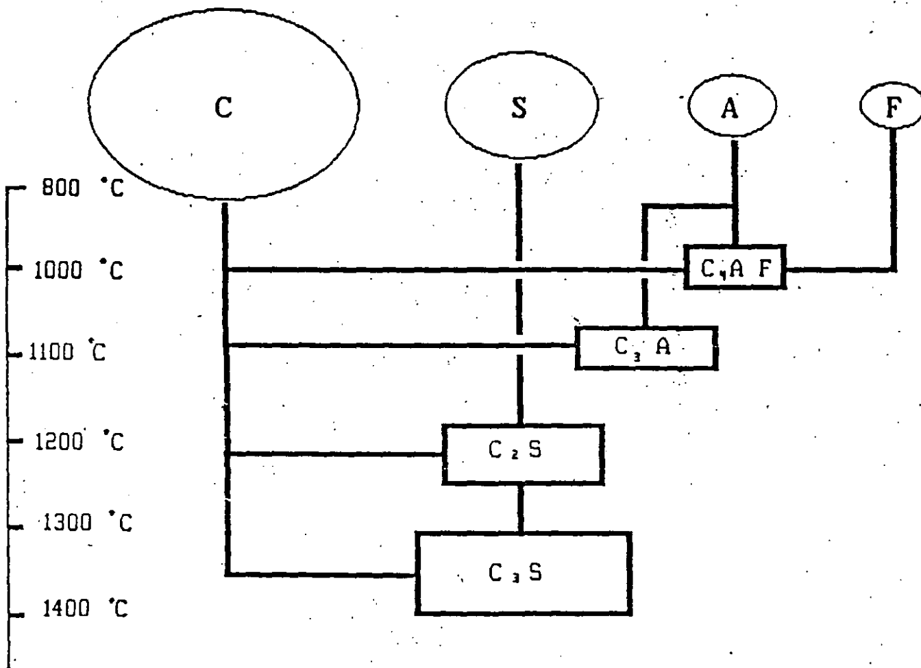
FIGURA 2.1 CLINKERIZACION
