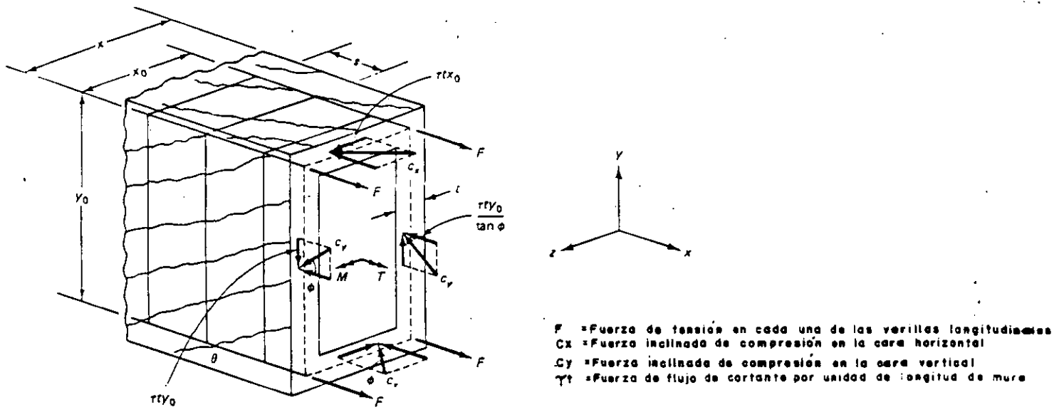
Fig.7.9 Fuerzas en la superficie del cajón hueco de concreto mediante la analogía con la armadura
