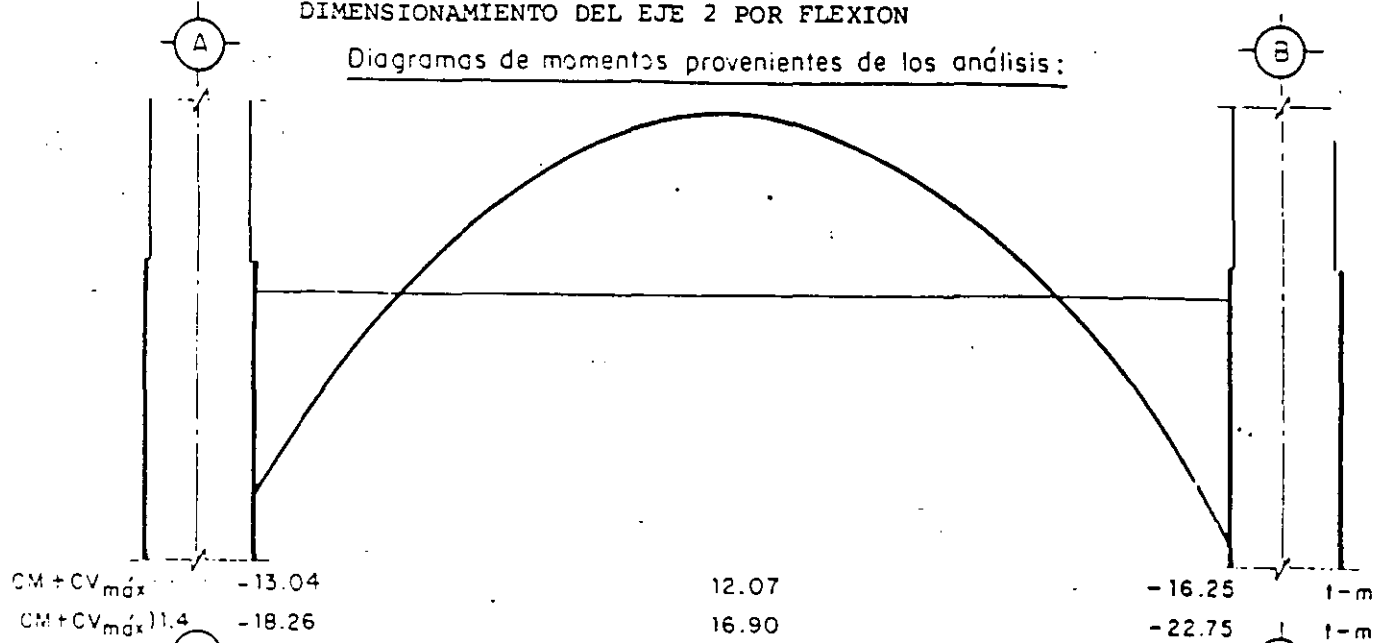
a) Bajo cargas muerta y viva máxima
