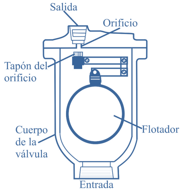
Figura 2.10. Válvula de expulsión de aire (VEA)
