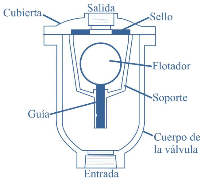
Figura 2.9. Válvula de admisión y expulsión de aire (VAEA)
