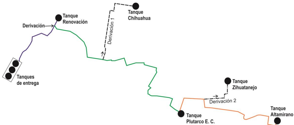
Figura 5.1. Acueducto Conejos-Médanos visto en planta
