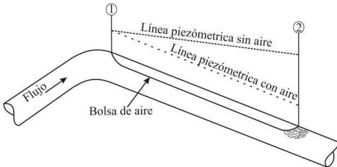
Figura 5.17. Bolsa de aire en una pendiente descendente (Edmunds, 1979)
