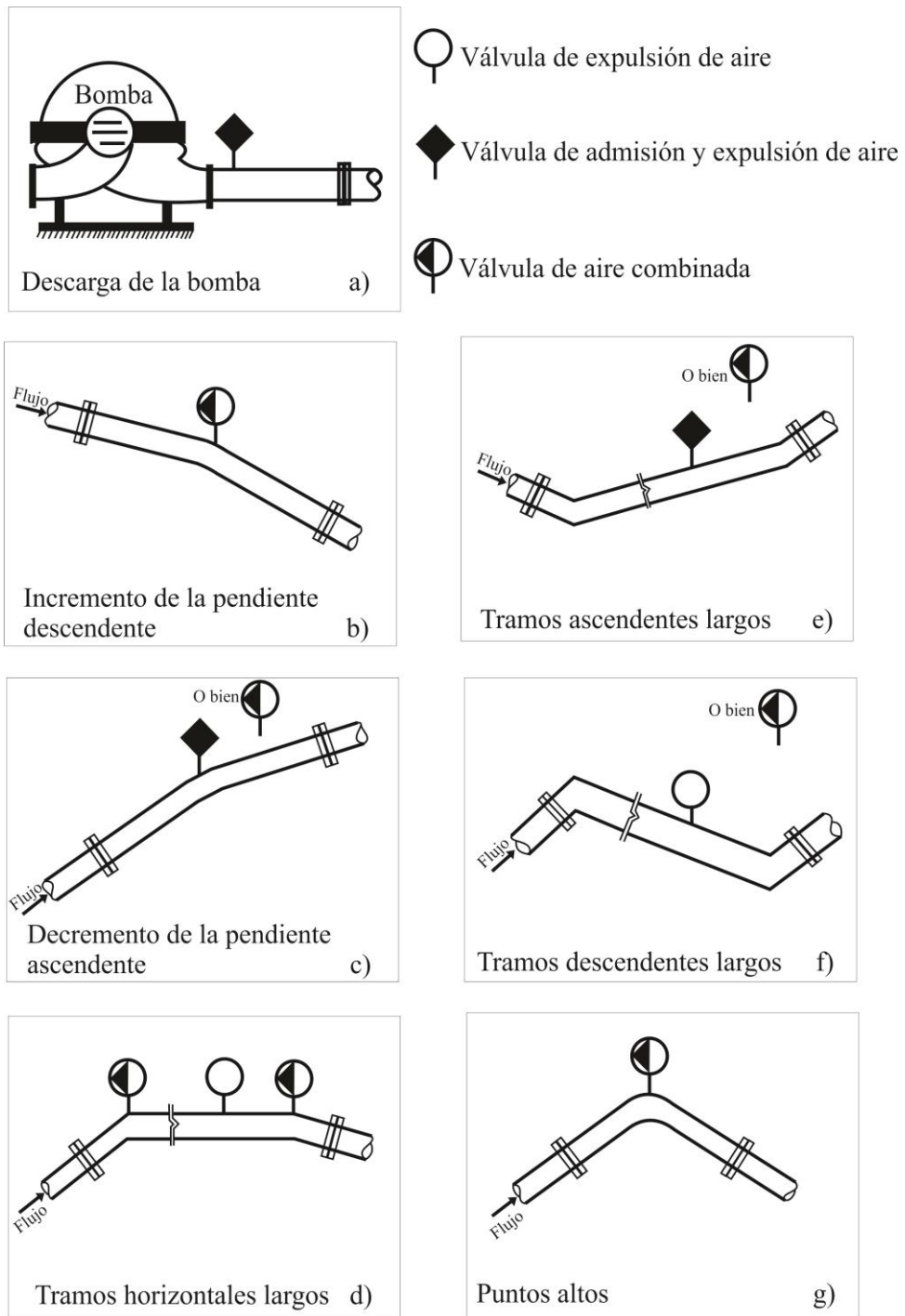
Figura 2.14. Localización de las válvulas de aire en un acueducto
