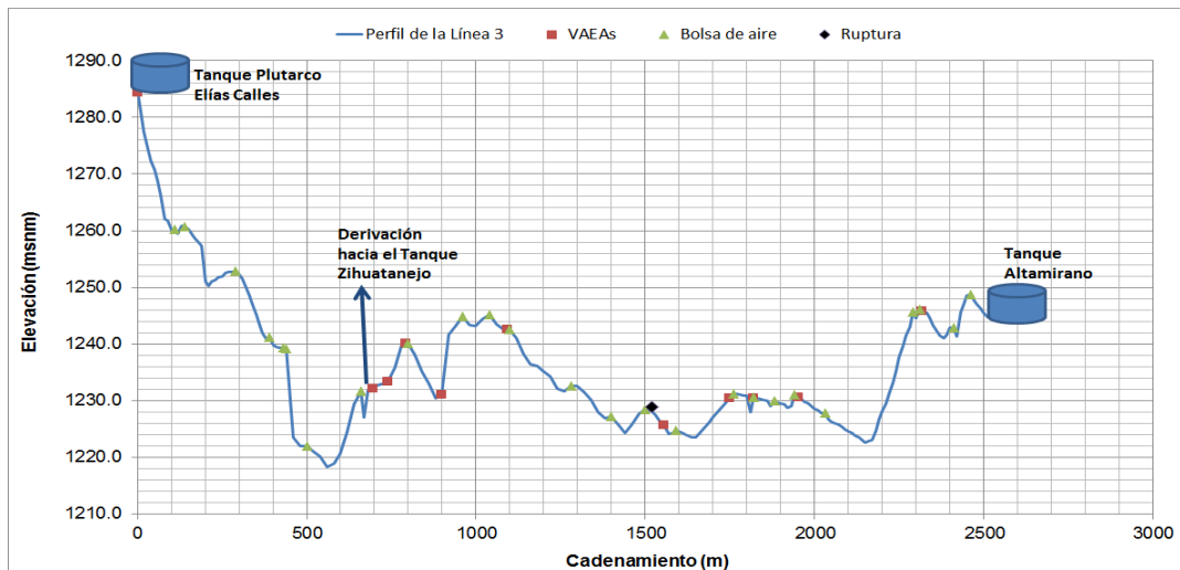
Figura 5.19. Bolsas de aire en la Línea 3, Gasto mínimo (Febrero 2012)
