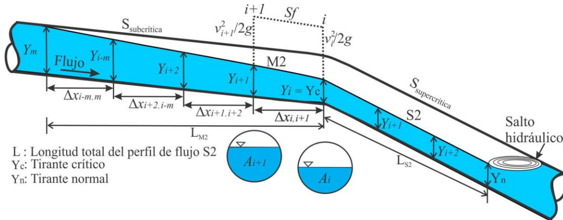
Figura 4.5. Variables utilizadas en el flujo gradualmente variado
