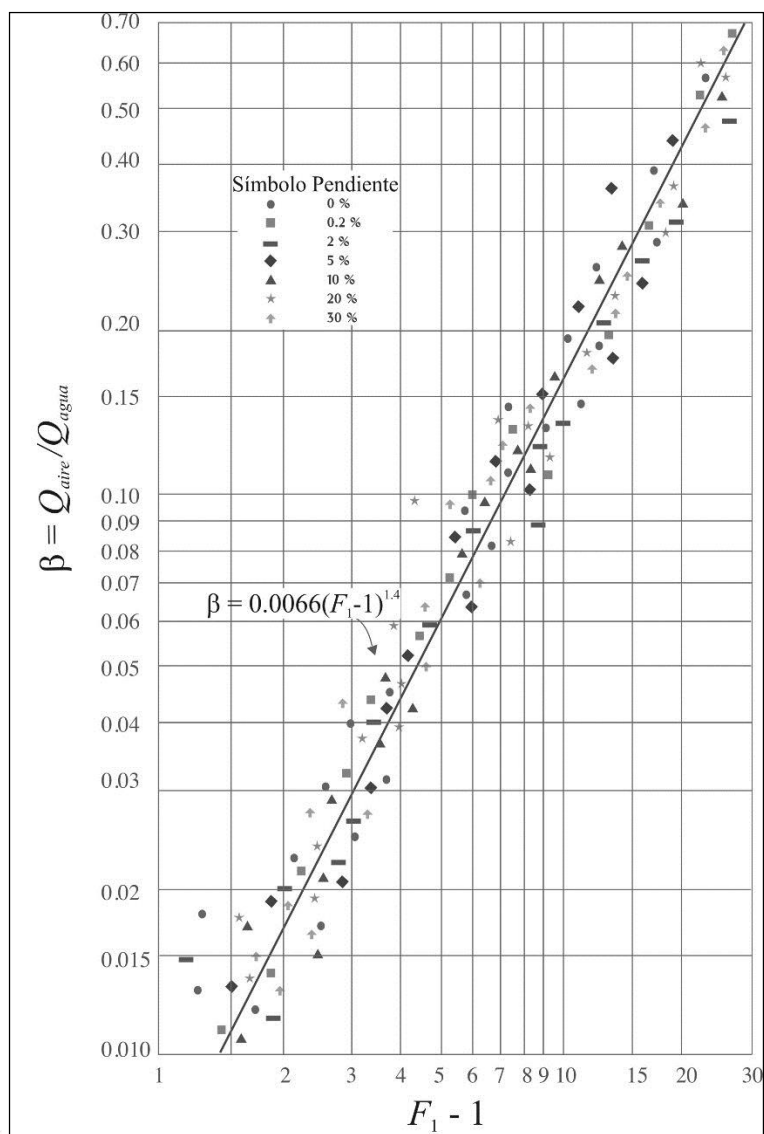
Figura 2.1. Aire ingresado en una tubería por un salto hidráulico (Kalinske y Robertson, 1943)
