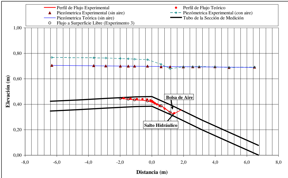
Figura 4.7. Perfiles de flujo A2 y S2, Q = 0.013 \text{ m}^3/\text{s} , V = 0.01 \text{ m}^3
