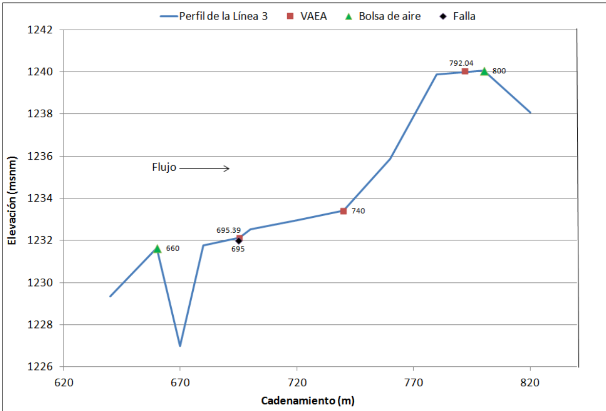
Figura 5.29. Detalle del tramo donde ocurrió la falla de la Línea 3 el 27 de mayo de 2011, Gasto mínimo de mayo de 2012
