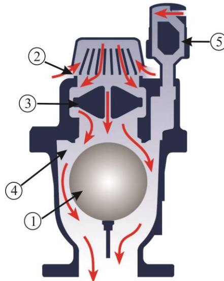
Figura 2.23. Admisión de aire
