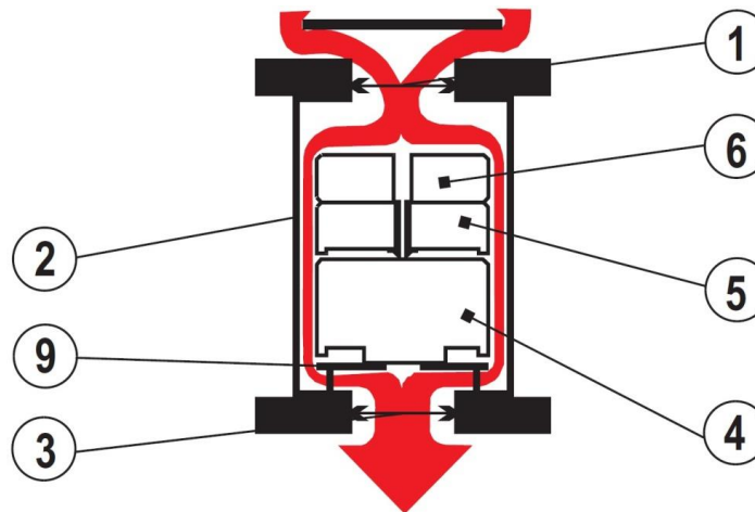
Figura 2.19. Admisión de aire
