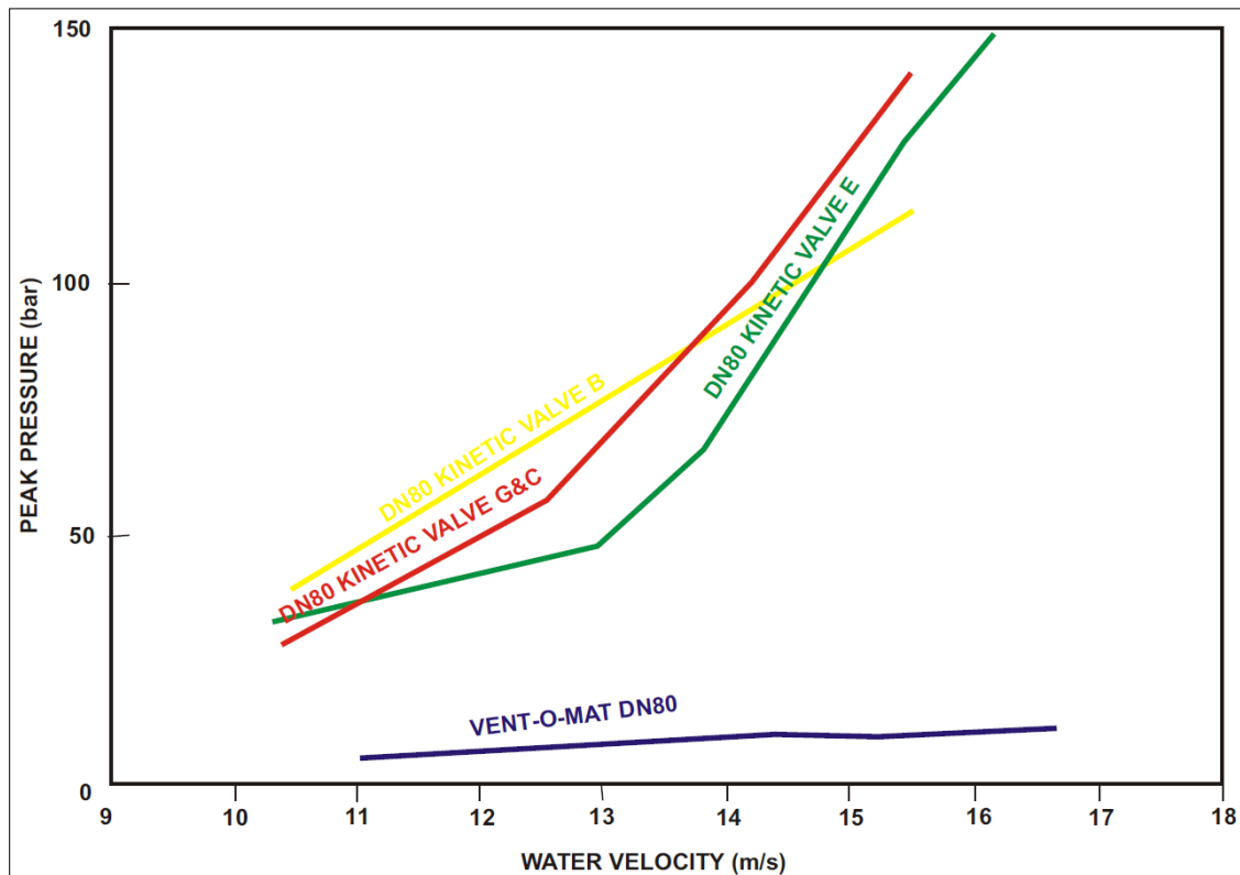
Figura 5.11. Pico de presión producido por el flujo de agua que cierra el flotador
