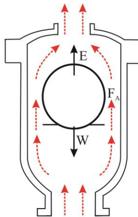
Figura 2.15. Balance de fuerzas sobre el flotador durante la expulsión de aire
