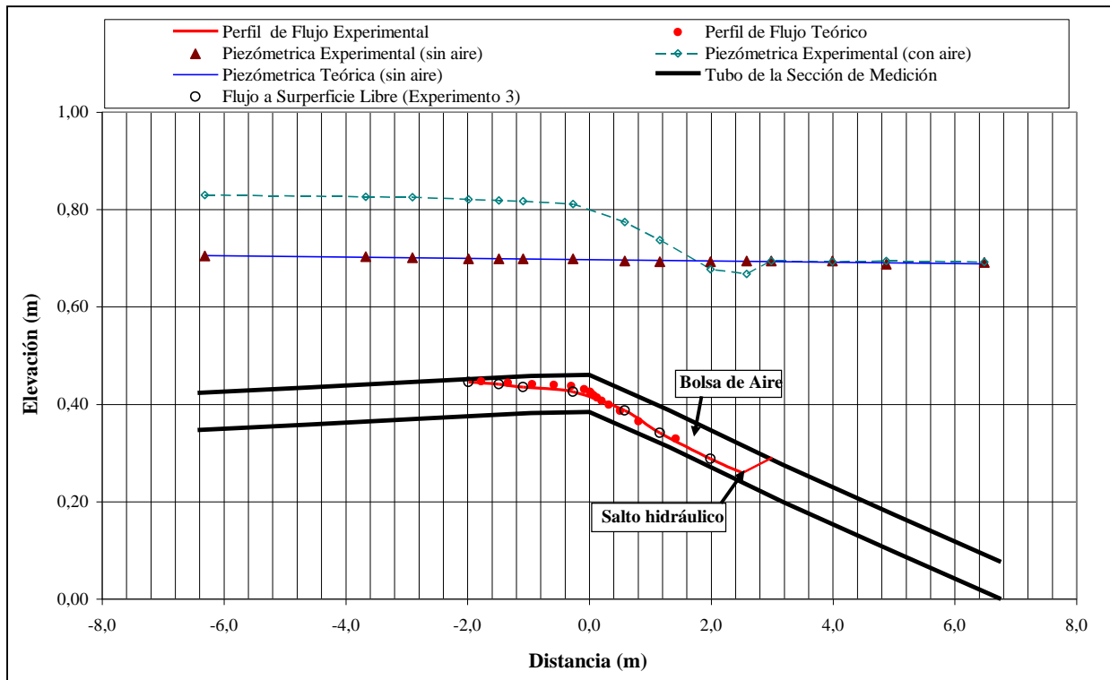
Figura 4.8. Perfiles de flujo A2 y S2, Q = 0.013 \text{ m}^3/\text{s} , V = 0.015 \text{ m}^3
