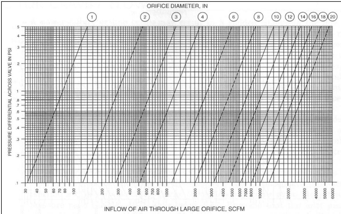
Figura 5.13. Diagrama para determinar el diámetro del orificio de una VAEA en caso de vaciar la tubería (M51 AWWA 2001)
