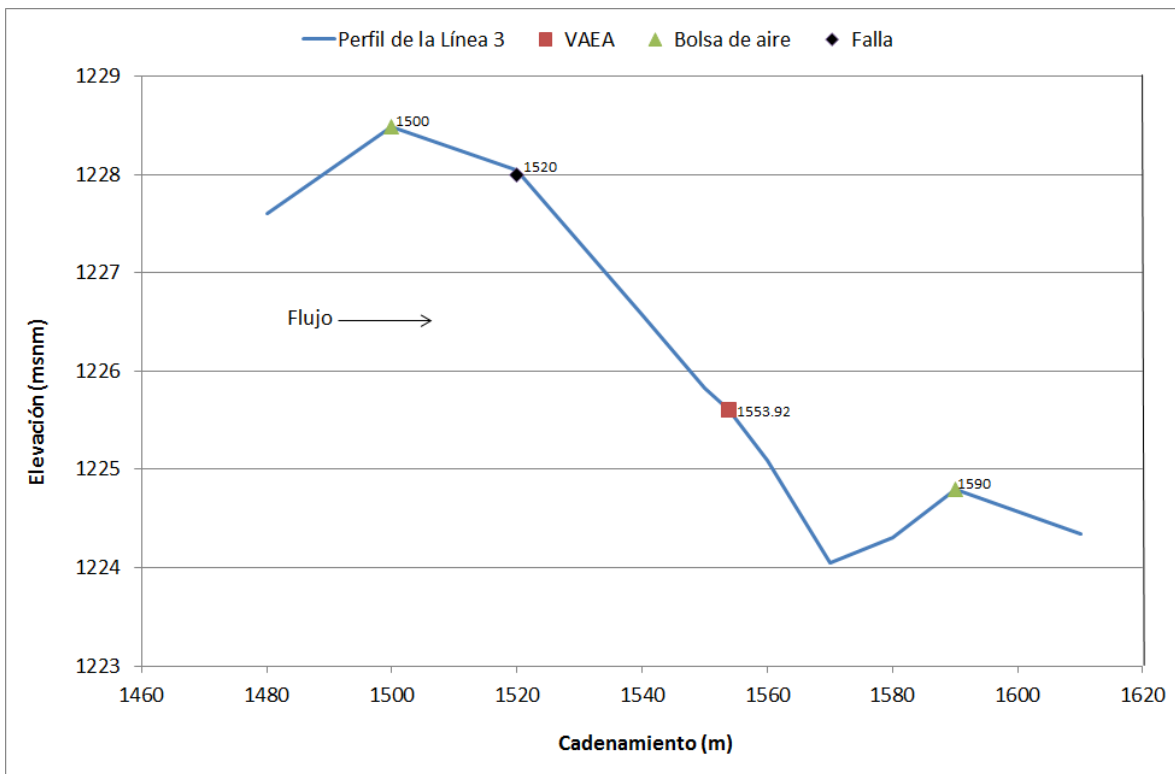
Figura 5.20. Detalle del tramo donde ocurrió la falla de la Línea 3 en febrero de 2011, Gasto mínimo de febrero de 2012
