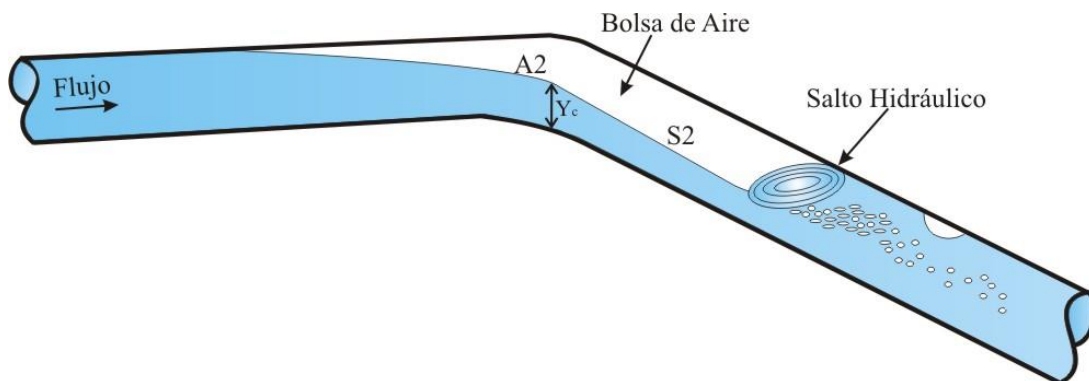
Figura 4.1. Perfiles de flujo A2 y S2
