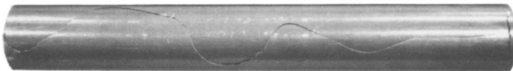
Figura 5.21. Fractura rápida en un tubo de PVC con aire atrapado
