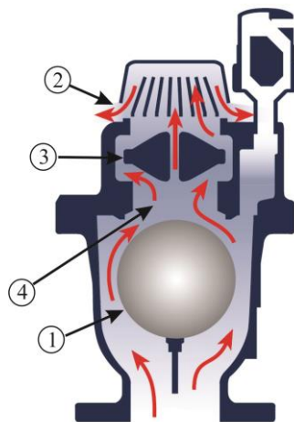
Figura 2.21. Salida de aire por orificio de menor tamaño
