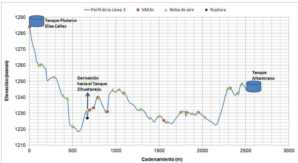
Figura 5.30. Bolsas de aire en la Línea 3, falla 12 de mayo de 2012, Gasto mínimo (Mayo 2012)
