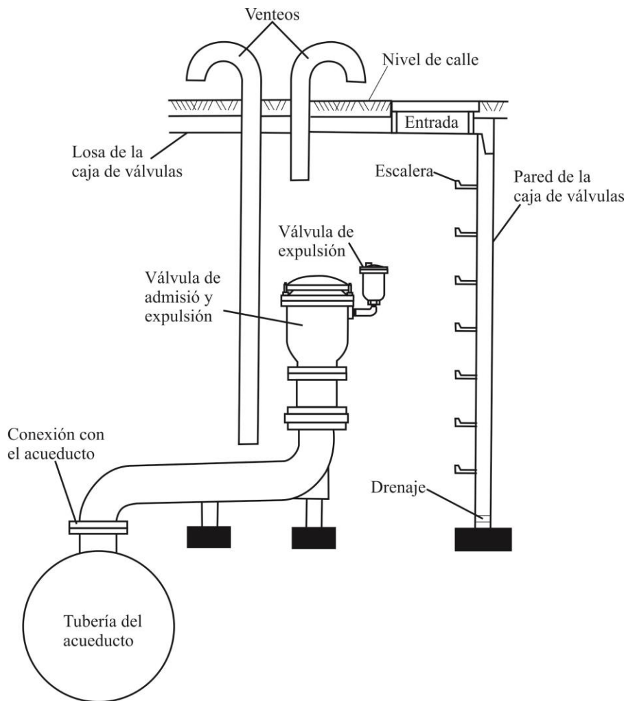
Figura 2.24 Caja de válvulas
