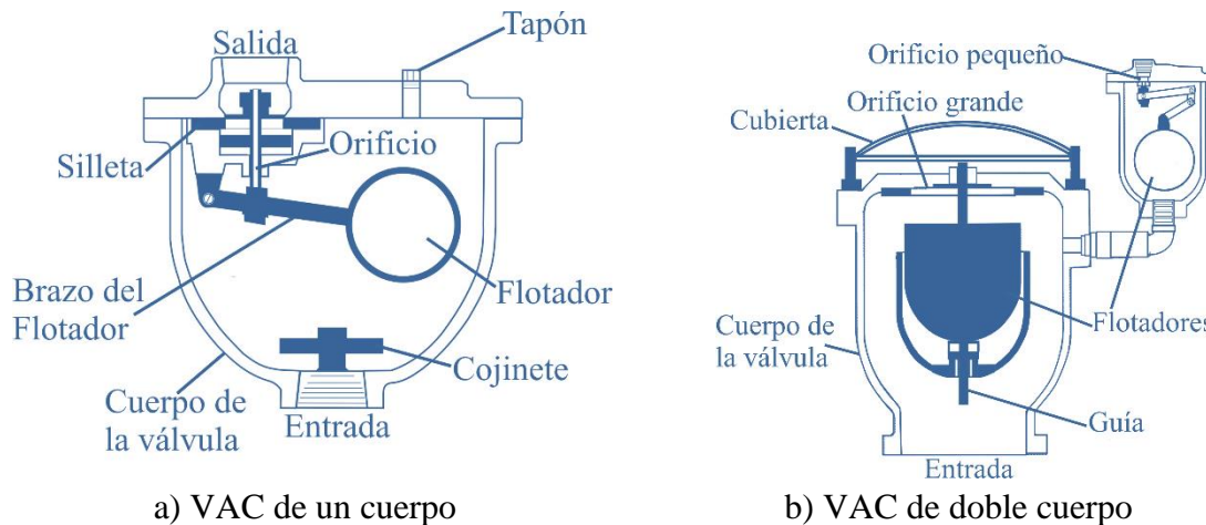
Figura 2.11. Válvulas de aire combinadas (VAC)
