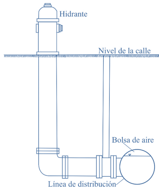
Figura 2.8. Hidrante
