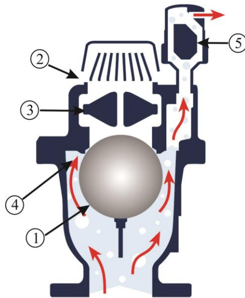
Figura 2.22. Purgador
