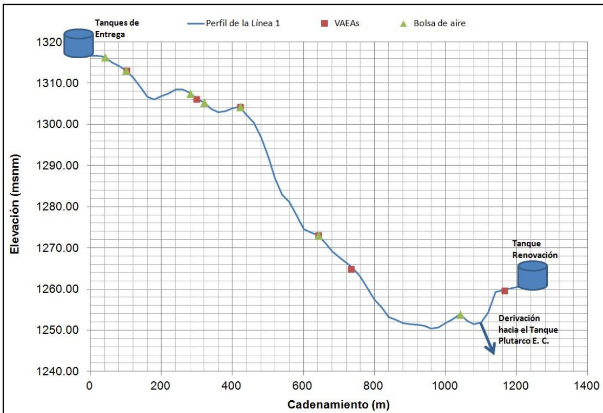
Figura 5.5. Bolsa de aire en la Línea 1, Q = 600 l/s (Julio 2012)
