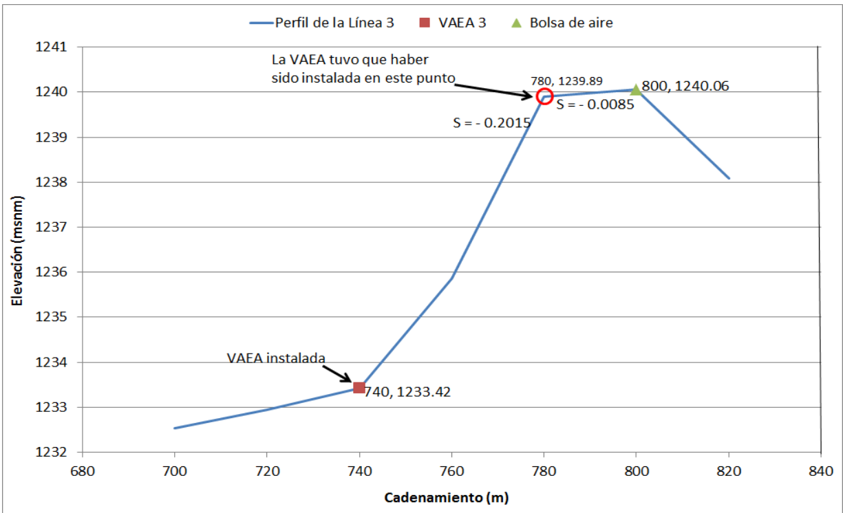
Figura 5.35. Ubicación incorrecta de la VAEA 3 en la Línea 3
