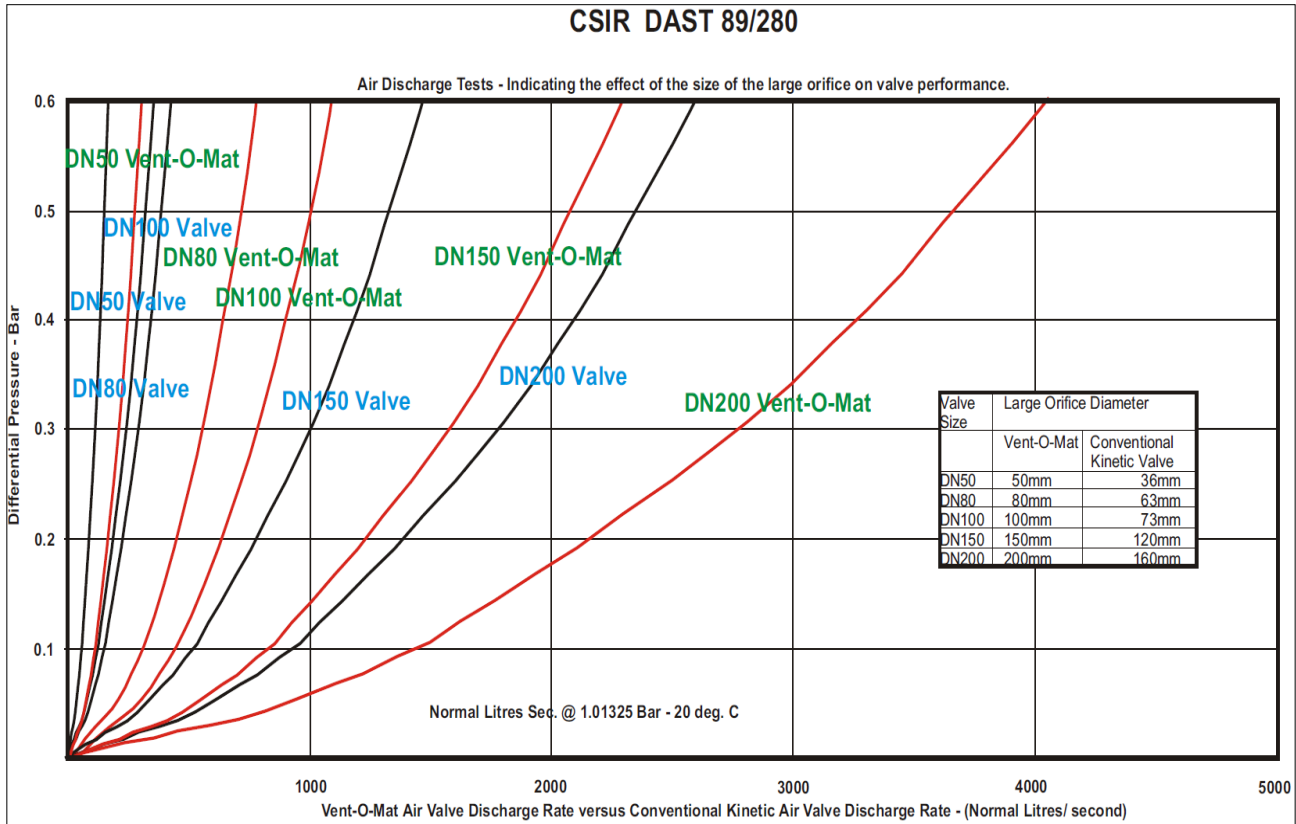
Figura 5.9. Pruebas de expulsión de aire para la VAEA Vent-O-Mat de la serie RBX y para válvulas de aire cinéticas convencionales (Plessis, 1989)
