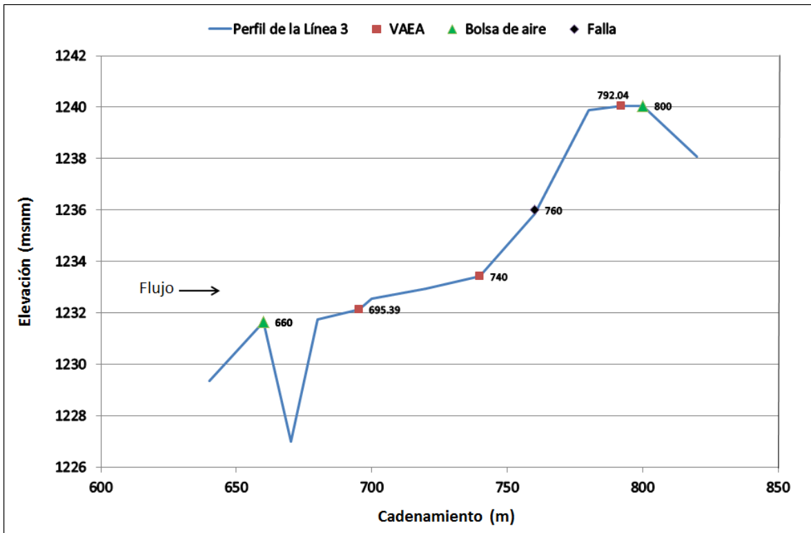
Figura 5.27. Detalle del tramo donde ocurrió la falla de la Línea 19 en abril de 2012, Gasto mínimo (Abril 2012)
