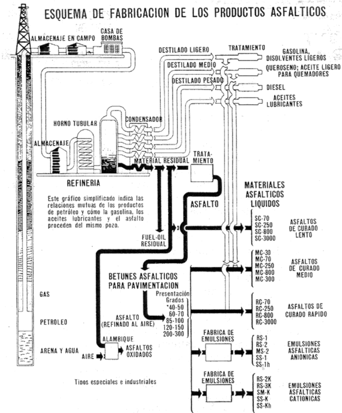
FIGURA 2.4 - DIAGRAMA DE FABRICACIÓN DE LOS PRODUCTOS ASFÁLTICOS
