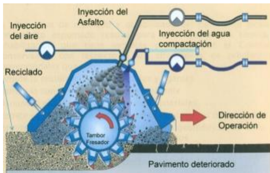
FIGURA 4.4.- PROCESO DEL ASFALTO ESPUMADO
