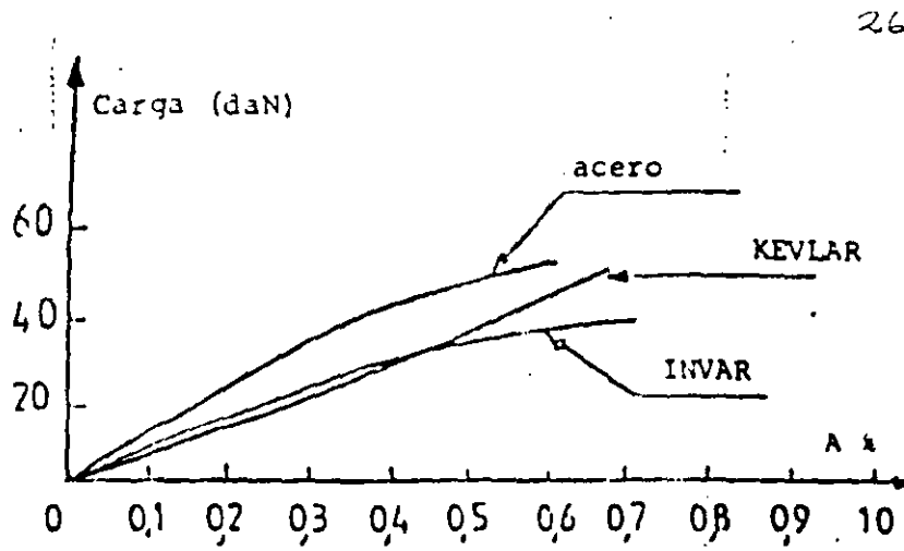
Fig. 5 r -13 Prueba de tensión para el elemento de refuerzo de la estructura cilíndrica ranurada.
