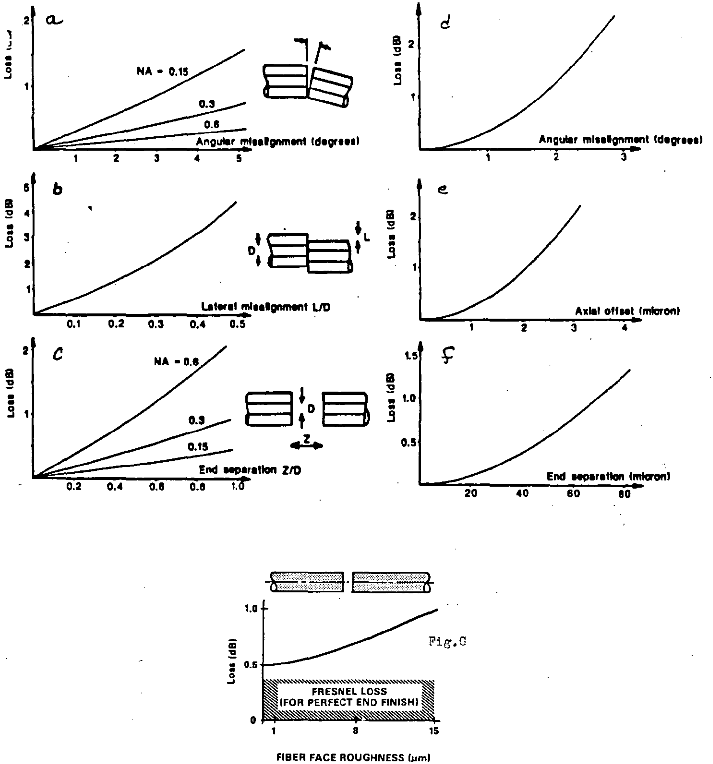
Fig.2 Pérdidas Extrínsecas. a-c y g) fibra multimodo d-f) fibra unimodo
