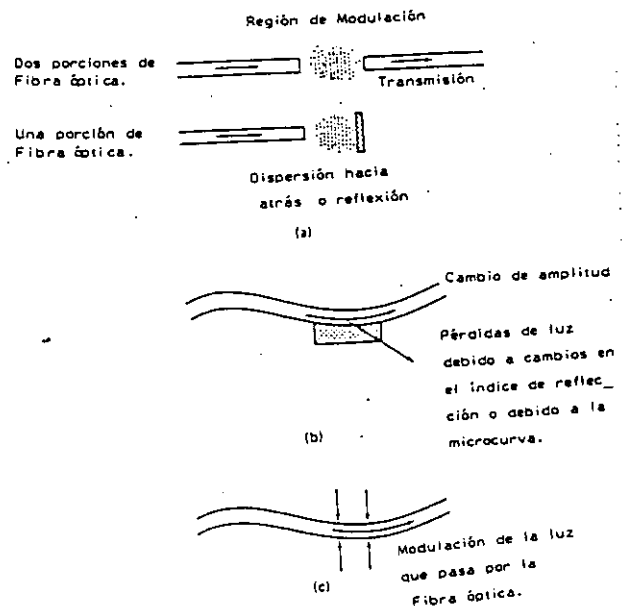
Fig. 1 Representación esquemática de los tres grupos de sensores vía fibra óptica: a) Extrínsecos, b) Evanescetes y c) Intrínsecos.
