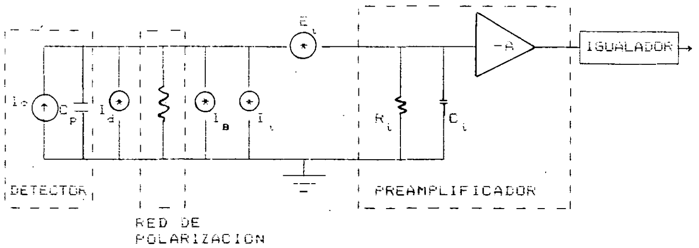
PREAMPLIFICADOR OPTICO DE ALTA IMPEDANCIA
