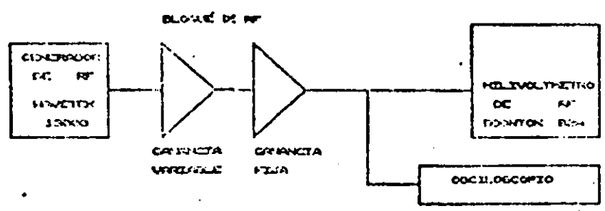
Fig.4.18.-Sistema de medición para la característica de amplitud-frecuencia del bloque de RF.
