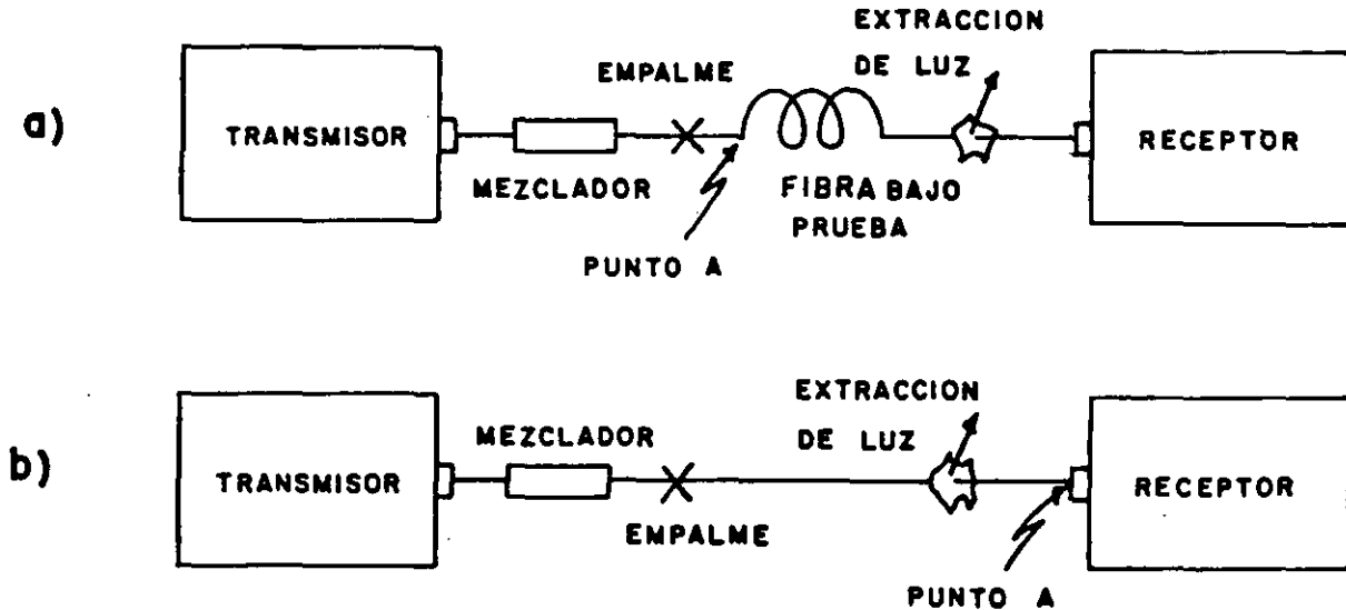
FIG. 11 .- MEDICION DE ATENUACION POR EL METODO DE CORTE REGRESIVO a) PARA EXTREMO LEJANO b) PARA EXTREMO CERCANO
