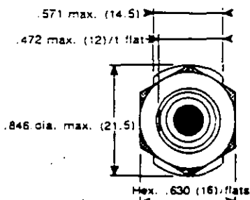
F 714 200 000 RECEPTACLE
