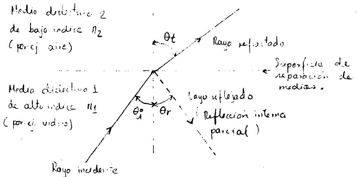
Fig. 2.2.- Refracción de rayos de luz que inciden en una interfaz de un medio de alto índice de refracción a uno de bajo índice de refracción, (por. ej. vidrio-aire).
