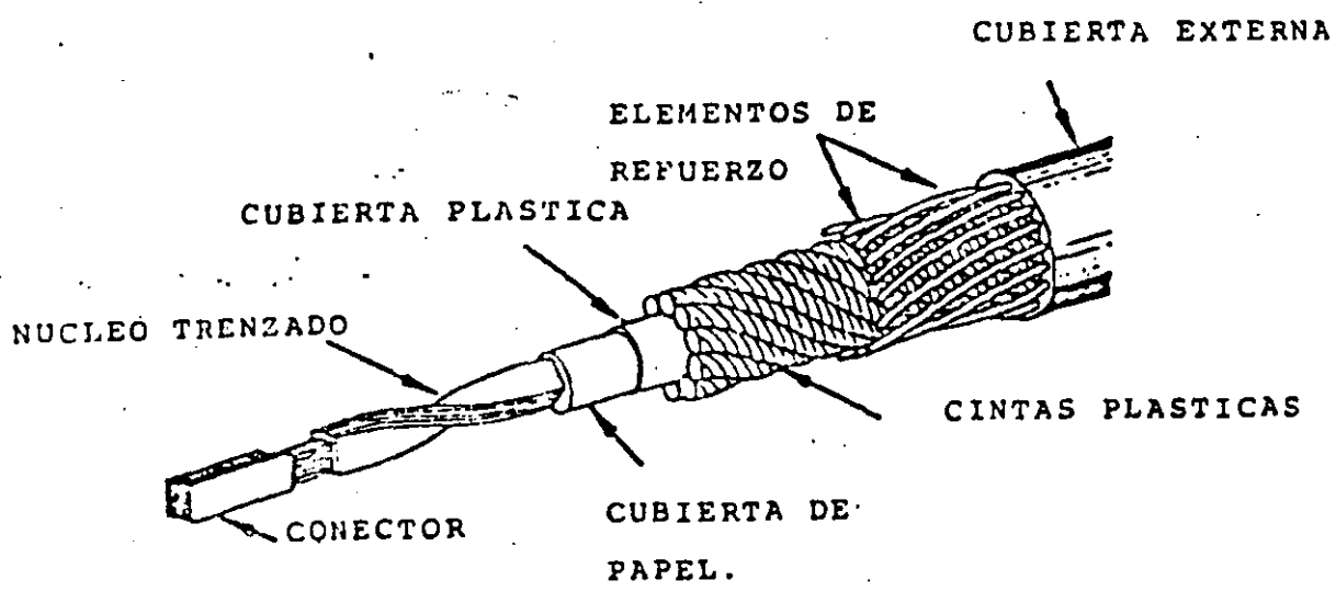
FIG. 5.-6 Cable óptico que contiene 144 fibras
