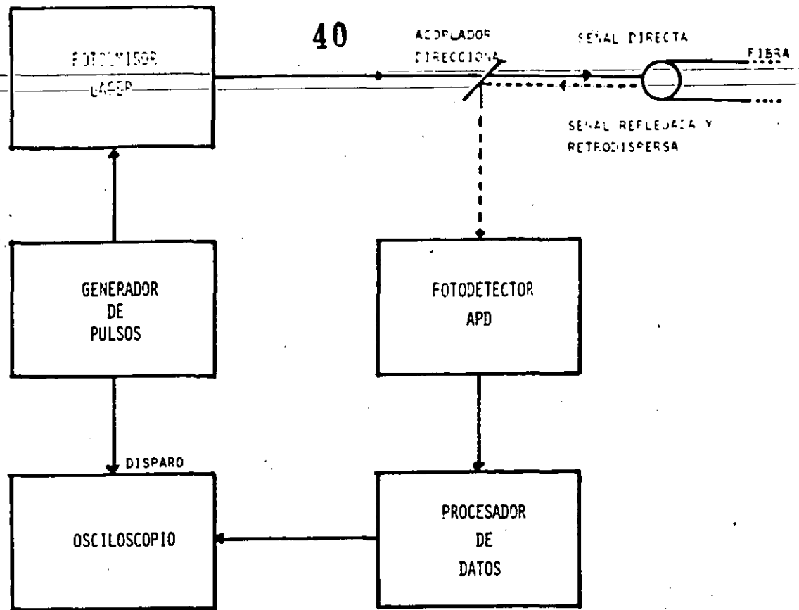
FIG. 13 DIAGRAMA BASICO DE UN ROFT
