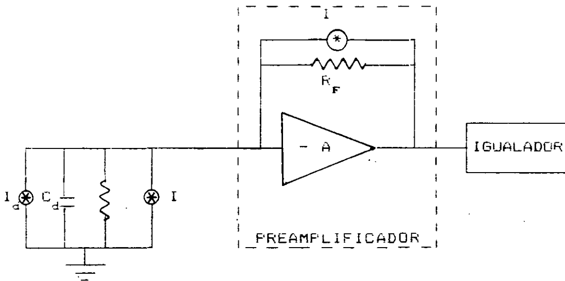
PREAMPLIFICADOR DE TRANSIMPEDANCIA
