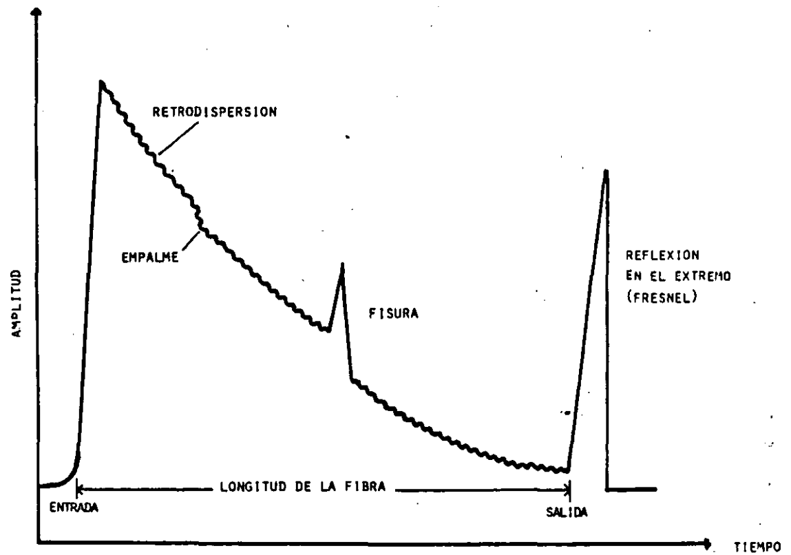
FIG. 14 SEÑAL QUE REGRESA COMO SE OBSERVA EN UN ROFT
