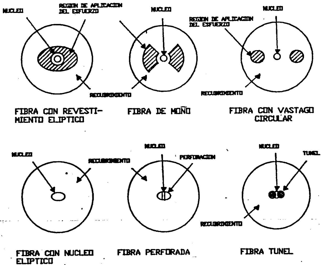
FIG. 1. TIPOS DE FIBRAS QUE CONSERVAN LA POLARIZACION
