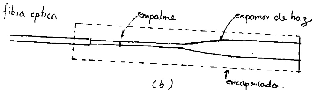
Fig. 10.- Expansores de haz para fibras unimodales.
