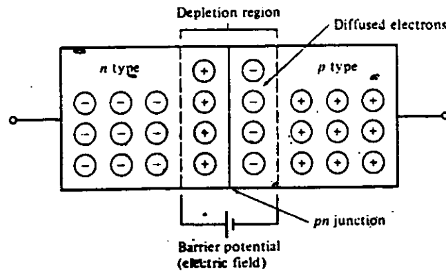
Fig. 2 Unión PN
