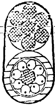
Fig. 5.-18 Cable óptico unido a mensajero
