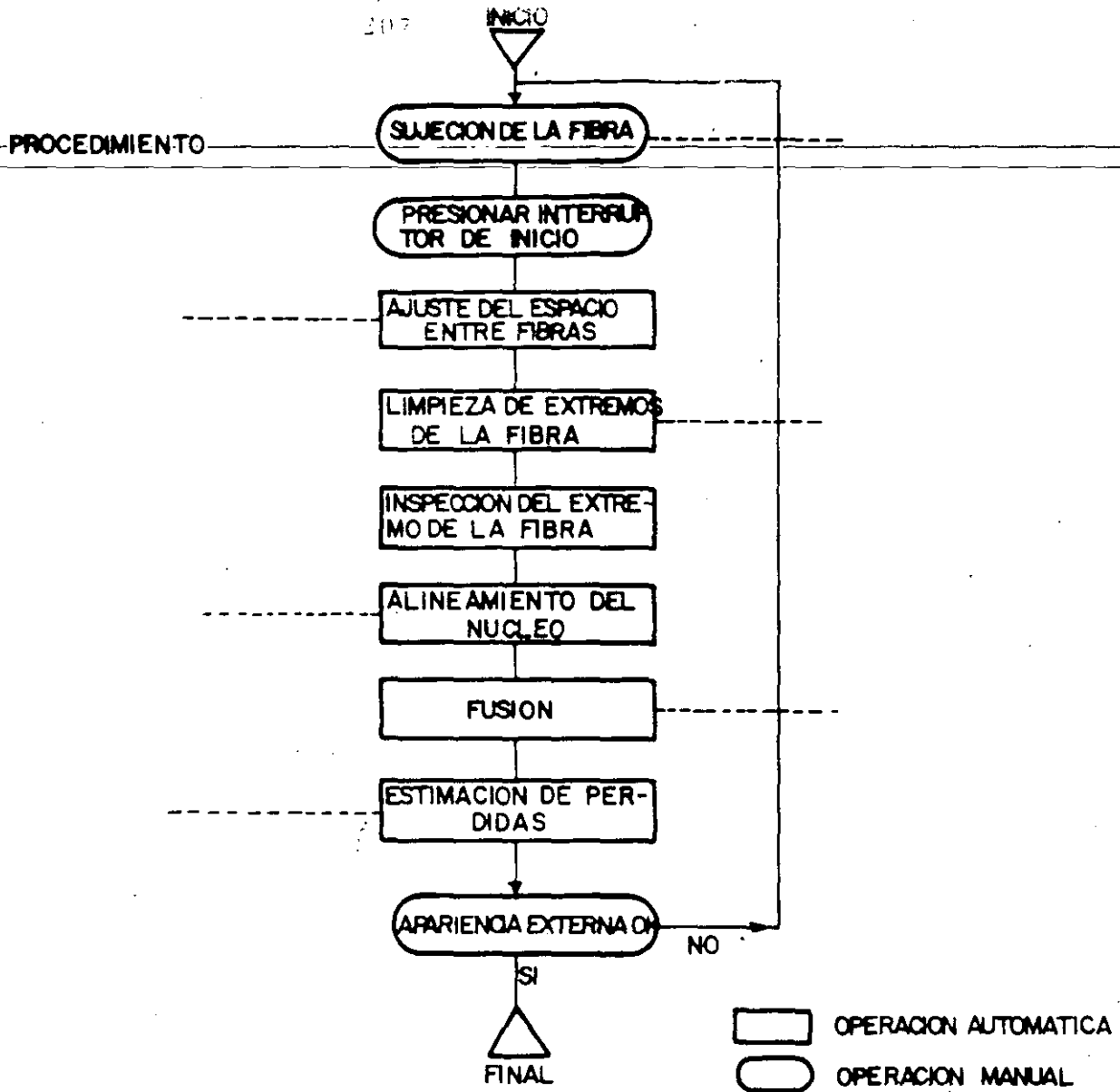
Fig. 7.19 Fusión automática de una fibra con la empalmadora Sumitomo 35.
