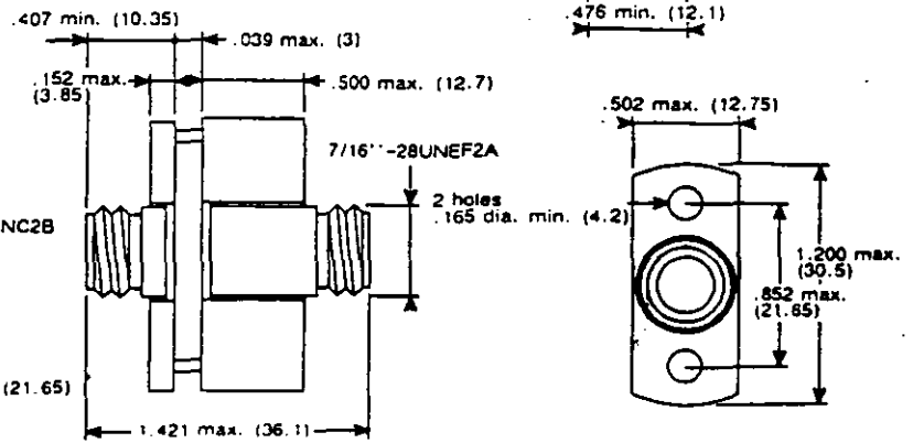
F 714 704 000 ADAPTOR
