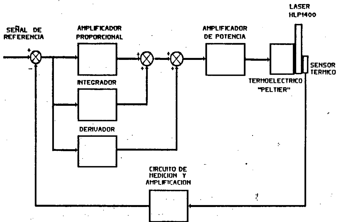
Figura 3. Diagrama o bloques del sistema de control de temperatura del láser.
