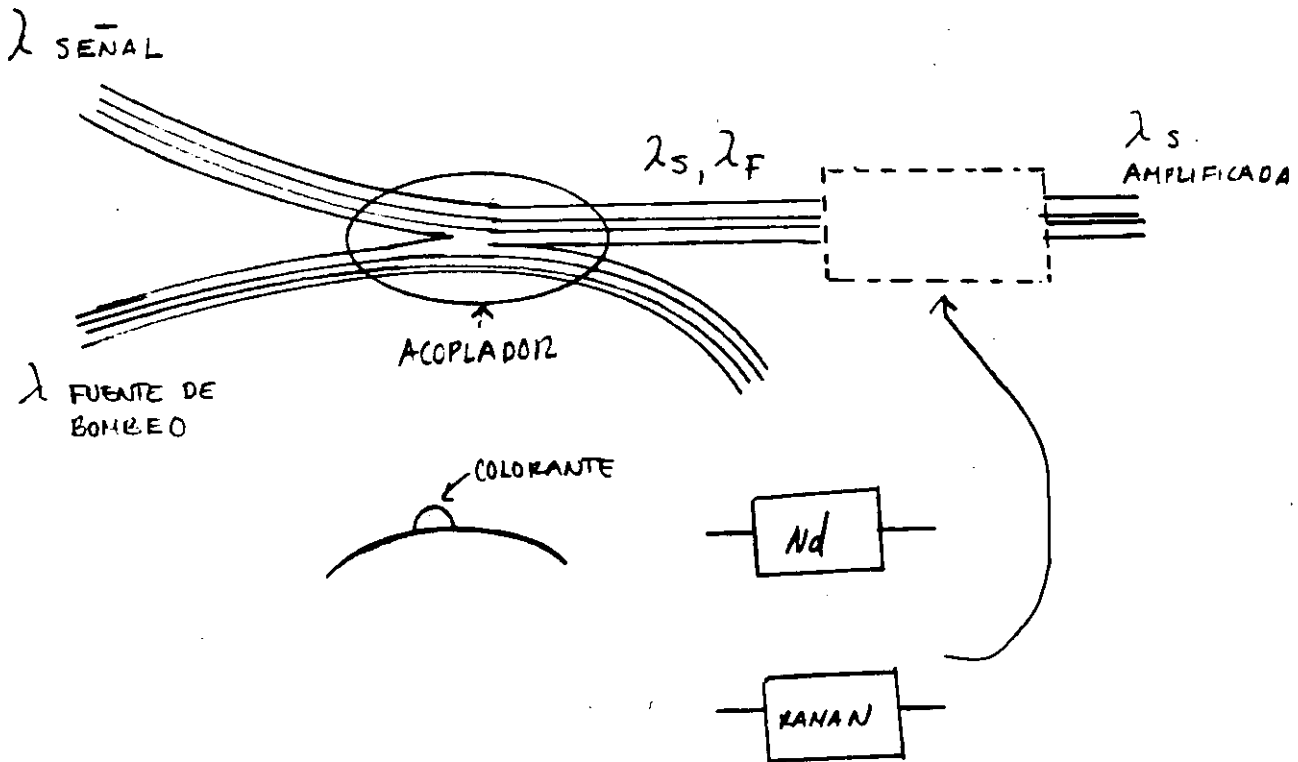
Fig. 12.- Amplificadores ópticos de fibra unimodal.
