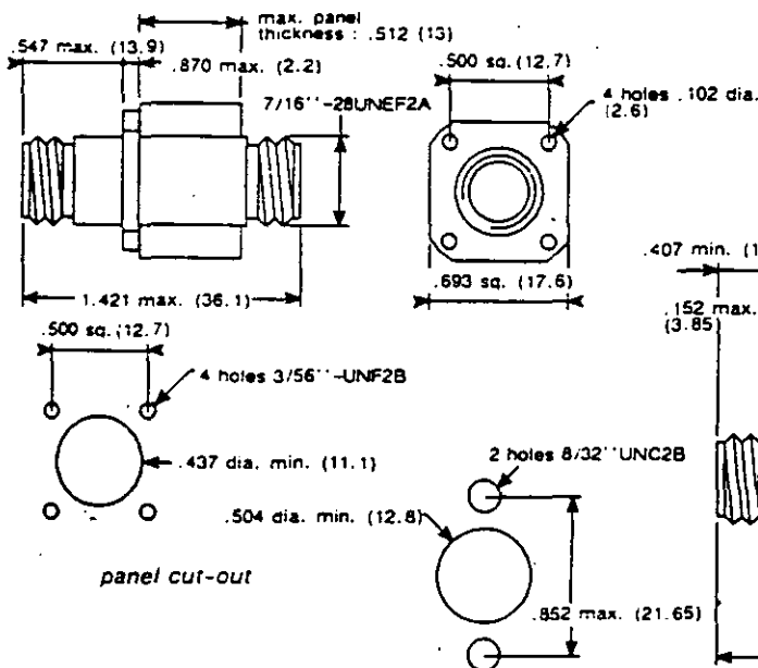
F 714 700 000 ADAPTOR
