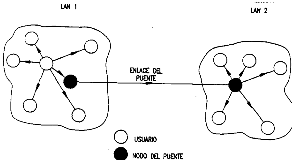
FIGURA 6. INTERCONEXION DE DOS LAN VIA UN PUENTE
