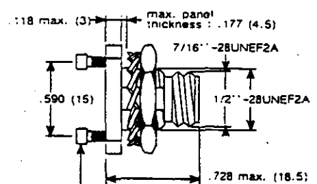
F 714 200 000 RECEPTACLE
