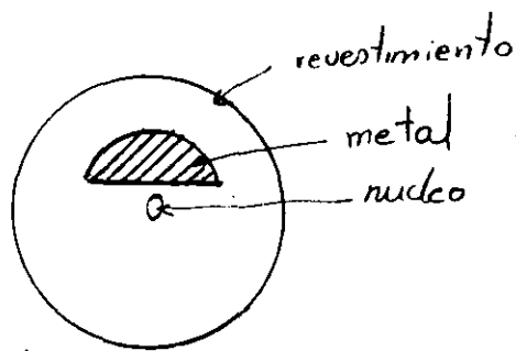
Fig. 8.- Sección transversal del polarizador de estructura compuesta fibra óptica unimodal-metal.
