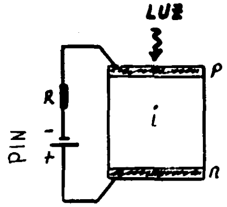
ESTRUCTURA DEL PIN
