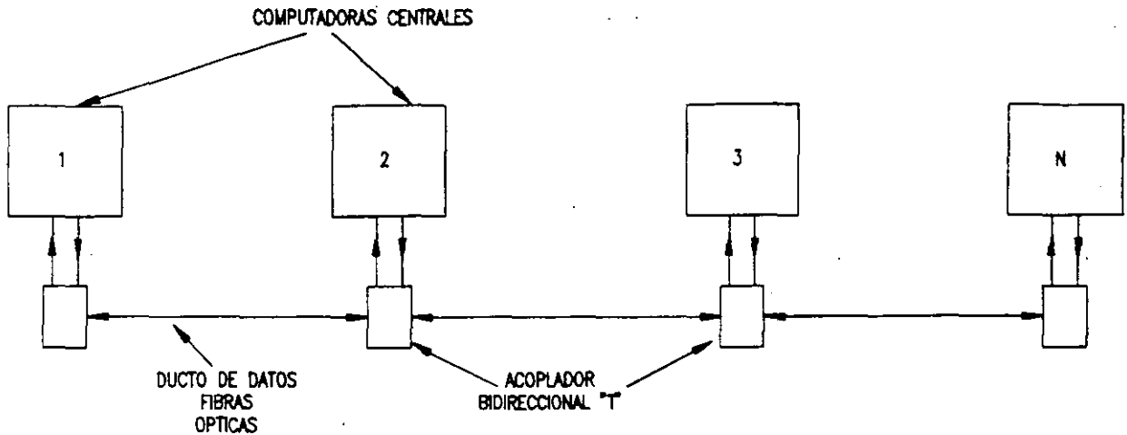
FIGURA 4. DERIVADOR EN DUCTO EN LINEA CON ACOPLADOR PASIVO EN "T"
