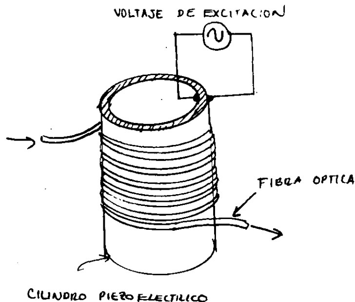
Fig. 11.- Modulación por contracción-expansión de un cilindro piezo-eléctrico.
