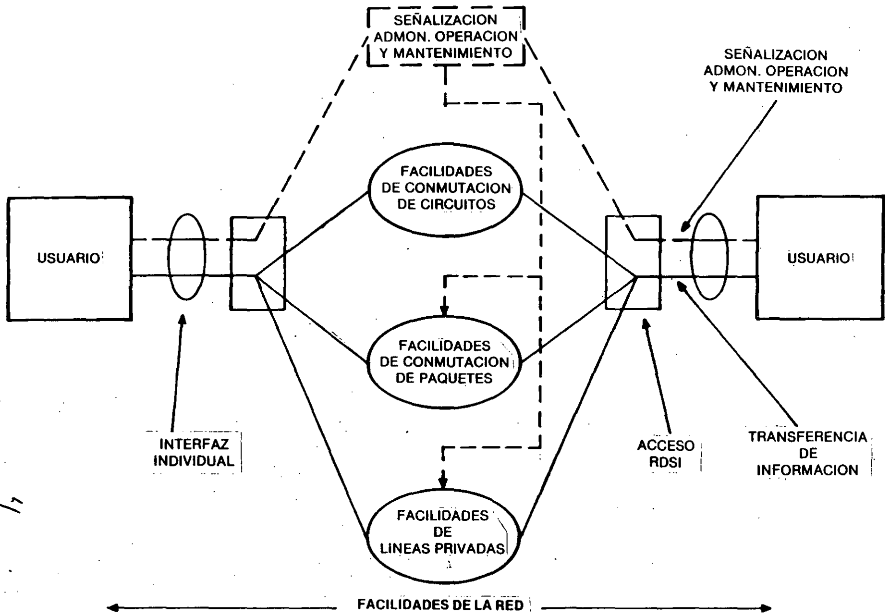
ARQUITECTURA BASICA DE LA RDSI
