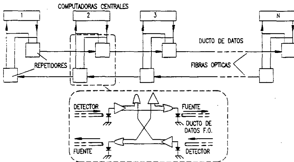
FIGURA 5. DERIVADOR DE DUCTO EN LINEA CON ACOPLADOR ACTIVO EN "T"
