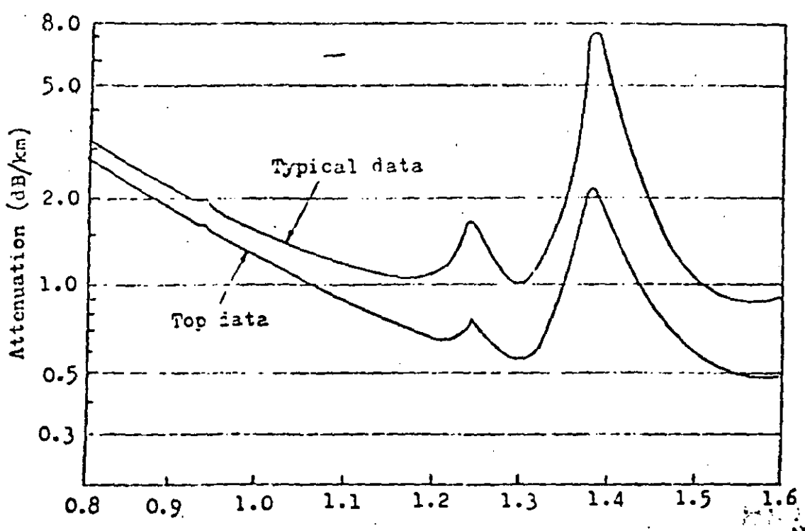
Figura (2.3.12).- Atenuación índice gradual (SUMITOMO)
