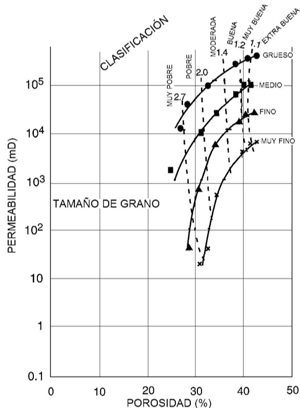
Figura 3.28 Gráfica que muestra la relación entre propiedades petrofísicas y sedimentos en arenas no consolidadas. (De Nagtegaal, 1978. Cortesía de la sociedad geológica de Londres.) 4 .
