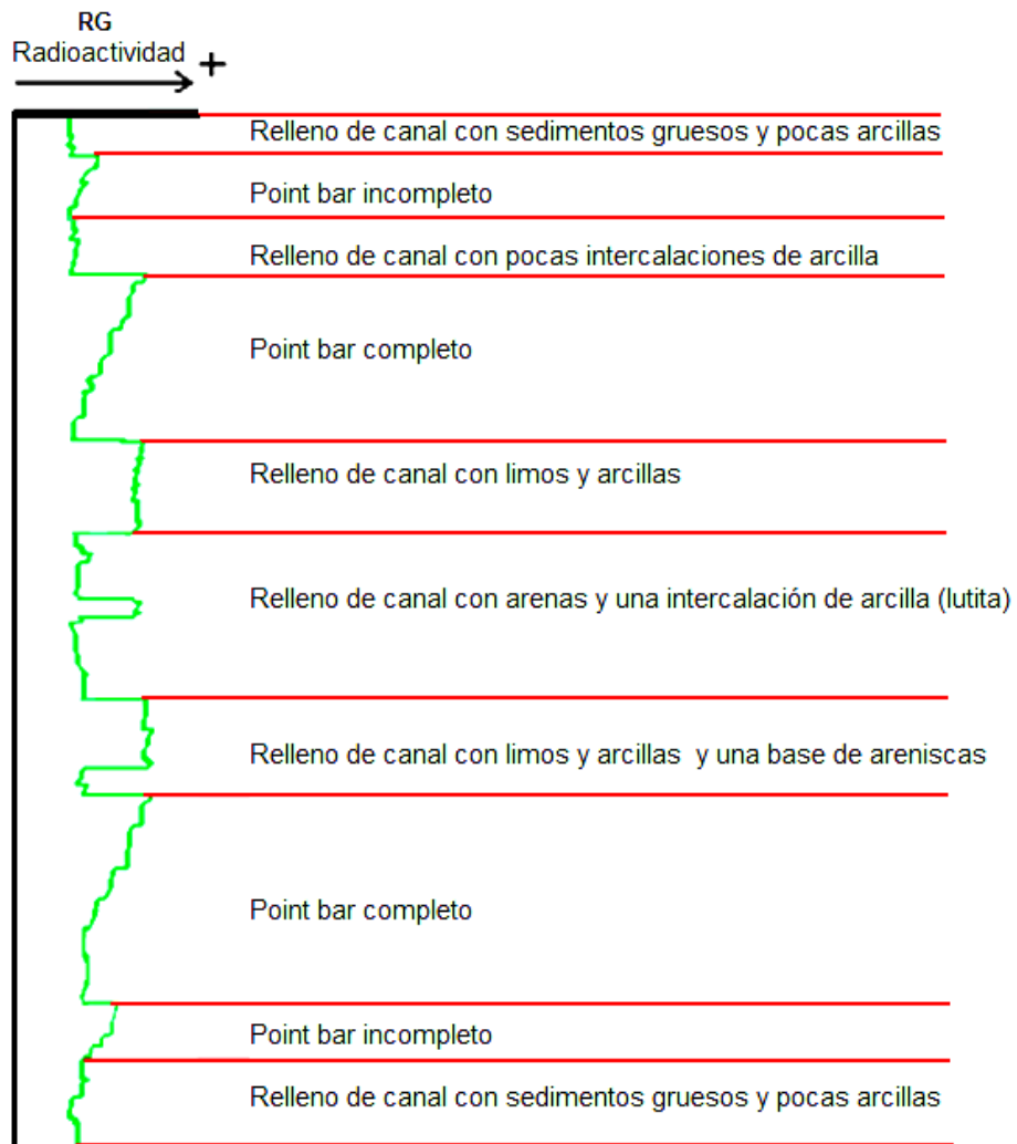
Figura 3.23 Perfil estratigráfico de relleno de valle, con base en el registro de radioactividad 2 .
