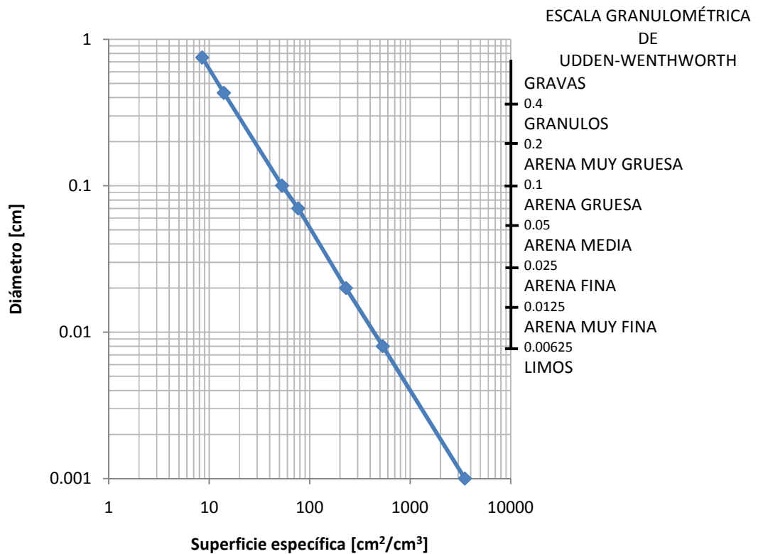
Figura 1.2.4 Relación gráfica entre el diámetro de esferas y la superficie específica de un medio poroso formado por esferas del mismo tamaño con empaquetamiento cúbico 14 .
