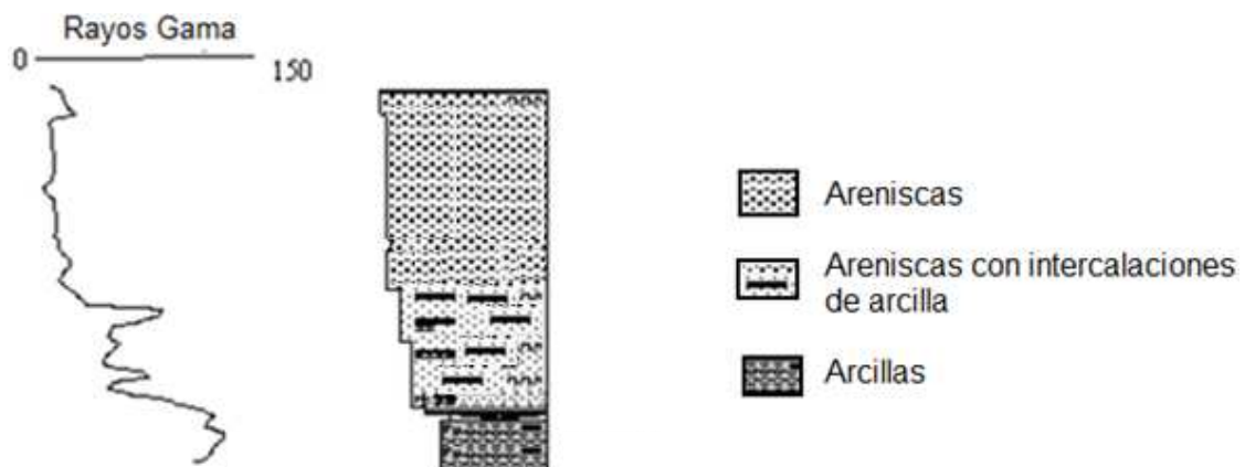
Figura 4.17. Comportamiento del registro de rayos gama del pozo A-10 del yacimiento Barúa. 7
