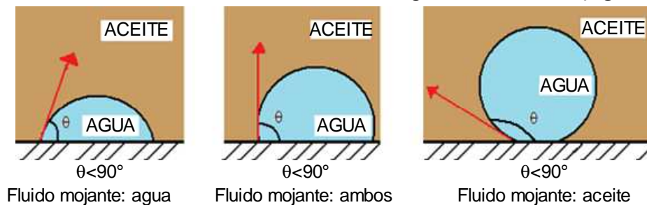
Figura 1.2.6 Determinación del fluido mojante en función del ángulo \theta . 14
