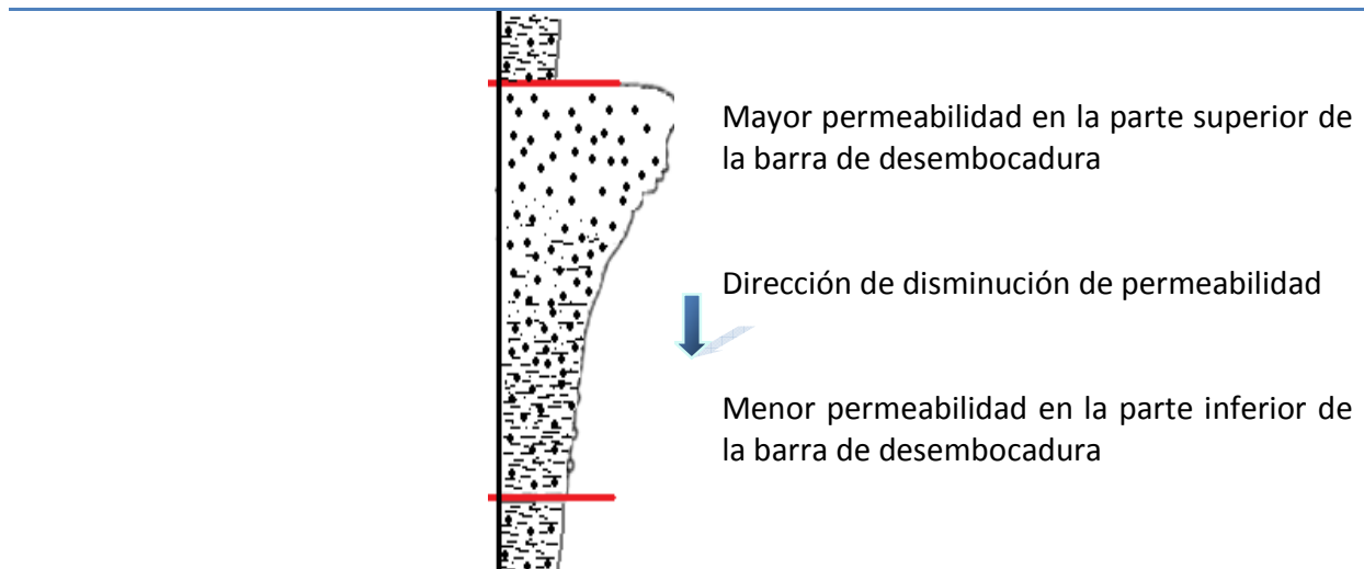
Figura 5.21 Distribución de permeabilidad en la barra de desembocadura
