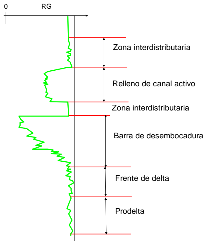
Figura 5.18 Ejemplo teórico de registro de radioactividad natural de un intervalo con espesor grande de un complejo deltaico 8
