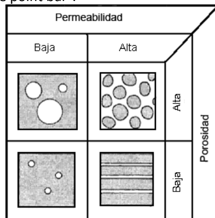
Figura 3.25 Relación de porosidad y permeabilidad con tamaño y arreglo de sedimentos 4 .
