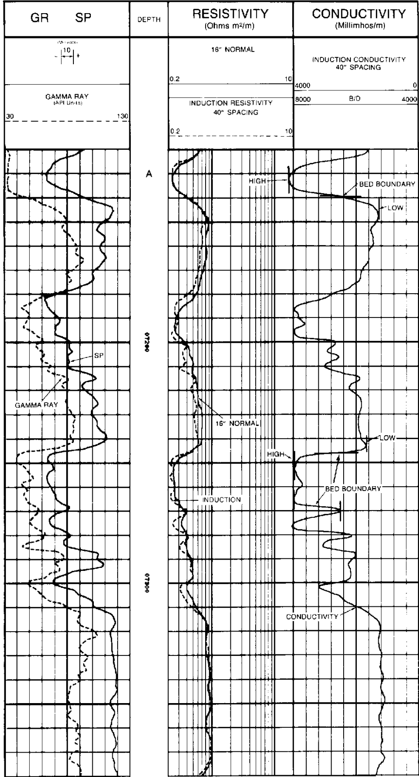
Figura 1.1.20 Ejemplo de registro de Rayos Gamma Naturales en combinación con SP y eléctricos 8
