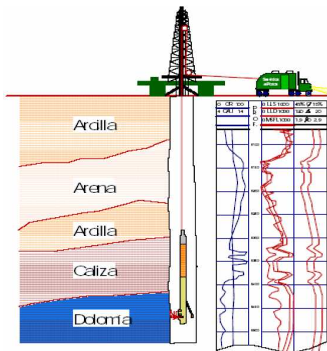
Figura 1.1.19 Diagrama esquemático de la toma de registros 7
