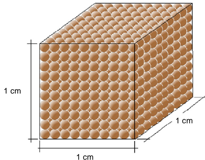
Figura 1.2.3 Esquema de arreglo cúbico de granos en un cubo de 1 cm por lado. La superficie de contacto entre granos es tan pequeña que no se considera en el cálculo de superficie específica 11
