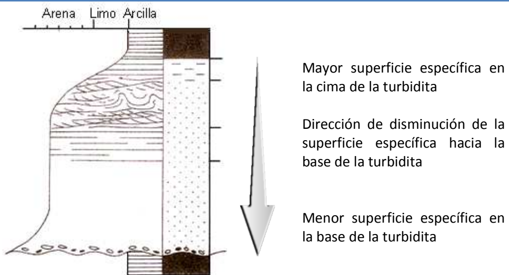
Figura 6.18 Distribución de la superficie específica en rocas de origen turbidítico
