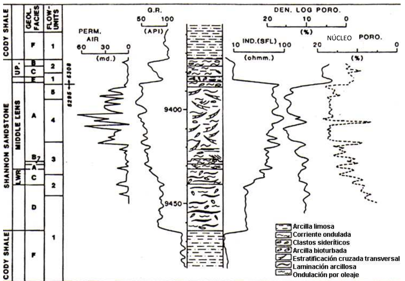
Figura 4.19 Perfil de propiedades geológicas y petrofísicas del yacimiento 8
