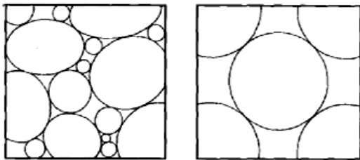
Figura 3.27 Un sedimento bien clasificado (derecha), tendrá mejor porosidad y permeabilidad que un sedimento pobremente clasificado (izquierda). En este último, los espacios entre granos son invadidos por sedimentos finos, disminuyendo la porosidad. La fábrica heterogénea disminuye la permeabilidad e incrementa la tortuosidad del sistema de poros 4 .
