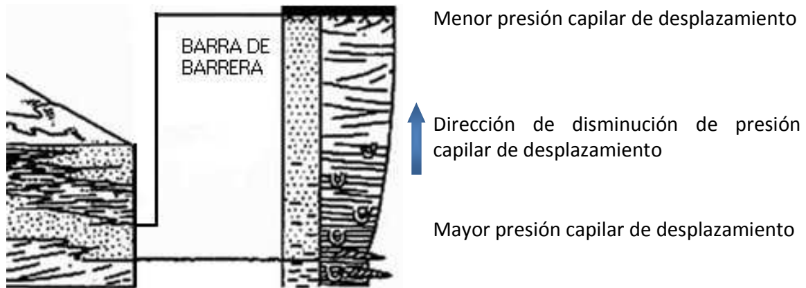
Figura 4.16 Distribución de presión capilar de desplazamiento en barras de barrera 2
