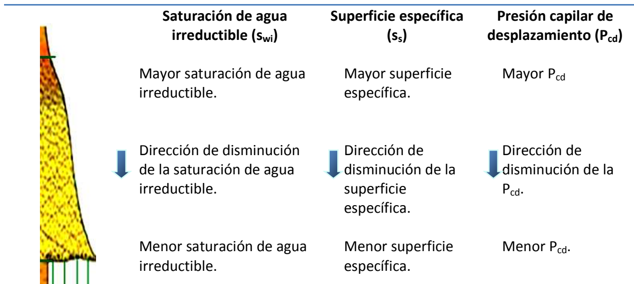
Figura 3.30 Distribución de saturación de agua irreductible ( s_{wi} ), superficie específica ( s_s ) y presión capilar de desplazamiento ( p_{cd} )
