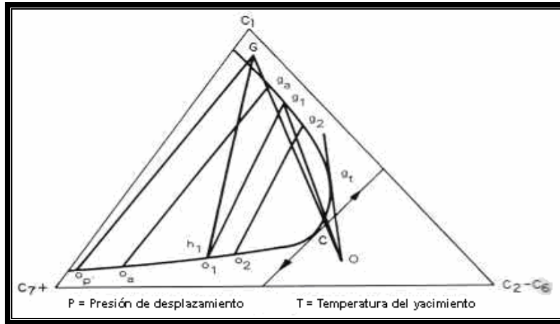
Figura 3.4 Esquematación de miscibilidad en un diagrama ternario
