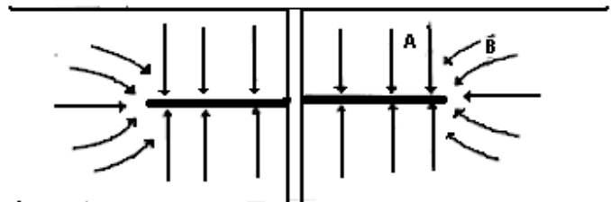
Figura 3.4 Distribución del flujo en una formación fracturada.
