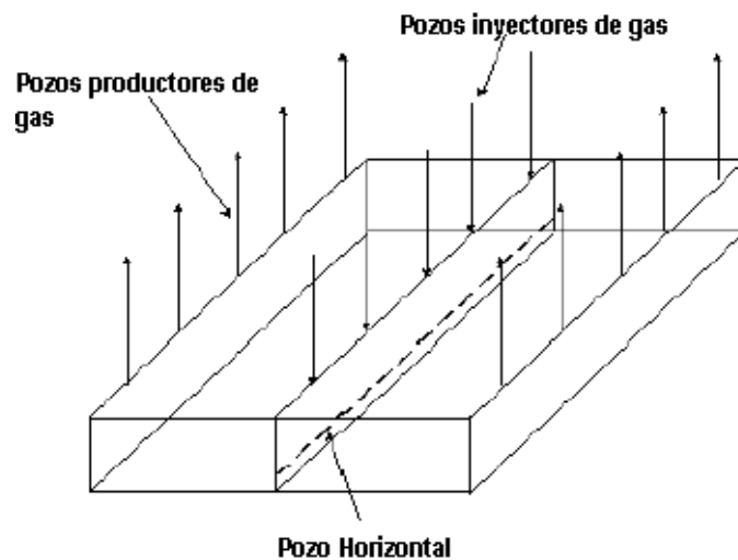
Figura 2.18 Disposición de los pozos en el proceso COSH.
