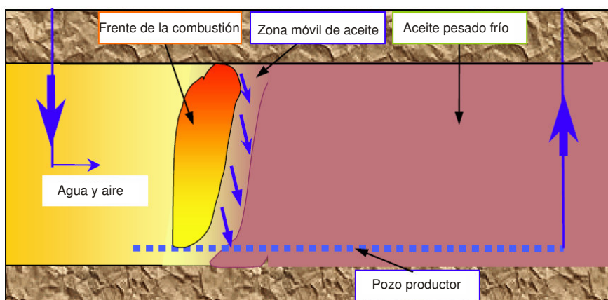
Figura 2.16 Proceso TTHW.
