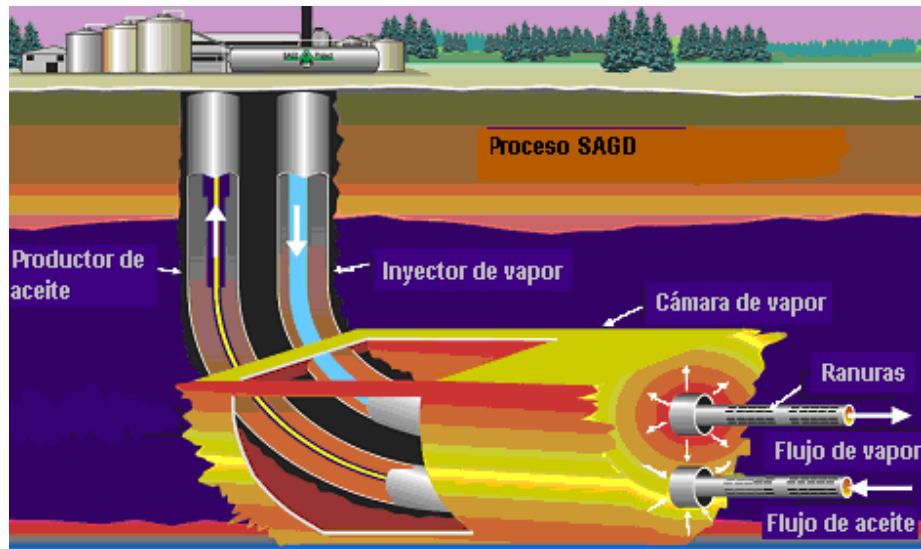
Figura 2.4 Proceso SAGD.
