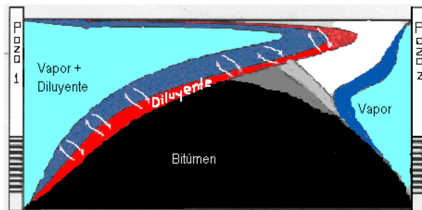
Figura 2.9 Proceso LASER.
