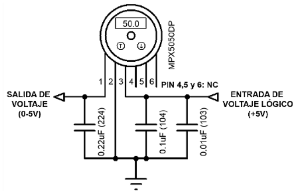
Fig. 24: Diagrama de conexión del sensor MPX5050DP.
