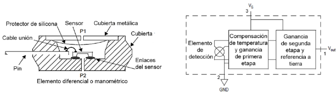
Fig. 23: Estructura física y diagrama de bloques interno del sensor MPX5050DP.
