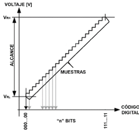
Fig. 34: Representación de la curva generada por un convertidor A/D. [41]
