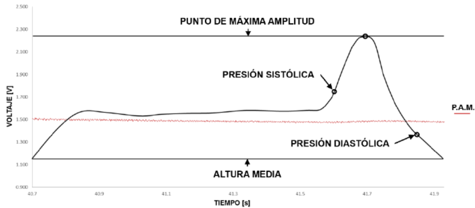
Fig. 45: Envolvente de la señal oscilométrica del muslo en el punto de máxima amplitud.
