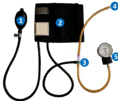
Fig. 25: Disposición de los elementos para la caracterización del sensor. 1: Pera de insuflado; 2: Manguito de hule recubierto de tela; 3: Válvula de tres vías; 4: Salida al sensor y 5: Manómetro aneroide.
