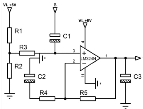
Fig. 29: Esquematzación del filtro para la detección de las oscilaciones. B : señal de voltaje a acondicionar. C : señal de voltaje acondicionada para ingresarse al convertidor A/D.
