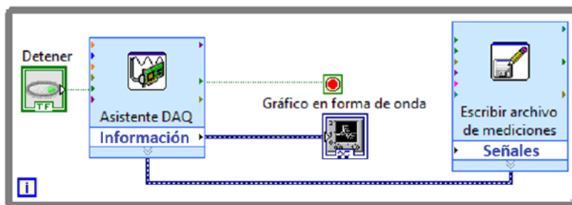
Fig. 37: Diagrama de bloques en LabView® para la interfaz de adquisición.
