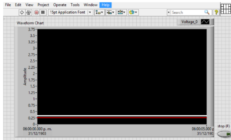
Fig. 38: Gráfico en tiempo real generado en LabView® cuando el dispositivo de detección de oscilaciones se mantiene en reposo. La línea roja representa la presión absoluta del sensor y la blanca a la señal de oscilación.
