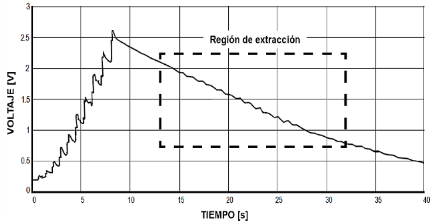
Fig. 32: Señal de presión en el manguito.
