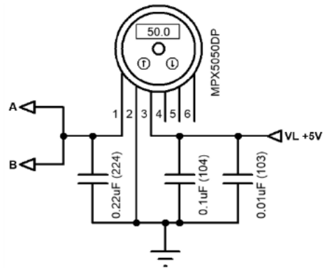
Fig. 28: Esquematzación de las señales de salida del sensor. A : señal de voltaje que puede ingresarse al convertidor A/D. B : señal de voltaje previa a acondicionamiento.
