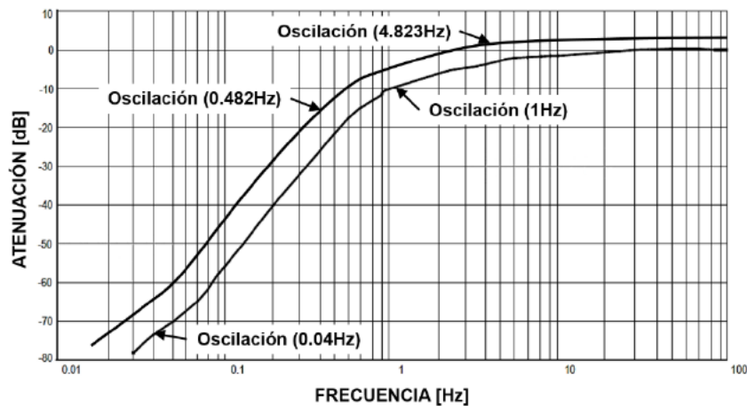
Fig. 30: Respuesta en frecuencia del filtro para la detección de oscilaciones.
