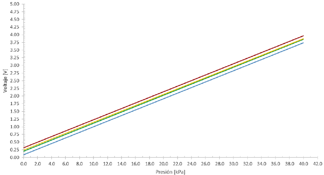
Fig. 27: Caracterización de la señal de salida. Rojo: voltaje máximo; azul: voltaje mínimo; verde: voltaje típico establecido por el fabricante; amarillo: voltaje real.
