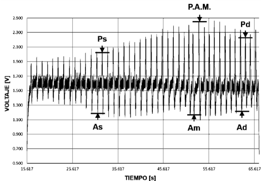
Fig. 44: Señal oscilométrica del muslo.
