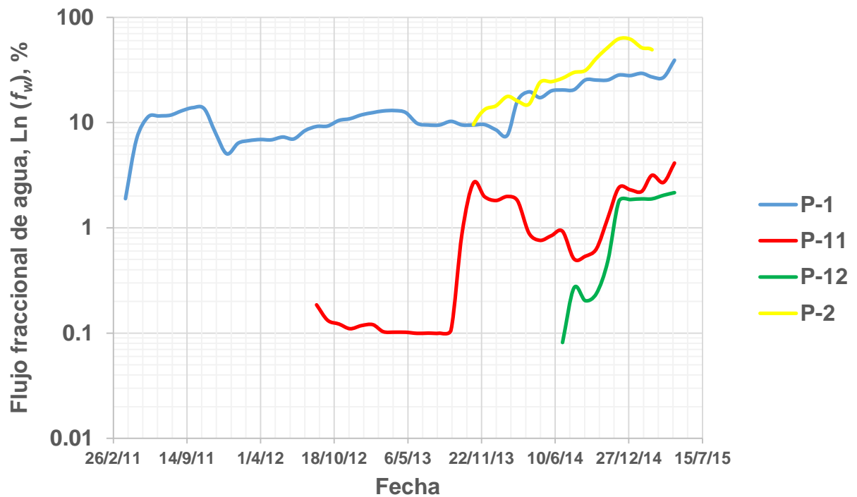
Figura 5.16. Logaritmo natural del flujo fraccional de agua ( \ln f_w ) del campo B.
