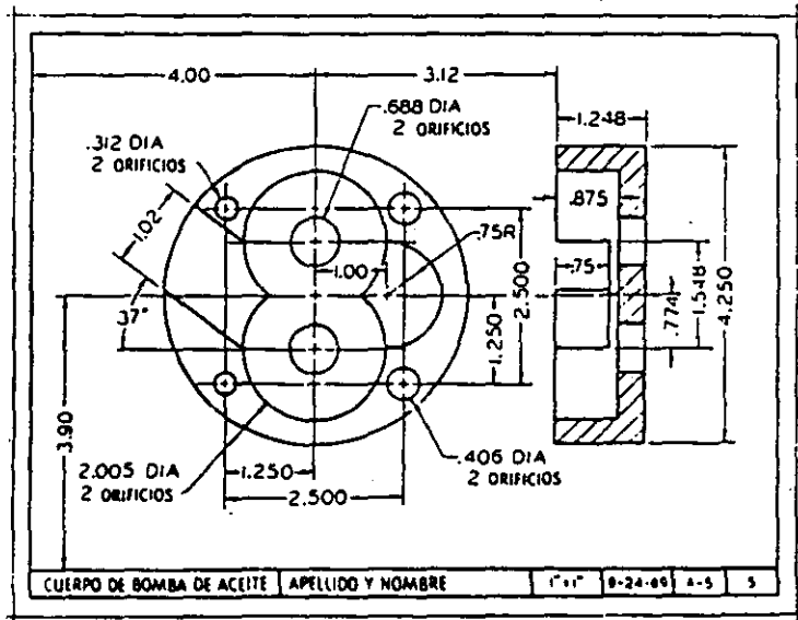
Fig. 2.88 Usando el plan A-2, trace vistas, a lápiz, tal como se muestra aquí. Use el lápiz de arco o ajuste para todos los arcos o círculos posibles dentro de los límites de su radio. Omita todas las dimensiones.
