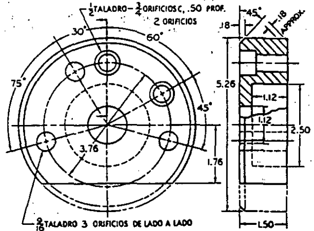
Fig. 2.90 Cubretapa. Usando el plan A-2, dibuje estas vistas a lápiz. Omite dimensiones y notas. Ver §7.8.
