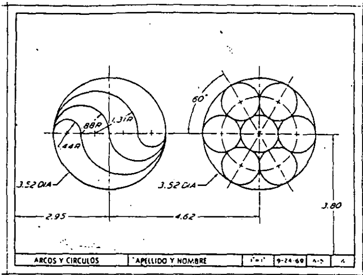
Fig. 2.87 Empleando el plan A-2, trace figuras a lápiz, como se muestra aquí. Use el lápiz de arco o ajuste para todos los arcos y círculos posibles dentro de los límites de su radio. Omita todas las dimensiones.
