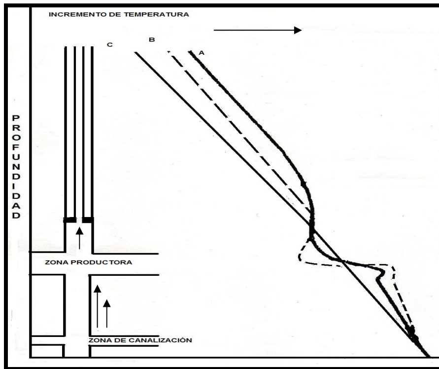
Fig. 4.3. Canalización de agua debajo de la zona productora.
