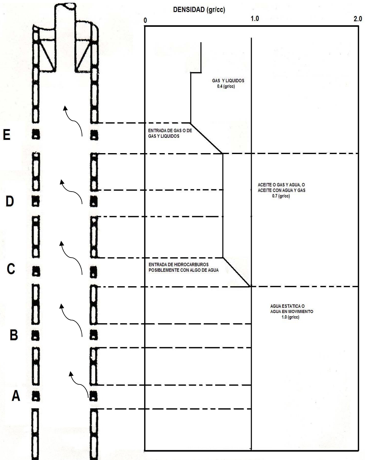
Fig. 4.8 Registro teórico del gradiomanómetro.
