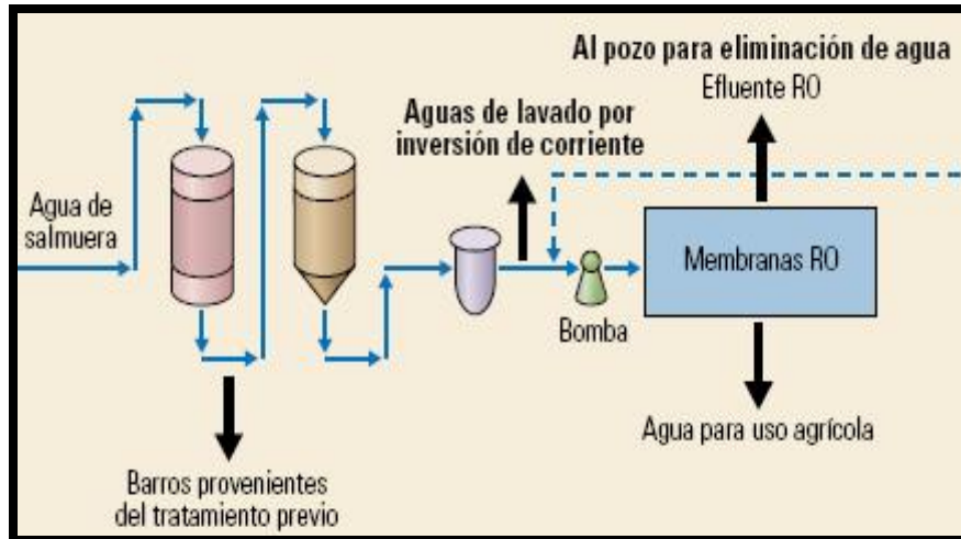
Fig. 3.3 Proceso para la eliminación de sales y contaminantes del agua producida.
