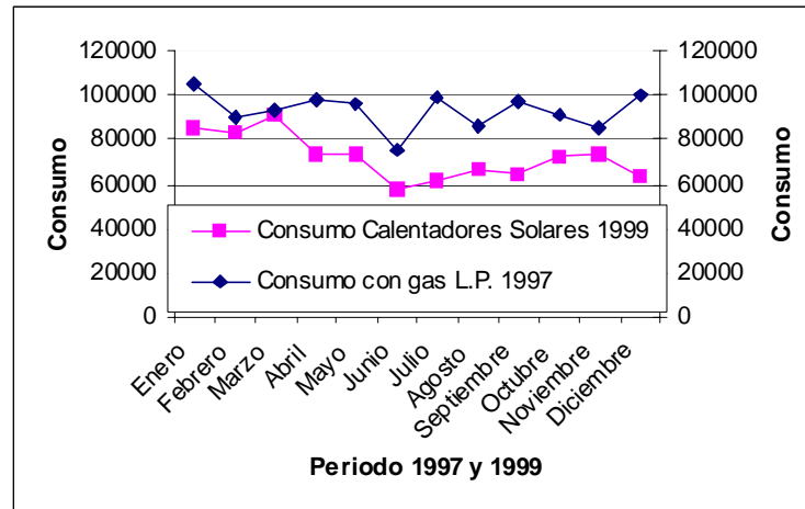
Gráfica 10 Comparativa del consumo de combustible antes y después del sistema solar
