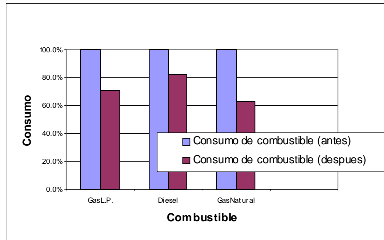
Gráfica 3 Consumo por tipo de combustible, antes y después de la instalación solar
