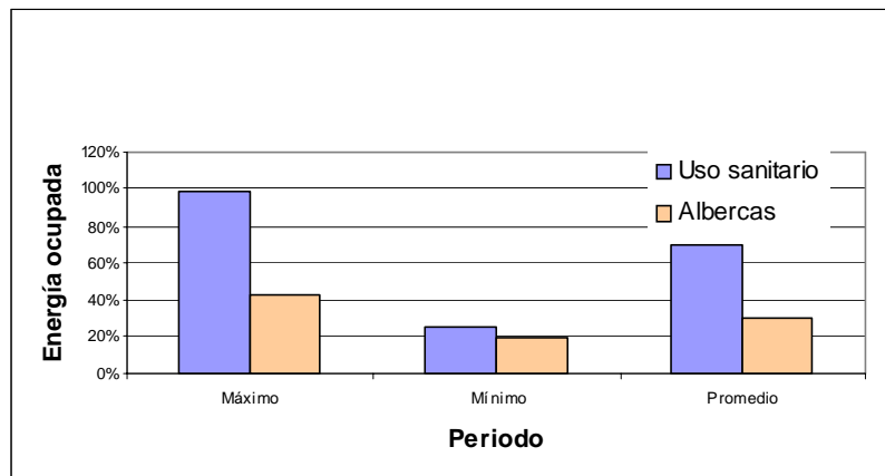
Gráfica 4 Porcentaje de uso de los colectores solares con referencia a la energía total ocupada
