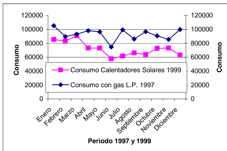
Gráfica 3 Comparativa del consumo de combustible antes y después del sistema solar
