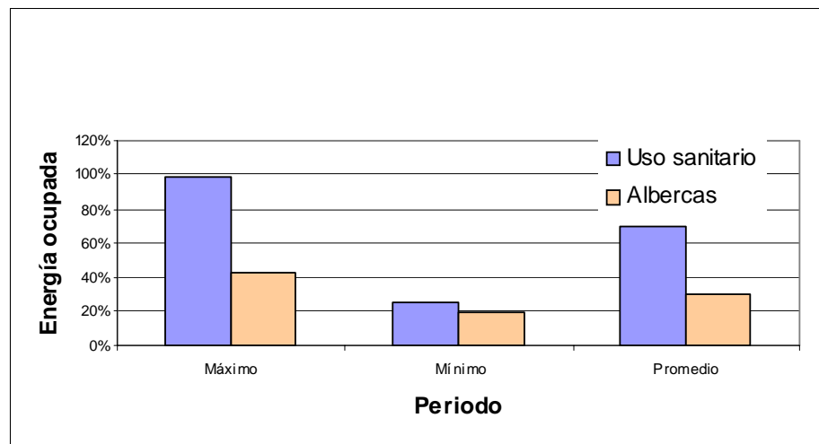
Gráfica 9 Porcentaje de uso de los colectores solares con referencia a la energía total ocupada
