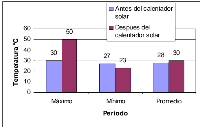
Gráfica 5 Temperatura del agua en albercas
