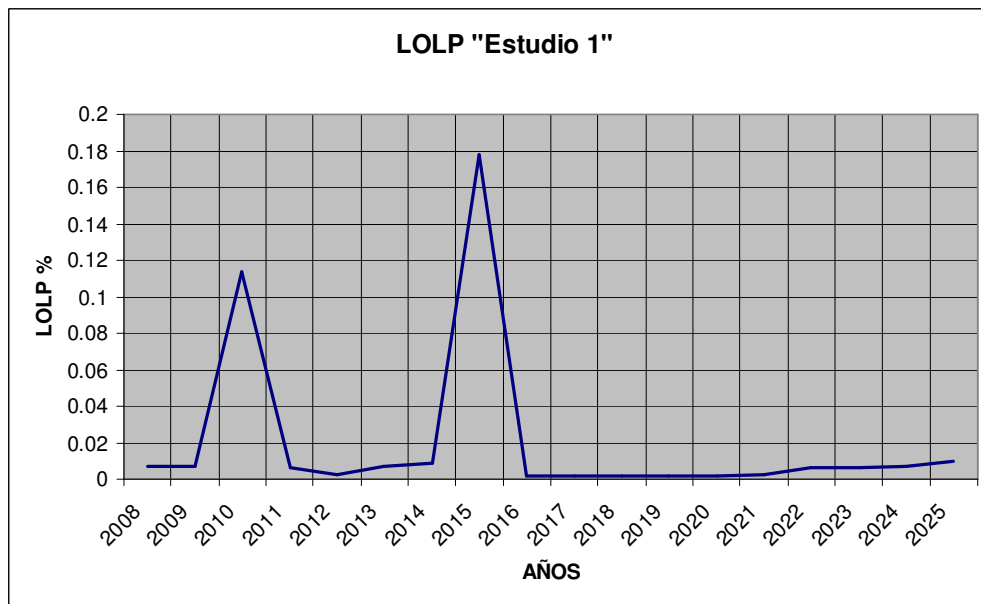
Gráfica 7.1.9 LOLP
