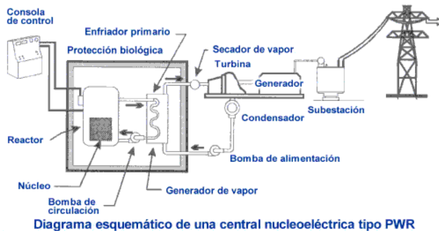
Figura 1.7.3.1 Central nucleoelectrica con reactor de agua a presión
