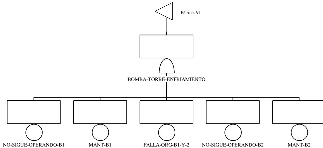
Figura 4.7. Falla de las bombas de la torre de enfriamiento.
