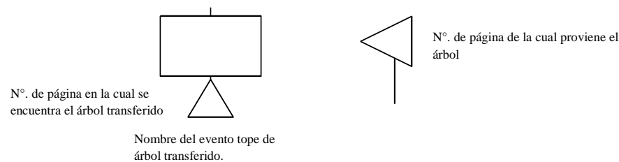
Figura 4.3. Simbología para transferencia de árboles de fallas.
