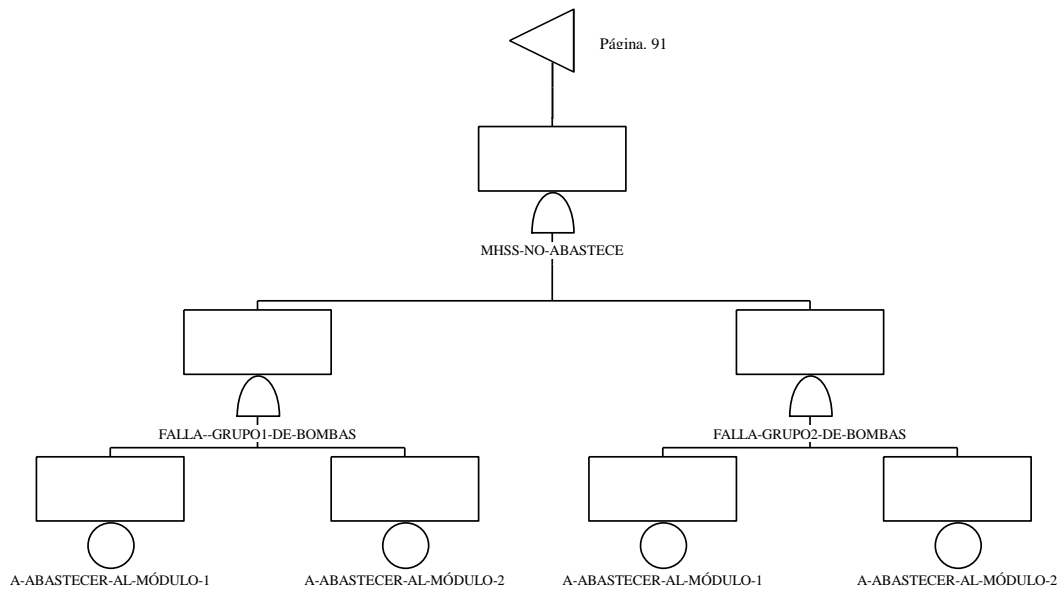
Figura 4.9. Falla a abastecer ambos módulos del MHSS.
