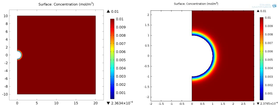
Figura 3.7 a) Concentration c1 b) Concentration c1 acercamiento P1_EDL.mph (Dimensiones en [\mu\text{m}] . Gráfico de colores en [\text{mol}/\text{m}^3] )
