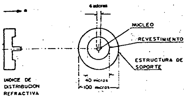
FIBRA OPTICA UNIMODO
