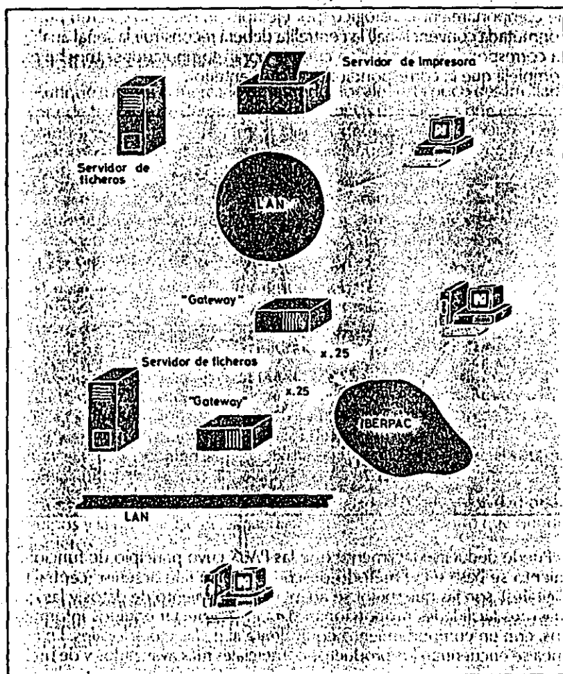
Figura 17. Servidores (servers) y pasarelas (gateways) en dos redes locales conectadas a través de una red de conmutación de paquetes.
