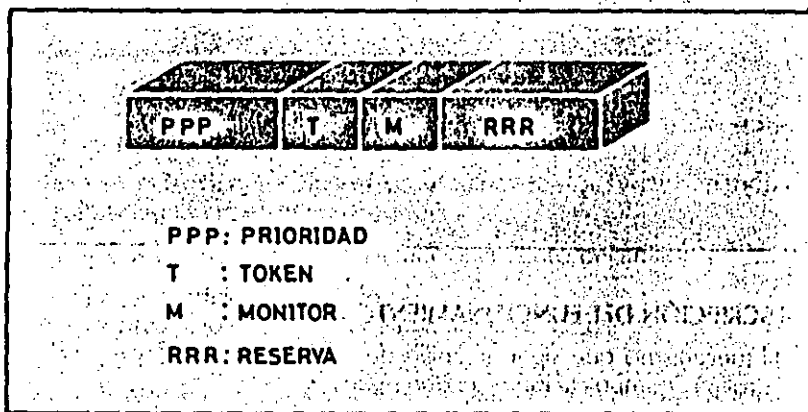
Figura 52. Formato del campo de Control de Acceso (AC).
