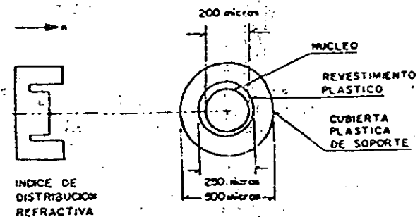
FIBRA OPTICA CON REVESTIMIENTO PLASTICO
