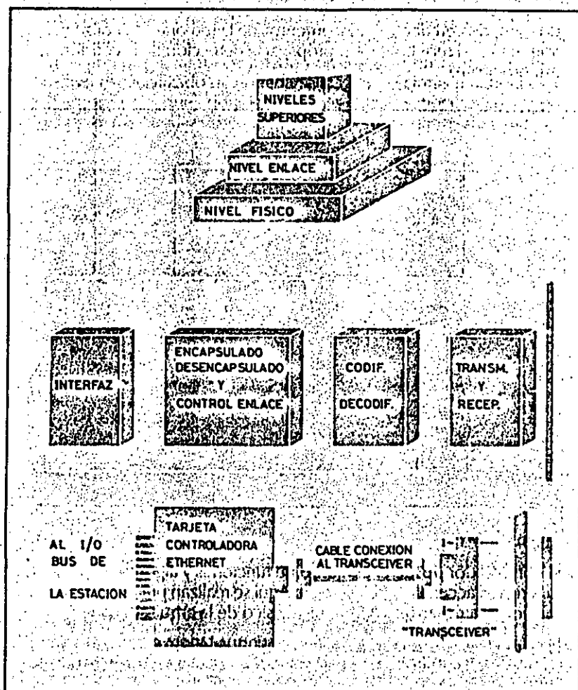
Figura 31. Equivalencia entre niveles de la arquitectura, funciones y componentes de la red Ethernet.
