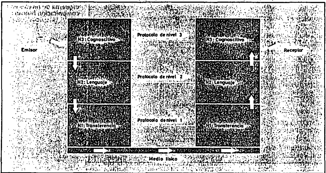
Figura 20. El mismo esquema anterior representando comunicaciones de pares entre niveles, homólogos y comunicaciones internas (servicios) entre niveles consecutivos de cada "estación".
