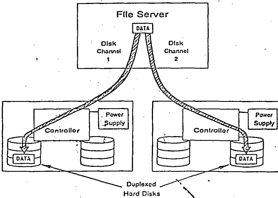
Fig. 12 Disk Duplexing
