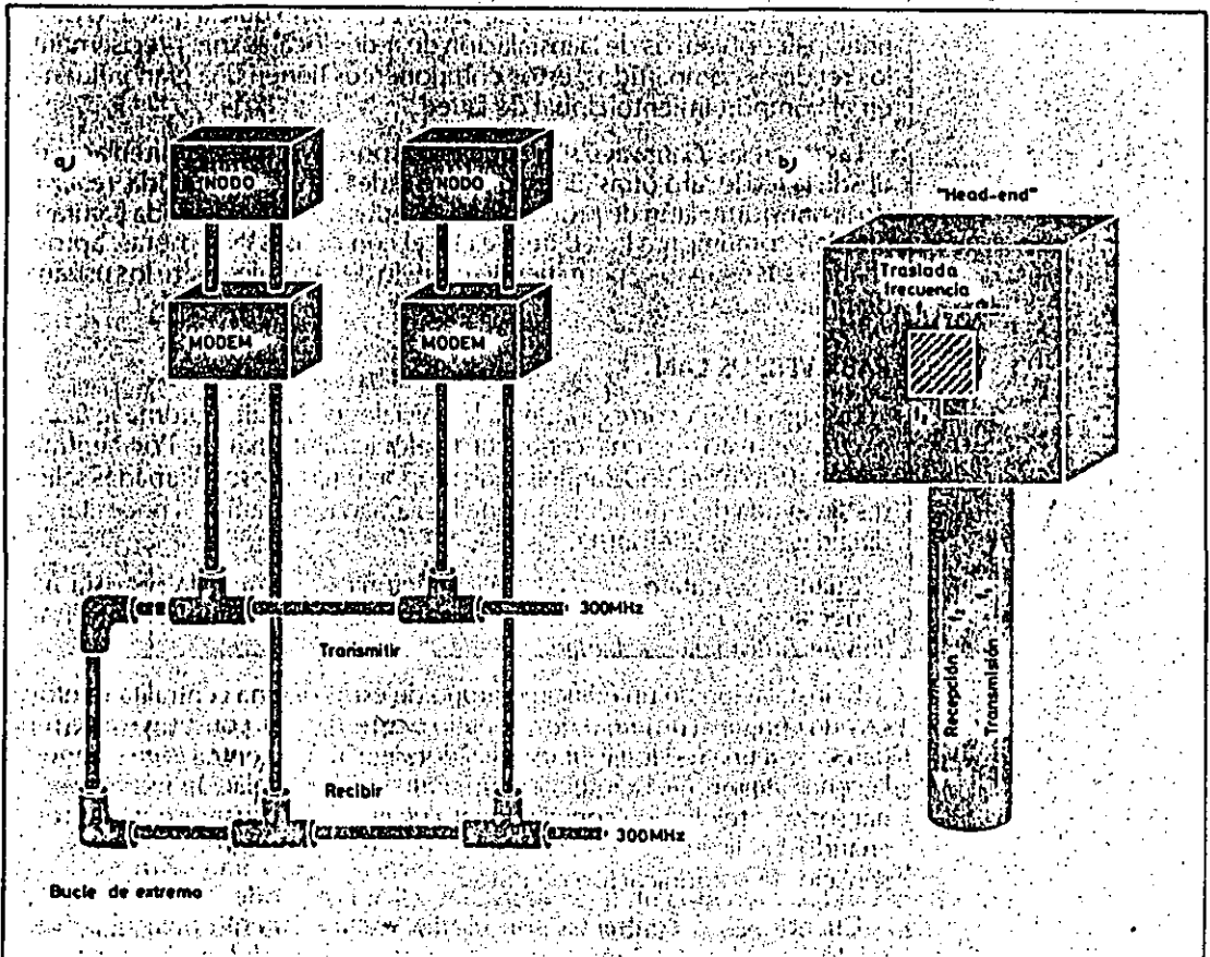
Figura 16. a) Sistema de banda ancha usando un cable para la transmisión y otro para la recepción. b) Sistema usando un cable único.
