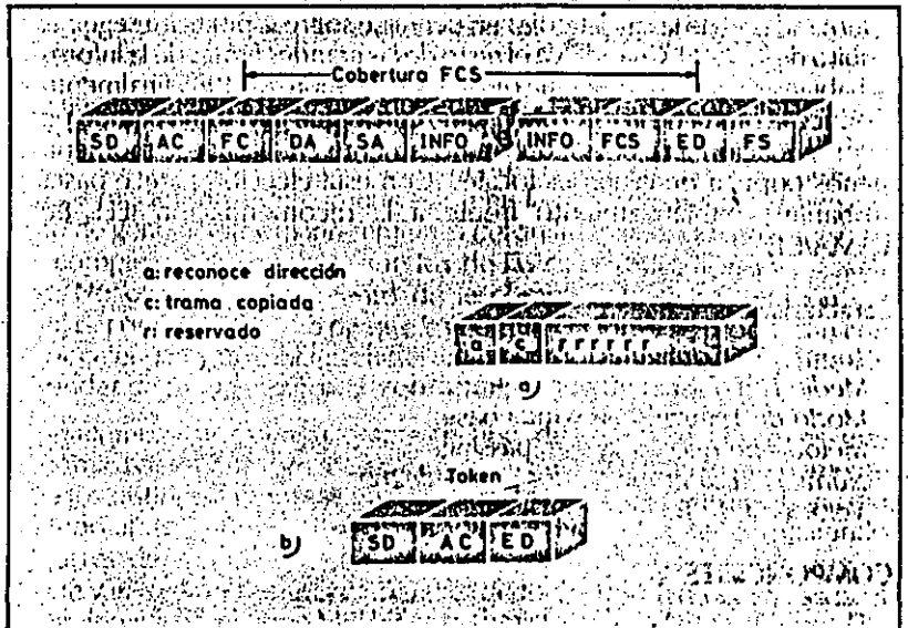
Figura 51. Formato de la trama de datos y token en la red en anillo.
