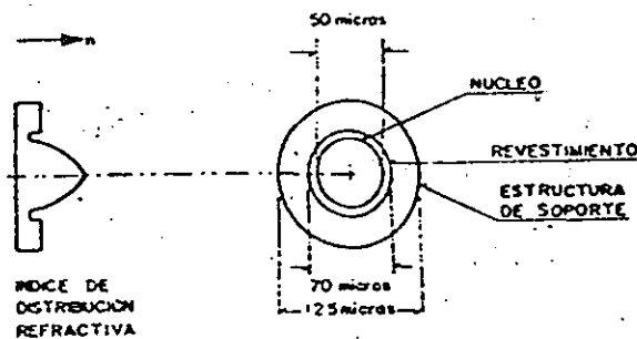
FIBRA OPTICA DE INDICE GRADUAL
