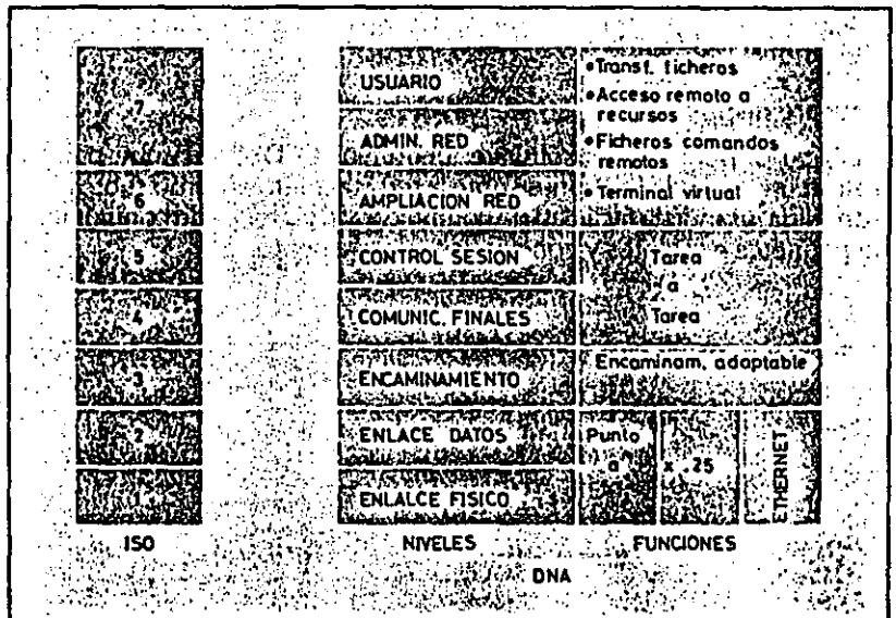
Figura 38. Paralelismo entre la división de niveles ISO y los propuestos en la arquitectura DNA.
