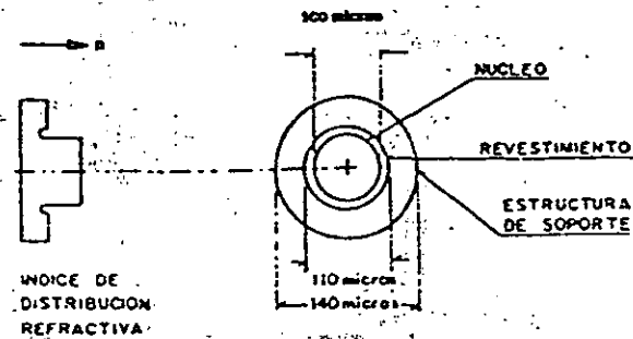
FIBRA DE INDICE ESCALONADO
