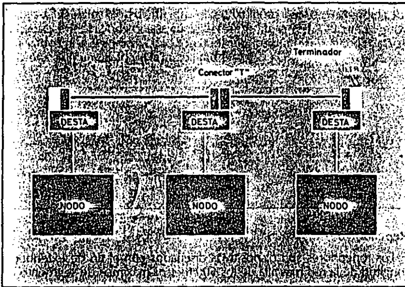
Figura 33. Conexión de nodos en una red Ethernet tipo "Thin Wire".
