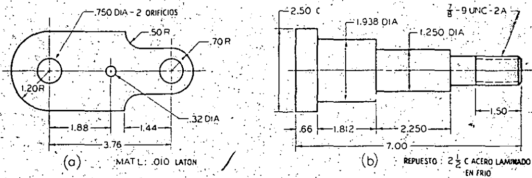
Fig. 5.42 Dibujos de una sola vista.
