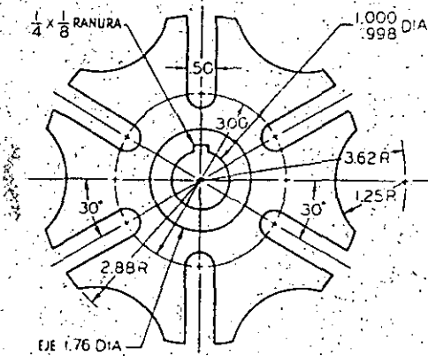
Fig. 2.91 Eje de levas tipo Ginebra. Empleando el plan A-2, dibuje a lápiz. Omite las dimensiones y las notas.
