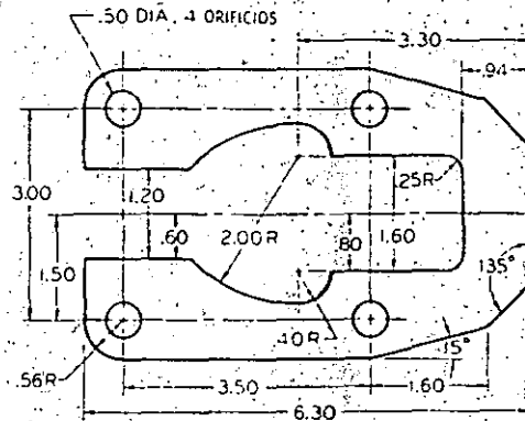
Fig. 2.94 Placa para cerradura. Usando el plan A-2, dibuje a lápiz. Omite dimensiones y notas.
