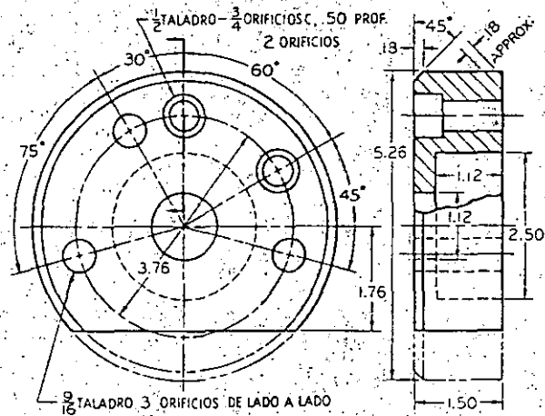
Fig. 2.90 Cubretapa. Usando el plan A-2, dibuje estas vistas a lápiz. Omite dimensiones y notas. Ver §7.8.
